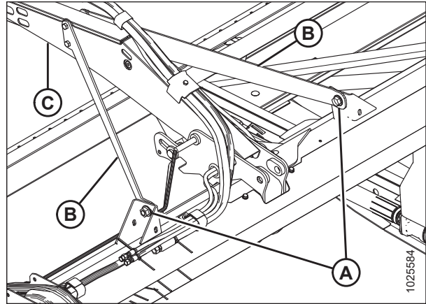
Рисунок 5.157: Центральный опорный рычаг мотовила
