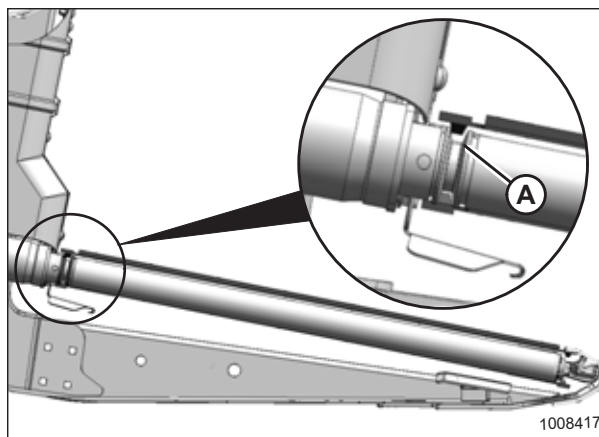
Рисунок 5.108: Приводной ролик
