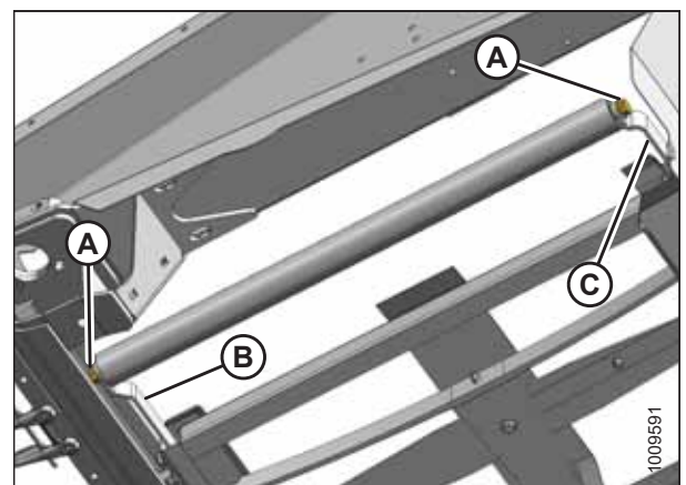
Рисунок 5.123: Натяжной ролик
