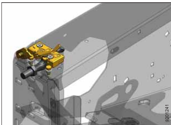
Рисунок 6.11: Защелка делителя
