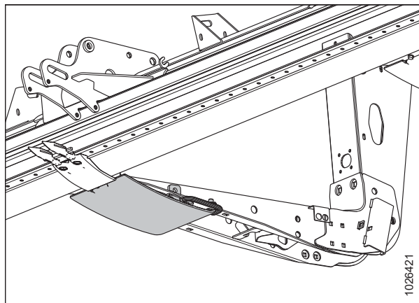
Рисунок 6.15: Центральный копирующий башмак — показана внутренняя сторона, внешняя аналогична
