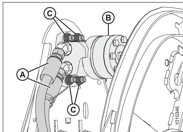
Рисунок 5.225: Мотор и шланги подбирающего мотовила
