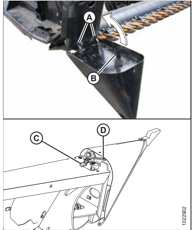
Рисунок 3.60: Делитель
