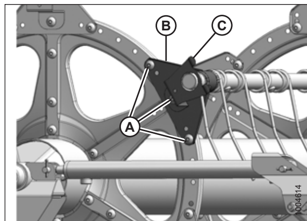
Рисунок 5.166: Хвостовик
