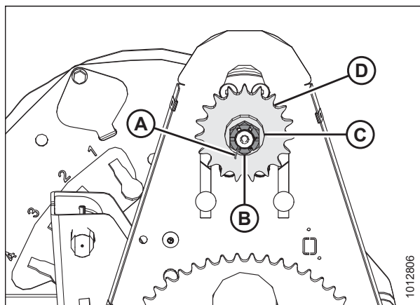
Рисунок 5.218: Привод мотовила
