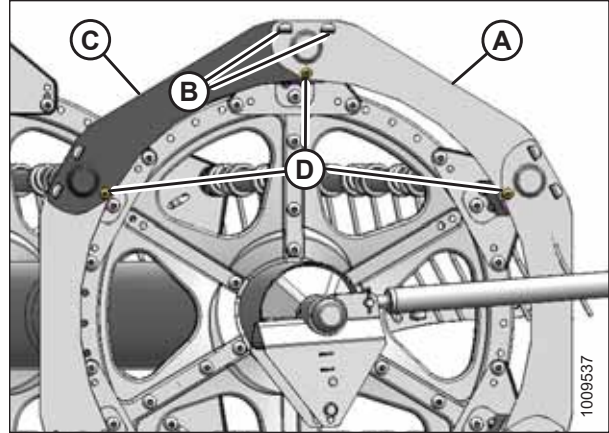
Рисунок 5.201: Боковые щитки мотовила
