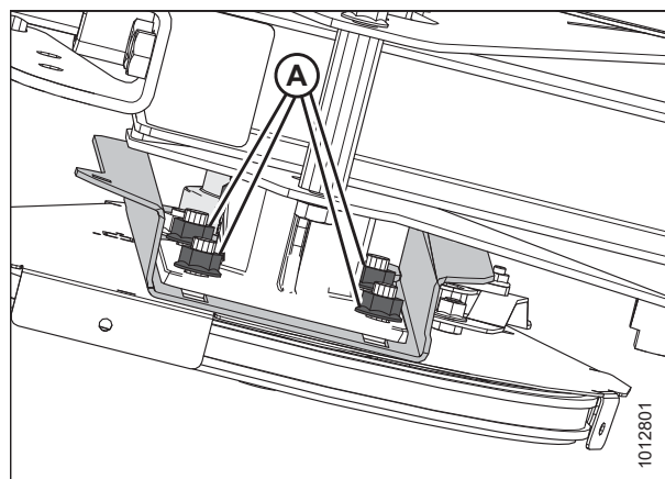
Рисунок 5.211: Привод одинарного мотовила — вид из-под низа мотовила
