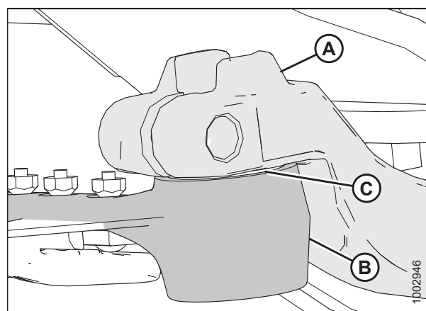
Рисунок 5.62: Головка ножа
