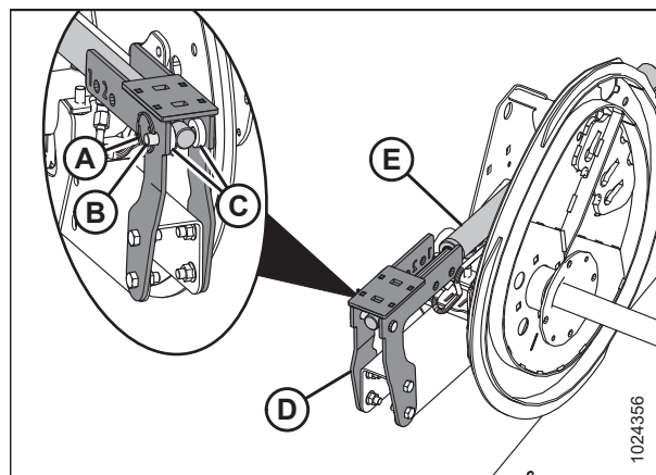
Рисунок 3.48: Правый рычаг мотвила в переднем положении
