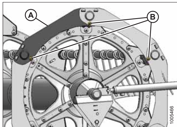
Рисунок 5.198: Боковые щитки подбирающего мотовила
