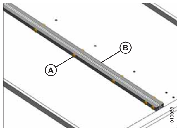
Рисунок 5.104: Стык полотна
