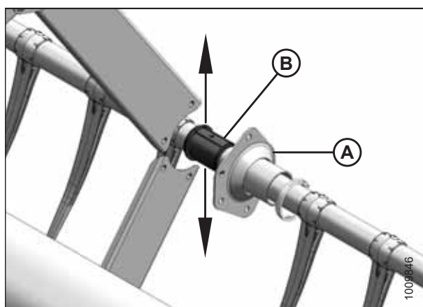
Рисунок 5.178: Опора
