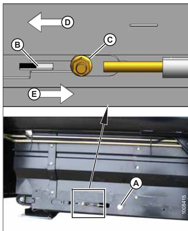
Рисунок 5.110: Натяжитель полотна
