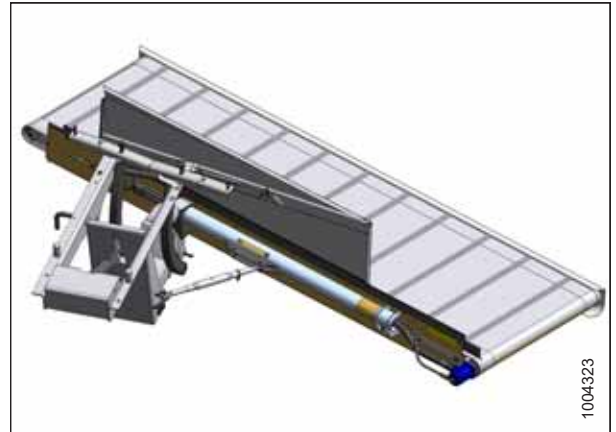
Рисунок 6.21: Навесное устройство для сдвигания валков
