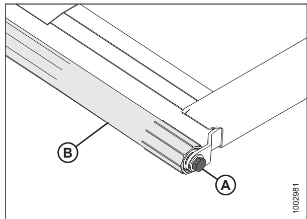
Рисунок 5.130: Приводной ролик
