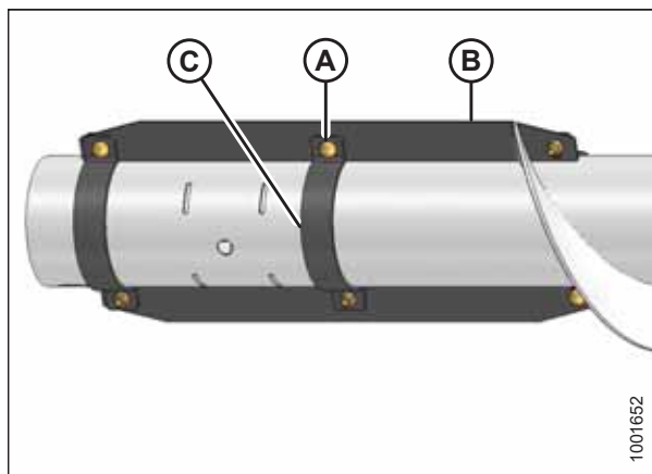
Рисунок 3.81: Молотильные планки
