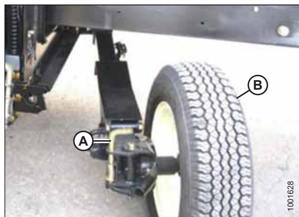
Рисунок 3.105: Правое заднее колесо
