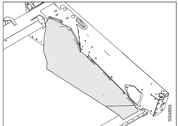
Рисунок 6.17: Широкий дефлектор полотна
