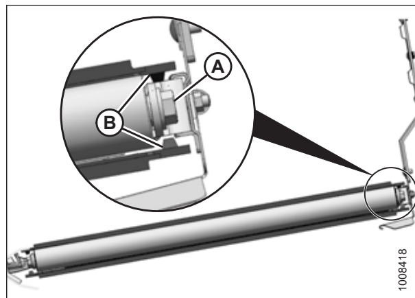
Рисунок 5.109: Натяжной ролик
