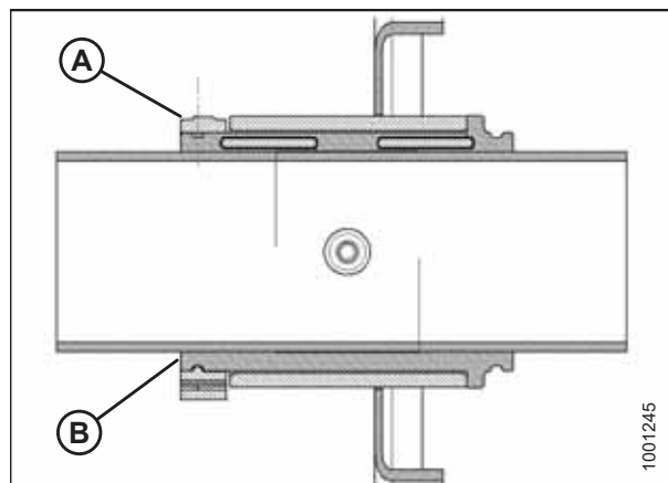
Рисунок 5.188: Втулка
