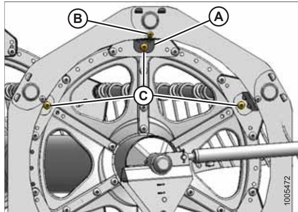
Рисунок 5.202: Опоры боковых щитков подбирающего мотовила
