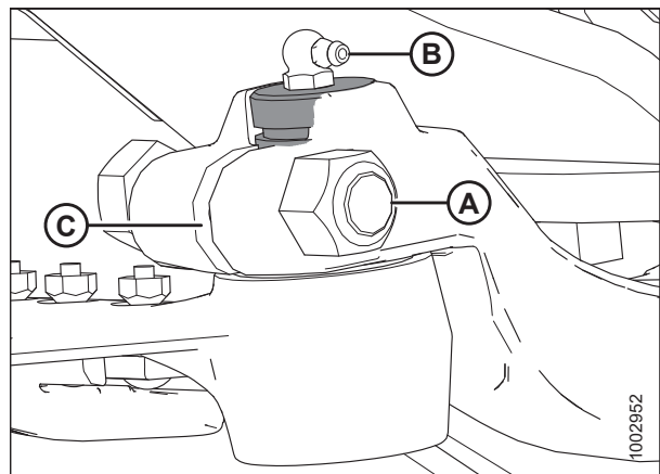
Рисунок 5.56: Головка ножа
