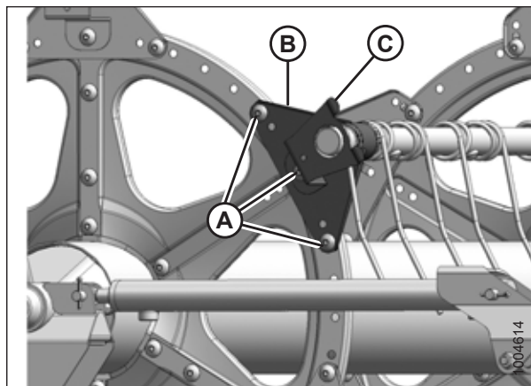
Рисунок 5.185: Хвостовик
