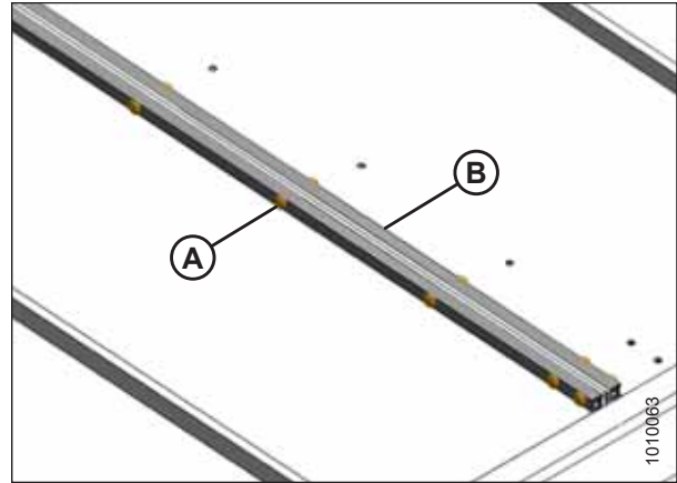
Рисунок 5.128: Стык полотна
