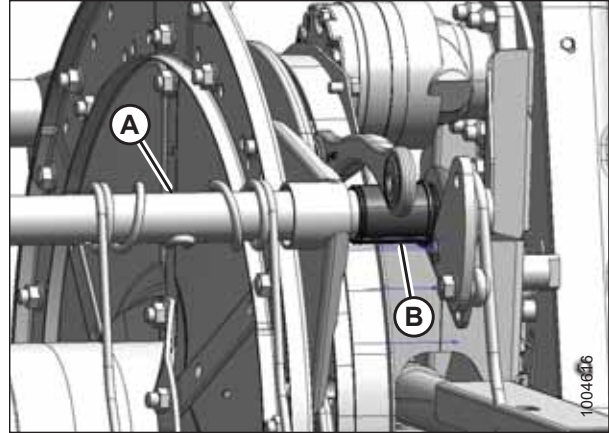
Рисунок 5.174: Сторона эксцентрика
