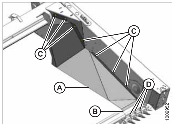
Рисунок 5.141: Широкий дефлектор
