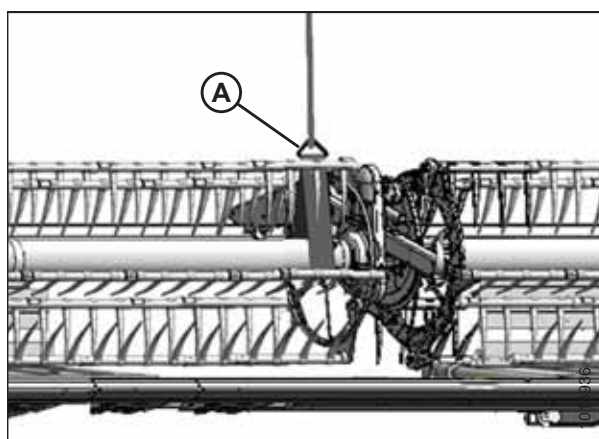
Рисунок 5.233: Вывешивание подбирающего мотовила
