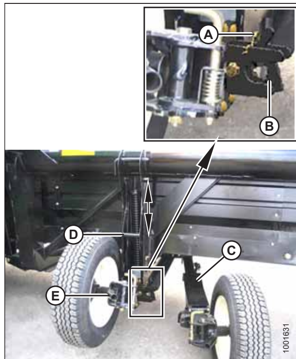
Рисунок 3.102: Разделение мостов
