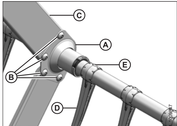
Рисунок 5.175: Опора граблины
