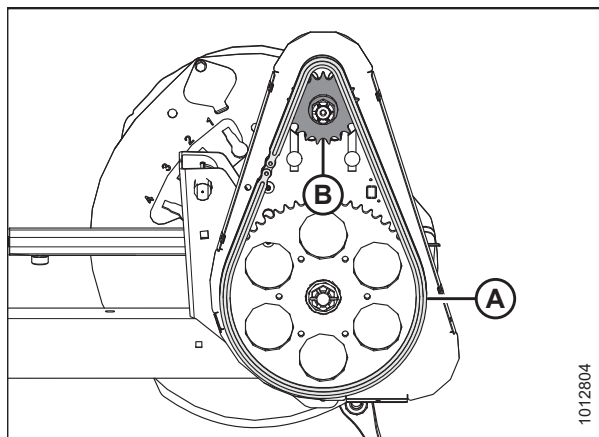
Рисунок 5.219: Привод мотовила
