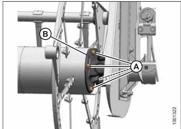
Рисунок 5.223: Карданный шарнир
