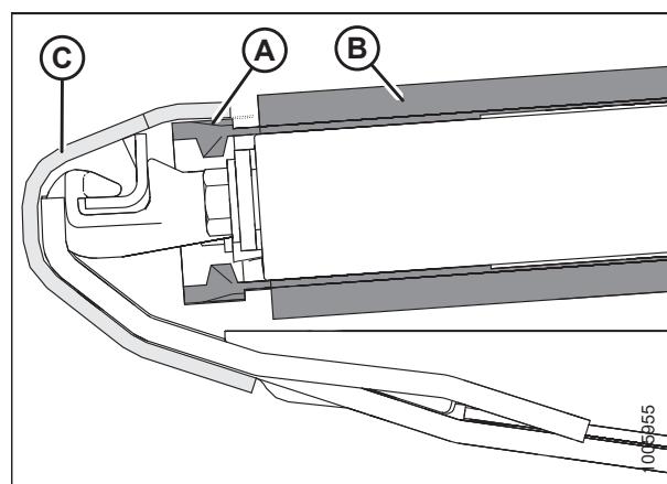
Рисунок 5.105: Уплотнение полотна
