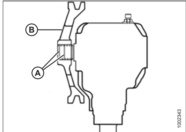
Рисунок 5.59: Редуктор привода ножа
