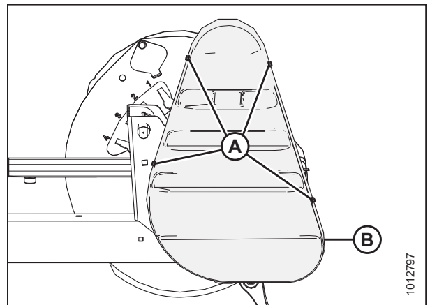
Рисунок 5.207: Крышка привода — единое мотовило
