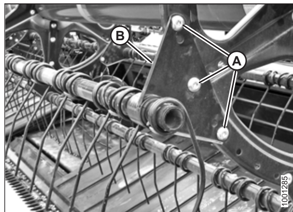
Рисунок 5.160: Кронштейн граблины
