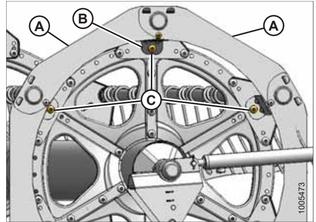
Рисунок 5.203: Опоры боковых щитков мотвила
