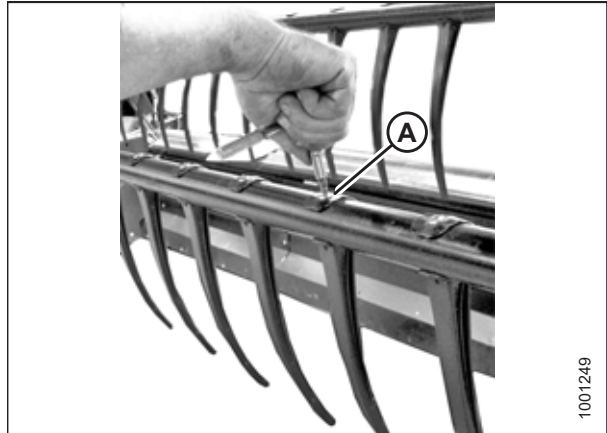
Рисунок 5.165: Установка пальца
