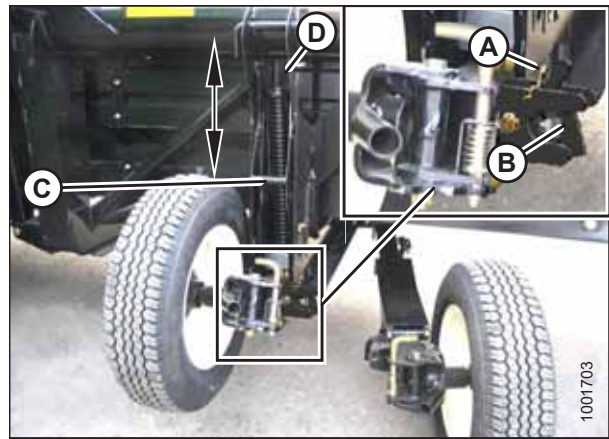
Рисунок 3.19: Правое колесо
