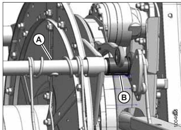
Рисунок 5.187: Сторона эксцентрика
