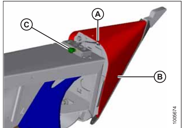
Рисунок 3.56: Делитель культуры
