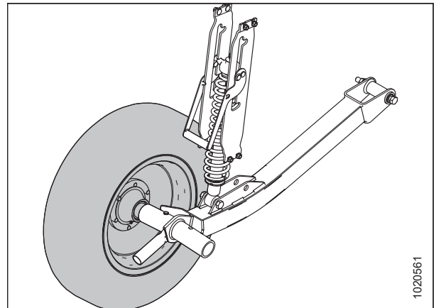
Рисунок 6.13: Вспомогательное стабилизирующее колесо
