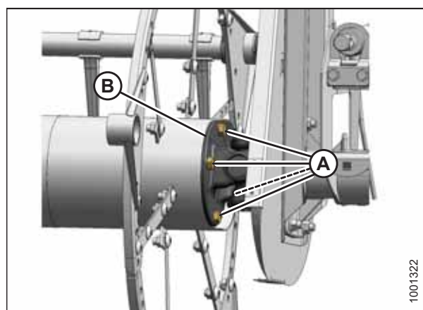
Рисунок 5.230: Карданный шарнир
