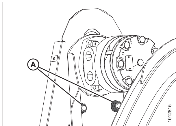
Рисунок 5.214: Изображен привод одинарного мотвила — привод сдвоенного мотвила имеет такую же конструкцию
