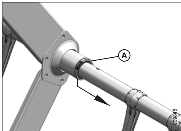
Рисунок 5.177: Хомут втулки
