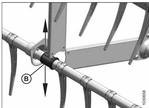
Рисунок 5.179: Противоположная опора
