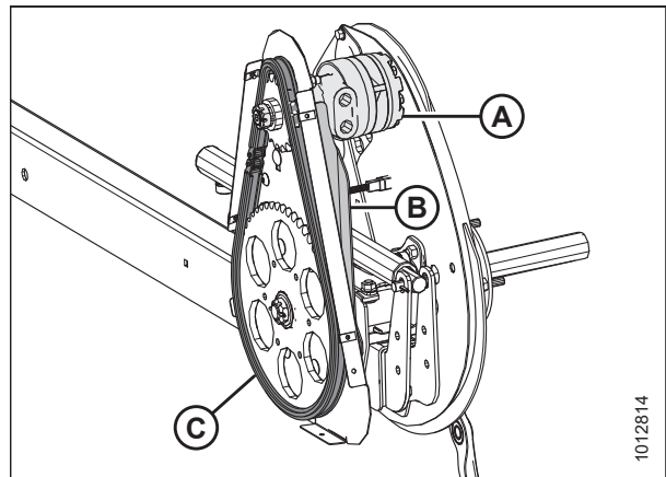
Рисунок 5.213: Изображен привод одинарного мотвила — привод сдвоенного мотвила имеет такую же конструкцию
