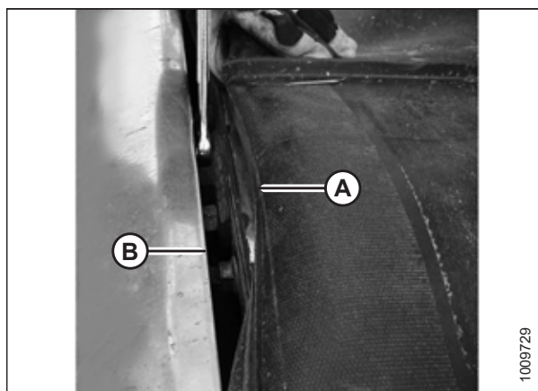
Рисунок 5.116: Регулировка деки
