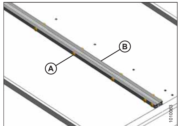
Рисунок 5.122: Стык полотна
