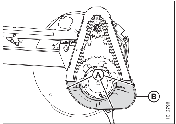
Рисунок 5.206: Крышка привода — сдвоенное мотовило
