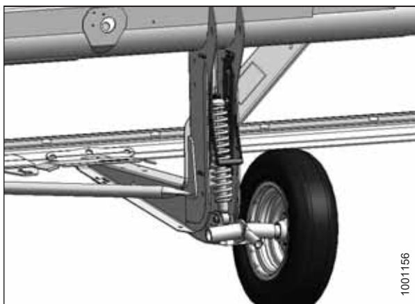
Рисунок 6.12: Стабилизирующее колесо
