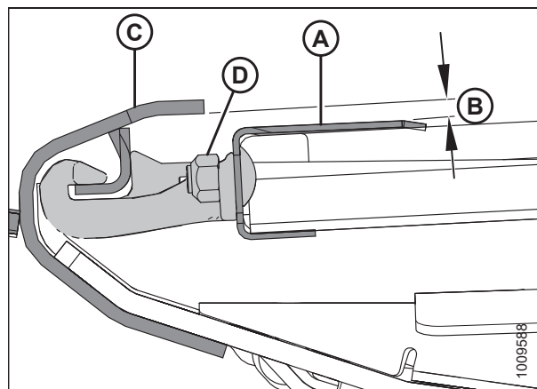
Рисунок 5.118: Опора деки
