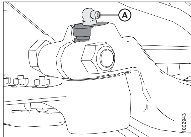
Рисунок 5.31: Головка ножа
