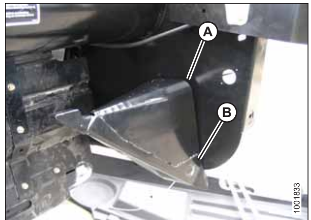
Рисунок 3.57: Делитель в отсеке для хранения
