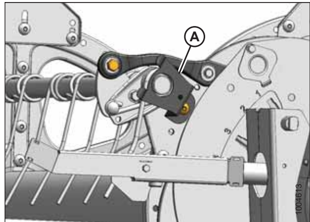
Рисунок 5.169: Сторона эксцентрика
