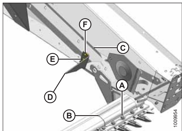
Рисунок 5.140: Опора дефлектора
