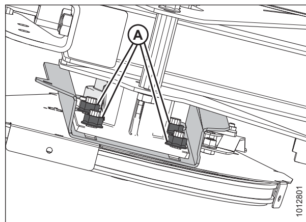
Рисунок 5.215: Привод одинарного мотовила — вид снизу мотовила
