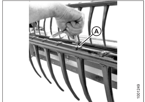
Рисунок 5.162: Снятие пластмассовых пальцев
