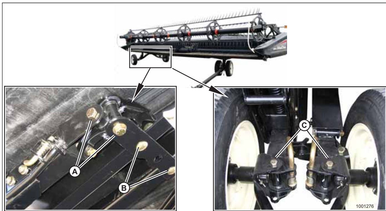
Рисунок 5.236: Болты моста
