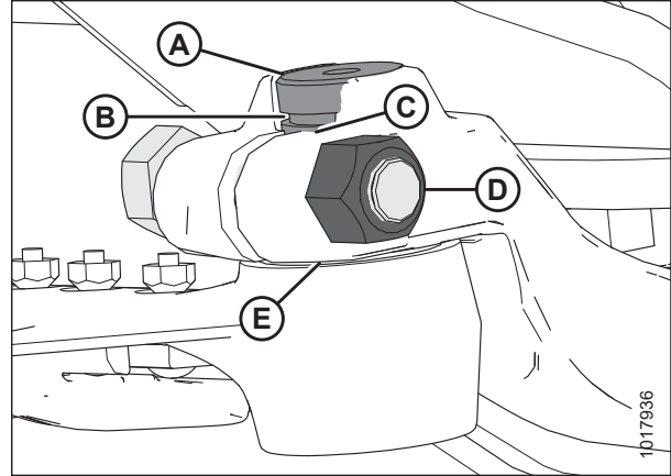
Рисунок 5.30: Головка ножа
