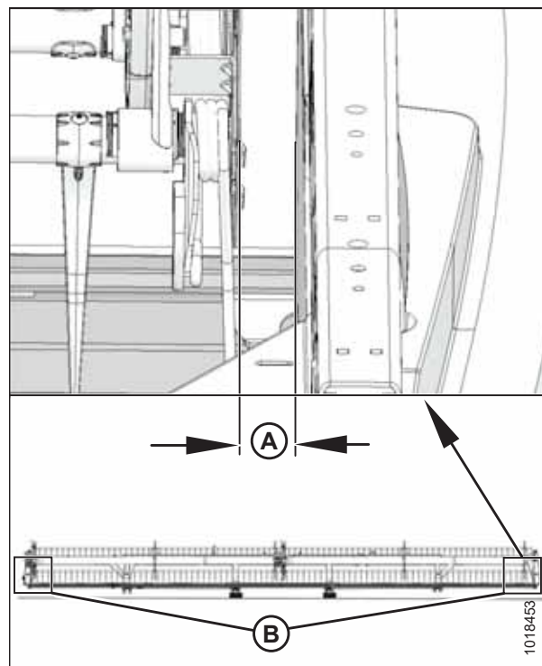
Рисунок 5.156: Центровка мотовила
