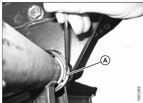
Рисунок 5.167: Хомут втулки
