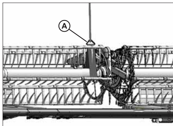
Рисунок 5.229: Вывешивание мотовила
