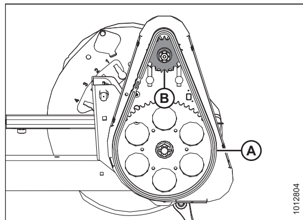
Рисунок 5.216: Привод мотовила
