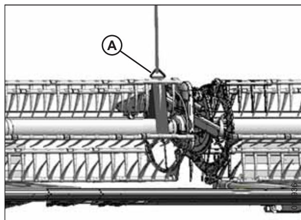
Рисунок 5.220: Вывешивание мотовила
