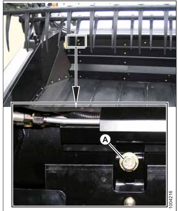
Рисунок 3.68: Механизм перемещения столов вручную
