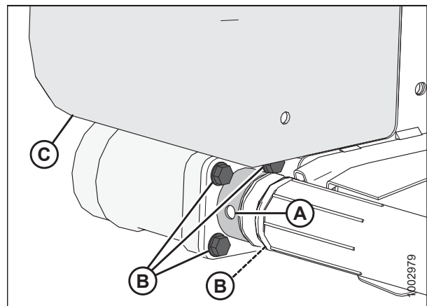
Рисунок 5.129: Приводной ролик
