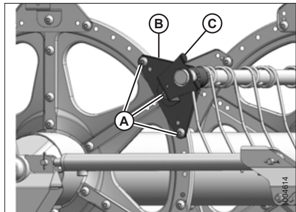
Рисунок 5.170: Хвостовик
