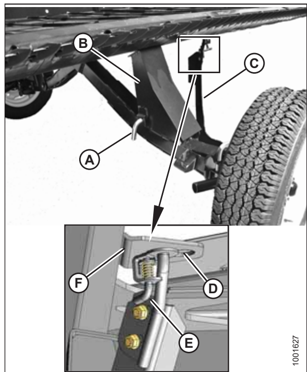
Рисунок 3.107: Положение заднего правого колеса
