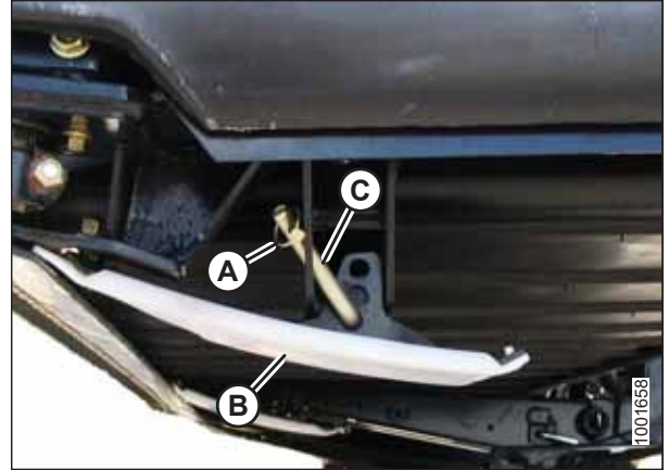
Рисунок 3.27: Внешний копирующий башмак
