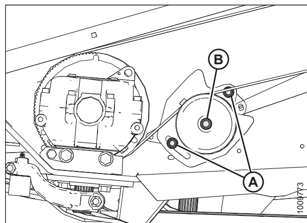
Рисунок 5.99: Привод ножа
