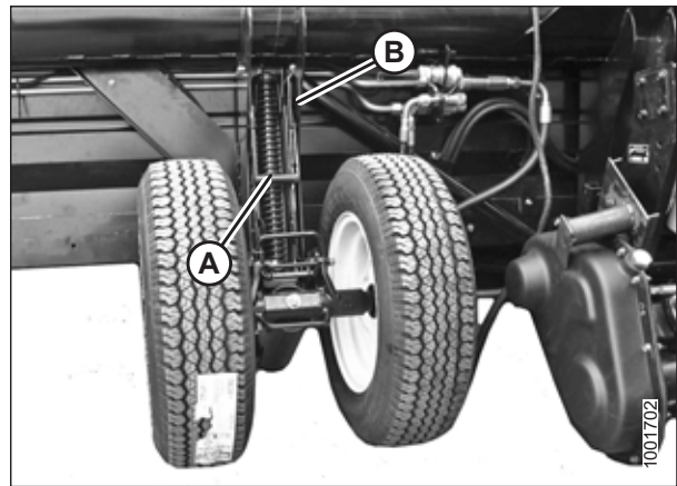
Рисунок 3.20: Левое колесо
