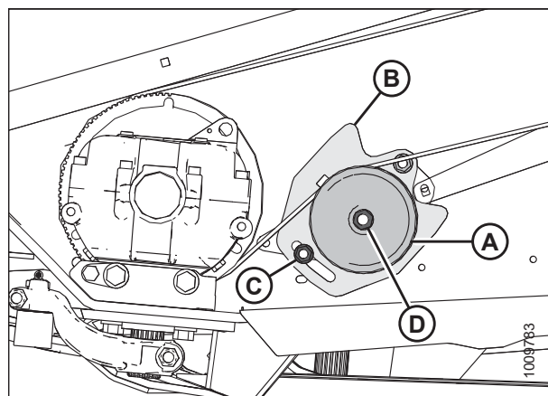
Рисунок 5.82: Привод ножа
