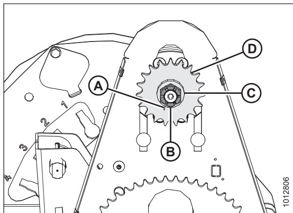
Рисунок 5.217: Привод мотовила
