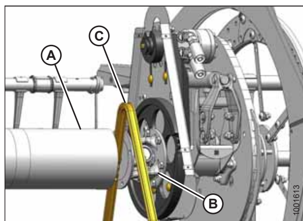
Рисунок 5.231: Замена цепи
