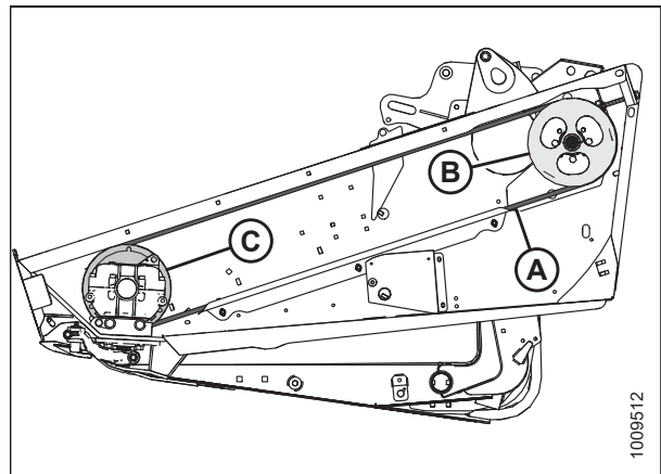
Рисунок 5.55: Привод ножа
