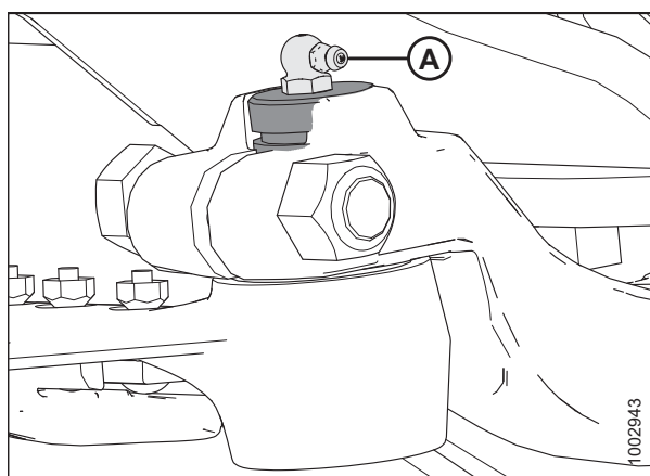
Рисунок 5.65: Головка ножа
