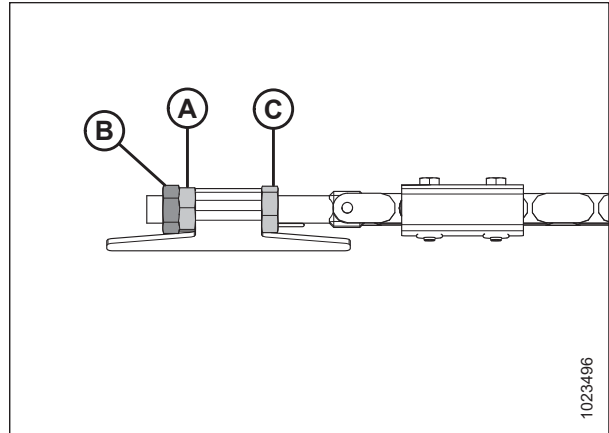
Рисунок 3.73: Болт регулировки цепи — показан левый, правый — аналогичный
