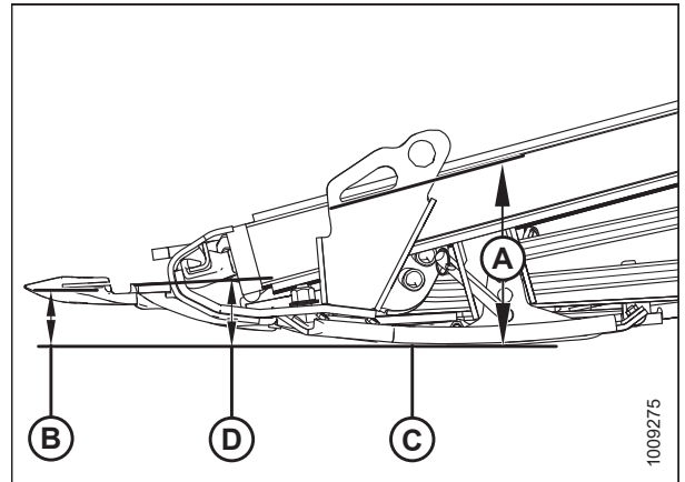
Рисунок 3.28: Угол атаки жатки
