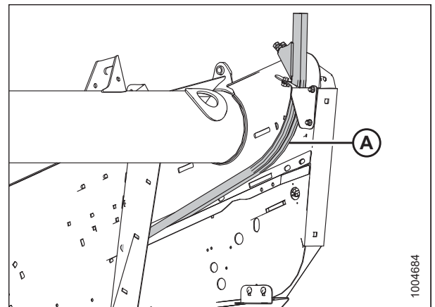
Рисунок 3.66: Правая боковина
