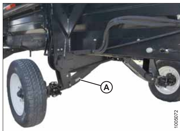
Рисунок 2: Опорно-транспортные/стабилизирующие колеса
