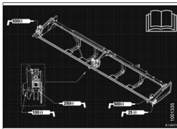
Рисунок 5.12: Наклейка с основными точками смазки на жатке с одинарным ножом
