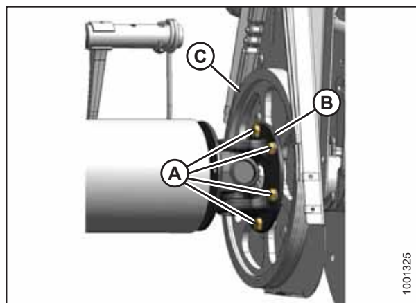
Рисунок 5.221: Карданный шарнир
