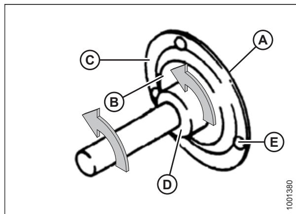
Рисунок 5.2: Герметизированный подшипник
