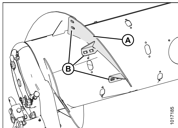
Рисунок 3.32: Средняя конфигурация (левая сторона)
