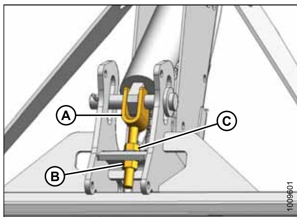
Рисунок 5.250: Нижняя сторона центрального рычага
