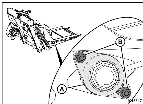
Рисунок 5.172: Подшипник приводного ролика
