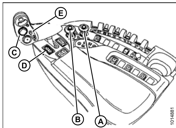
Рисунок 3.372: Органы управления комбайнов New Holland
