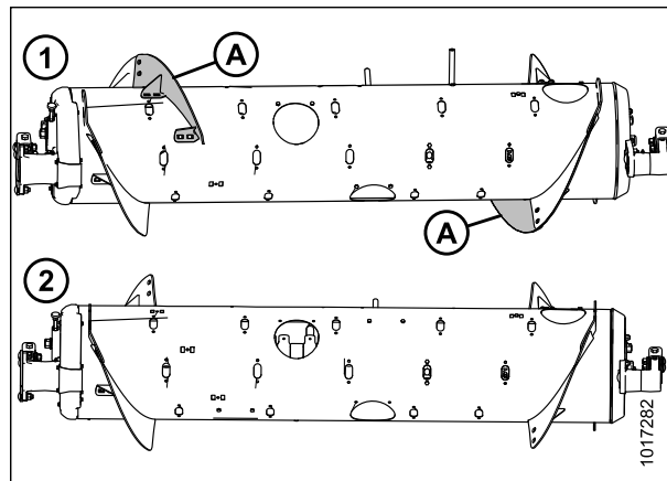
Рисунок 3.40: Конфигурации шнека (вид сзади)
