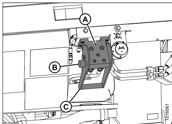
Рисунок 4.76: Гнездо модуля флотации
