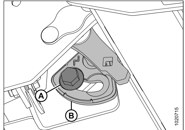
Рисунок 3.150: Рычаг регулировки флотации шнека — левая сторона
