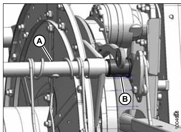
Рисунок 5.276: Сторона эксцентрика
