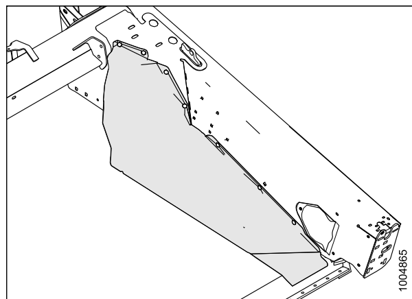
Рисунок 6.18: Дефлектор полотна (широкий)
