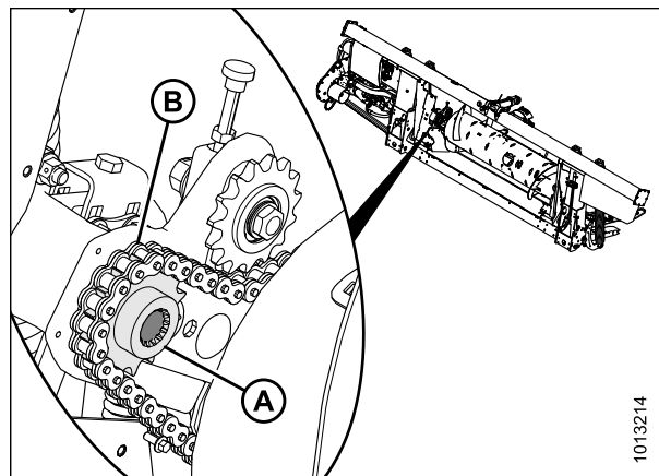
Рисунок 5.63: Привод шнека
