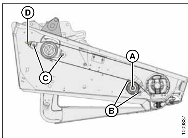
Рисунок 5.162: Привод ножа – правая сторона
