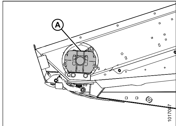
Рисунок 5.110: Показан левый редуктор привода ножа — правый аналогичен левому
