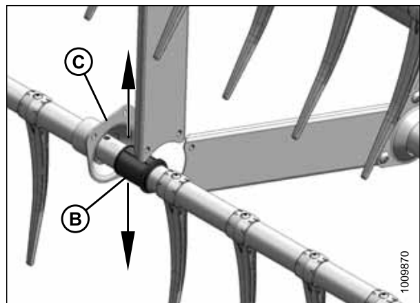
Рисунок 5.274: Противоположная опора
