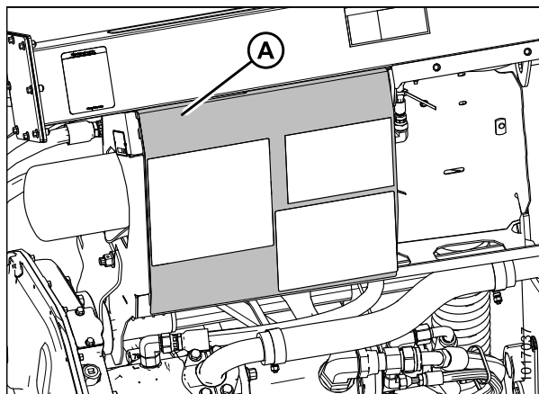
Рисунок 3.90: Крышка гидравлического распределителя
