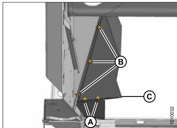
Рисунок 5.240: Задний дефлектор
