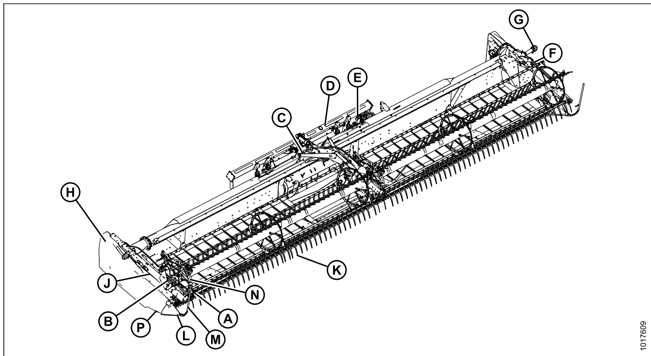
Рисунок 2.2: Жатка комбайна серии D1 — показано двойное мотовило
