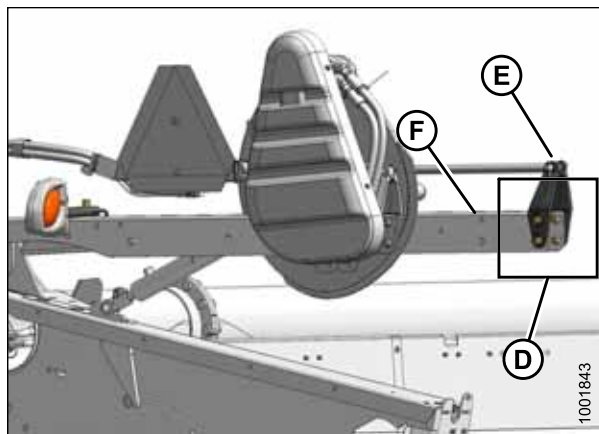
Рисунок 3.103: Цилиндр правого рычага мотовила в переднем положении
