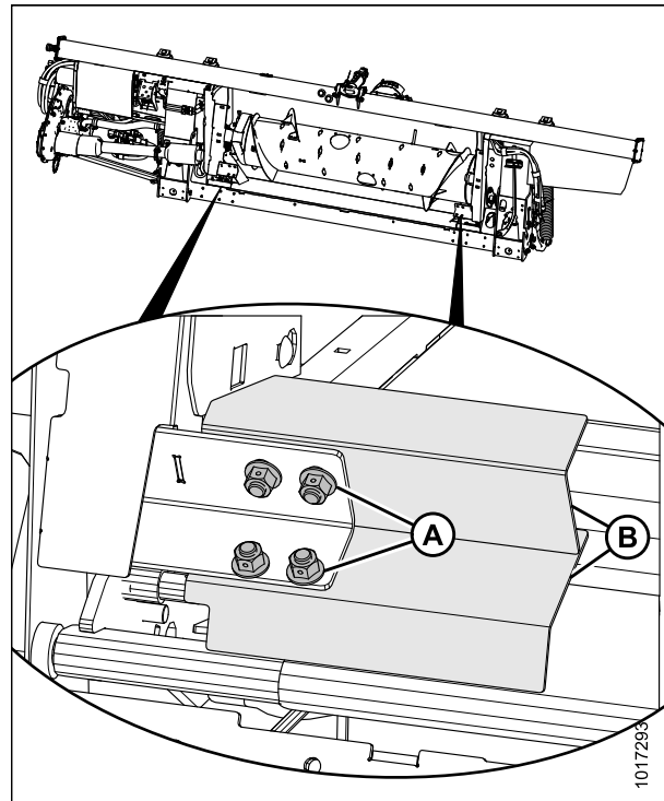
Рисунок 5.201: Чистик
