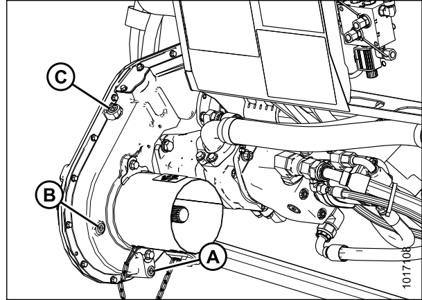
Рисунок 5.28: Редуктор привода жатки
