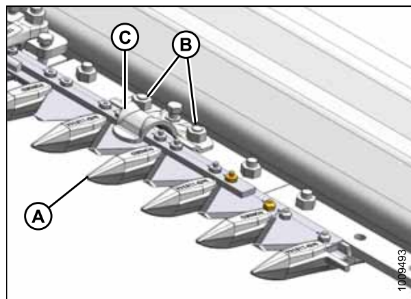
Рисунок 5.98: Заостренные противорежущие пальцы
