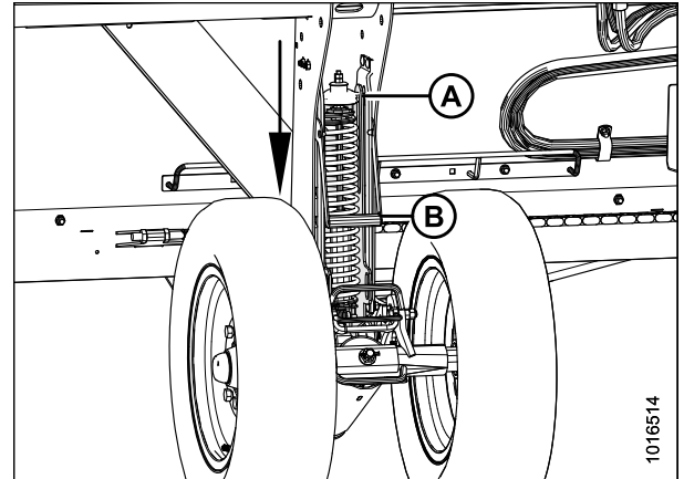
Рисунок 3.416: Передние (левые) колеса
