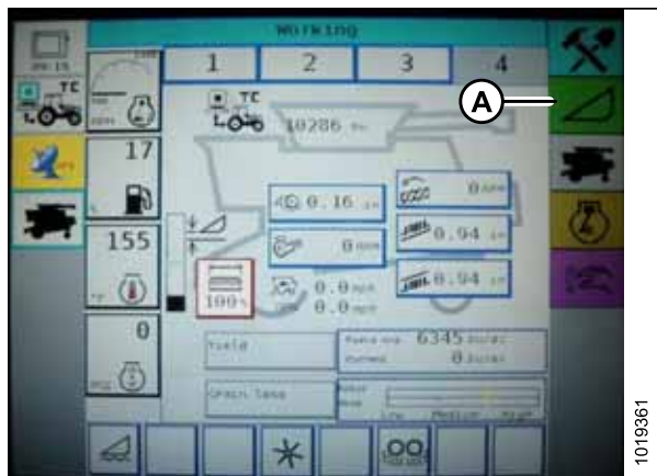
Рисунок 3.213: Приборная панель комбайна Challenger
