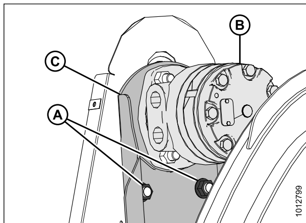
Рисунок 5.305: Привод единого мотвила
