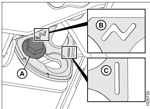
Рисунок 3.149: Положения флотации шнека
