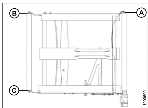
Рисунок 5.223: Рычаги роликов
