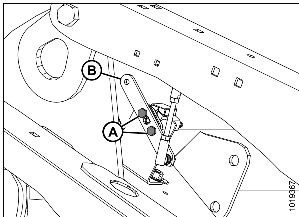
Рисунок 3.97: Датчик высоты мотовила — правый рычаг мотовила
