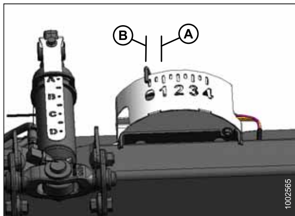
Рисунок 3.373: Блок индикатора флотации
