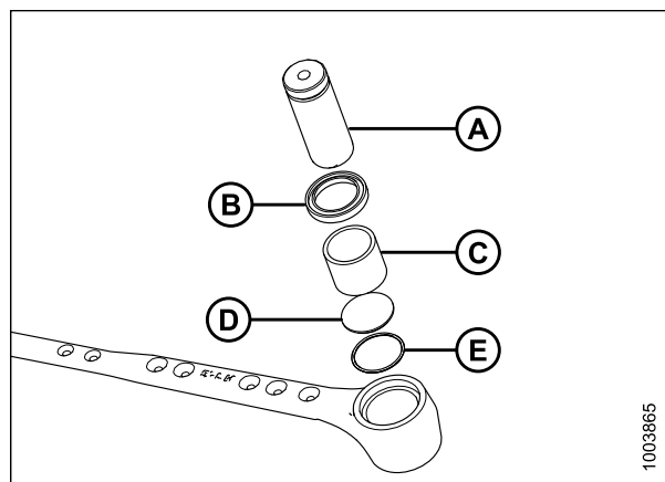
Рисунок 5.91: Подшипник головки ножа в сборе
