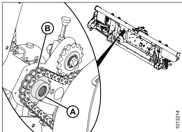
Рисунок 5.60: Привод шнека
