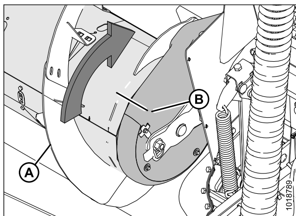
Рисунок 5.53: Привод шнека
