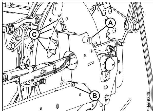
Рисунок 3.133: Положения диска эксцентрика
