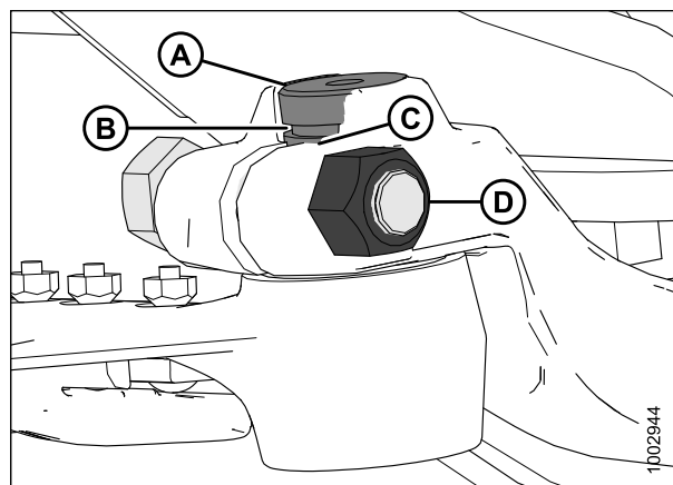
Рисунок 5.93: Головка ножа
