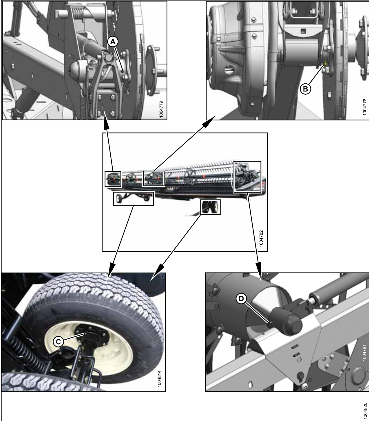
A — правый подшипник подбарающего мотовила (одно место) B — центральный подшипник подбарающего мотовила (одно место) C — подшипники колес (четыре места) D — левый подшипник подбарающего мотовила (одно место)
