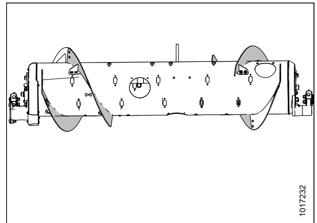
Рисунок 3.19: Узкая конфигурация (вид сзади)
