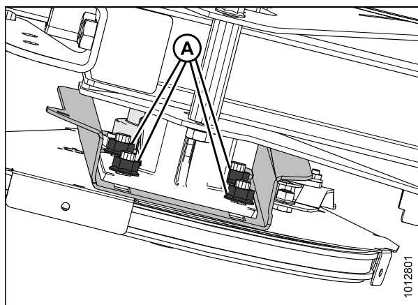
Рисунок 5.306: Привод единого мотвила — вид со стороны нижней части подбирающего мотвила
