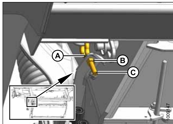
Рисунок 3.18: Натяжитель пружины
