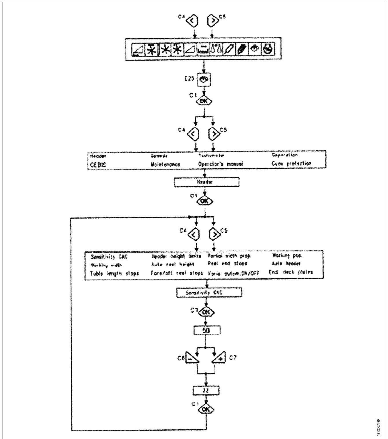
Рисунок 3.333: Схема действий по установке чувствительности механизма оптимизации флотации
