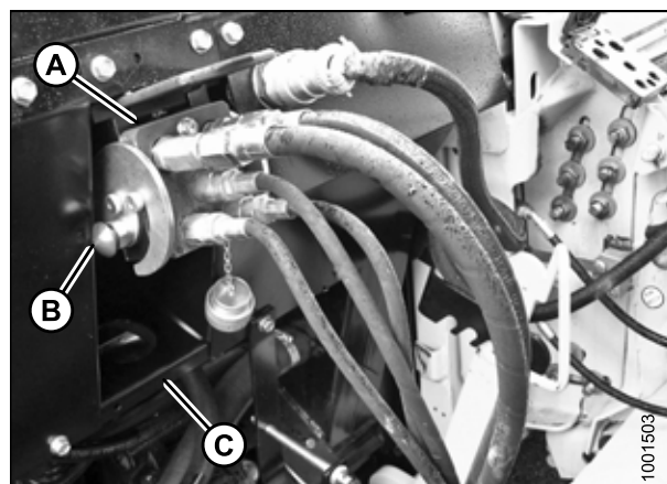
Рисунок 4.85: Соединения модуля флотации
