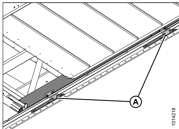
Рисунок 5.218: Опоры направляющей полотна
