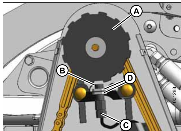
Рисунок 5.334: Датчик скорости
