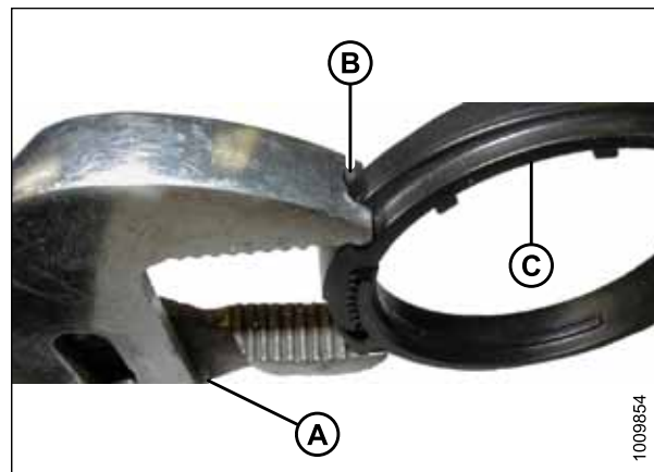
Рисунок 5.275: Модифицированные клещи
