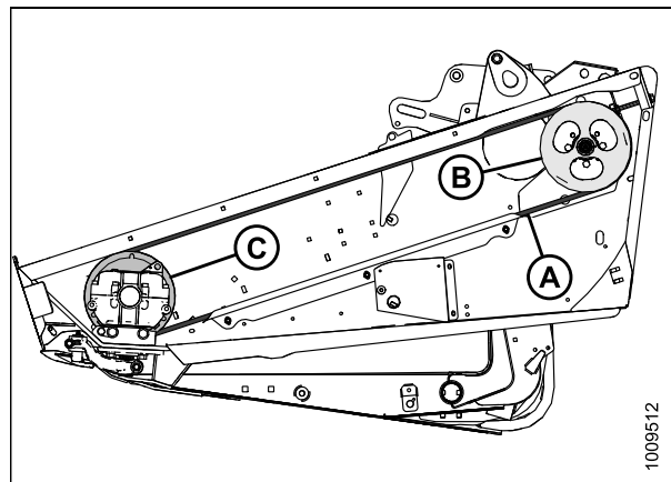
Рисунок 5.134: Привод ножа
