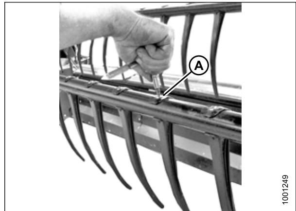
Рисунок 5.260: Установка пластмассового пальца
