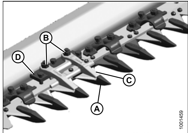
Рисунок 5.101: Центральные противорежущие пальцы
