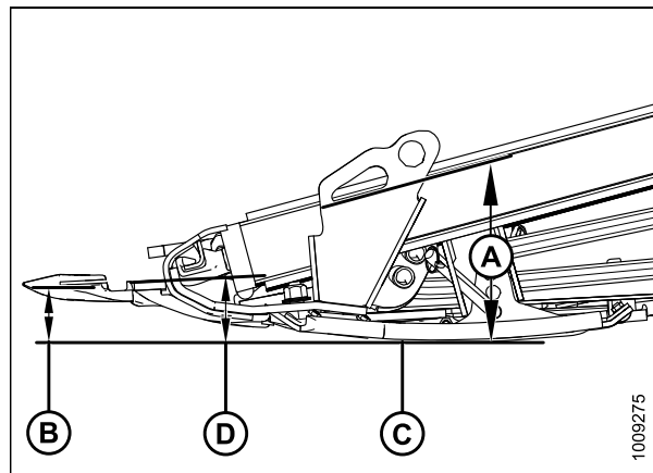
Рисунок 3.87: Угол атаки жатки
