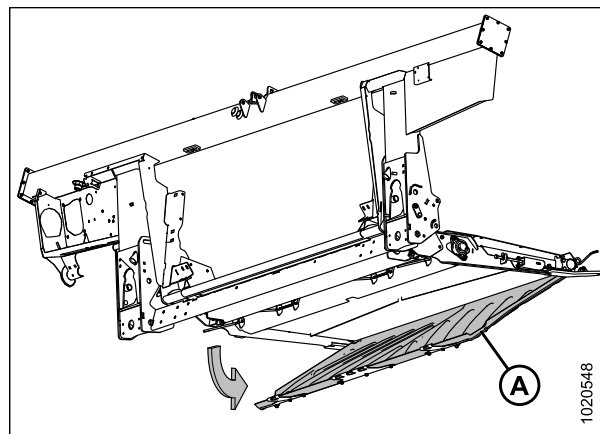
Рисунок 5.197: Поддон направляющей подачи (вид сзади)
