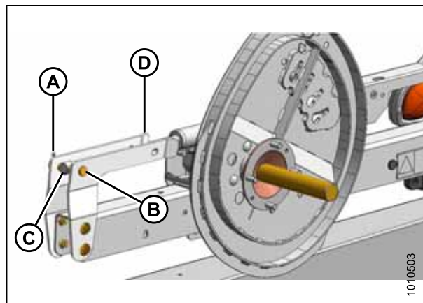
Рисунок 3.117: Правый рычаг мотовила в переднем положении
