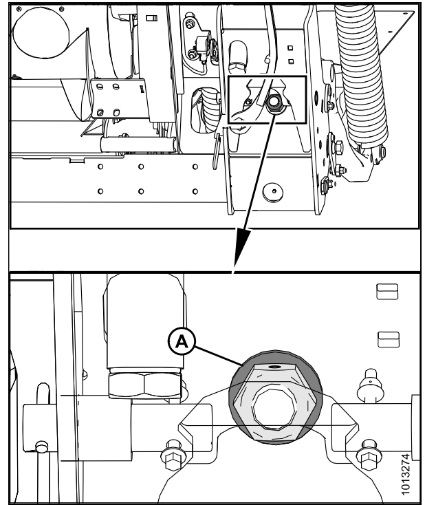
Рисунок 3.218: Блокировка флотации
