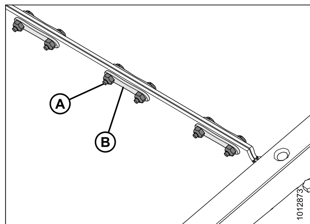
Рисунок 5.167: Накладки стыковочной планки полотна
