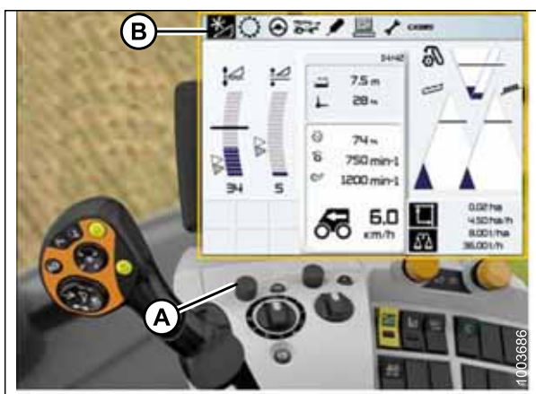
Рисунок 3.342: Приборная панель, консоль и рычаг управления комбайна
