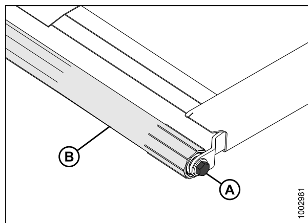
Рисунок 5.236: Приводной ролик
