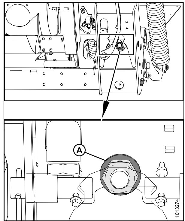
Рисунок 3.357: Блокировка флотации
