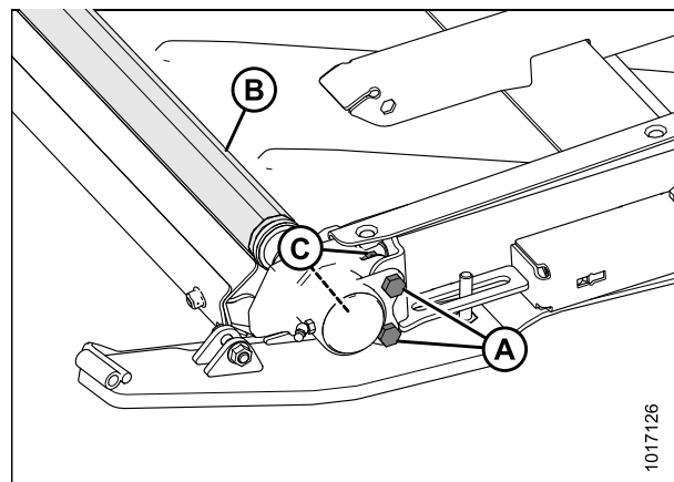
Рисунок 5.192: Натяжной ролик
