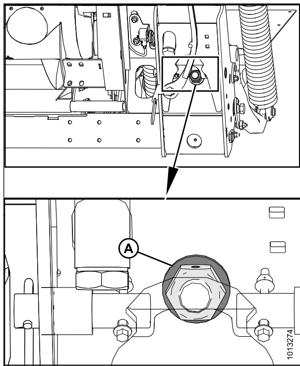
Рисунок 5.49: Блокировка флотации
