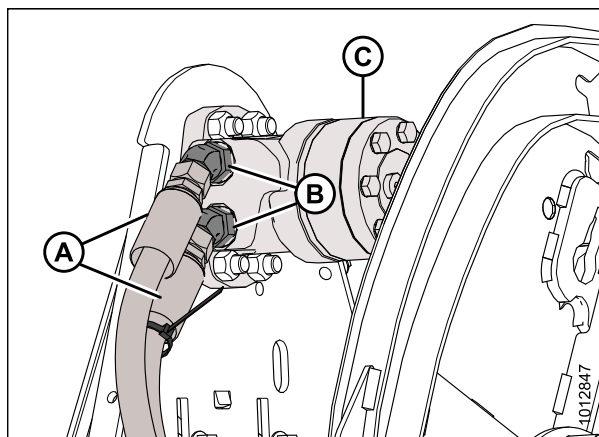
Рисунок 5.323: Мотор и шланги подбирающего мотовила
