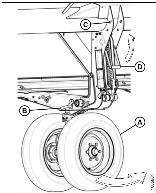
Рисунок 3.414: Передние (левые) колеса
