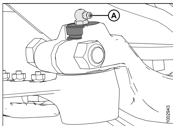
Рисунок 5.94: Головка ножа
