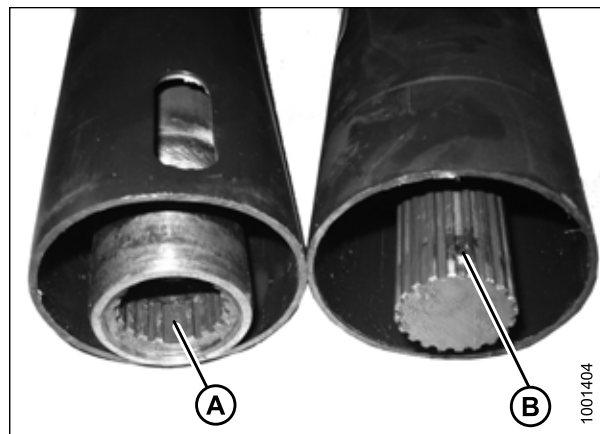
Рисунок 5.46: Привод
