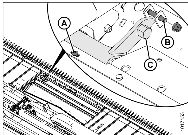
Рисунок 4.111: Защелка модуля флотации
