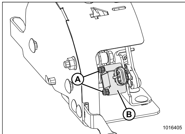
Рисунок 3.164: Датчик АННС в сборе
