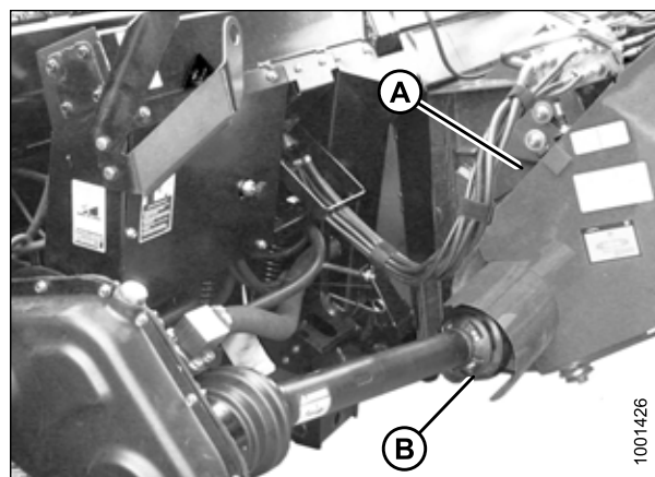
Рисунок 4.48: Привод
