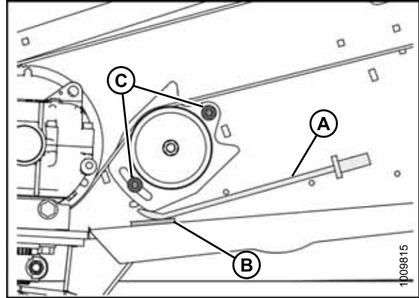
Рисунок 5.149: Привод ножа – левая сторона
