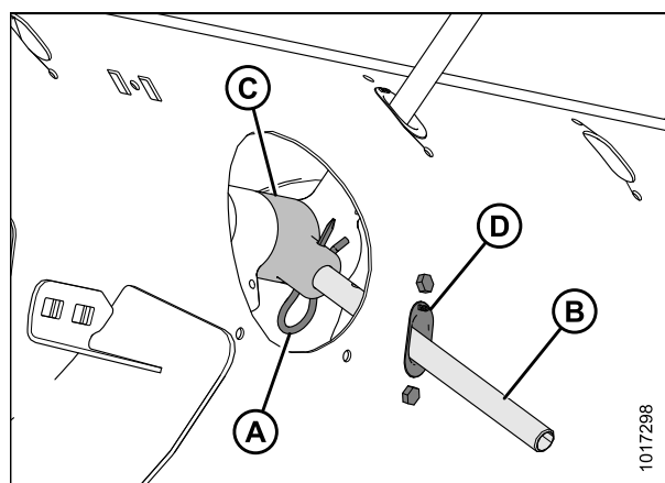
Рисунок 5.77: Палец шнека
