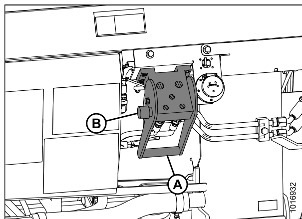
Рисунок 4.86: Ответные части модуля флотации
