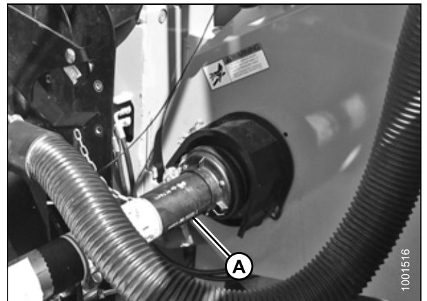
Рисунок 4.63: Привод и выходной вал
