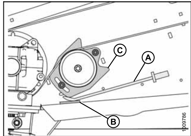
Рисунок 5.155: Показана левая сторона – правая сторона в зеркальном отображении
