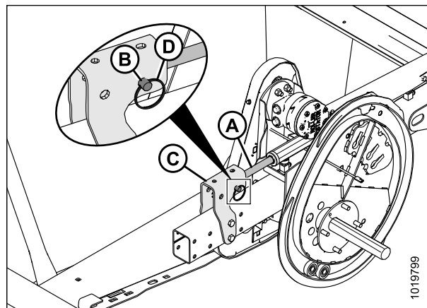
Рисунок 3.121: Центральный рычаг мотовила в заднем положении
