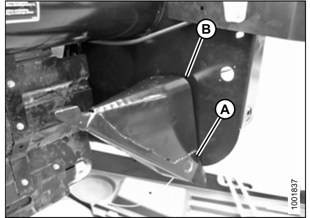
Рисунок 3.140: Делитель в отсеке для хранения
