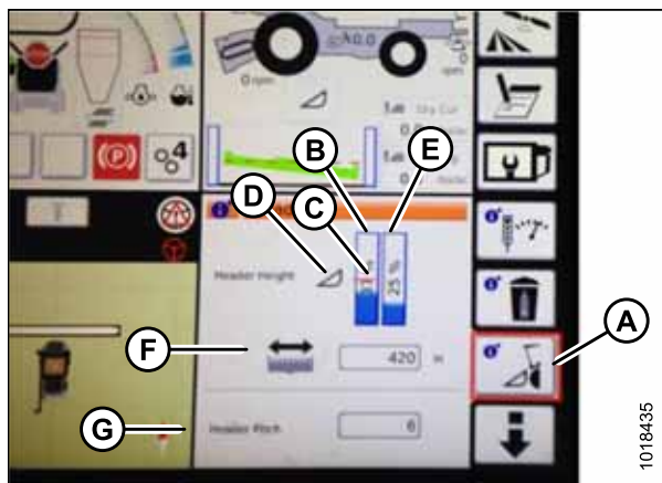
Рисунок 3.262: Группы жатки
