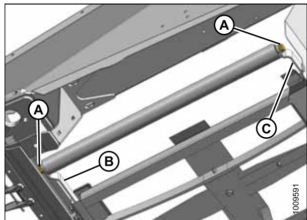
Рисунок 5.226: Натяжной ролик
