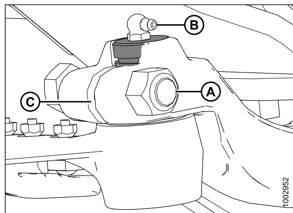
Рисунок 5.90: Головка ножа
