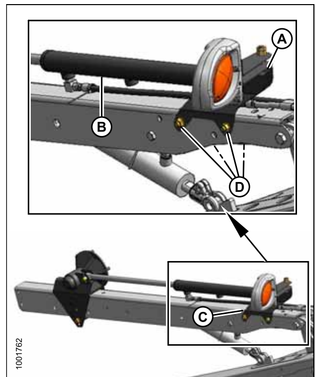
Рисунок 3.112: Левый рычаг — заднее положение
