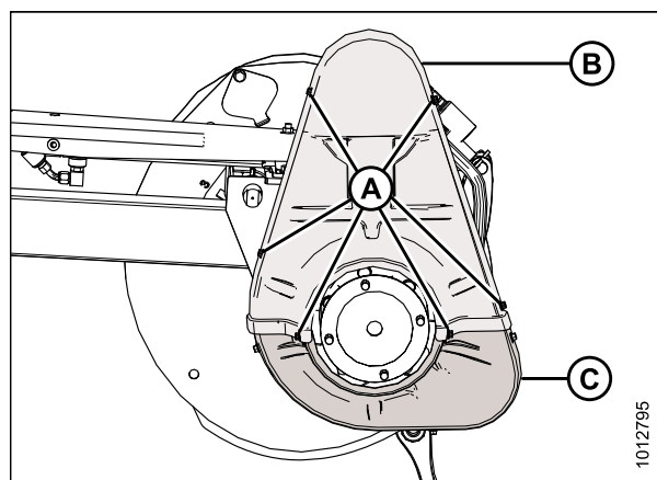
Рисунок 5.304: Крышка привода — сдвоенное мотовило
