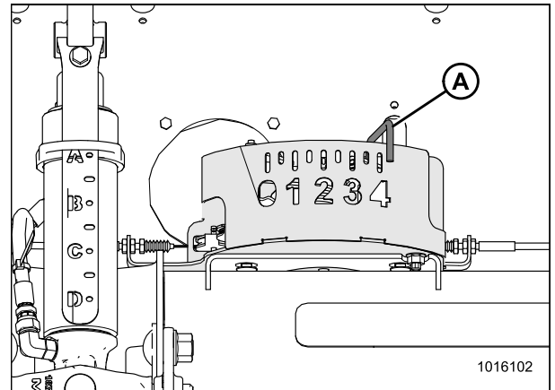
Рисунок 3.162: Блок индикатора флотации
