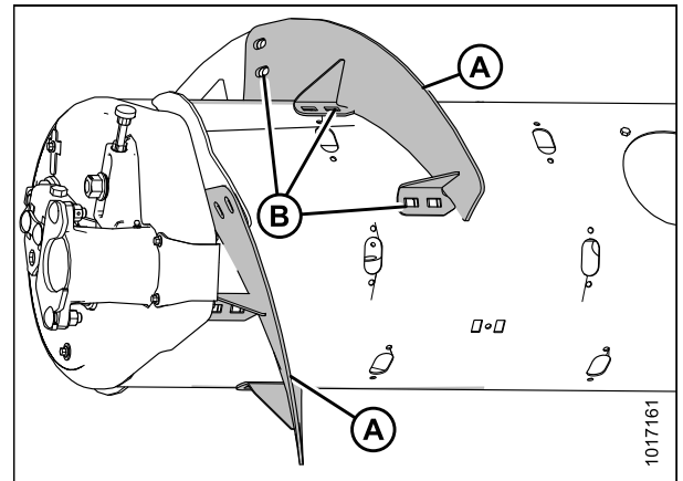
Рисунок 3.27: Средняя конфигурация (левая сторона)
