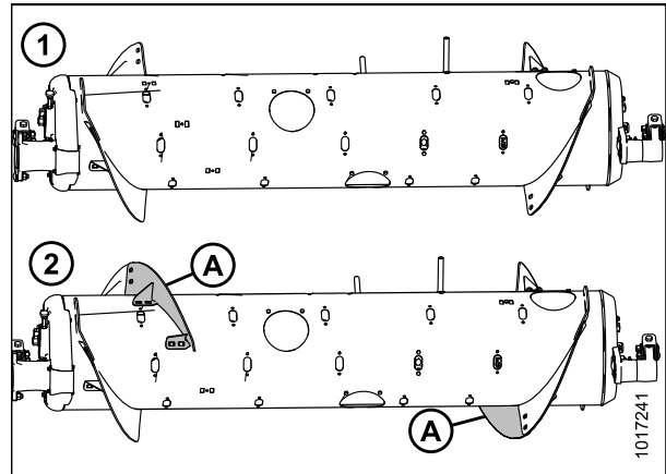
Рисунок 3.29: Конфигурации шнека (вид сзади)
