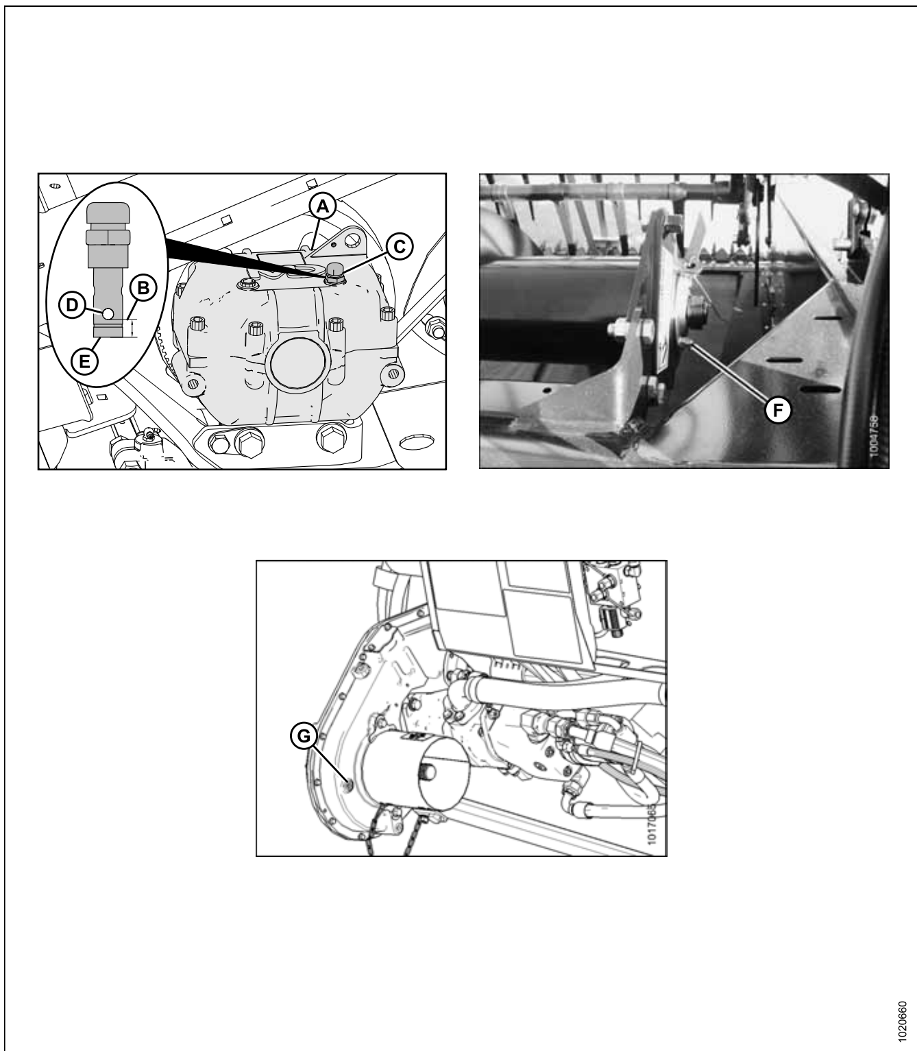
Рисунок 5.9: Каждые 100 часов
