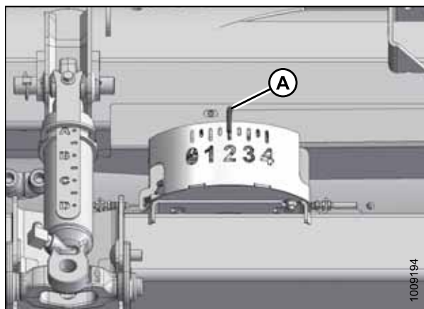
Рисунок 3.76: Срезание по давлению на почву
