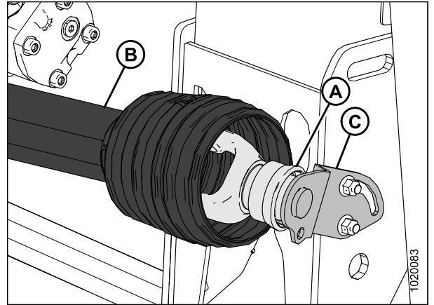
Рисунок 4.62: Привод
