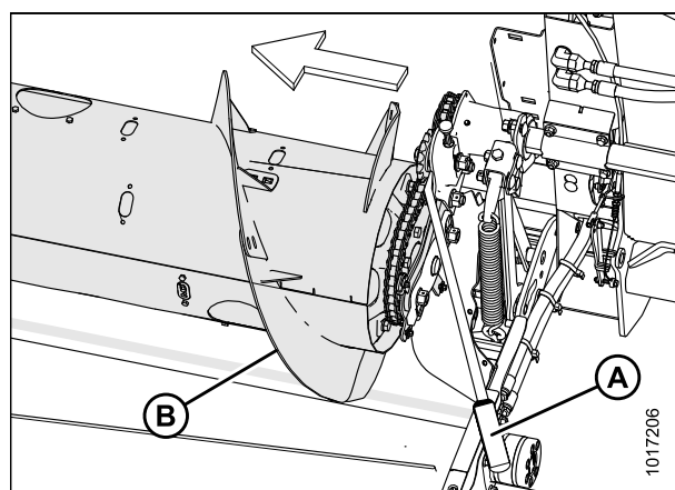
Рисунок 5.59: Привод шнека
