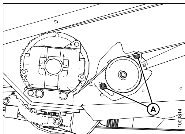
Рисунок 5.147: Привод ножа – левая сторона
