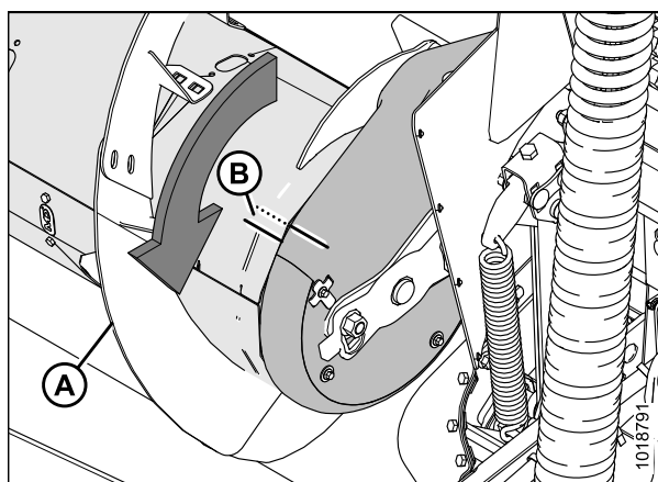
Рисунок 5.54: Привод шнека
