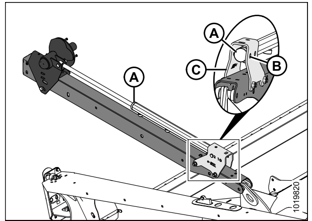
Рисунок 3.126: Цилиндр левого рычага мотвила
