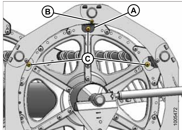
Рисунок 5.297: Опоры боковых щитков подбирающего мотовила
