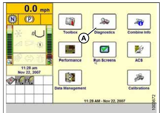
Рисунок 3.184: Приборная панель комбайна Case IH
