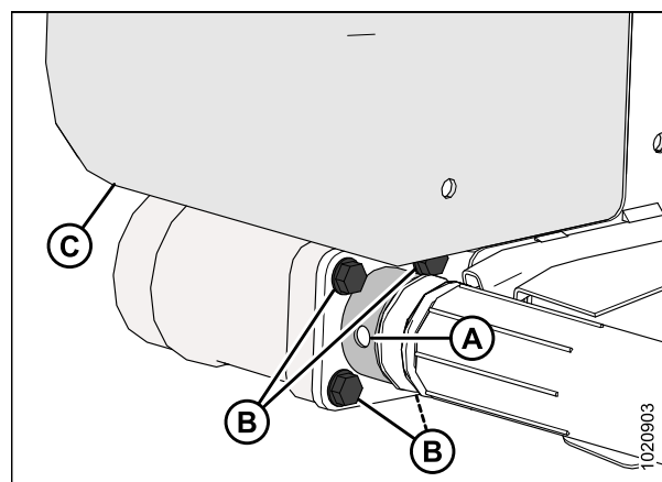
Рисунок 5.237: Приводной ролик
