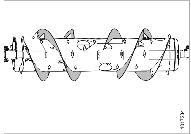
Рисунок 3.22: Ультразвуковая конфигурация (вид сзади)
