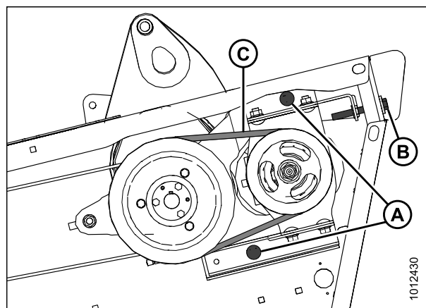
Рисунок 5.139: Клиновые ремни привода ножа
