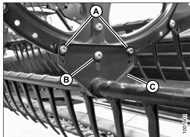
Рисунок 5.252: Кронштейн подбирающего мотовила
