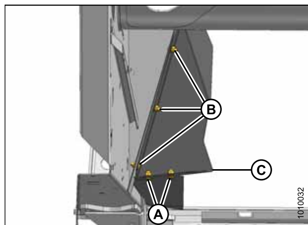
Рисунок 5.243: Задний дефлектор
