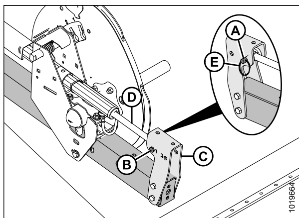
Рисунок 3.124: Цилиндр правого рычага мотовила в заднем положении
