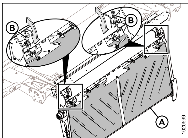
Рисунок 5.196: Нижняя сторона поддона направляющей подачи
