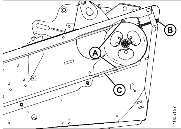
Рисунок 5.136: Привод двойного ножа без синхронизации
