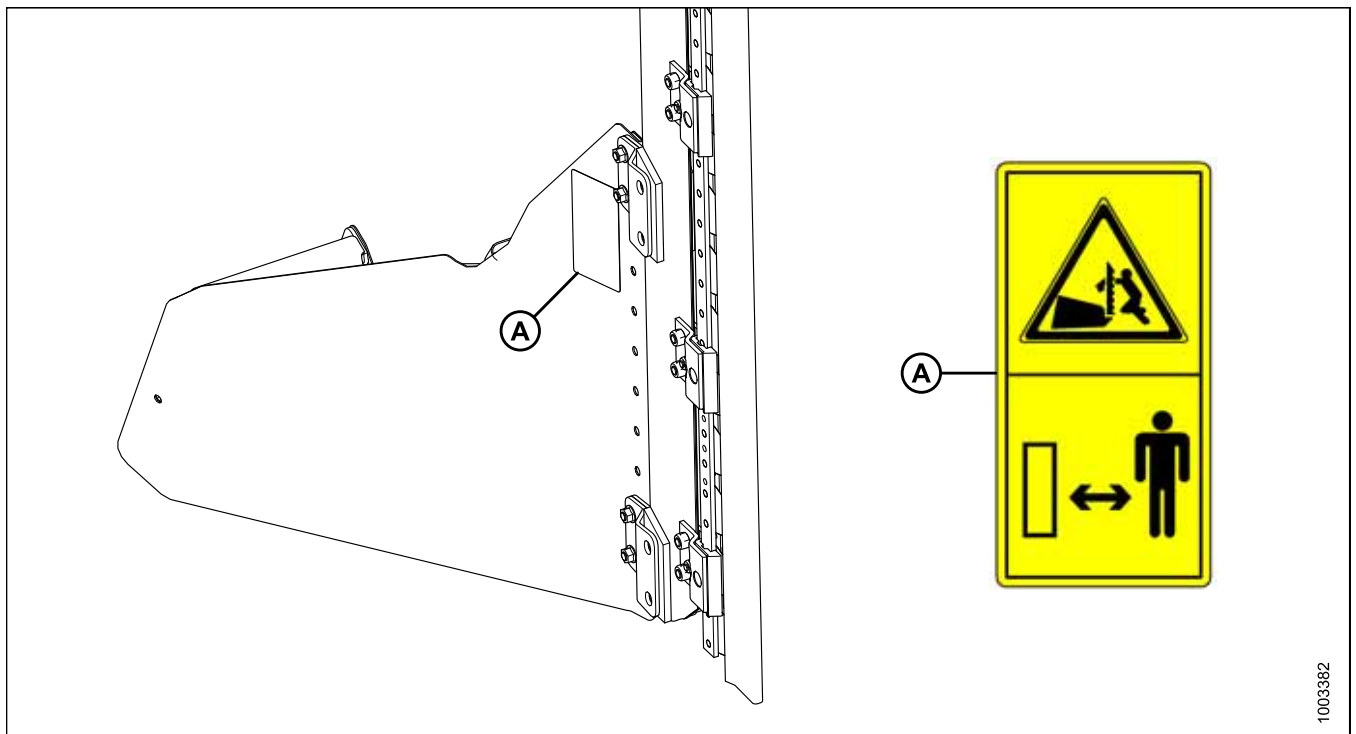
Рисунок 1.18: Вертикальный нож
