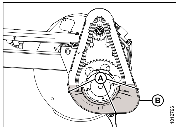
Рисунок 5.19: Нижняя крышка привода (верхняя крышка снята)
