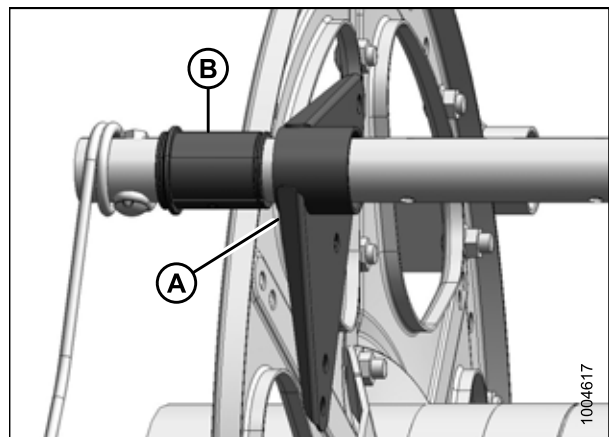
Рисунок 5.263: Втулка
