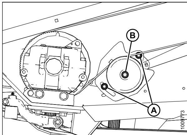
Рисунок 5.140: Привод ножа
