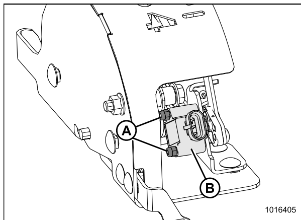
Рисунок 3.165: Датчик АННС в сборе
