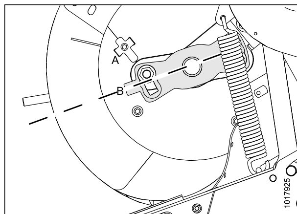
Рисунок 5.83: Настройка В шнека
