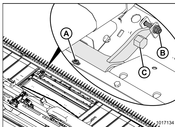
Рисунок 4.103: Защелка модуля флотации
