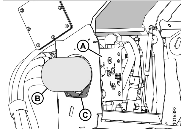
Рисунок 5.32: Гидравлическое оборудование FM100 (на изображении крышка снята, чтобы был виден коллектор)
