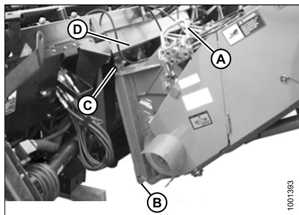
Рисунок 4.39: Комбайн и модуль флотации
