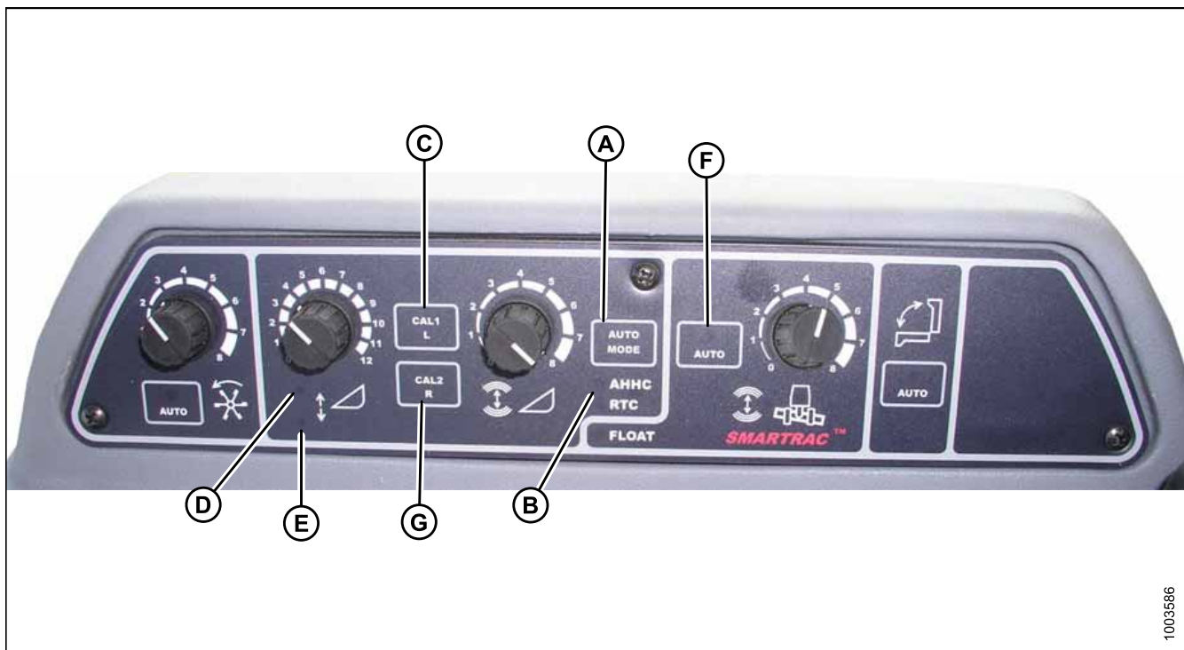
Рисунок 3.223: Элементы управления автоматического контроля высоты жатки комбайна
