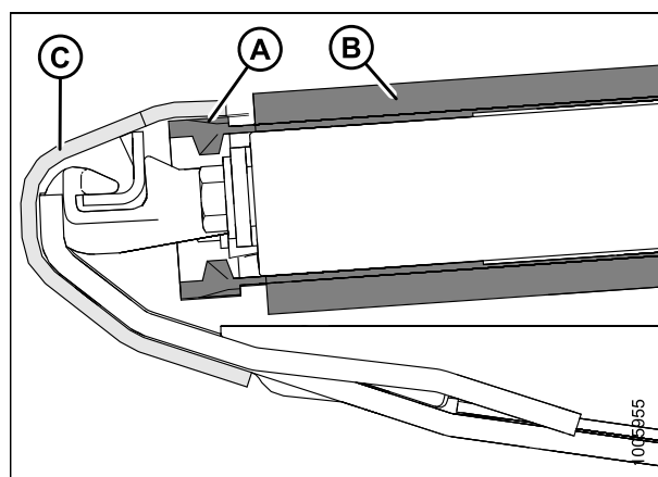
Рисунок 5.208: Уплотнение полотна
