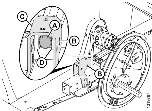
Рисунок 3.120: Центральный рычаг подбирающего мотовила
