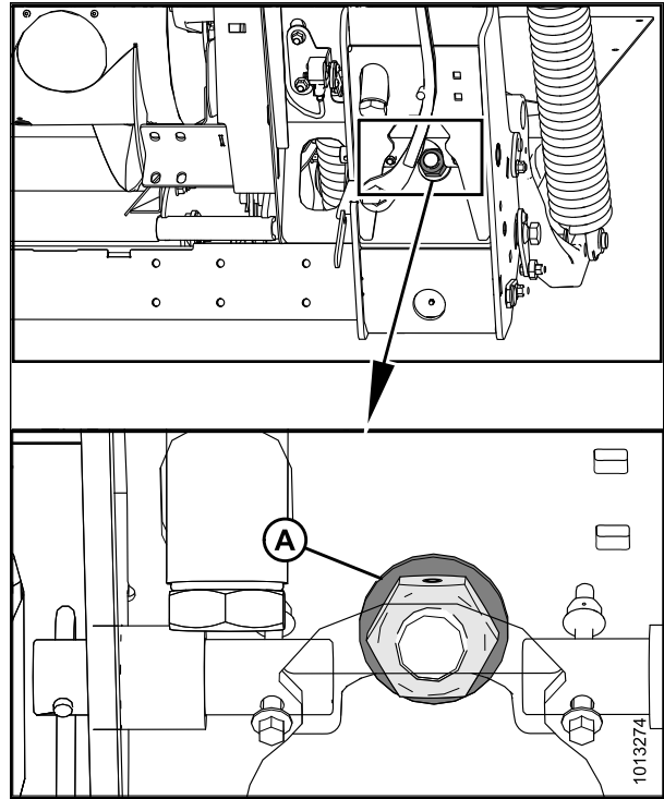
Рисунок 3.182: Блокировка флотации
