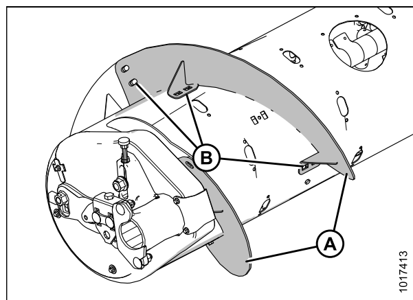
Рисунок 3.54: Левая сторона шнека
