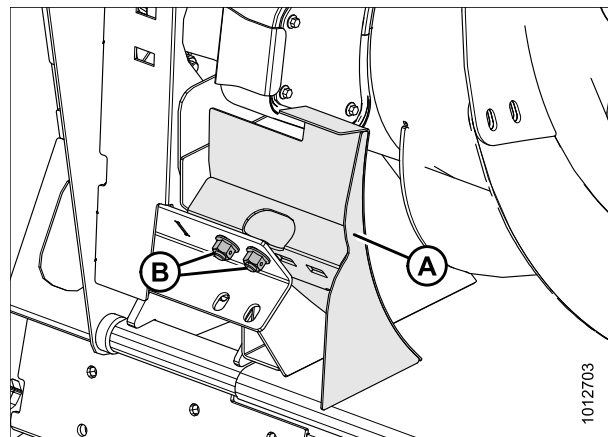
Рисунок 5.202: Дефлектор наклонной камеры
