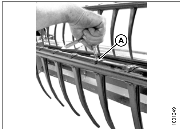
Рисунок 5.257: Снятие пластмассового пальца
