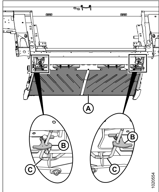
Рисунок 5.199: Поддон направляющей подачи (вид сзади)
