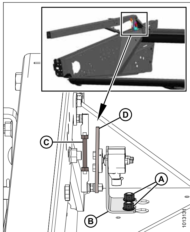
Рисунок 3.100: Датчик высоты мотовила — правый рычаг мотовила (вид спереди)
