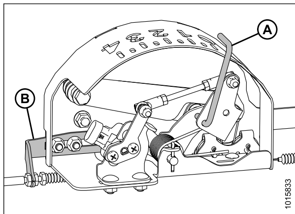
Рисунок 3.176: Блок индикатора флотации
