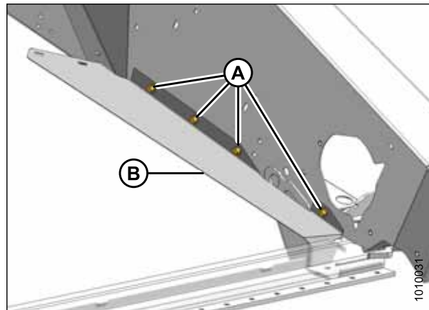
Рисунок 5.242: Передний дефлектор
