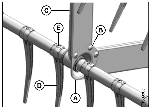
Рисунок 5.292: Противоположная опора
