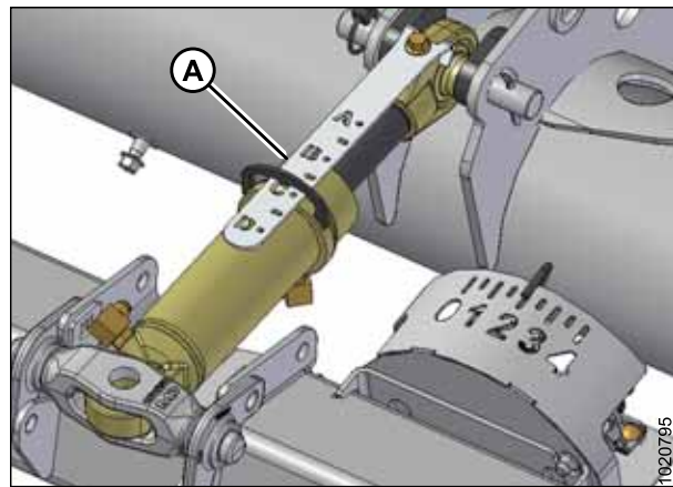
Рисунок 3.77: Центральное соединение
