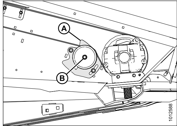
Рисунок 5.154: Привод ножа – правая сторона
