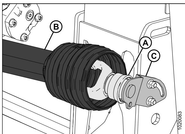
Рисунок 4.29: Привод
