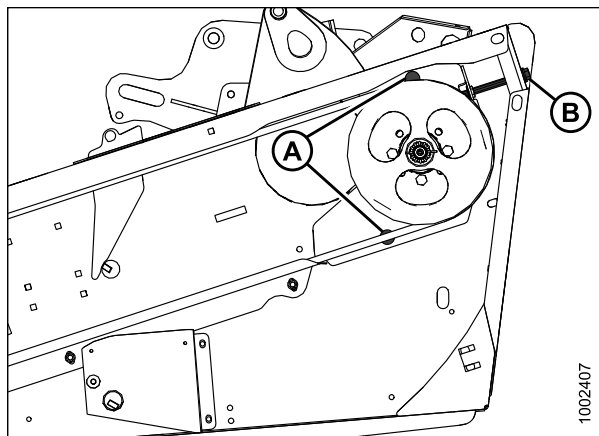
Рисунок 5.131: Привод двойного ножа без синхронизации
