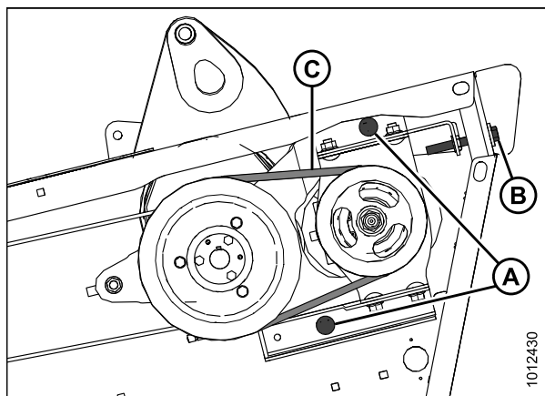
Рисунок 5.141: Клиновые ремни привода ножа
