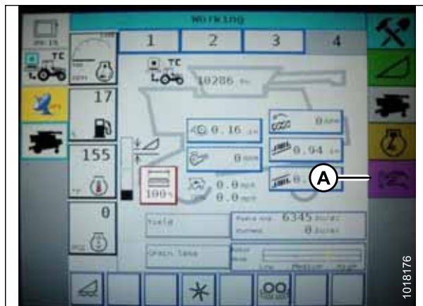
Рисунок 3.207: Приборная панель комбайна Challenger
