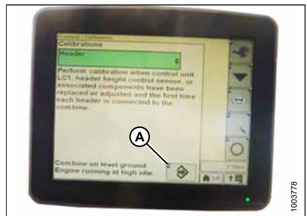
Рисунок 3.301: Дисплей комбайна John Deere
