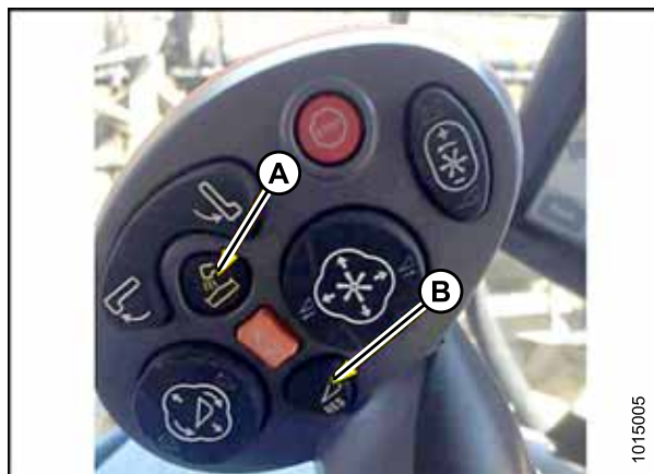
Рисунок 3.381: Органы управления комбайнов New Holland
