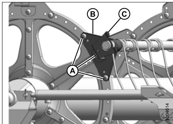
Рисунок 5.265: Хвостовик
