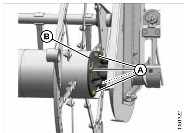
Рисунок 5.318: Крестовина
