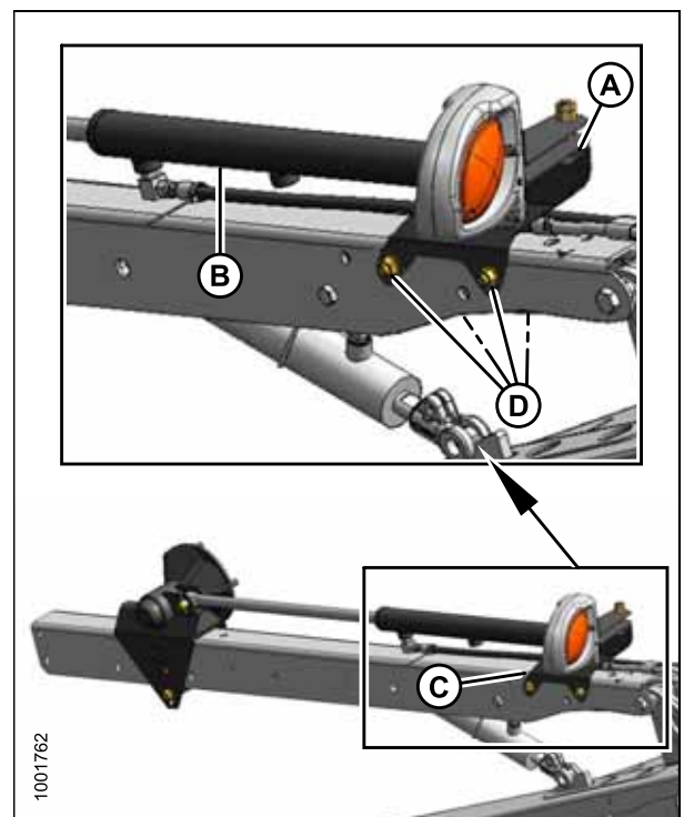
Рисунок 3.106: Цилиндр левого рычага мотовила в заднем положении
