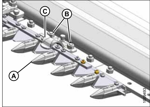
Рисунок 5.100: Заостренные противорежущие пальцы
