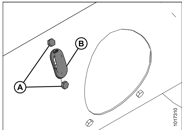
Рисунок 5.86: Направляющая пальца шнека
