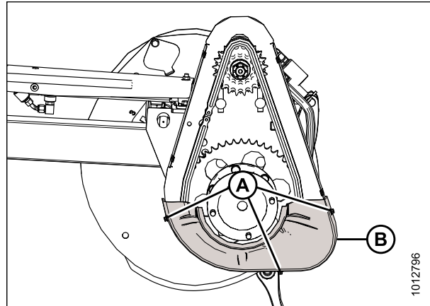
Рисунок 5.301: Нижняя крышка привода (верхняя крышка снята)
