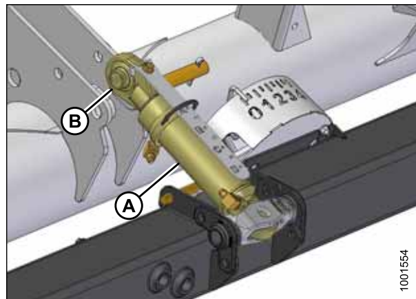
Рисунок 4.97: Центральное соединение
