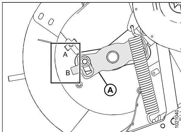
Рисунок 5.80: Индикатор синхронизации пальцев граблины шнека
