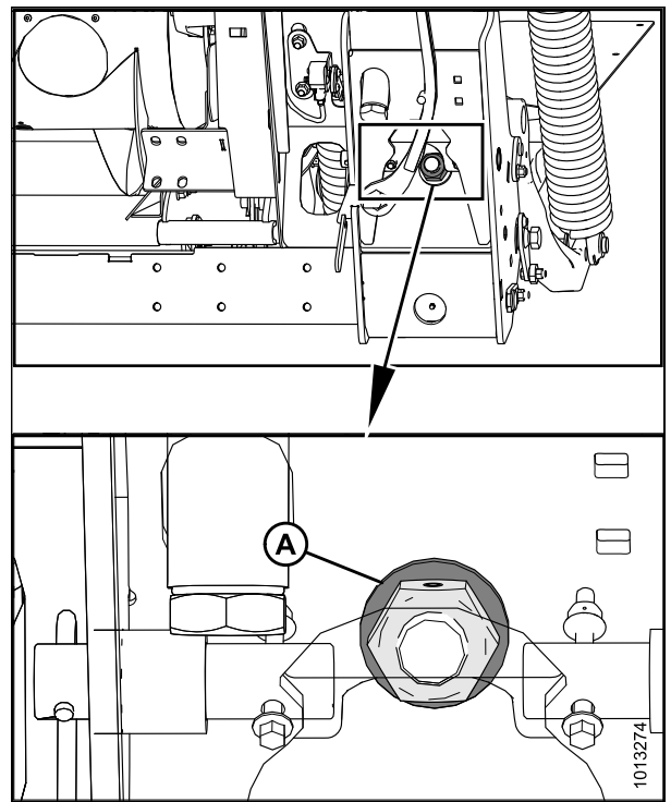
Рисунок 3.291: Блокировка флотации
