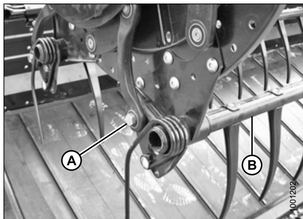
Рисунок 5.267: Сторона эксцентрика
