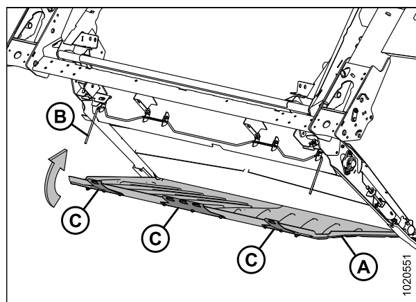
Рисунок 5.198: Нижняя сторона поддона направляющей подачи (вид сзади)
