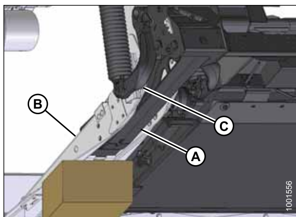
Рисунок 4.96: Нижняя сторона модуля флотации
