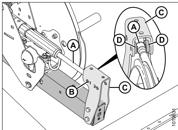
Рисунок 3.123: Цилиндр правого рычага мотовила
