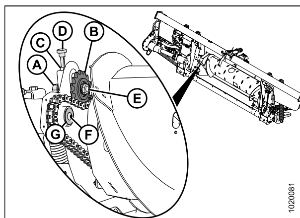
Рисунок 5.65: Привод шнека
