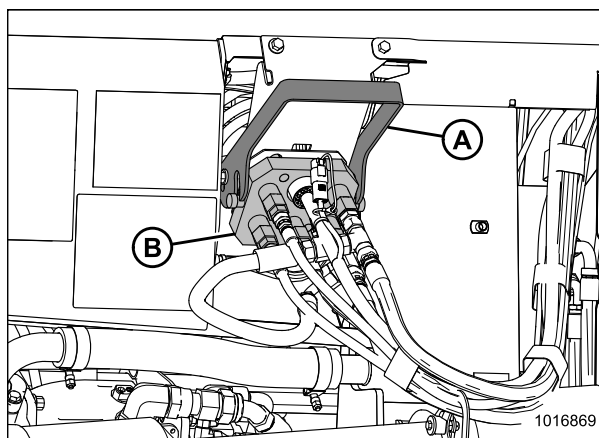
Рисунок 4.26: Многоканальная муфта модуля флотации
