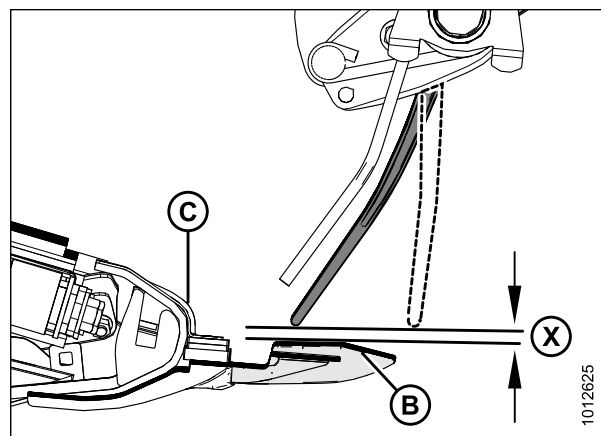
Рисунок 5.246: Зазор
