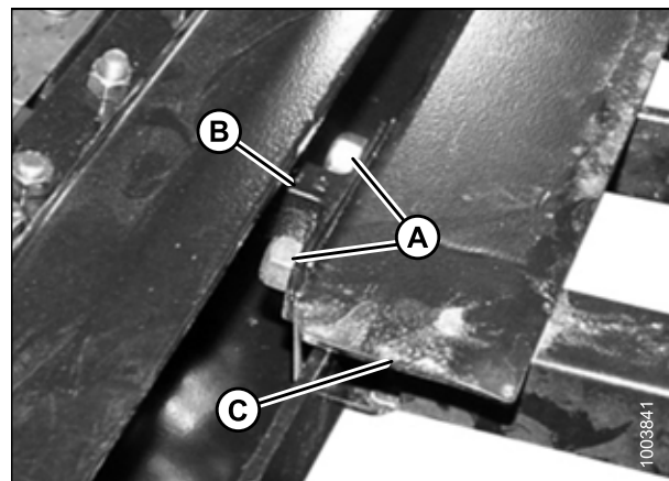
Рисунок 5.220: Опора направляющей
