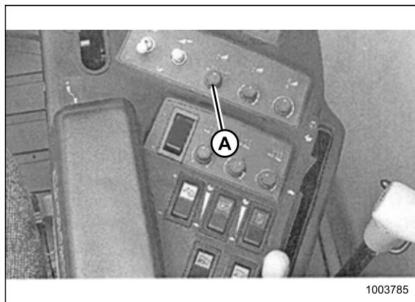
Рисунок 3.170: Правая консоль
