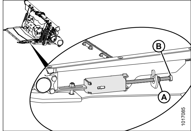
Рисунок 5.179: Натяжитель подающего полотна
