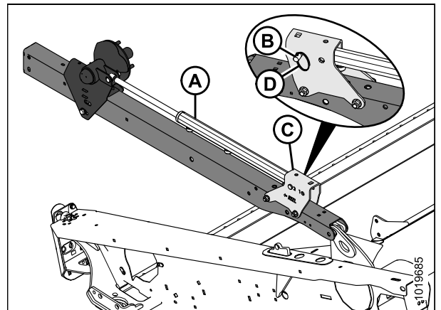
Рисунок 3.127: Цилиндр левого рычага мотвила в заднем положении
