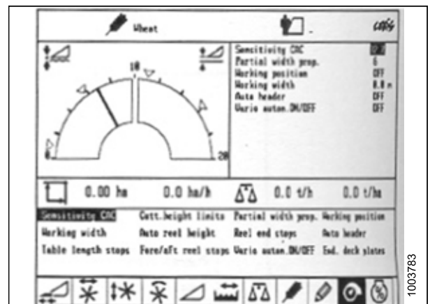
Рисунок 3.325: Приборная панель комбайна CLAAS
