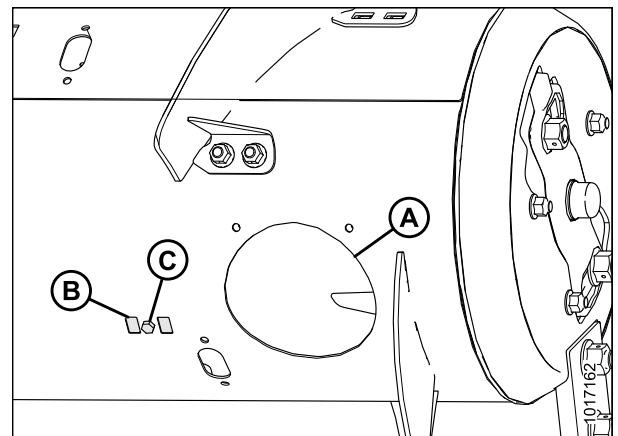
Рисунок 3.28: Заглушка витков спирали в средней конфигурации (правая сторона)
