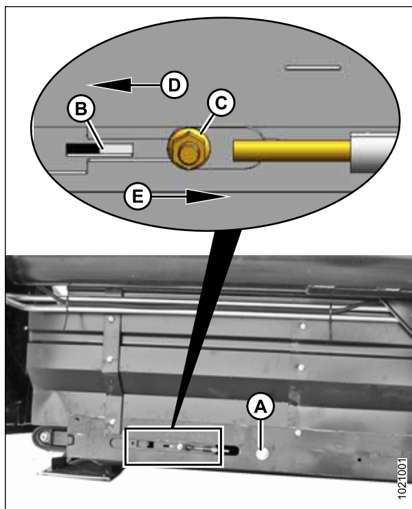
Рисунок 5.213: Показан левый регулятор натяжения — правый находится на противоположной стороне
