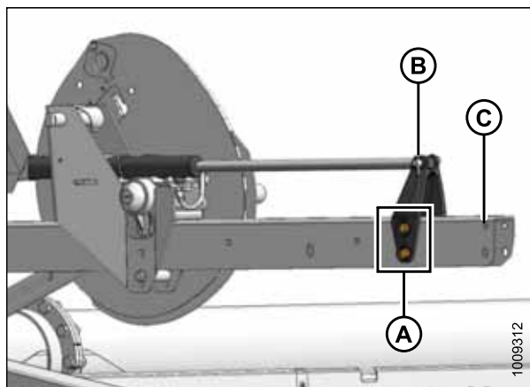
Рисунок 3.110: Цилиндр правого рычага мотовила в заднем положении
