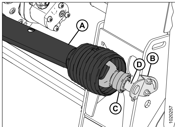
Рисунок 4.67: Привод
