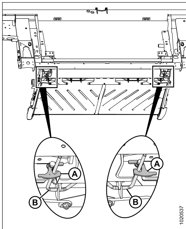
Рисунок 5.195: Поддон направляющей подачи (вид сзади)
