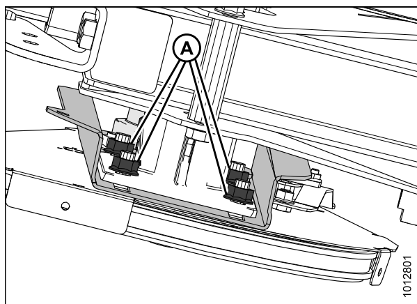
Рисунок 5.310: Привод единого мотвила — вид со стороны нижней части подбирающего мотвила
