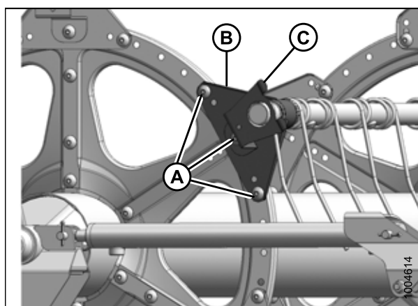
Рисунок 5.285: Хвостовик
