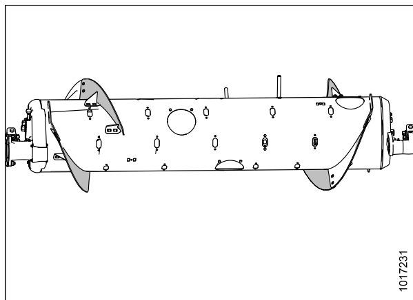
Рисунок 3.20: Средняя конфигурация (вид сзади)
