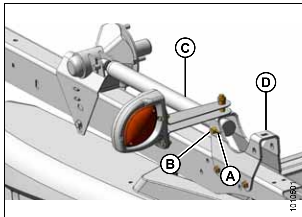
Рисунок 3.113: Левый рычаг мотовила в переднем положении
