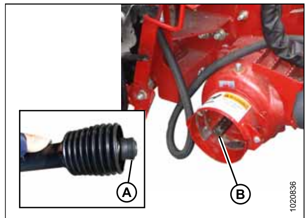
Рисунок 4.11: Выходной вал комбайна
