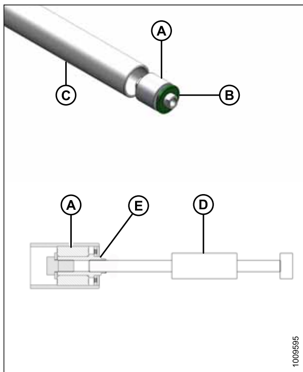
Рисунок 5.234: Подшипник натяжного ролика
