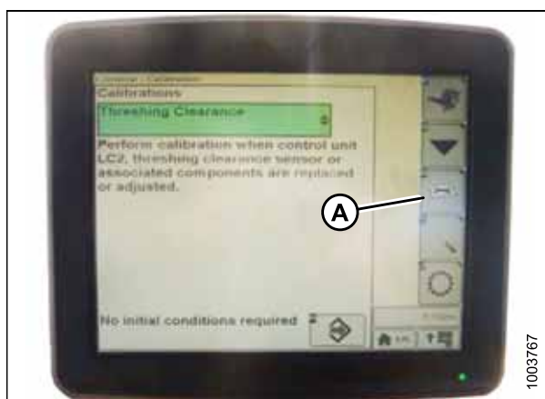
Рисунок 3.294: Дисплей комбайна John Deere
