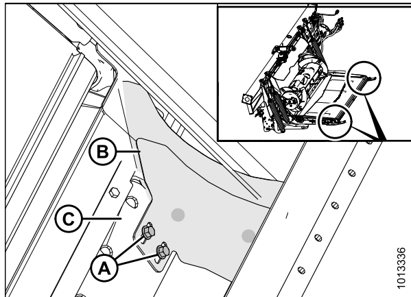
Рисунок 4.110: Укладчики
