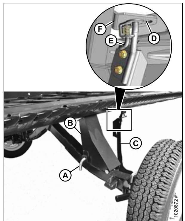
Рисунок 3.431: Положение заднего правого колеса
