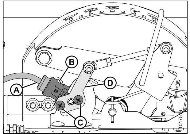
Рисунок 3.402: Датчик АННС
