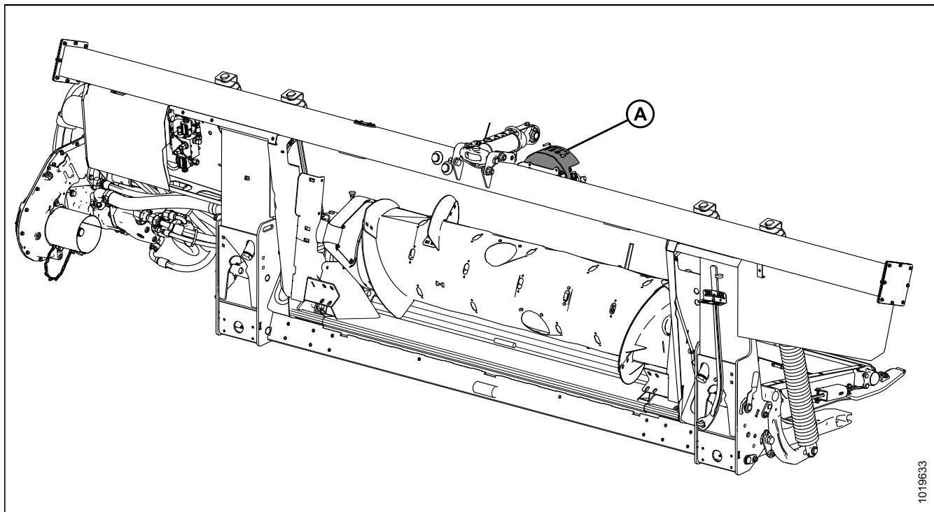
Рисунок 3.152: Модуль флотации FM100
