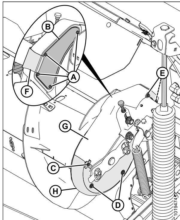
Рисунок 5.66: Привод шнека
