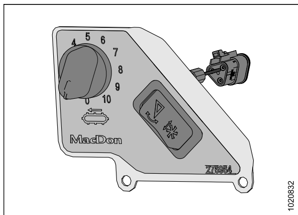
Рисунок 6.16: Регулятор ICDSC в кабине (показано для комбайна John Deere, Generic и Case New Holland аналогичны)
