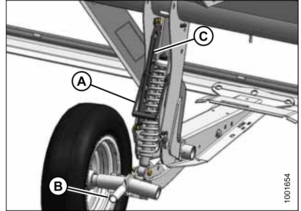
Рисунок 3.70: Стабилизирующее колесо
