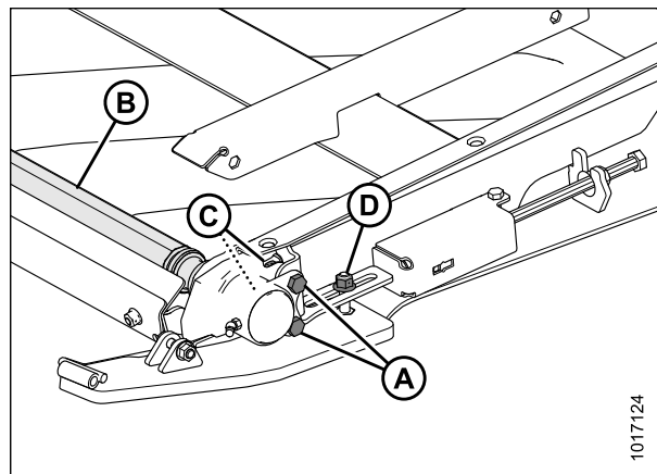
Рисунок 5.187: Натяжной ролик
