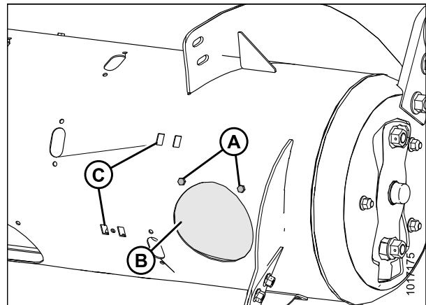
Рисунок 3.30: Широкая конфигурация (правая сторона)
