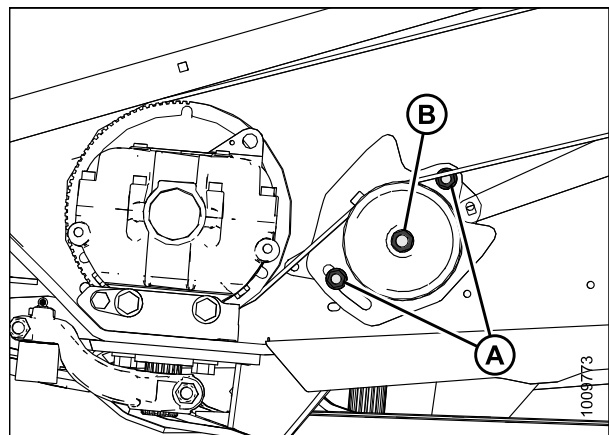
Рисунок 5.115: Привод двойного ножа с синхронизацией
