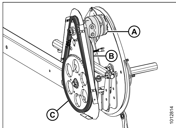
Рисунок 5.308: Изображен привод единого мотовила — привод сдвоенного мотовила имеет такую же конструкцию
