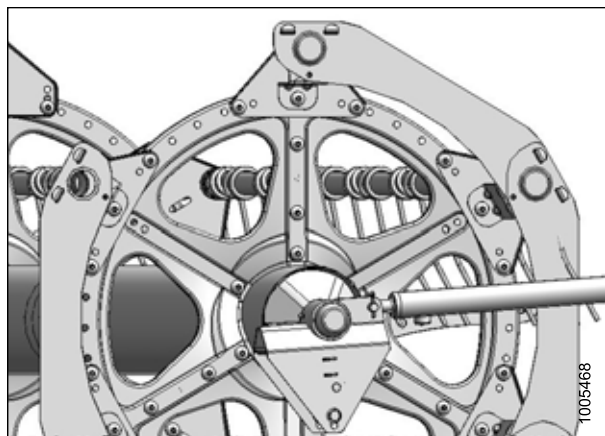
Рисунок 5.295: Боковые щитки подбирающего мотовила
