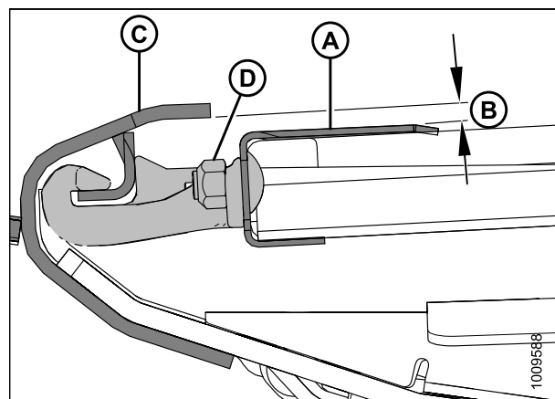
Рисунок 5.221: Опора направляющей
