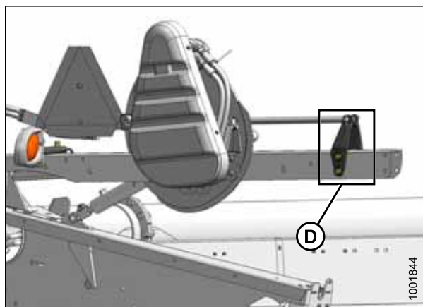
Рисунок 3.104: Цилиндр правого рычага мотовила в заднем положении
