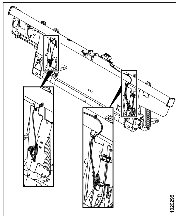
Рисунок 6.14: Сдвоенные датчики АННС
