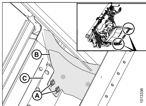
Рисунок 4.104: Укладчики
