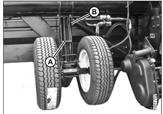
Рисунок 3.67: Левое колесо
