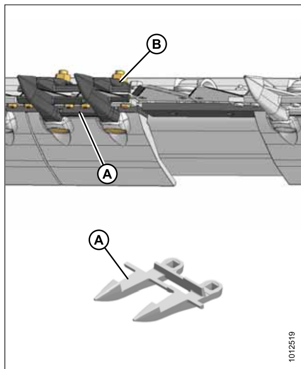
Рисунок 5.102: Центральные противорежущие пальцы
