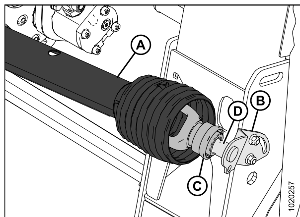
Рисунок 4.33: Привод
