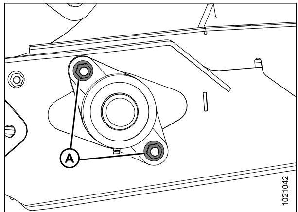
Рисунок 5.181: Подшипник приводного ролика подающего полотна
