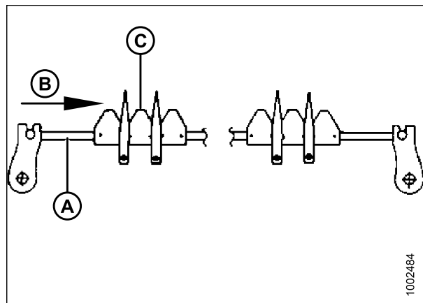
Рисунок 5.151: Регулировка синхронизации – левая сторона
