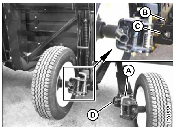
Рисунок 3.420: Задние рычаги
