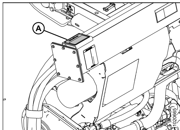
Рисунок 3. Модуль флотации
