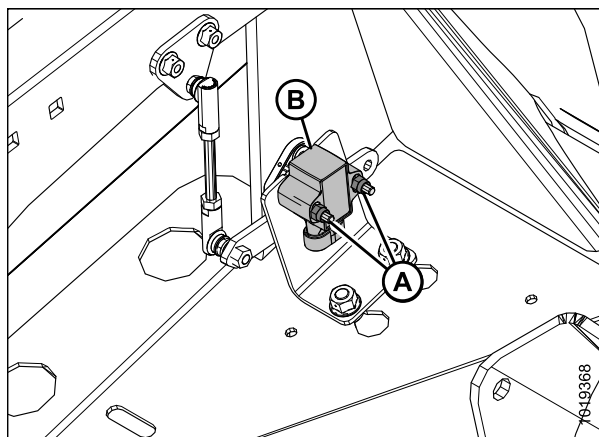
Рисунок 3.98: Датчик высоты мотовила — правый рычаг мотовила
