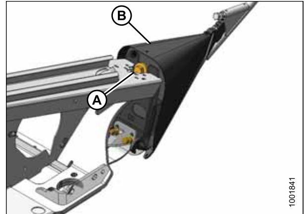
Рисунок 3.136: Делитель
