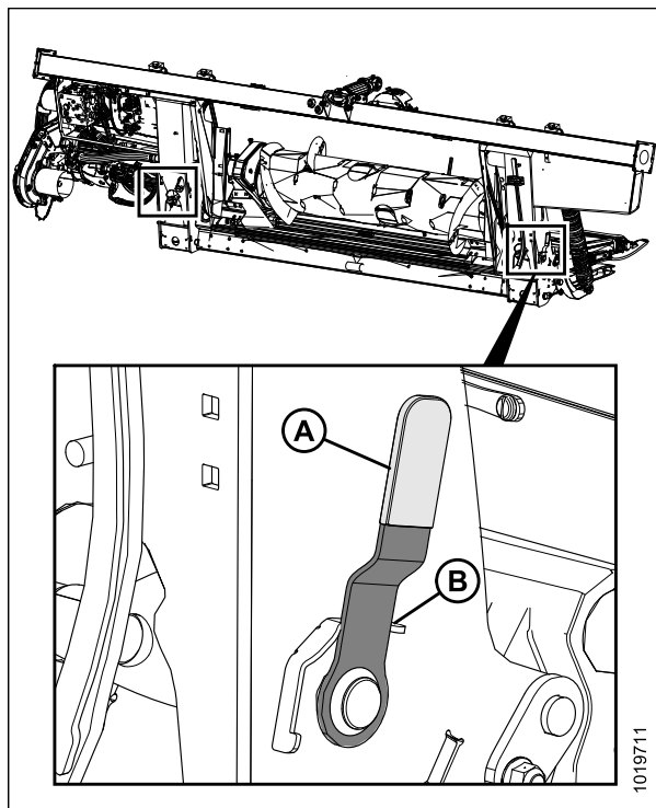
Рисунок 4.109: Ручка замка флотации (подробно показана правая сторона, левая сторона напротив)
