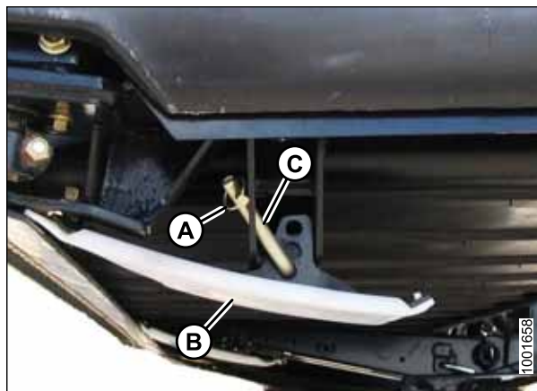
Рисунок 3.74: Внешний копирующий башмак
