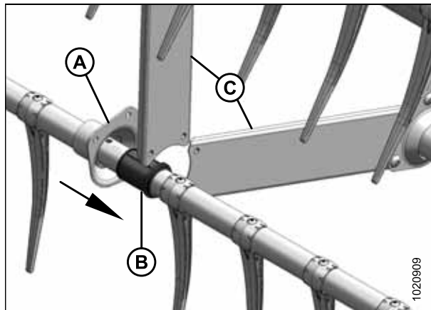
Рисунок 5.288: Противоположная опора
