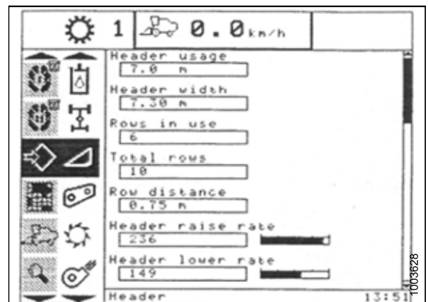
Рисунок 3.369: Приборная панель комбайнов New Holland
