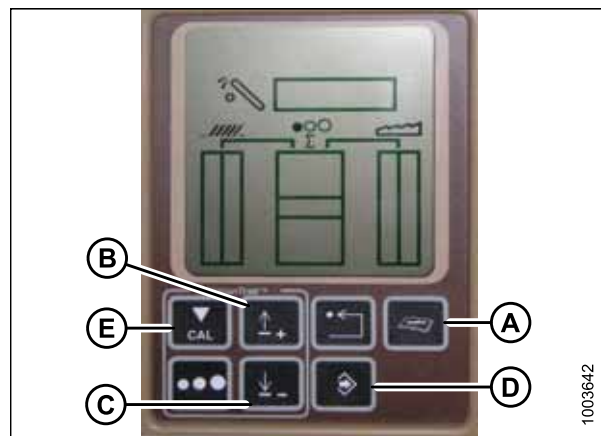
Рисунок 3.272: Дисплей комбайна John Deere
