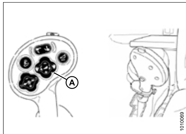
Рисунок 3.172: Рычаг управления (Case IH 5088/6088/7088)
