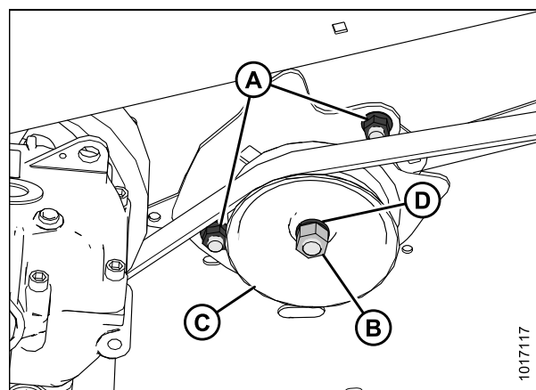
Рисунок 5.160: Привод ножа
