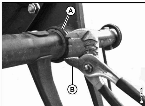
Рисунок 5.290: Установка хомута
