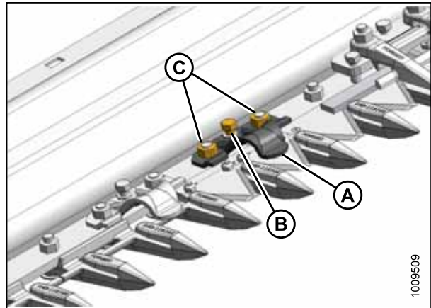
Рисунок 5.106: Прижим стандартного противорезущего пальца
