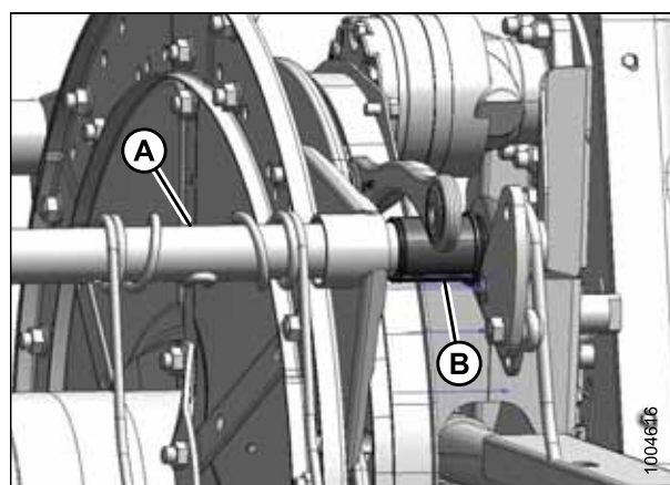
Рисунок 5.282: Страна эксцентрика
