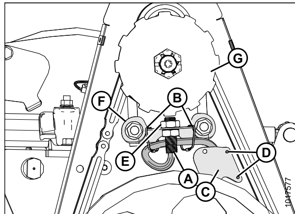
Рисунок 5.335: Датчик скорости
