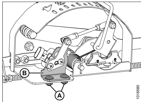
Рисунок 3.166: Датчик АННС в сборе
