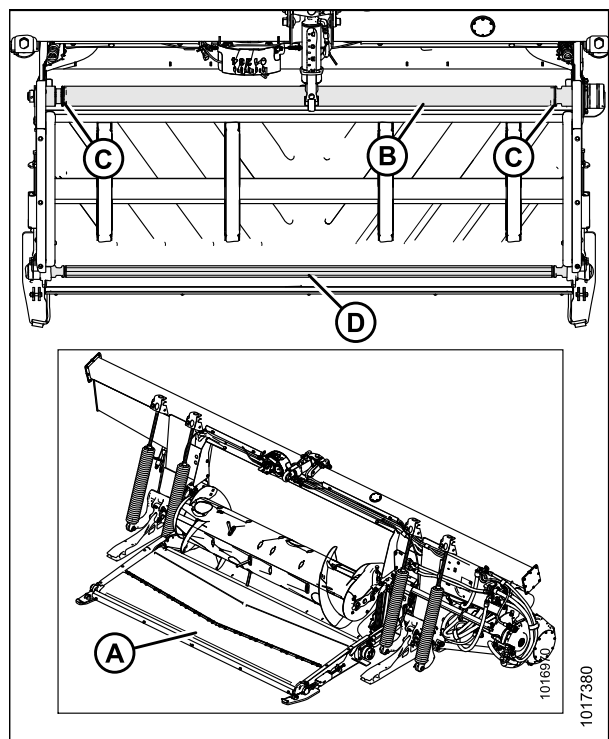
Рисунок 5.166: Подающее полотно модуля флотации
