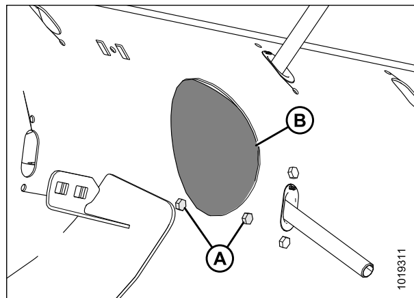
Рисунок 5.67: Крышка технологического люка щека
