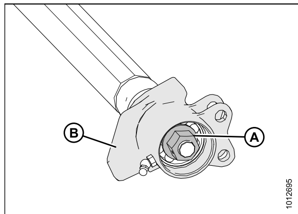
Рисунок 5.189: Натяжной ролик
