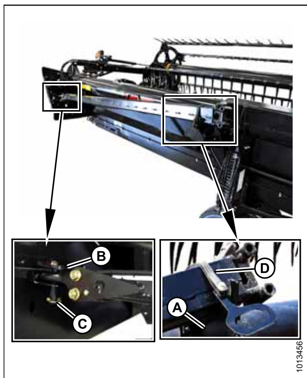
Рисунок 3.411: Хранение буксирной тяги — левая сторона
