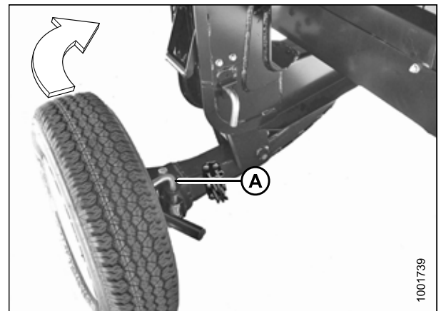
Рисунок 3.417: Заднее колесо — левая сторона
