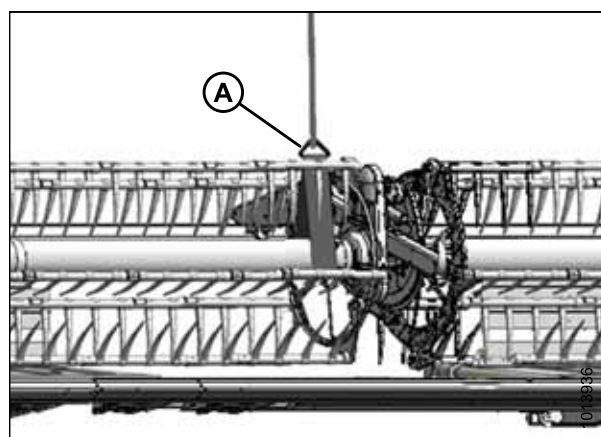
Рисунок 5.319: Вывешивание подбирающего мотвила
