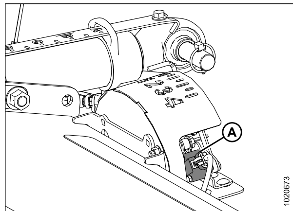
Рисунок 3.154: Блок индикатора флотации
