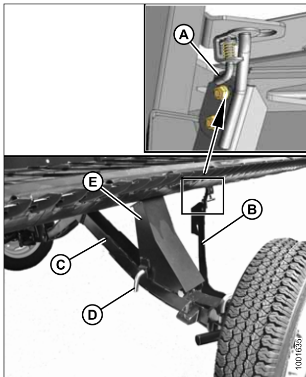
Рисунок 3.419: Правый задний рычаг
