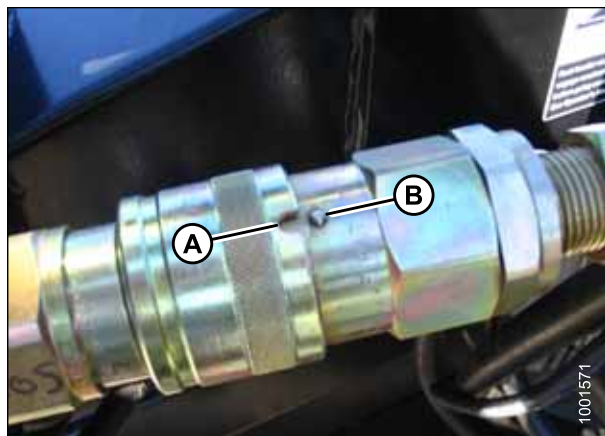
Рисунок 4.116: Быстроразъемное муфтовое соединение
