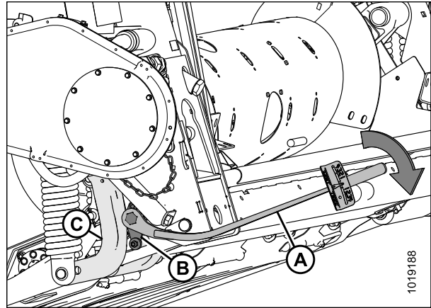
Рисунок 3.82: левая сторона
