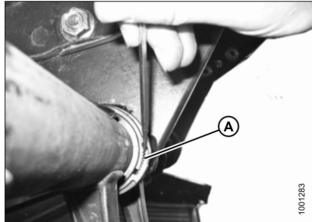
Рисунок 5.268: Хомут втулки
