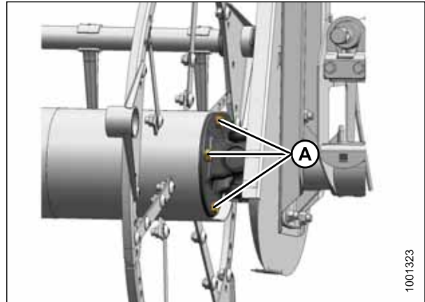
Рисунок 5.327: Крестовина
