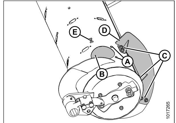
Рисунок 3.50: Широкая конфигурация (правая сторона)
