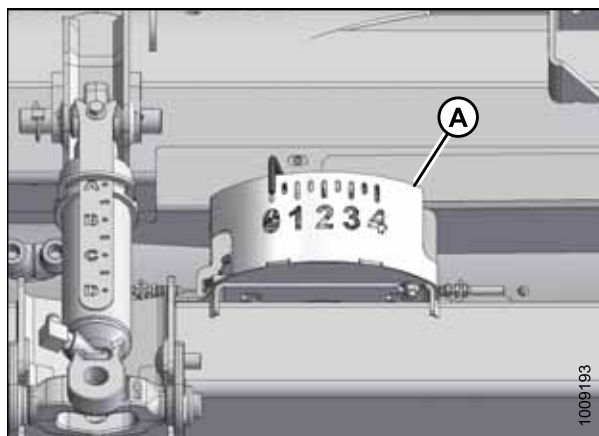
Рисунок 3.75: Индикатор флотации
