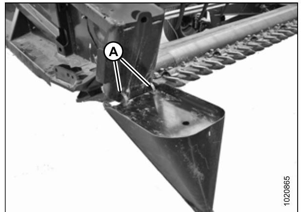
Рисунок 3.141: Делитель
