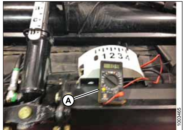
Рисунок 3.158: Измерение напряжения на блоке индикатора флотации
