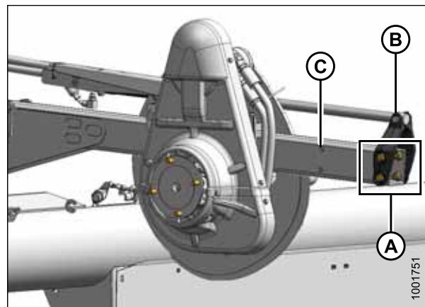
Рисунок 3.107: Правый рычаг — переднее положение
