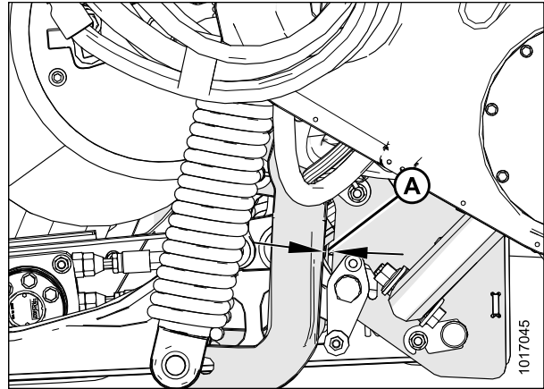
Рисунок 3.407: Угловой рычаг
