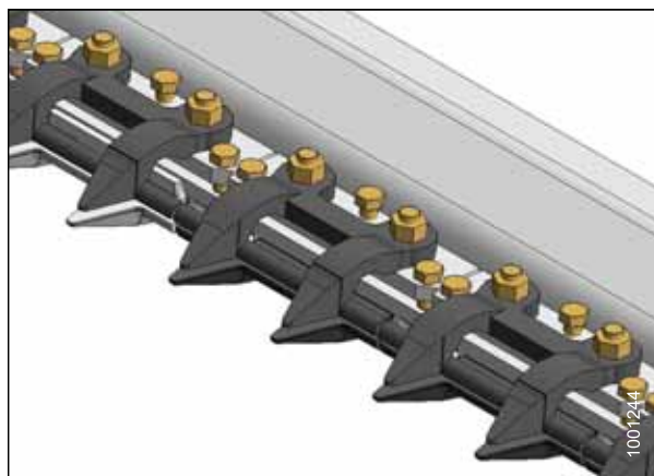
Рисунок 6.9: Сдвоенные противорежущие пальцы
