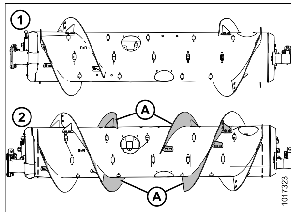
Рисунок 3.60: Конфигурации шнека (вид сзади)
