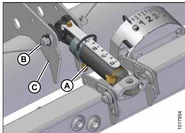
Рисунок 4.98: Центральное соединение
