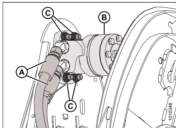
Рисунок 5.320: Мотор и шланги подбирающего мотовила
