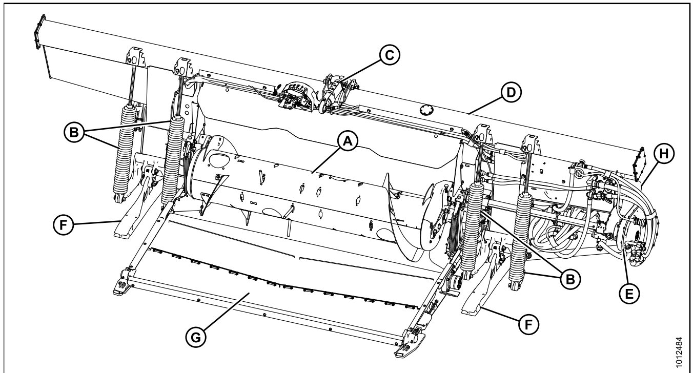
Рисунок 2.3: Модуль флотации FM100 со стороны жатки
