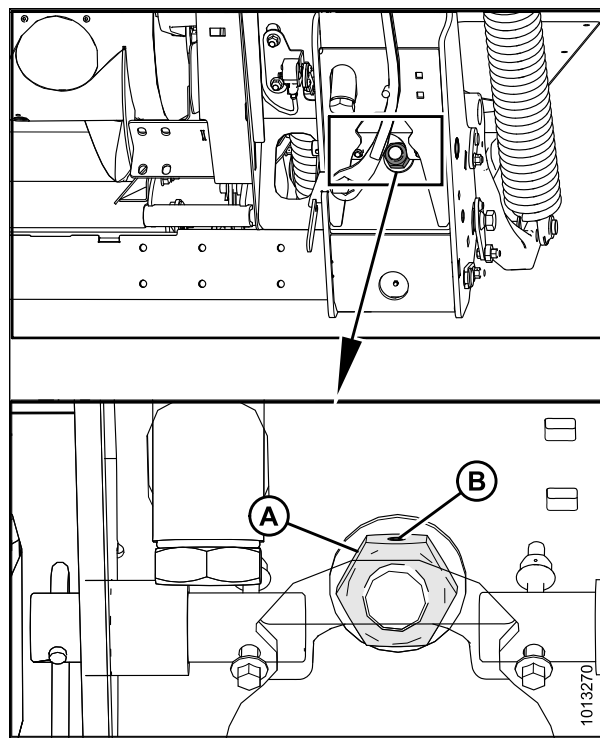
Рисунок 3.406: Блокировка флотации
