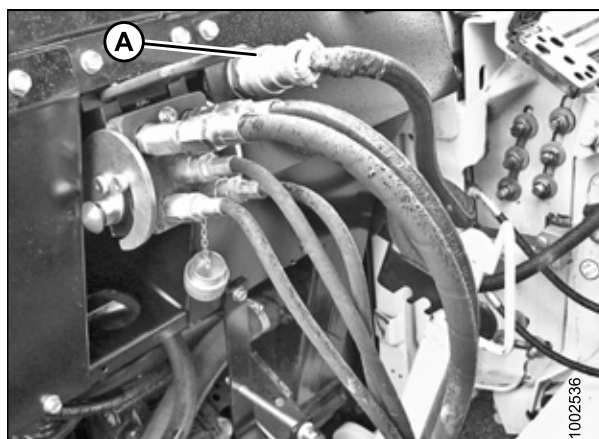
Рисунок 4.88: Соединения модуля флотации
