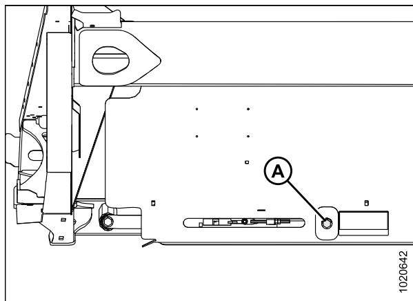
Рисунок 5.230: Натяжитель
