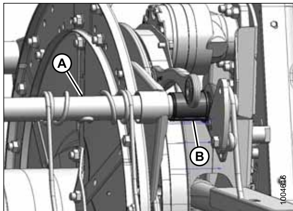
Рисунок 5.286: Сторона эксцентрика
