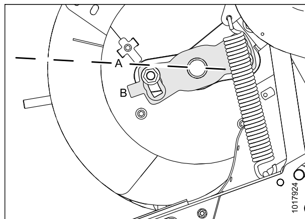
Рисунок 5.82: Настройка А шнека
