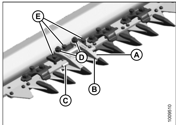
Рисунок 5.107: Прижим центрального противорезущего пальца
