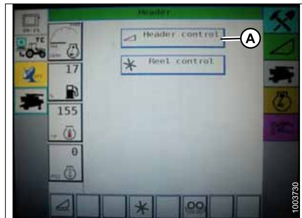
Рисунок 3.214: Приборная панель комбайна Challenger
