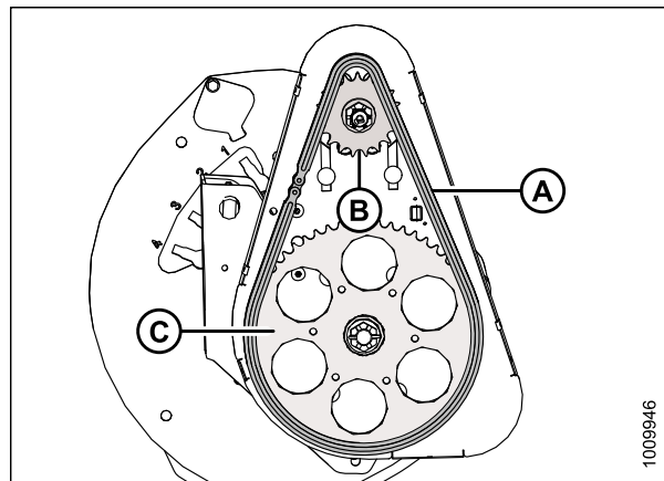
Рисунок 5.329: Привод подбирающего мотовила
