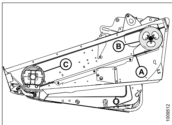
Рисунок 5.133: Привод ножа
