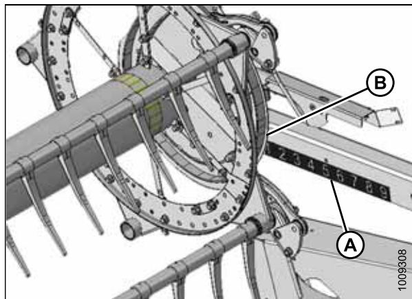
Рисунок 3.101: Шкала продольного смещения
