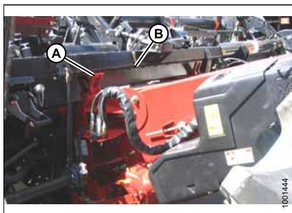
Рисунок 4.2: Комбайн и модуль флотации
