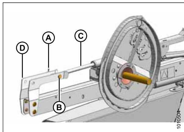
Рисунок 3.118: Правый рычаг мотовила в заднем положении
