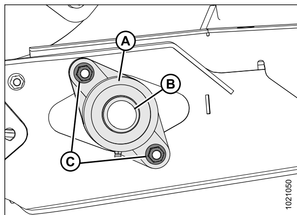
Рисунок 5.183: Подшипник приводного ролика подающего полотна
