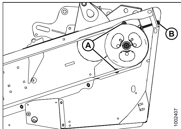
Рисунок 5.116: Привод двойного ножа без синхронизации
