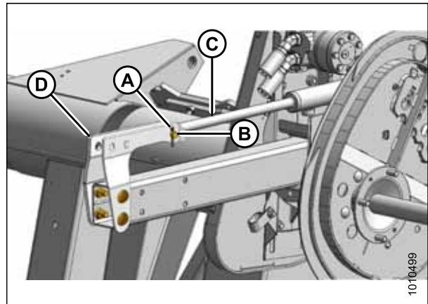
Рисунок 3.116: Центральный рычаг мотовила в заднем положении
