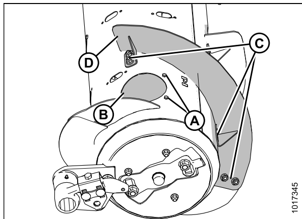
Рисунок 3.24: Узкая конфигурация (правая сторона)
