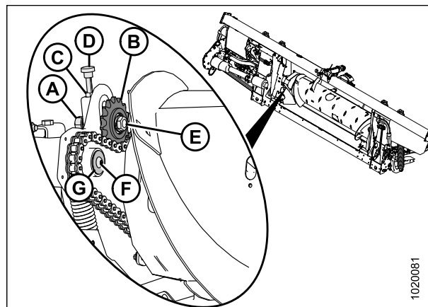
Рисунок 5.57: Привод шнека
