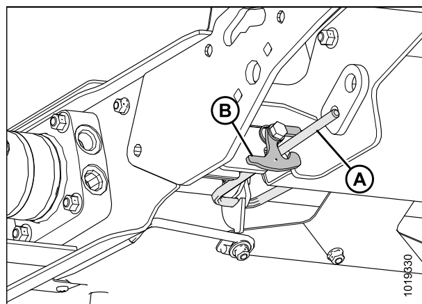
Рисунок 5.164: Ручка поддона направляющей подачи и защелка ручки поддона левой стороны
