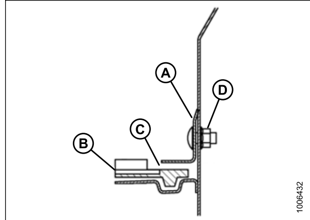
Рисунок 5.209: Уплотнение полотна
