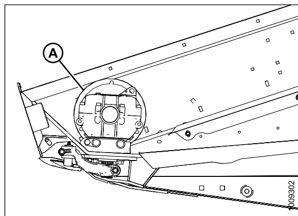
Рисунок 3.94: Шкив привода ножа
