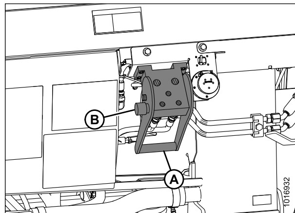
Рисунок 4.18: Гнездо модуля флотации
