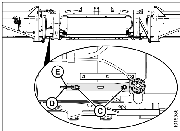
Рисунок 5.215: Приводной ролик левой направляющей (показан левый, правый напротив)
