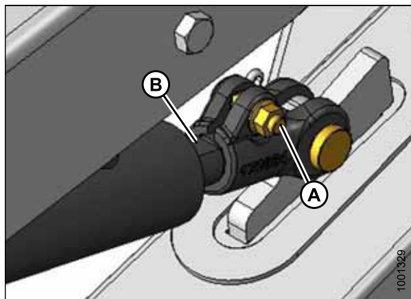
Рисунок 5.249: Внешний рычаг подбирающего мотовила
