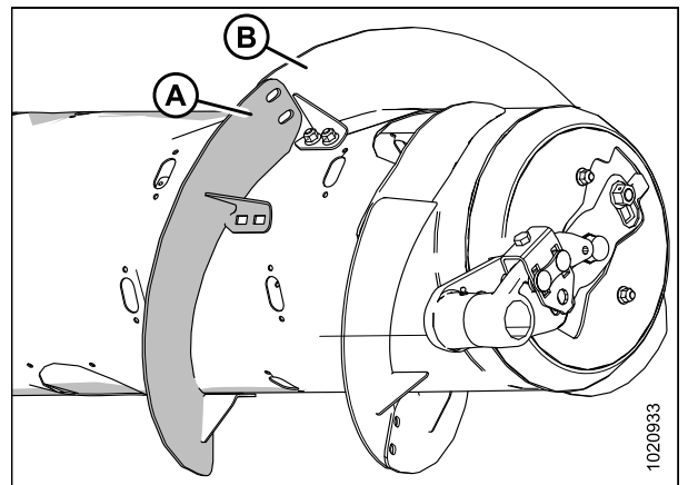
Рисунок 3.65: Витки спирали на правой стороне шнека
