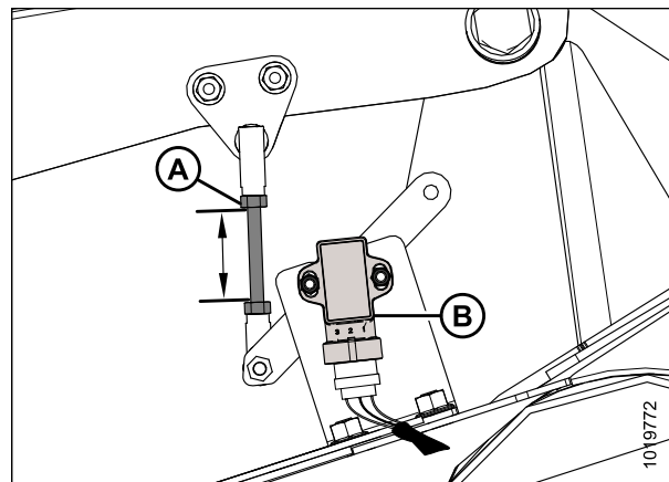
Рисунок 3.95: Датчик высоты мотовила — правый рычаг мотовила (мотовило вниз)
