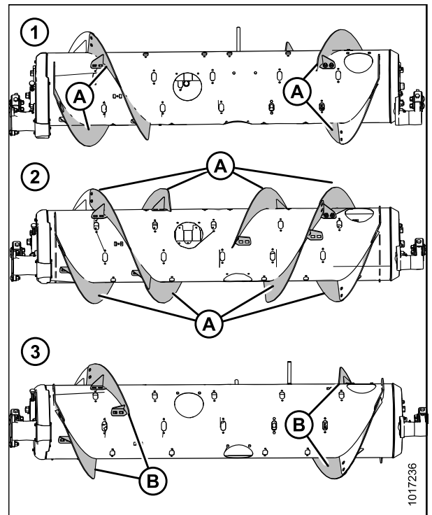
Рисунок 3.23: Конфигурации шнека (вид сзади)
