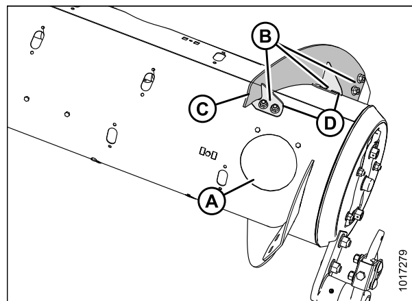
Рисунок 3.48: Широкая конфигурация (правая сторона)
