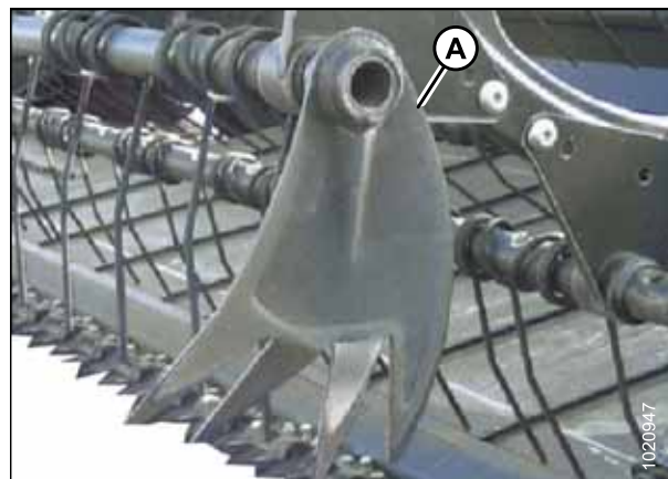
Рисунок 6.4: Пальцы для полеглых культур
