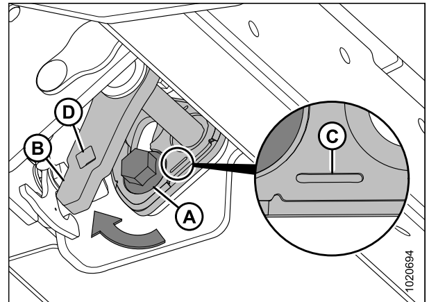
Рисунок 3.151: Рычаг регулировки флотации шнека — левая сторона
