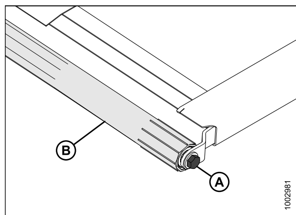
Рисунок 5.233: Приводной ролик
