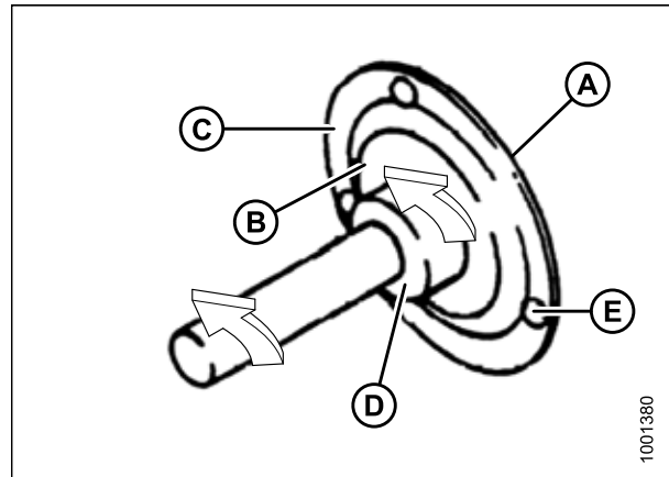
Рисунок 5.1: Герметизированный подшипник
