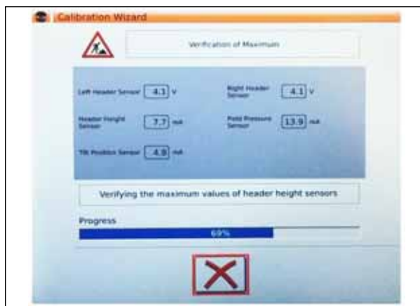
Рисунок 3.255: Выполнение калибровки
