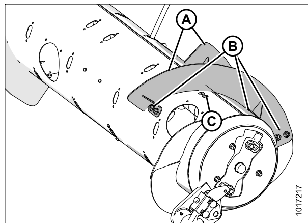
Рисунок 3.36: Узкая конфигурация (правая сторона)
