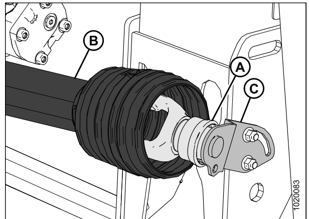
Рисунок 4.10: Привод
