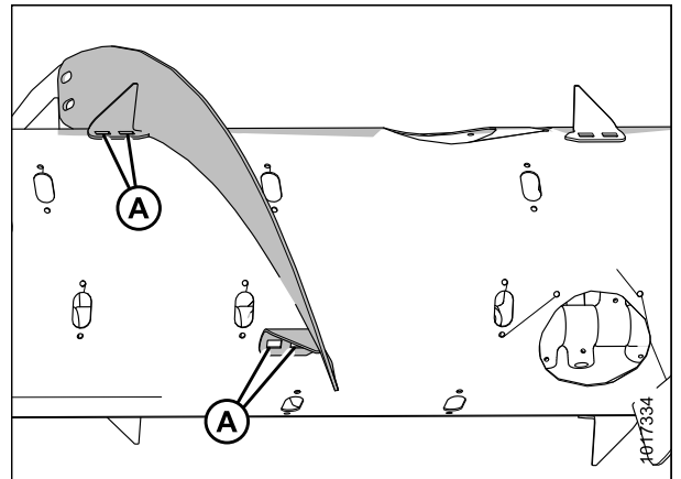
Рисунок 3.64: Витки спирали на левой стороне шнека
