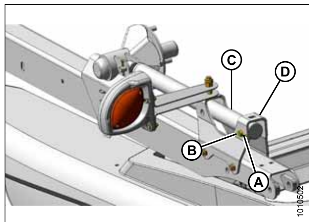
Рисунок 3.114: Левый рычаг мотовила в заднем положении
