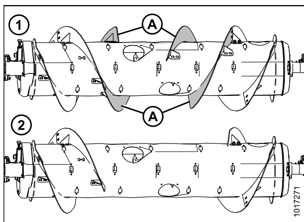
Рисунок 3.38: Конфигурации шнека (вид сзади)
