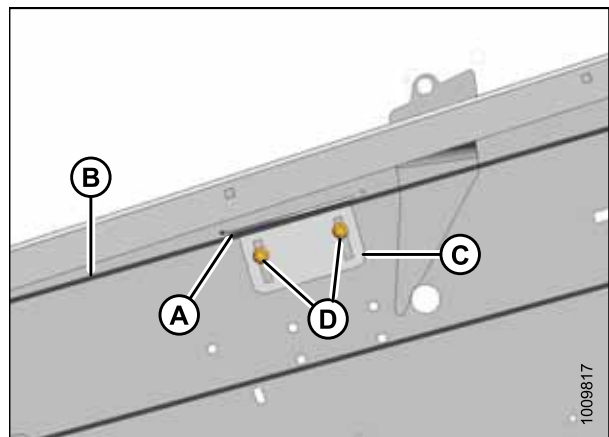
Рисунок 5.150: Направляющая ремня – левая сторона
