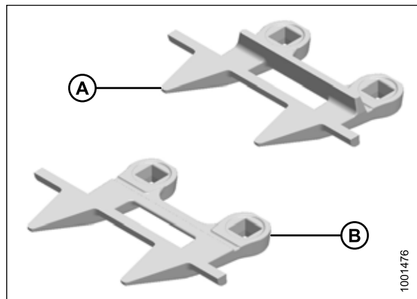
Рисунок 5.104: Сдвоенные противорезущие пальцы
