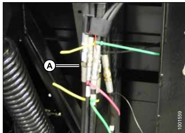
Рисунок 4.99: Гидравлическая система подбирающего мотвила
