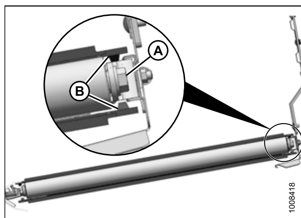
Рисунок 5.212: Натяжной ролик
