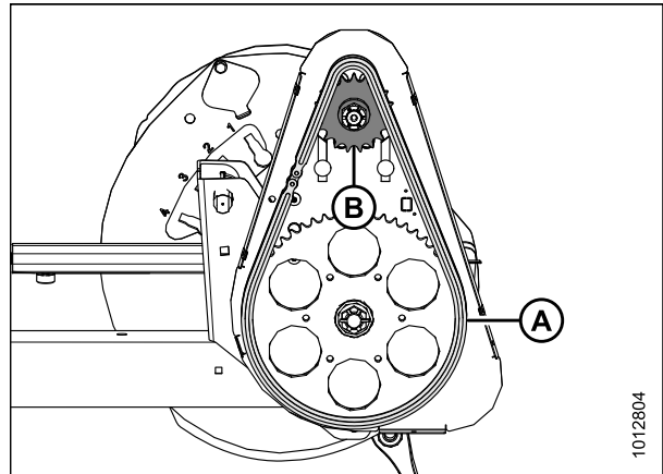
Рисунок 5.314: Привод подбирающего мотовила
