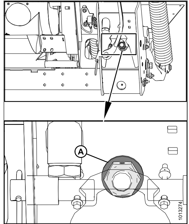
Рисунок 3.374: Блокировка флотации
