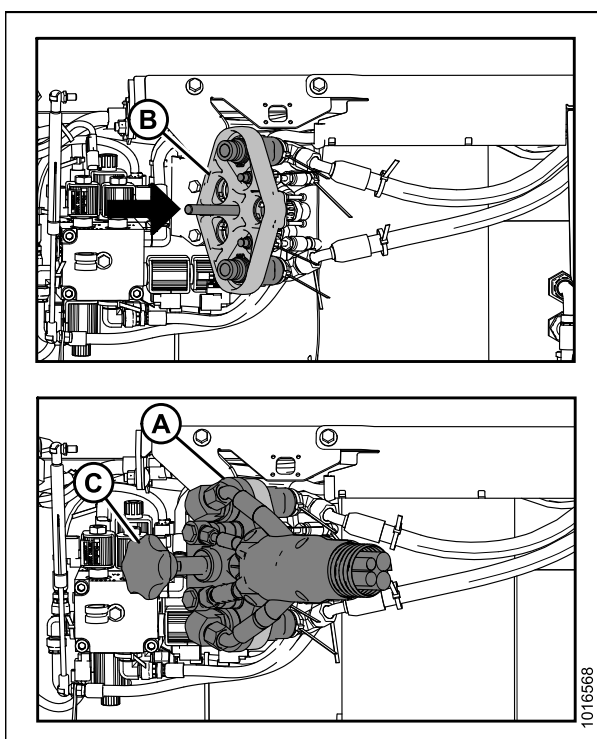
Рисунок 4.61: Муфта
