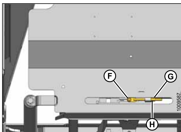
Рисунок 5.216: Натяжной ролик левой направляющей (показан левый, правый напротив)
