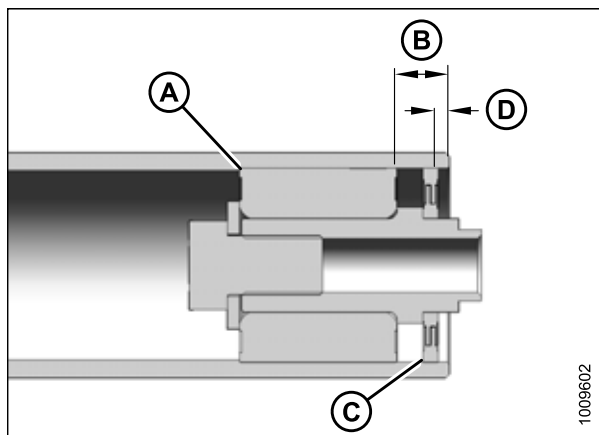
Рисунок 5.235: Подшипник натяжного ролика
