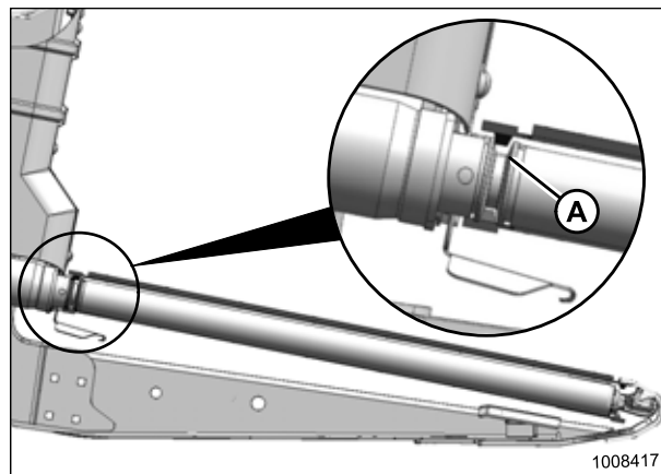
Рисунок 5.211: Приводной ролик
