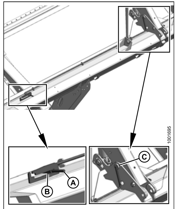
Рисунок 3.4: Предохранительный упор подбирающего мотовила — центральный рычаг
