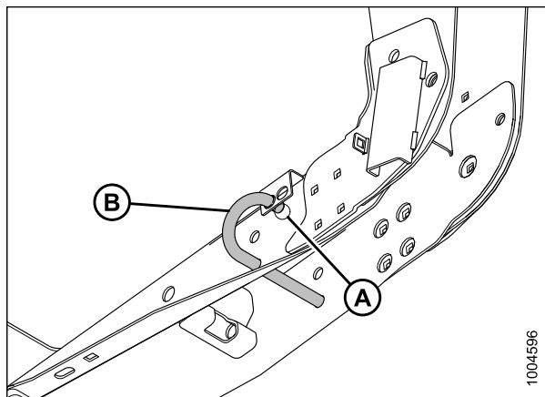
Рисунок 4.119: Опора жатки
