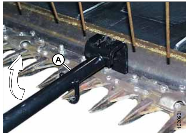
Рисунок 5.96: Правка вверх
