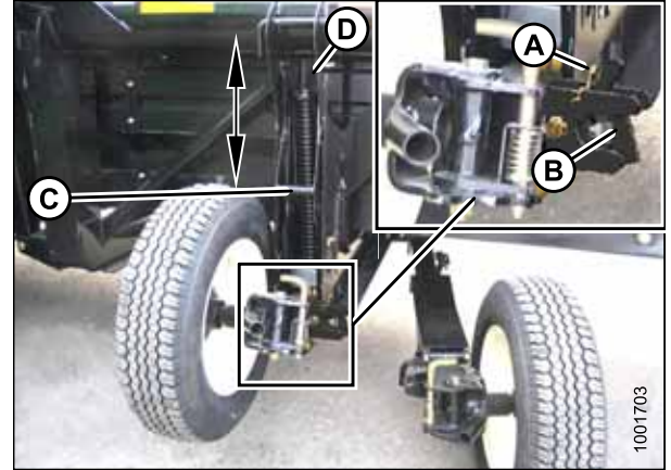
Рисунок 3.66: Правое колесо
