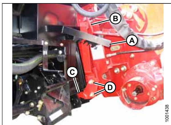
Рисунок 4.3: Комбайн и модуль флотации
