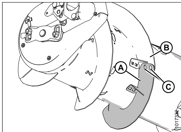
Рисунок 3.61: Левая сторона шнека
