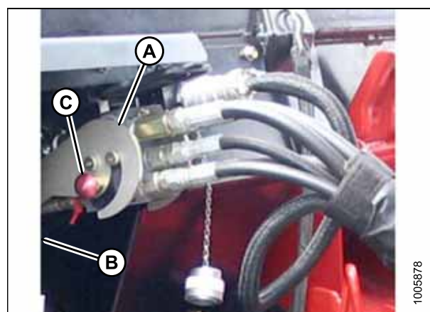
Рисунок 4.6: Гидравлическое соединение
