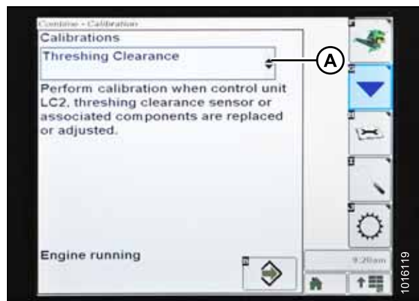
Рисунок 3.318: Дисплей комбайна John Deere
