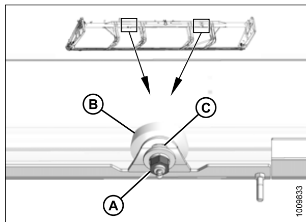
Рисунок 5.159: Опора поперечного вала
