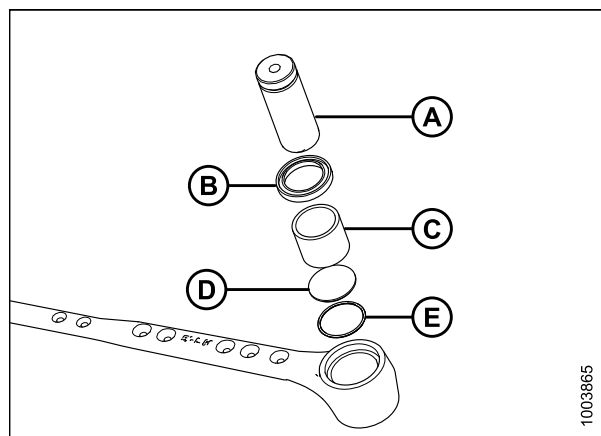
Рисунок 5.92: Подшипник головки ножа в сборе
