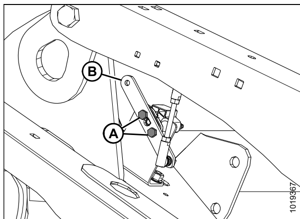
Рисунок 3.99: Датчик высоты мотовила — правый рычаг мотовила
