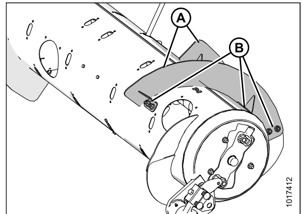
Рисунок 3.52: Правая сторона шнека
