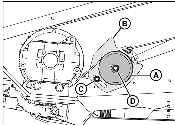
Рисунок 5.145: Привод ножа
