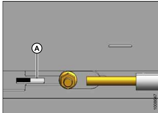
Рисунок 5.210: Показан левый регулятор натяжения — правый находится на противоположной стороне
