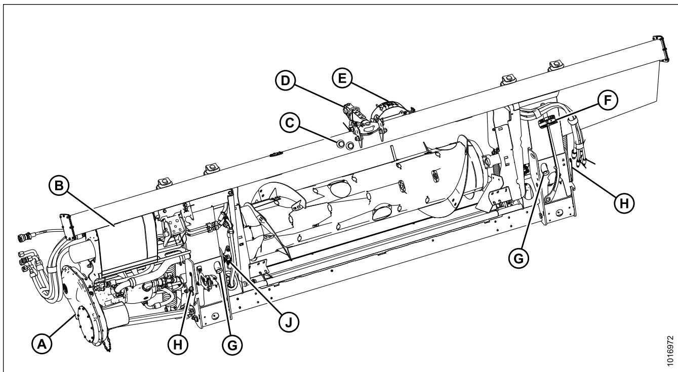
Рисунок 2.4: Модуль флотации FM100 со стороны комбайна
