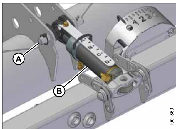
Рисунок 4.114: Гидравлическое центральное звено
