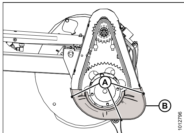
Рисунок 5.303: Нижняя крышка привода — сдвоенное мотовило
