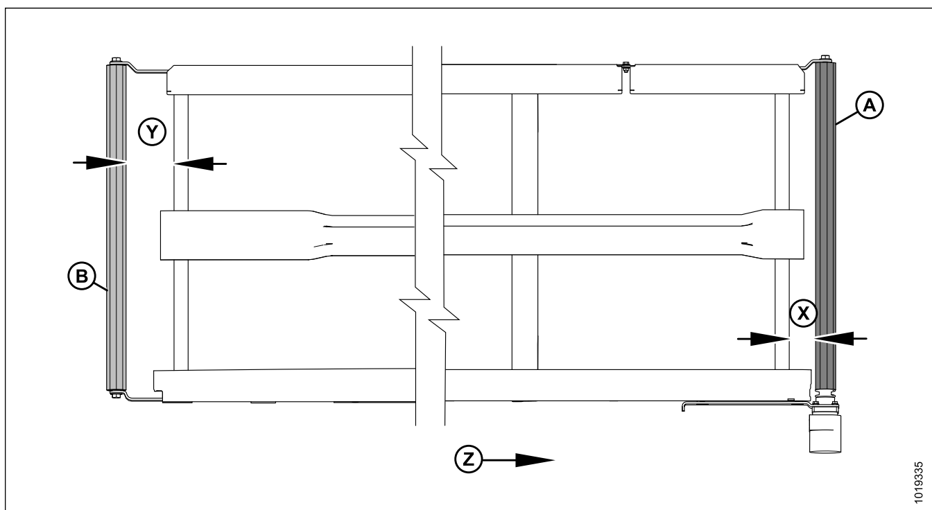
Рисунок 5.214: Регулировки хода полотна
