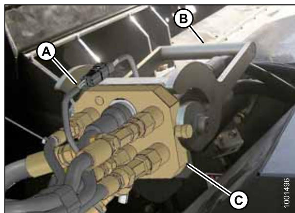
Рисунок 4.34: Многоканальная муфта
