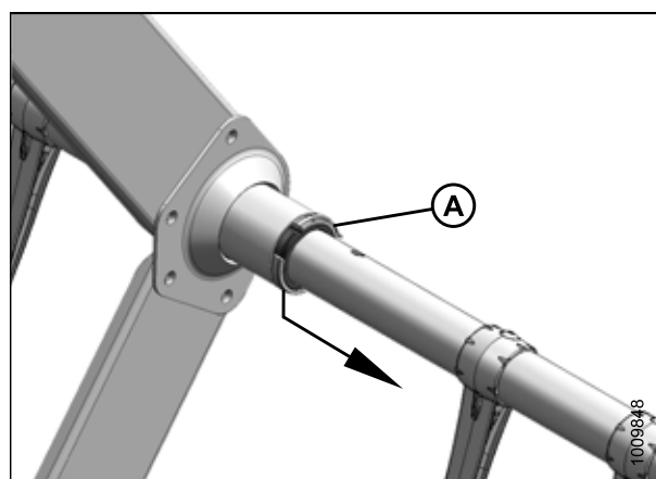
Рисунок 5.272: Хомут втулки
