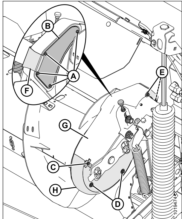
Рисунок 5.56: Привод шнека
