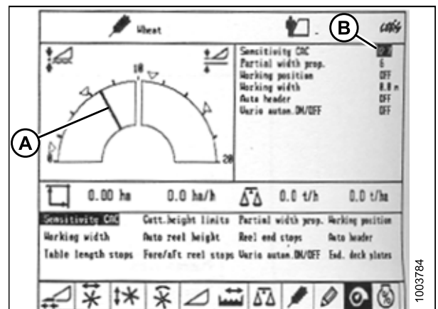
Рисунок 3.326: Приборная панель комбайна CLAAS
