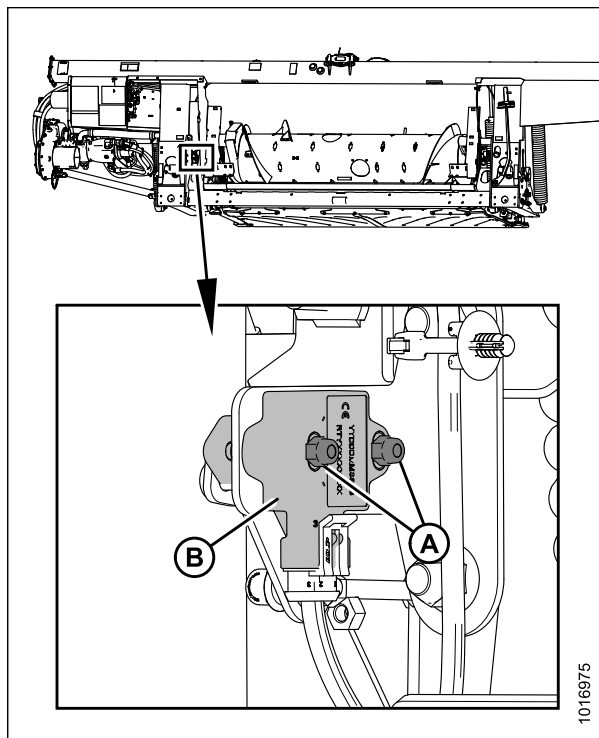
Рисунок 3.167: Дополнительный комплект с двумя датчиками — левый датчик
