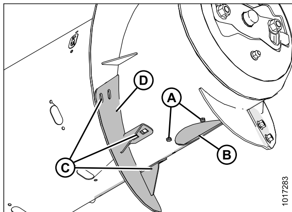
Рисунок 3.41: Правая сторона в средней конфигурации
