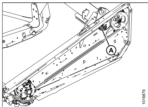
Рисунок 5.95: Запасной нож
