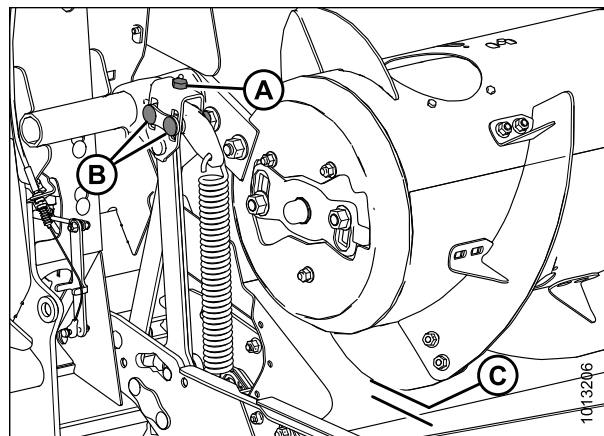
Рисунок 5.52: Зазор шнека
