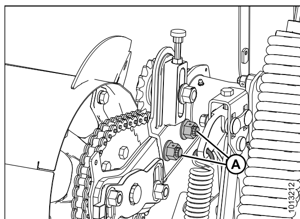
Рисунок 5.64: Привод шнека
