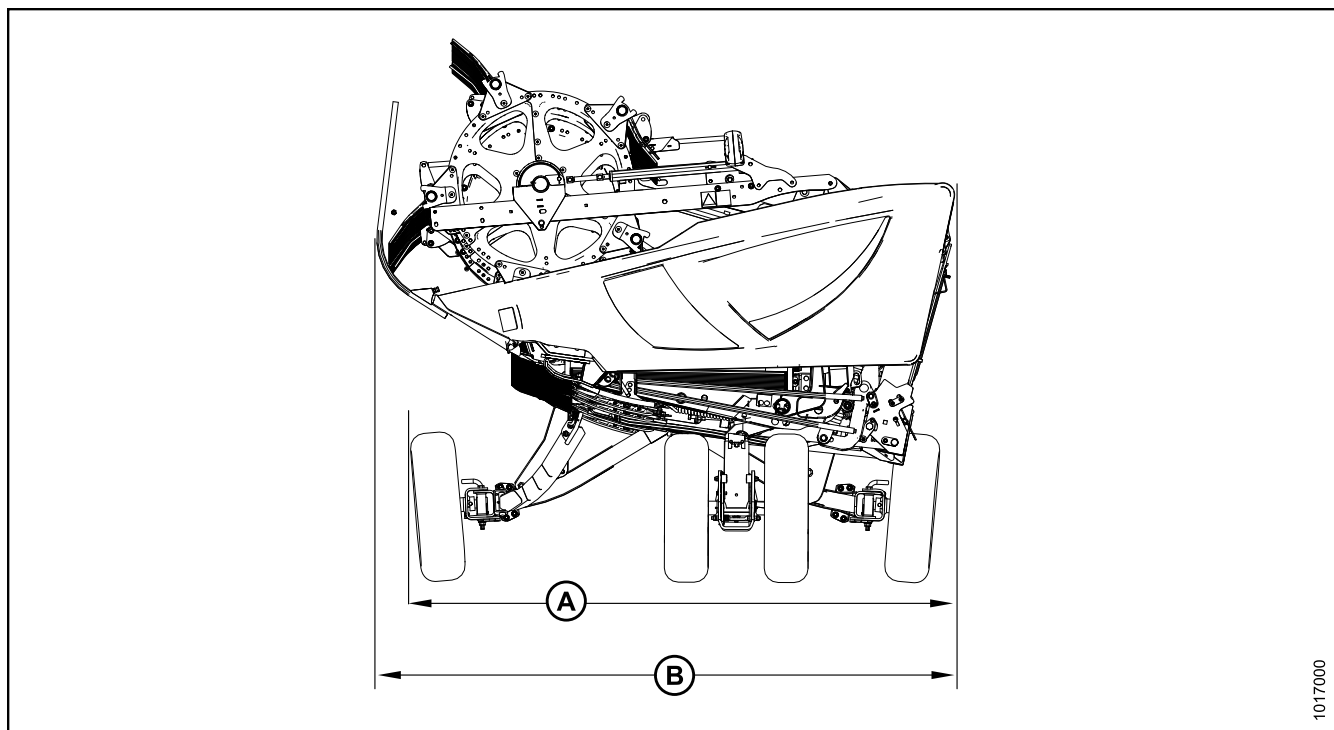
Рисунок 2.1: Ширина жатки
