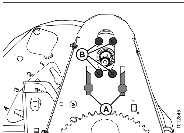
Рисунок 5.321: Монтажные отверстия мотора привода подбирающего мотовила
