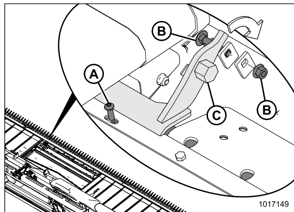
Рисунок 4.102: Защелка модуля флотации
