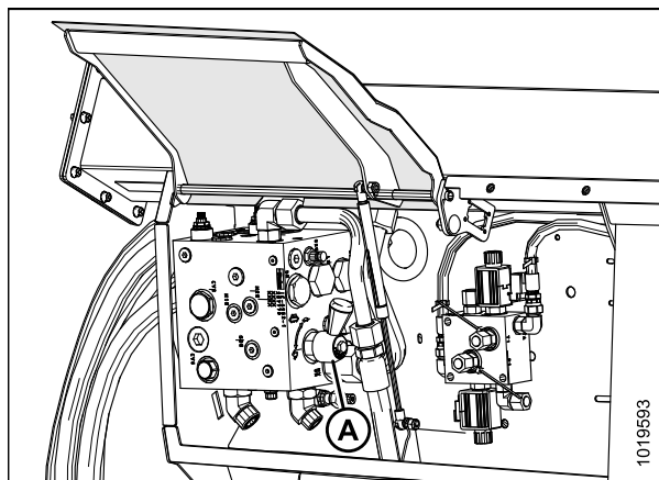
Рисунок 3.91: Распределительный клапан (некоторые детали убраны для наглядности)
