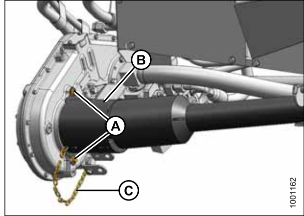
Рисунок 5.34: Кардан привода жатки на стороне модуля флотации
