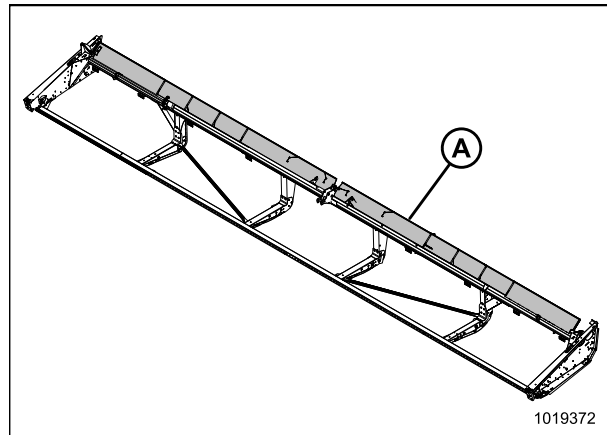
Рисунок 6.13: Удлинители заднего щитка
