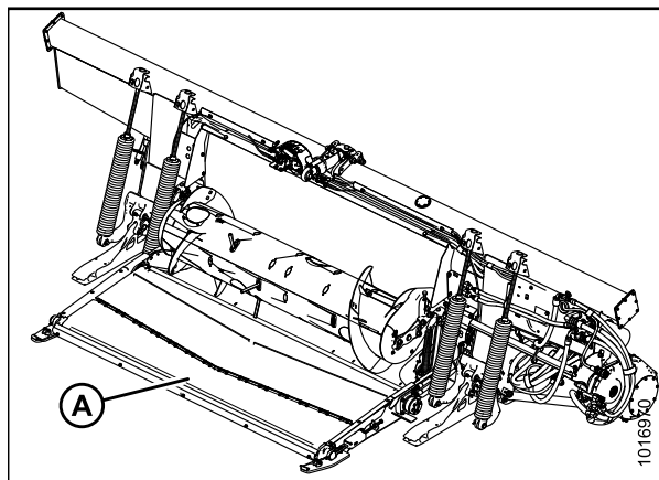
Рисунок 3.92: Модуль флотации FM100
