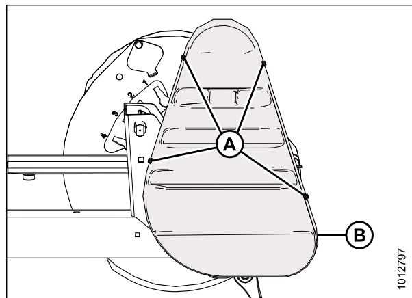
Рисунок 5.299: Крышка привода — единое мотовило
