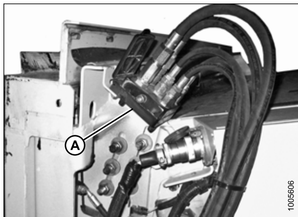
Рисунок 4.77: Муфта комбайна
