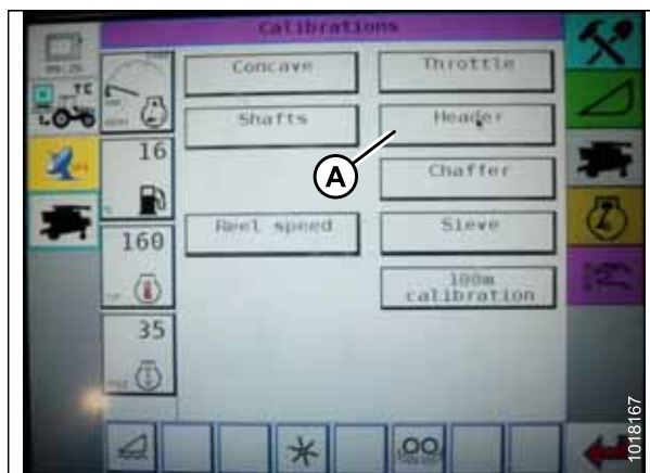
Рисунок 3.209: Приборная панель комбайна Challenger
