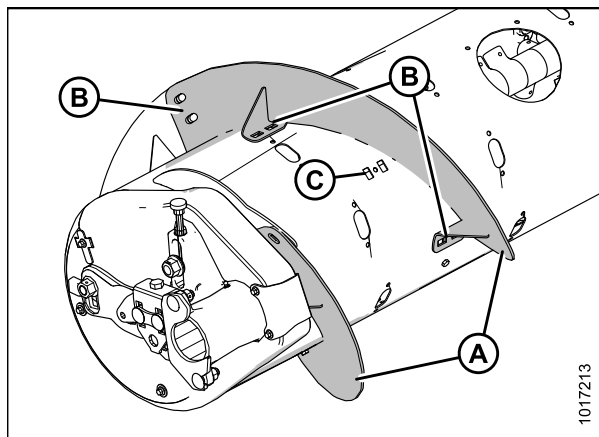
Рисунок 3.37: Узкая конфигурация (левая сторона)
