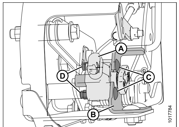
Рисунок 3.404: Датчик АННС
