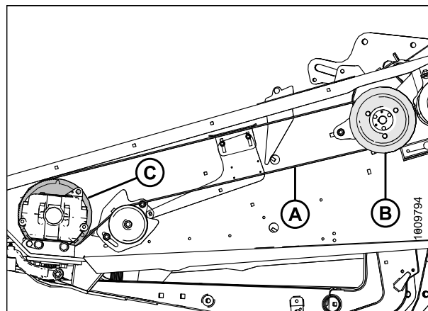
Рисунок 5.143: Показана левая сторона – Правая сторона аналогична
