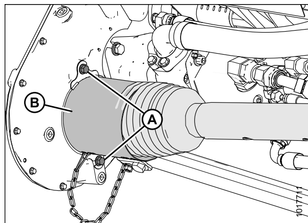
Рисунок 5.37: Кардан привода жатки на стороне модуля флотации
