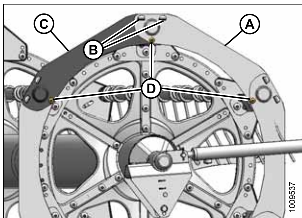
Рисунок 5.296: Боковые щитки подбирающего мотовила
