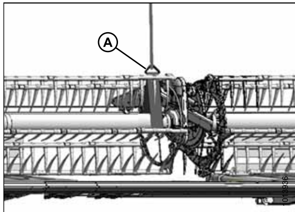
Рисунок 5.315: Вывешивание подбирающего мотовила
