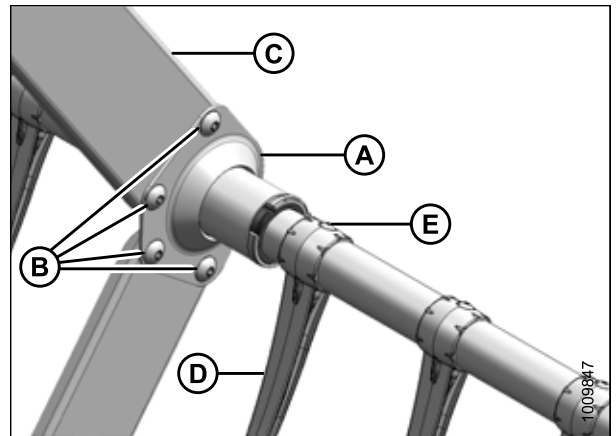
Рисунок 5.291: Опора
