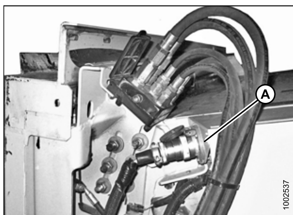
Рисунок 4.89: Муфты комбайна
