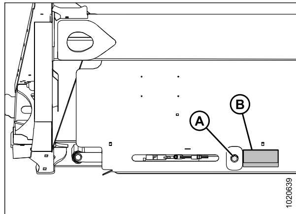
Рисунок 5.239: Натяжение полотна (показана левая сторона, правая сторона напротив)
