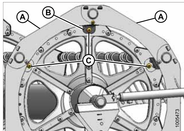
Рисунок 5.298: Опоры боковых щитков подбирающего мотовила
