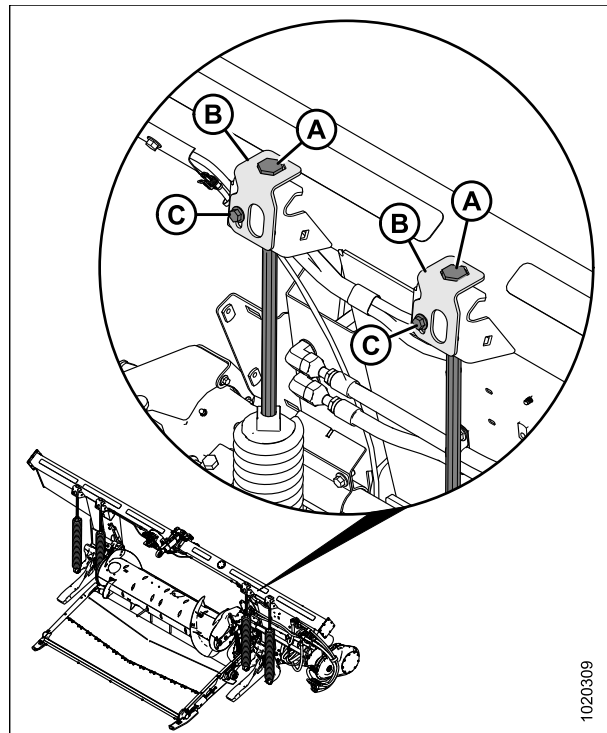
Рисунок 3.85: Регулировка флотации (на рисунке показана левая сторона)
