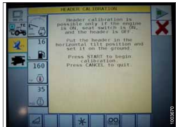
Рисунок 3.211: Приборная панель комбайна Challenger
