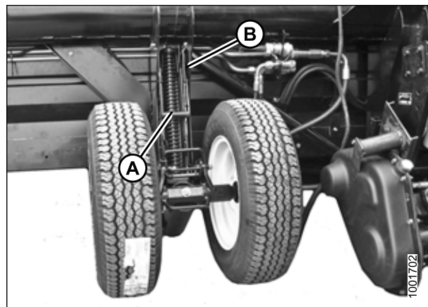
Рисунок 3.80: Левое колесо
