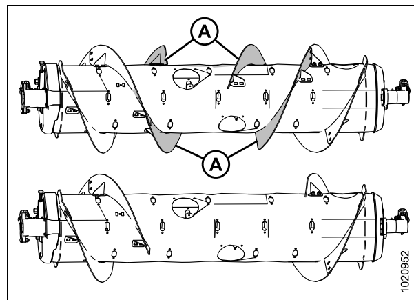
Рисунок 6.15: Витки подающего шнека FM100
