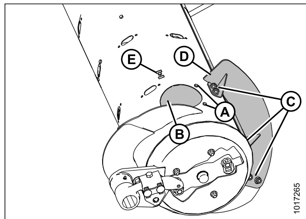
Рисунок 3.34: Широкая конфигурация (правая сторона)
