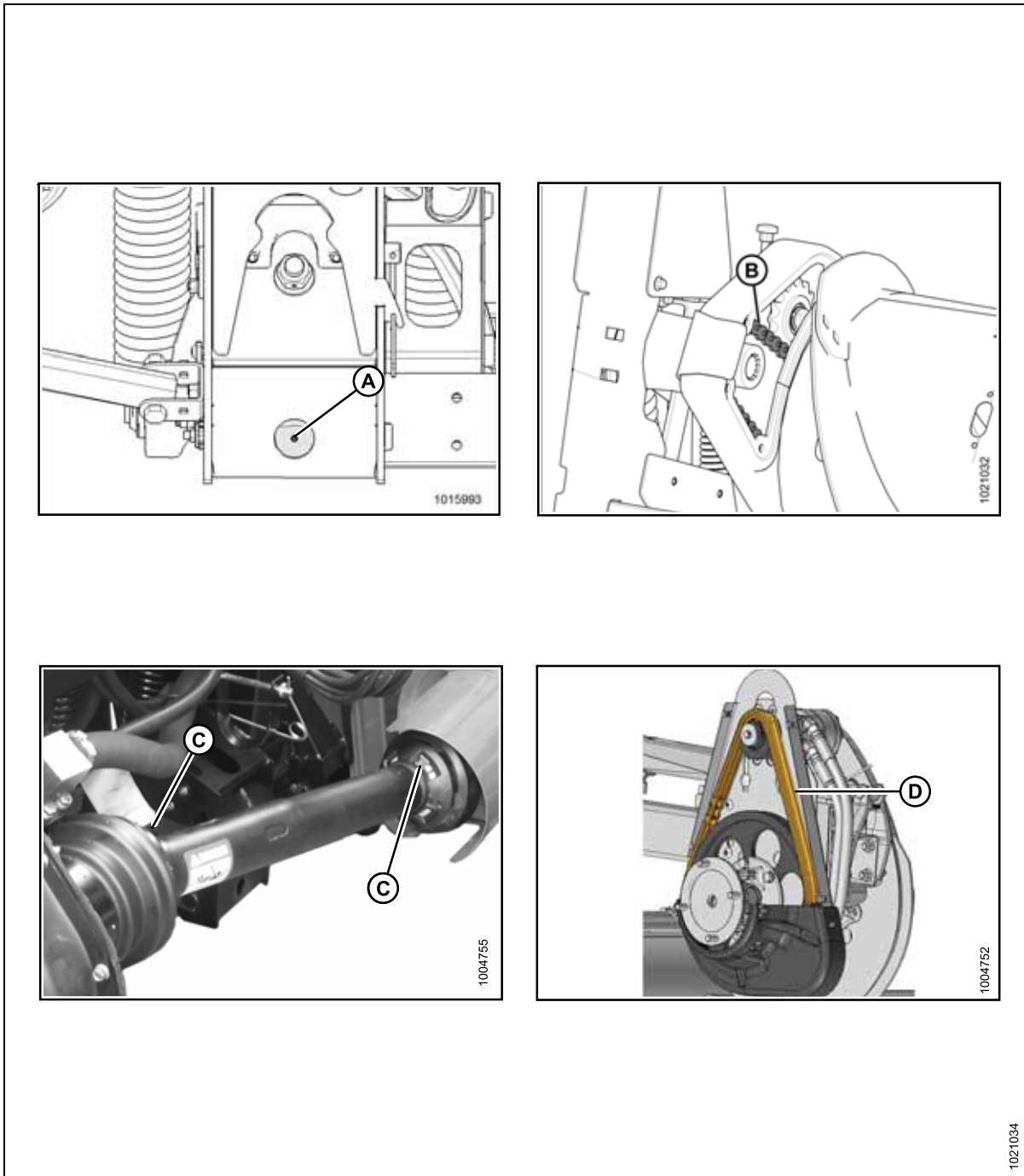
Рисунок 5.8: Каждые 100 часов
