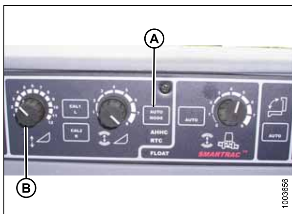
Рисунок 3.226: Консоль АННС
