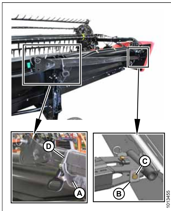
Рисунок 3.412: Хранение буксирной тяги — правая сторона
