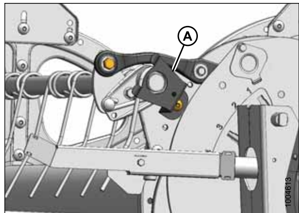
Рисунок 5.264: Страна эксцентрика
