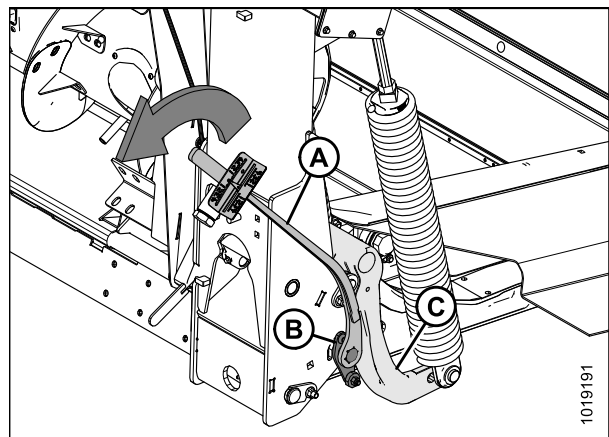
Рисунок 3.83: правая сторона
