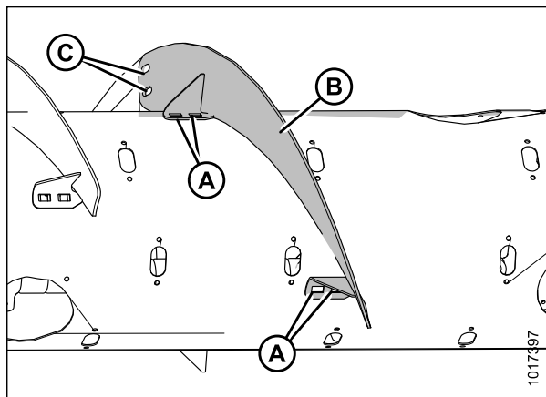
Рисунок 3.58: Левая сторона шнека
