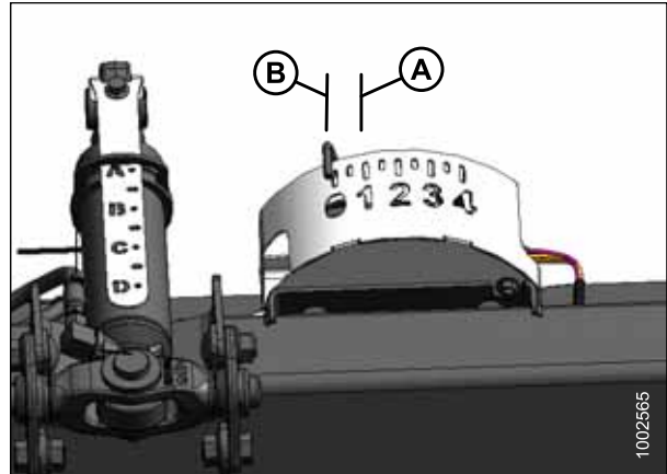
Рисунок 3.200: Блок индикатора флотации
