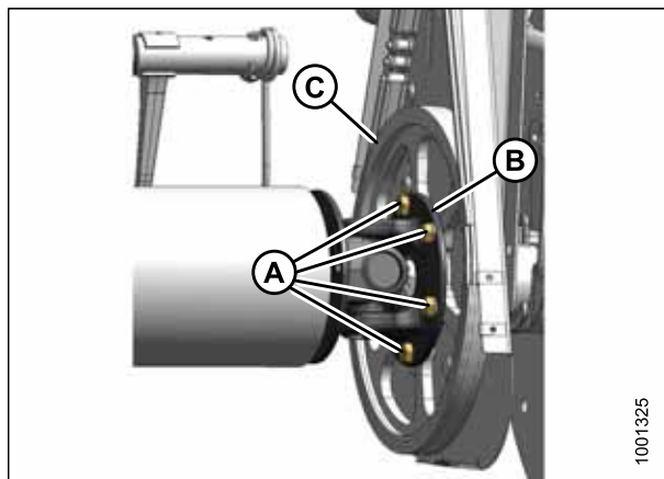
Рисунок 5.316: Крестовина
