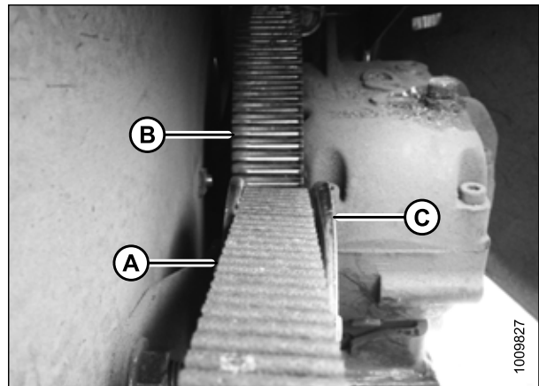
Рисунок 5.158: Ремень привода ножа
