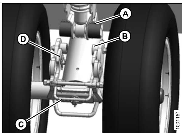
Рисунок 3.415: Передние (левые) колеса
