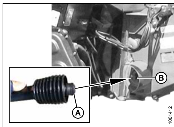
Рисунок 4.45: Привод
