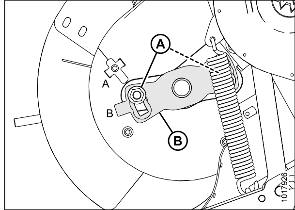
Рисунок 5.84: Индикатор синхронизации пальцев граблины шнека
