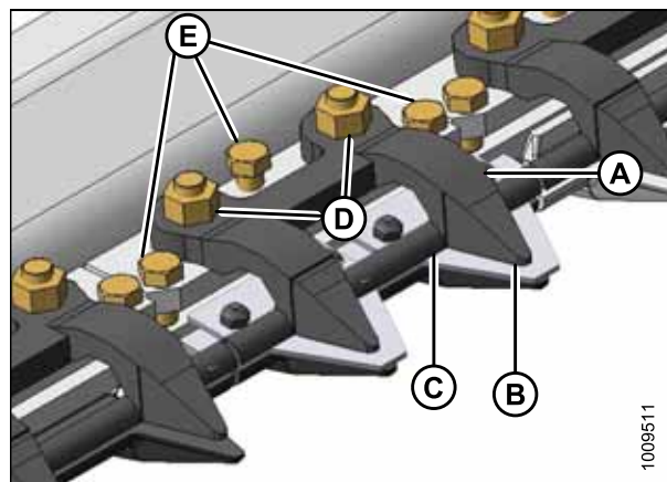
Рисунок 5.108: Сдвоенные противорежущие пальцы
