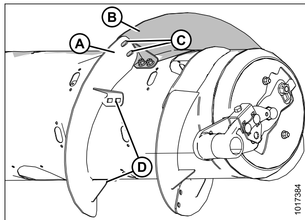
Рисунок 3.53: Правая сторона шнека
