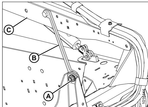
Рисунок 5.254: Опорный рычаг подбирающего мотовила
