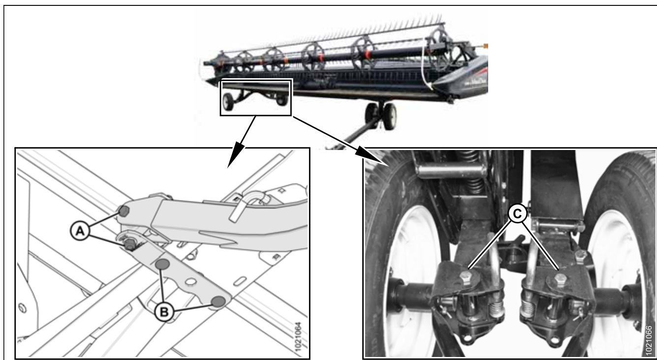
Рисунок 5.337: Болты рычагов
