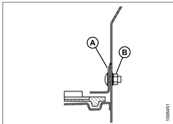
Рисунок 5.206: Уплотнение полотна
