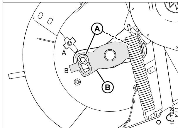
Рисунок 5.81: Индикатор синхронизации пальцев граблины шнека
