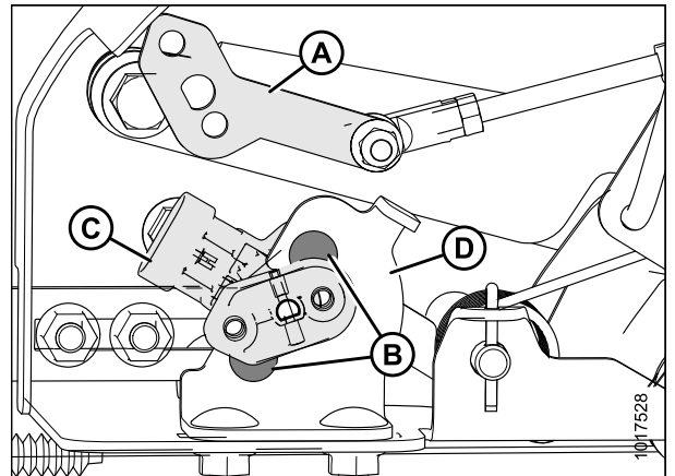
Рисунок 3.403: Датчик АННС
