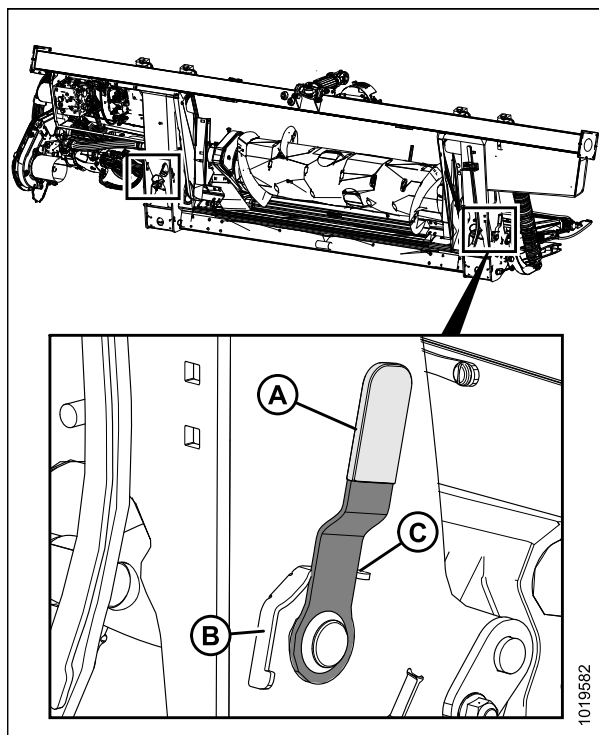
Рисунок 3.86: Замок флотации (в запертом положении)
