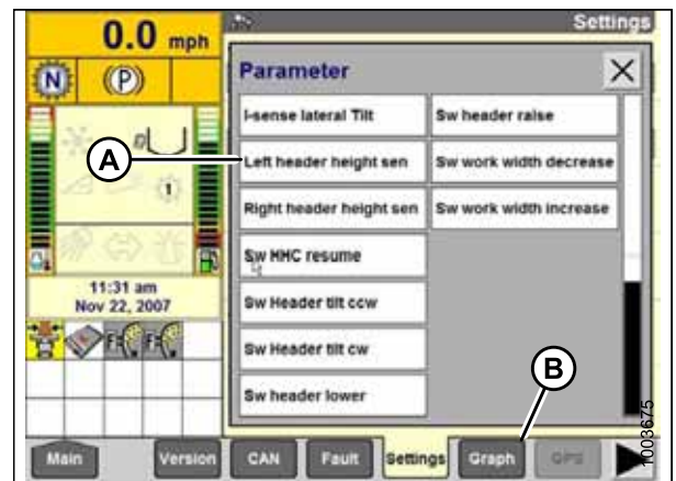
Рисунок 3.362: Приборная панель комбайнов New Holland
