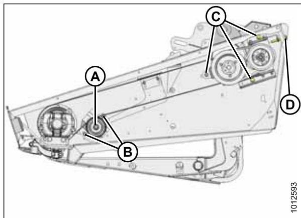
Рисунок 5.161: Привод ножа – левая сторона
