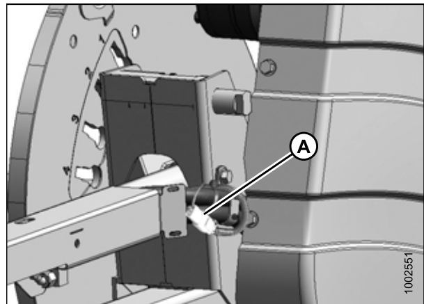
Рисунок 5.332: Жгут электропроводки
