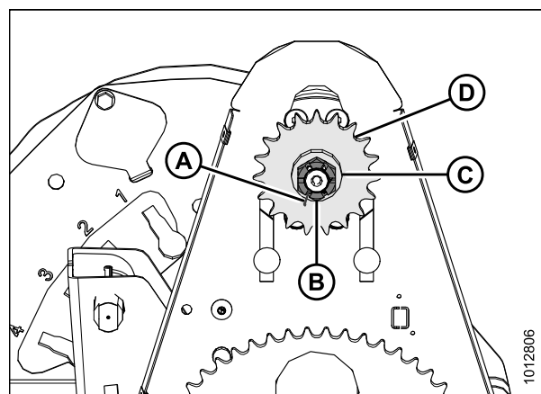
Рисунок 5.312: Привод подбирающего мотовила
