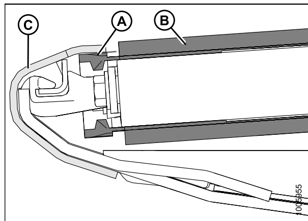
Рисунок 5.217: Уплотнение полотна
