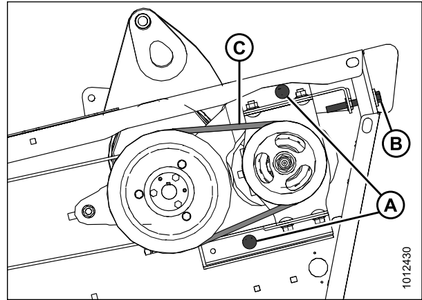
Рисунок 5.144: Клиновые ремни привода ножа
