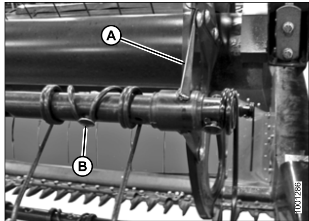
Рисунок 5.256: Граблина
