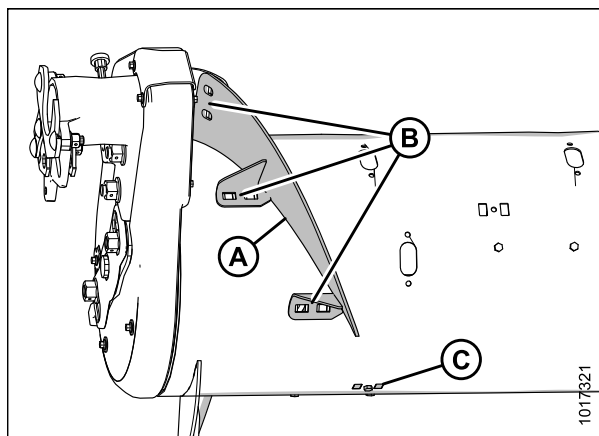
Рисунок 3.46: Широкая конфигурация (левая сторона)
