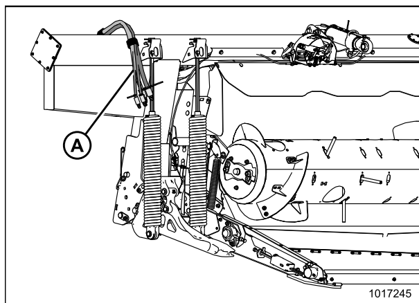
Рисунок 4.118: Место хранения шлангов
