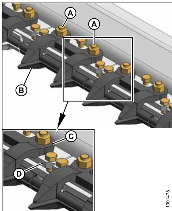
Рисунок 5.103: Сдвоенные противорежущие пальцы
