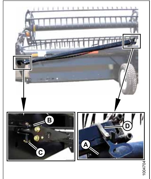
Рисунок 3.433: Снятие буксирной тяги — левая сторона
