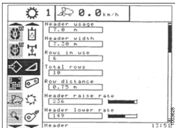
Рисунок 3.370: Приборная панель комбайнов New Holland
