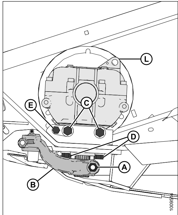
Рисунок 5.120: Редуктор привода ножа
