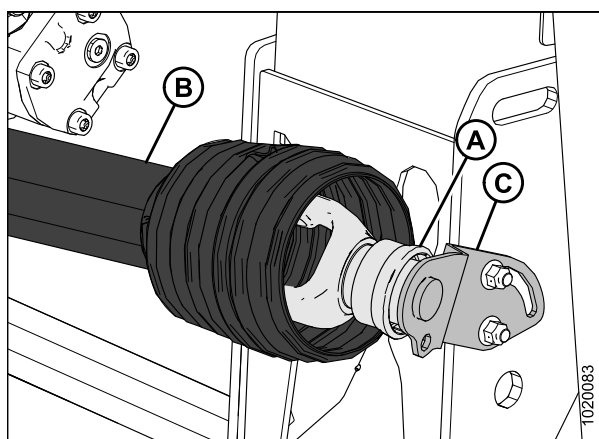
Рисунок 4.79: Привод
