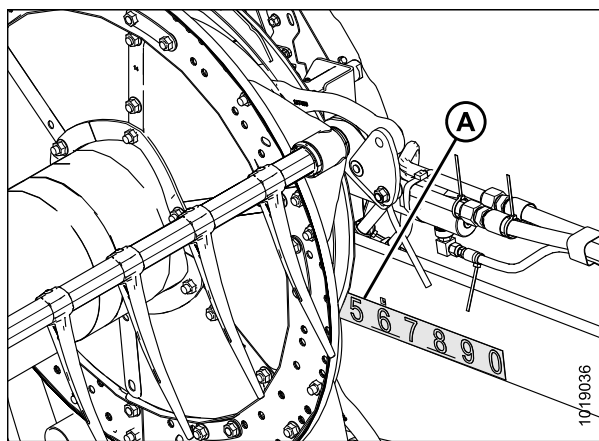
Рисунок 5.245: Продольное положение
