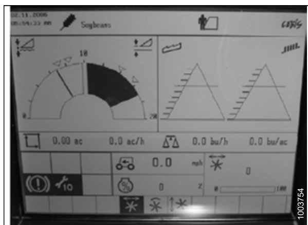
Рисунок 3.339: Приборная панель комбайна CLAAS
