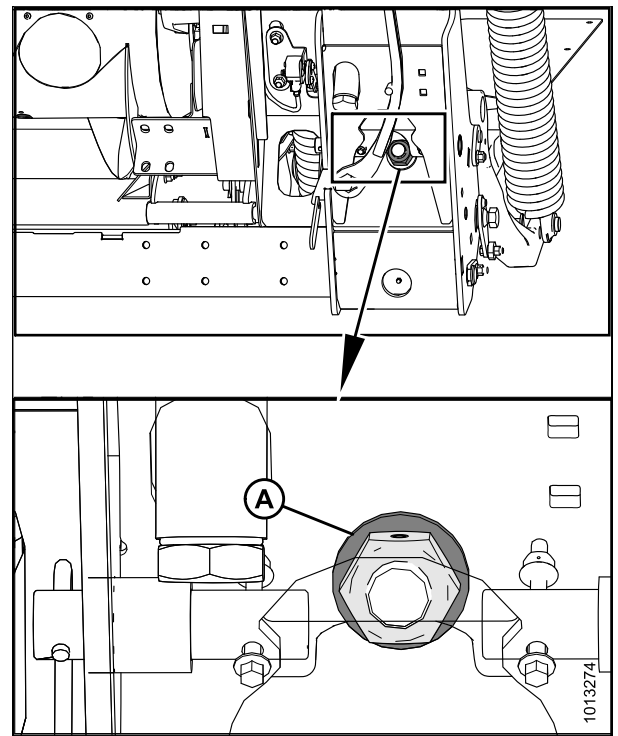
Рисунок 3.175: Блокировка флотации
