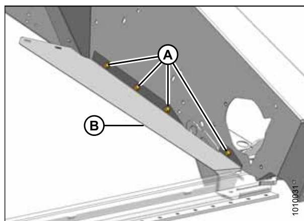
Рисунок 5.241: Передний дефлектор
