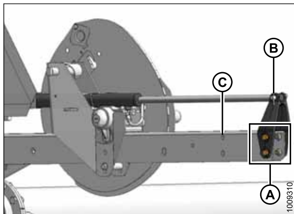
Рисунок 3.109: Цилиндр правого рычага мотовила в переднем положении
