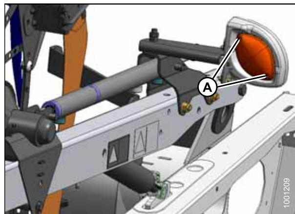
Рисунок 5.33: Транспортный фонарь
