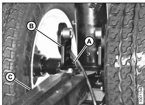
Рисунок 3.410: Защелка буксирной тяги
