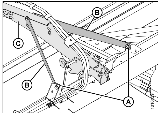
Рисунок 5.253: Центральный опорный рычаг подбирающего мотовила
