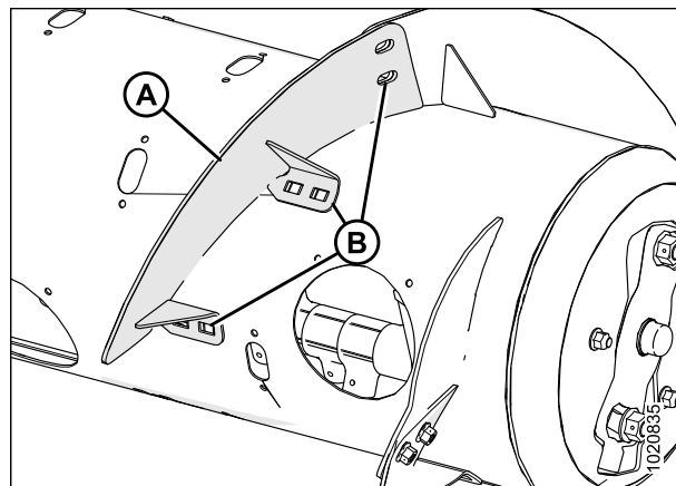
Рисунок 3.31: Средняя конфигурация (правая сторона)
