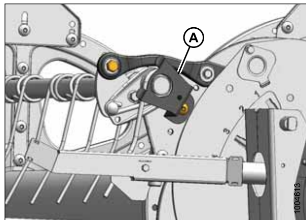
Рисунок 5.281: Страна эксцентрика
