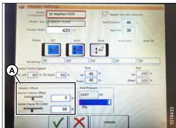
Рисунок 3.247: Настройки сдвига жатки
