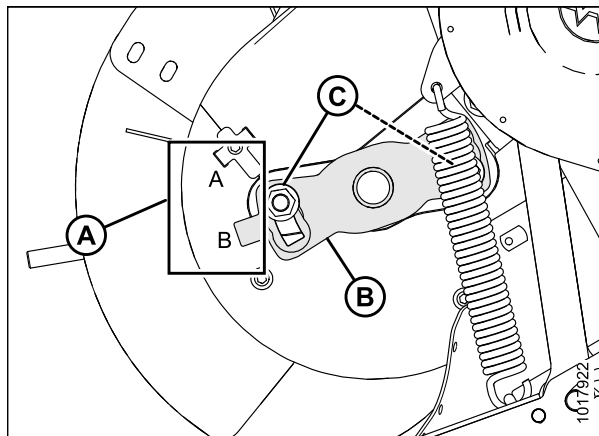
Рисунок 5.79: Синхронизация пальцев шнека (на рисунке показана левая сторона)
