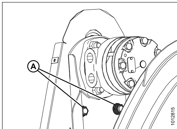
Рисунок 5.309: Изображен привод единого мотвила — привод сдвоенного мотвила имеет такую же конструкцию
