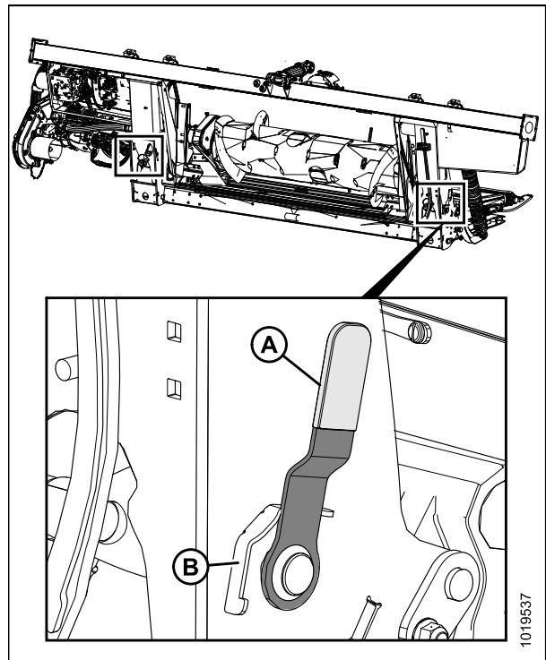
Рисунок 3.79: Замок флотации жатки (в запертом положении)
