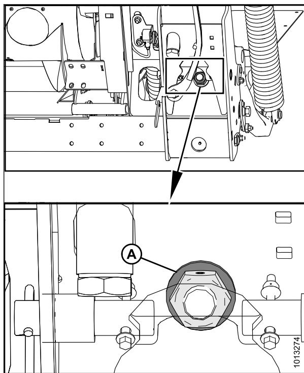
Рисунок 3.276: Блокировка флотации
