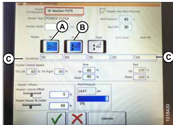
Рисунок 3.245: Органы автоматического управления и настройки чувствительности
