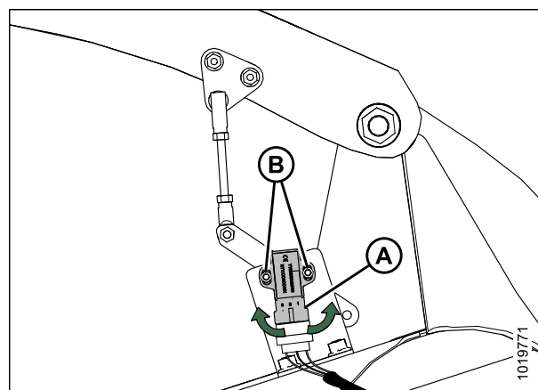
Рисунок 3.96: Датчик высоты мотовила — правый рычаг мотовила (мотовило вверх)
