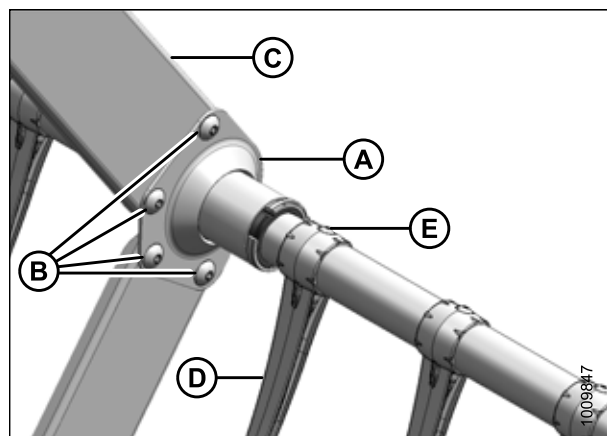
Рисунок 5.270: Опора трубы пальцев граблины
