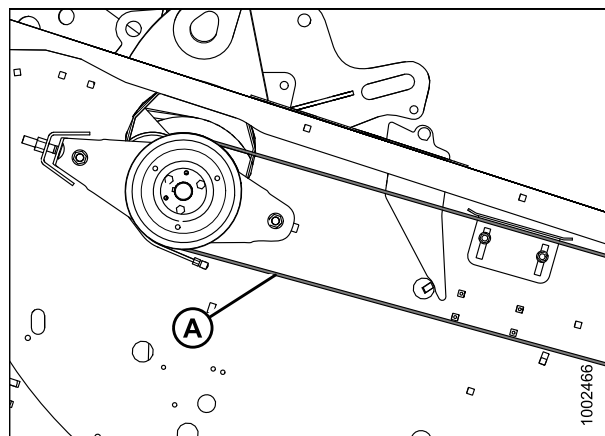
Рисунок 5.153: Привод ножа – правая сторона
