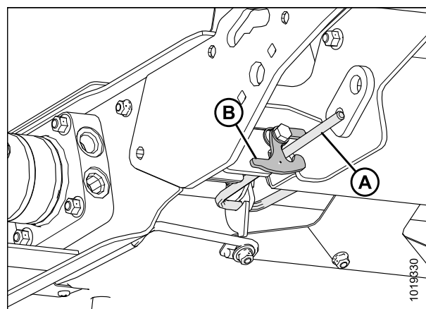
Рисунок 5.168: Ручка поддона направляющей подачи и защелка ручки поддона левой стороны
