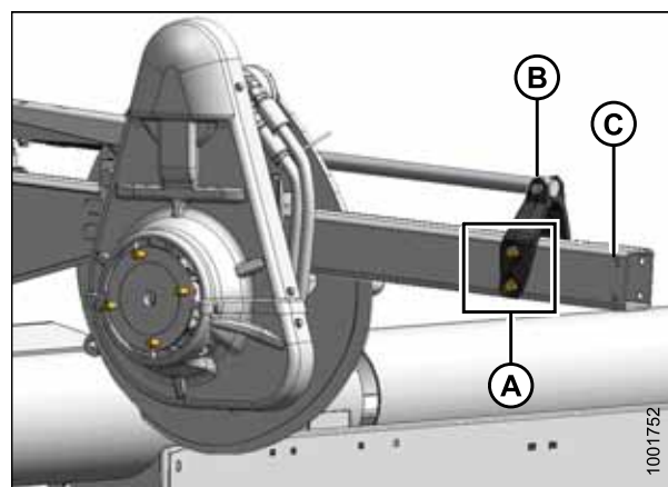
Рисунок 3.108: Правый рычаг — заднее положение
