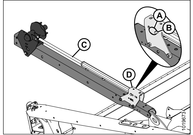
Рисунок 3.125: Цилиндр левого рычага мотвила в переднем положении
