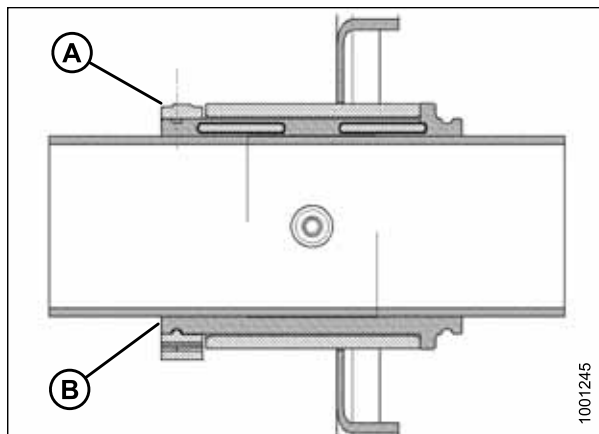
Рисунок 5.289: Втулка
