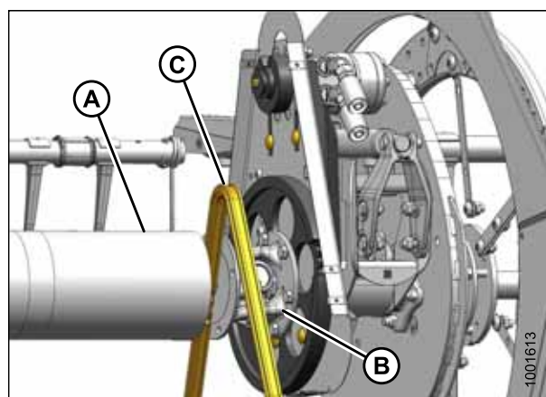
Рисунок 5.326: Замена цепи
