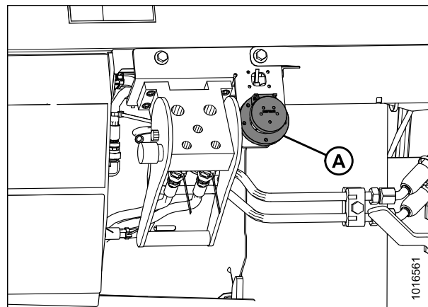
Рисунок 4.90: Ответные части модуля флотации
