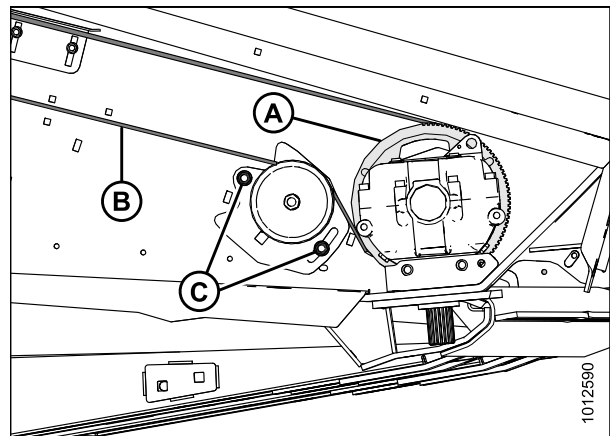
Рисунок 5.156: Привод ножа – правая сторона
