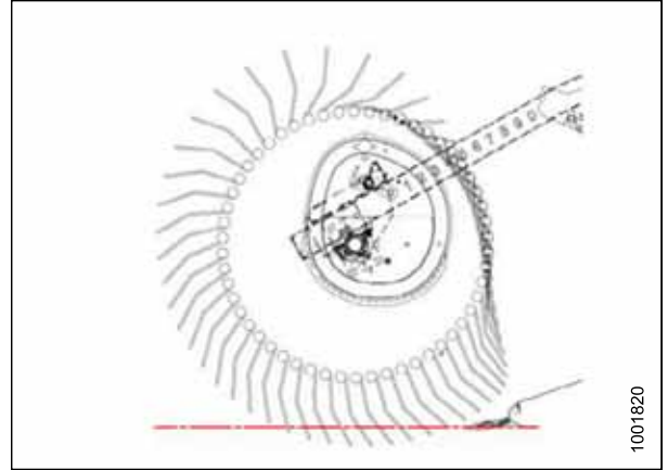
Рисунок 3.129: Вертикальное сечение пальца — положение 2
