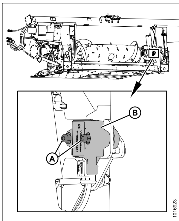
Рисунок 3.168: Дополнительный комплект с двумя датчиками — правый датчик
