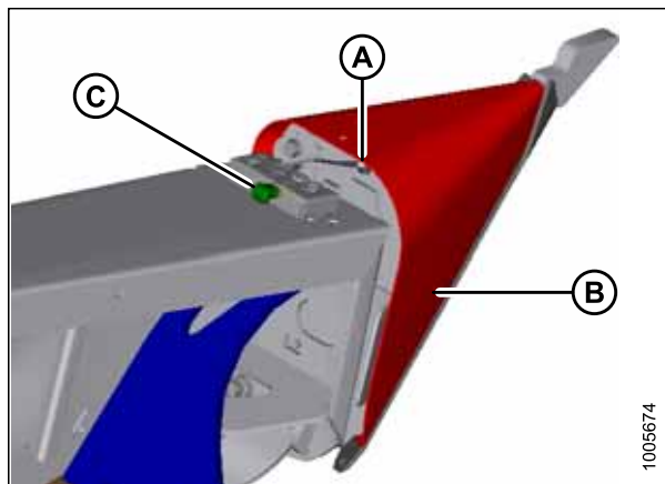
Рисунок 3.134: Делитель
