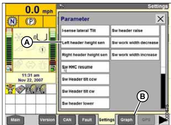
Рисунок 3.187: Приборная панель комбайна Case IH
