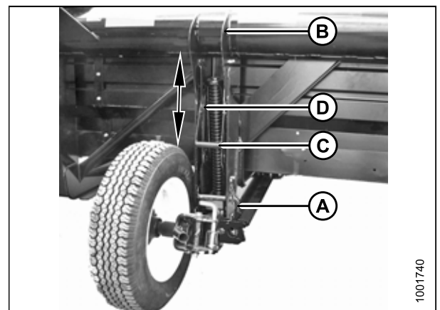
Рисунок 3.418: Заднее колесо — левая сторона
