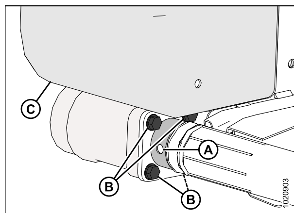
Рисунок 5.232: Приводной ролик
