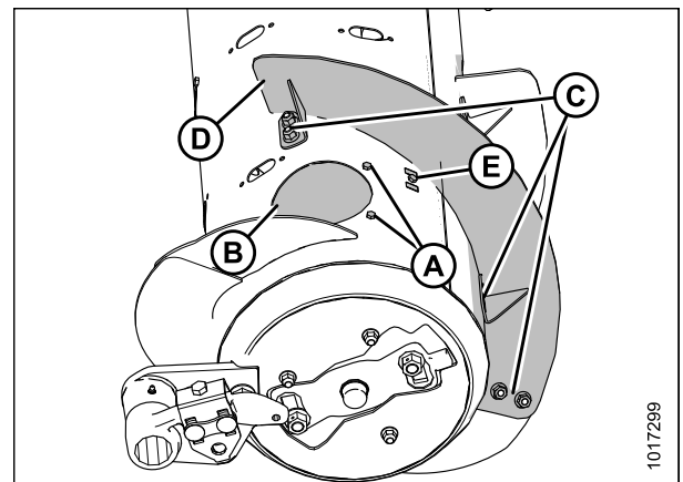
Рисунок 3.44: Узкая конфигурация (правая сторона)
