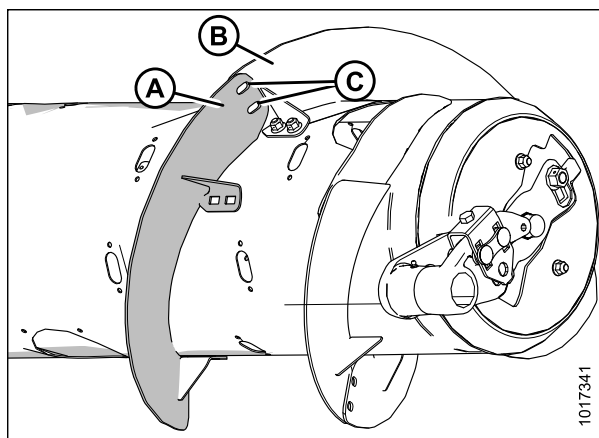
Рисунок 3.59: Правая сторона шнека
