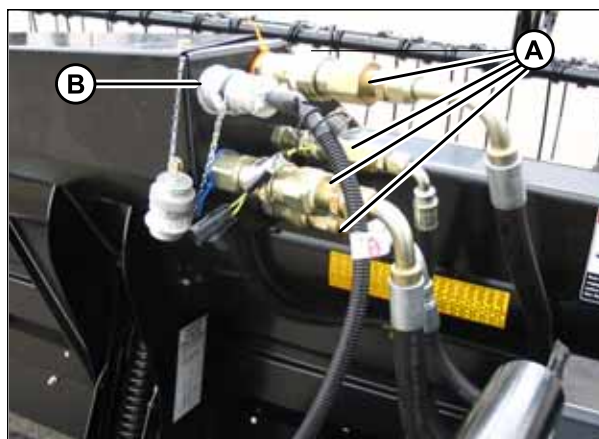
Рисунок 4.115: Соединения жатки
