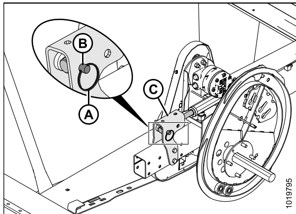
Рисунок 3.119: Центральный рычаг мотовила в переднем положении
