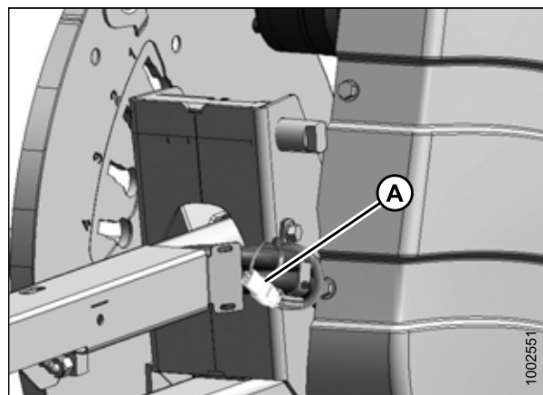
Рисунок 5.330: Жгут электропроводки
