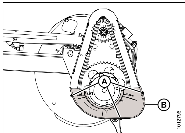
Рисунок 5.21: Нижняя крышка привода — сдвоенное мотовило
