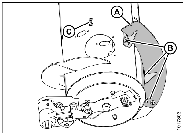
Рисунок 3.45: Широкая конфигурация (правая сторона)
