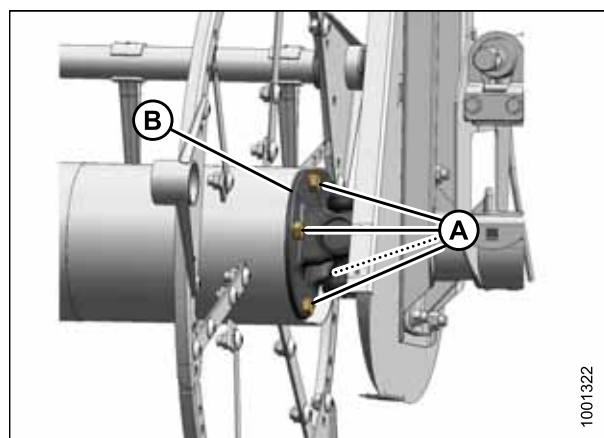
Рисунок 5.325: Крестовина
