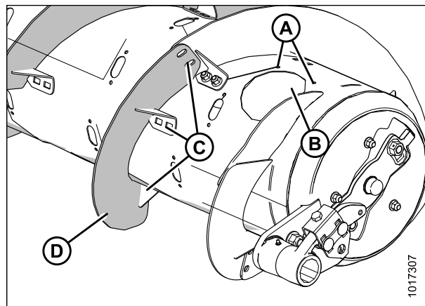
Рисунок 3.39: Ультразвуковая конфигурация (правая сторона)
