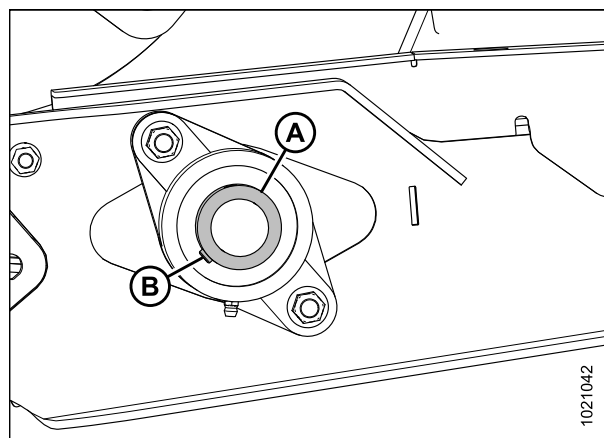
Рисунок 5.184: Подшипник приводного ролика подающего полотна
