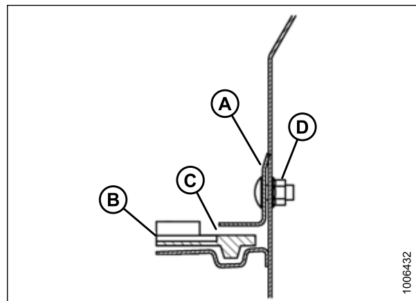
Рисунок 5.222: Дефлектор заднего щитка
