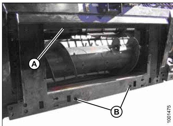
Рисунок 4.21: Модуль флотации
