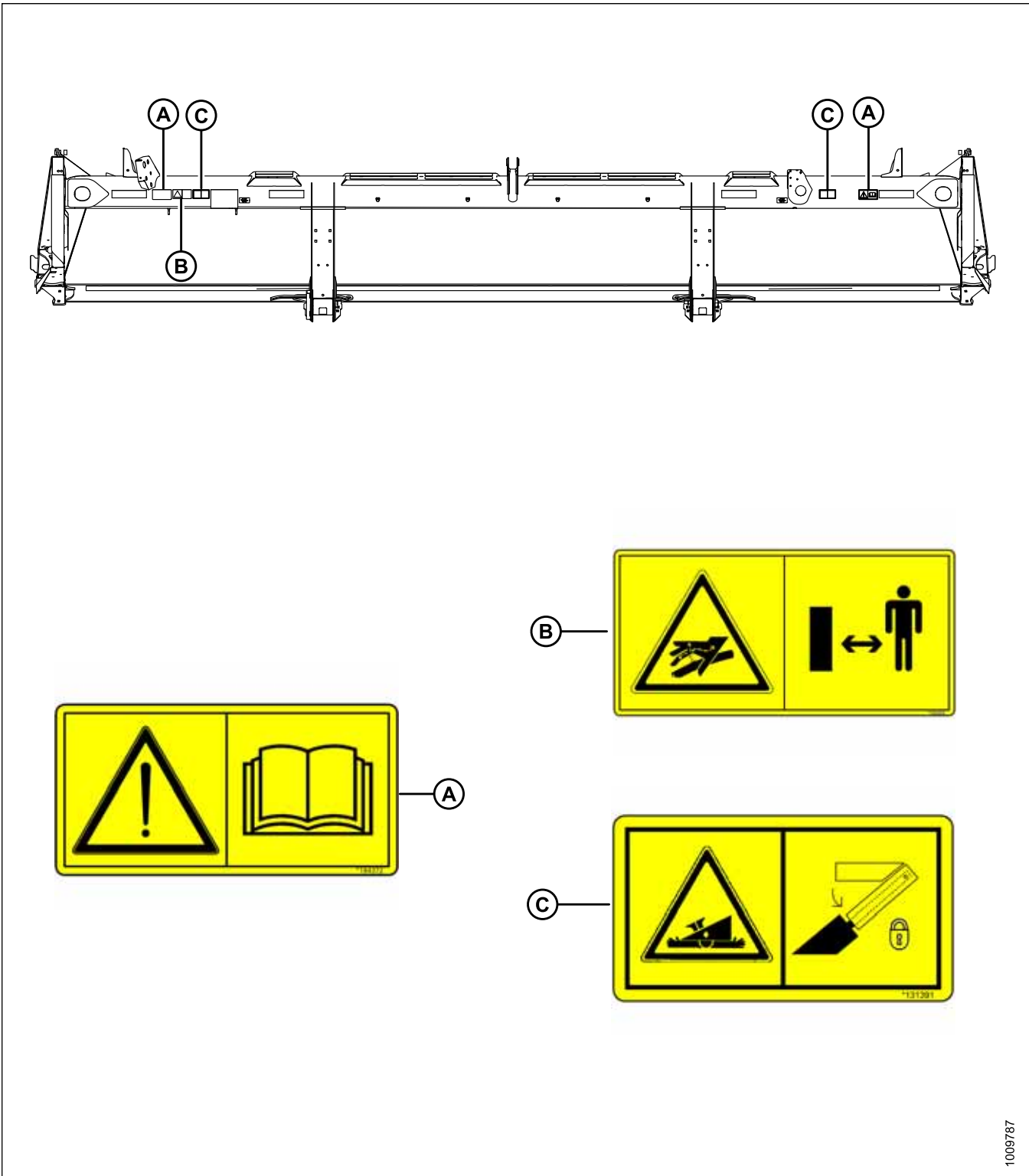
Рисунок 1.21: Задняя труба: 20-футовая жатка
