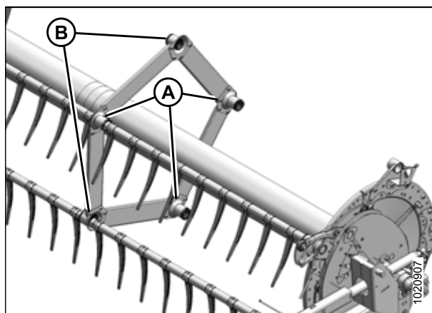
Рисунок 5.266: Держатели трубы пальцев граблины
