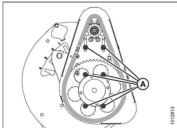
Рисунок 5.307: Изображен привод единого мотовила — привод сдвоенного мотовила имеет такую же конструкцию
