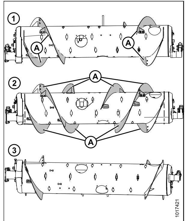
Рисунок 3.43: Конфигурации шнека (вид сзади)
