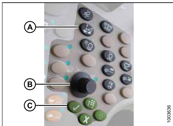
Рисунок 3.289: Консоль управления комбайна John Deere
