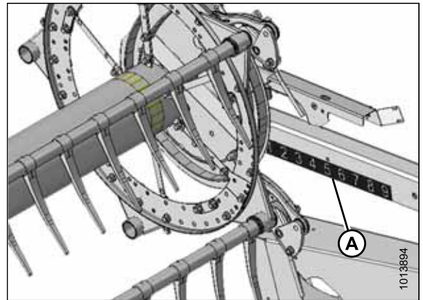
Рисунок 3.102: Шкала продольного смещения
