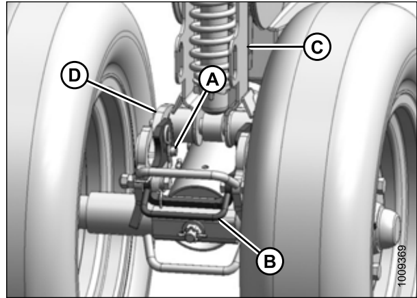
Рисунок 3.423: Левые передние колеса
