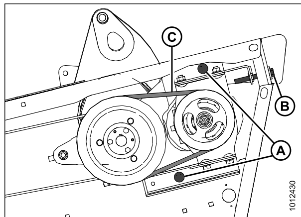
Рисунок 5.138: Клиновые ремни привода ножа
