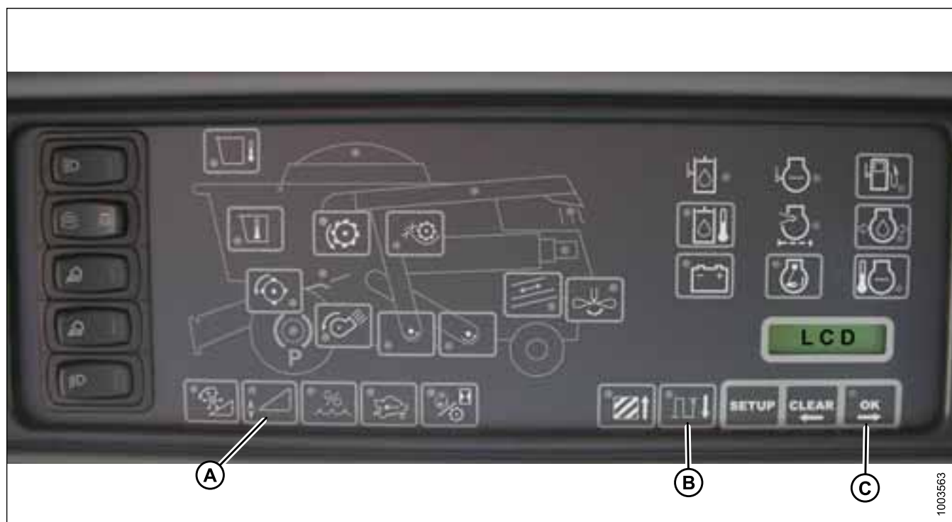
Рисунок 3.220: Верхняя панель приборов комбайна
