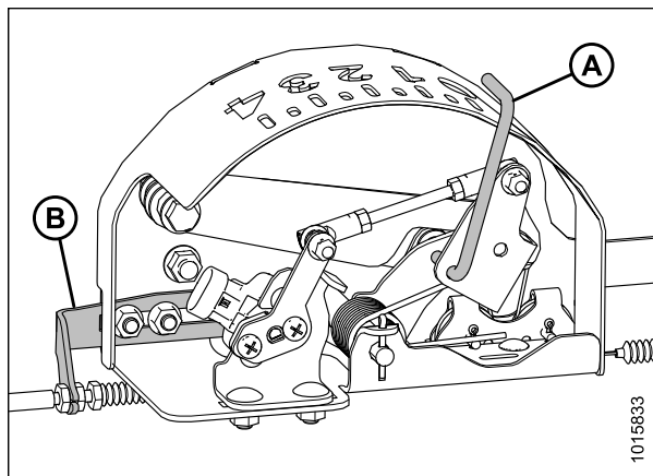
Рисунок 3.292: Блок индикатора флотации
