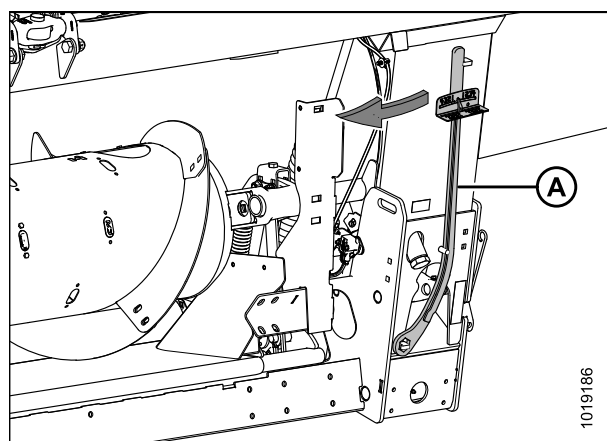
Рисунок 3.81: Место хранения динамометрического ключа
