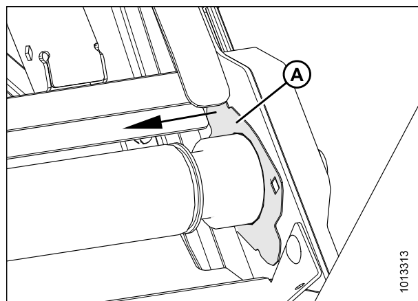
Рисунок 5.173: Приводной ролик
