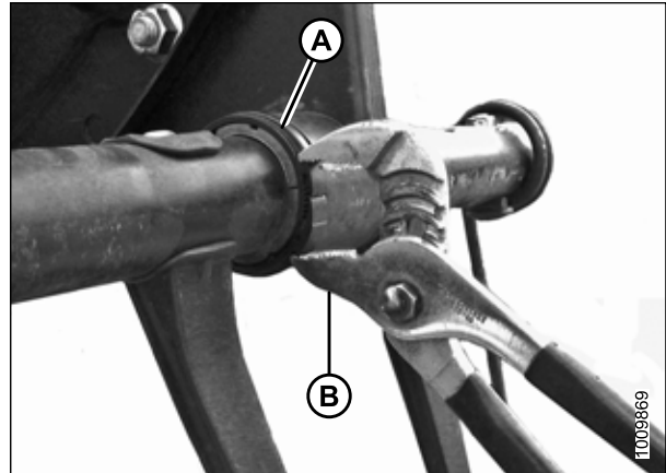
Рисунок 5.278: Установка хомута
