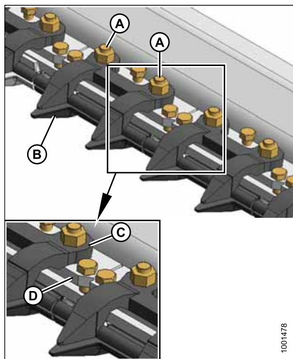
Рисунок 5.105: Сдвоенные противорезущие пальцы
