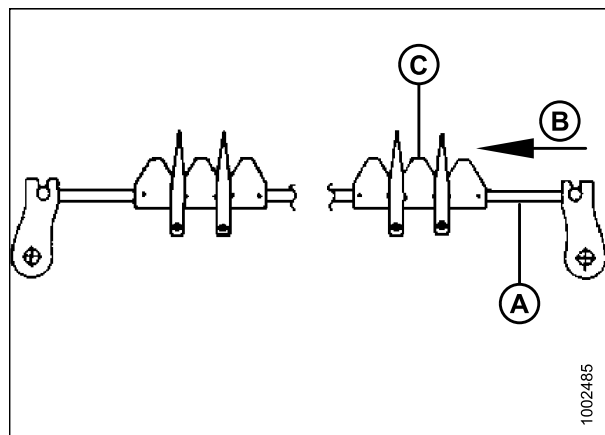
Рисунок 5.152: Регулировка синхронизации – правая сторона
