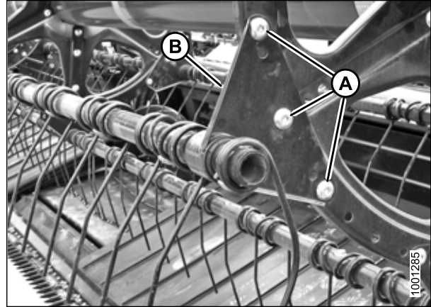
Рисунок 5.255: Рычаг подбирающего мотвила
