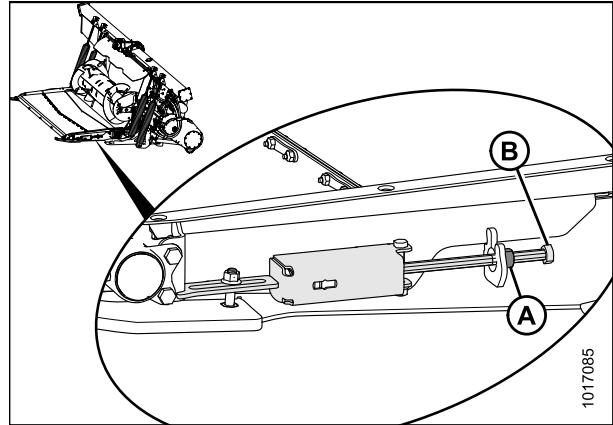
Рисунок 5.185: Натяжитель подающего полотна
