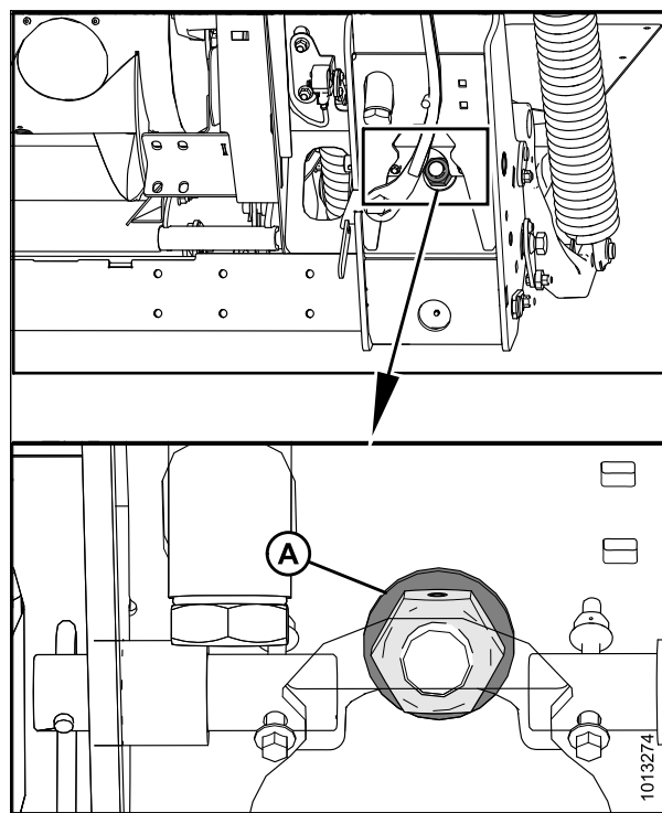
Рисунок 3.201: Блокировка флотации
