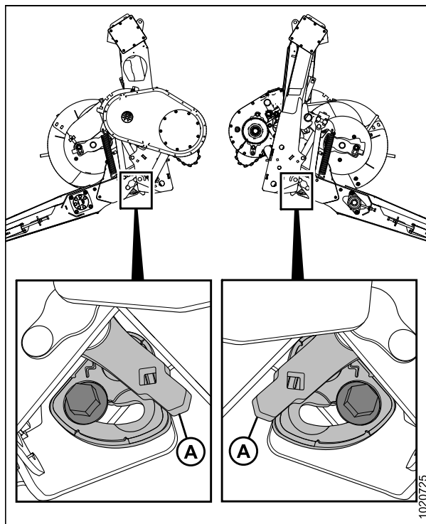
Рисунок 3.148: Рычаги регулирования флотации шнека
