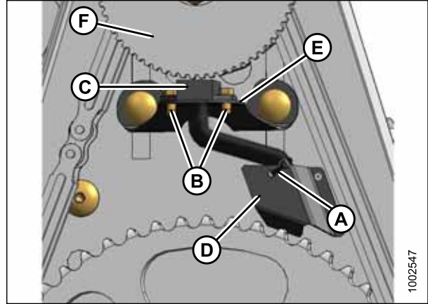
Рисунок 5.331: Датчик скорости
