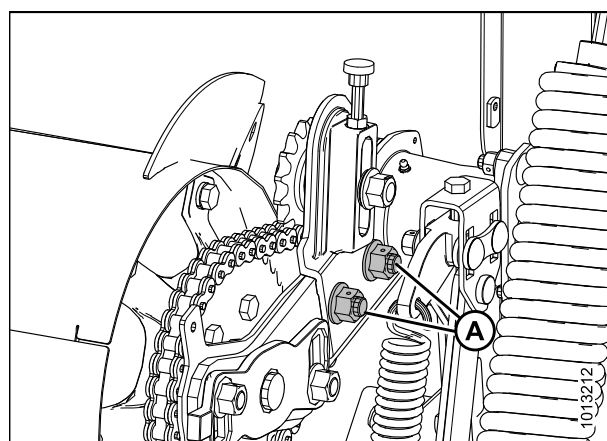
Рисунок 5.58: Опорный рычаг шнека
