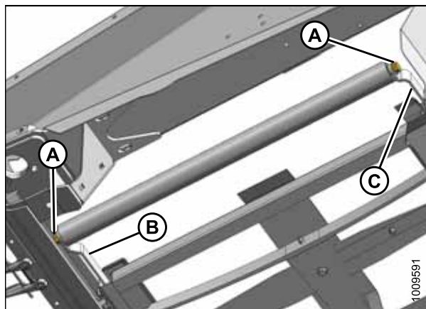
Рисунок 5.229: Натяжной ролик
