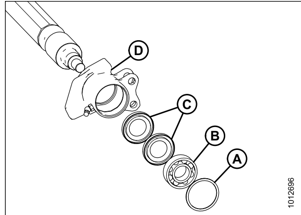
Рисунок 5.190: Подшипник в сборе
