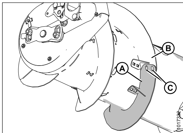
Рисунок 3.62: Левая сторона шнека
