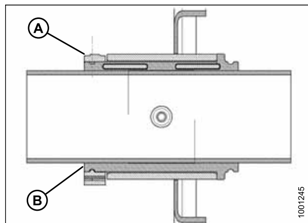
Рисунок 5.277: Втулка
