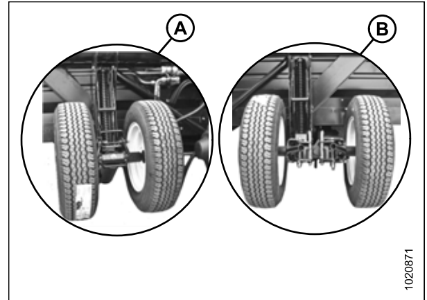
Рисунок 3.421: Рабочее положение
