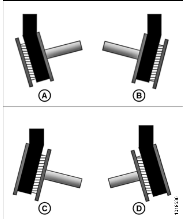
Рисунок 5.157: Шкив привода ножа
