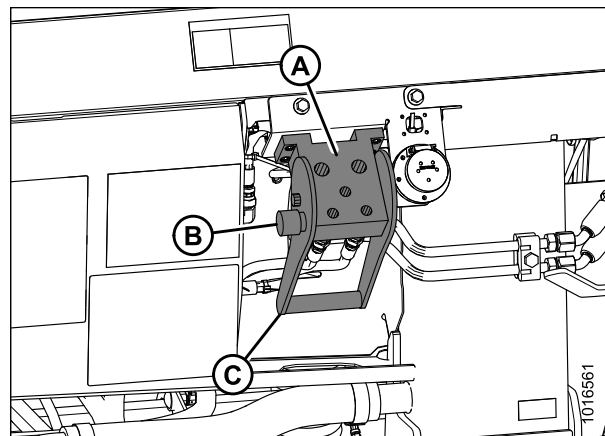
Рисунок 4.4: Гнездо модуля флотации
