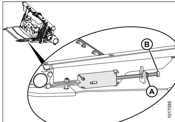
Рисунок 5.170: Натяжитель подающего полотна
