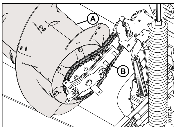
Рисунок 5.61: Привод шнека
