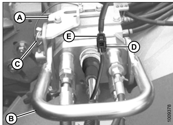
Рисунок 4.43: Многоканальная муфта
