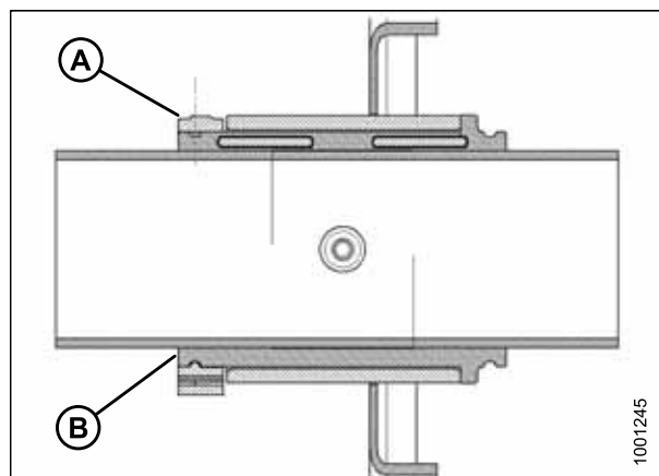
Рисунок 5.283: Втулка
