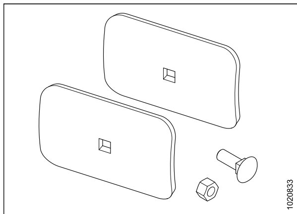
Рисунок 6.20: Комплект для ремонта вмятин на шнеке
