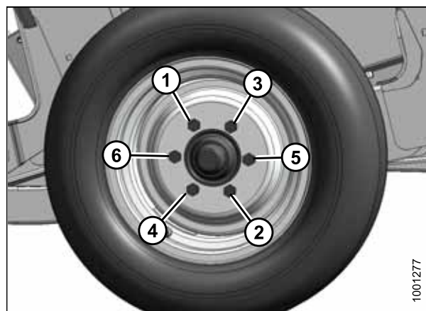
Рисунок 5.336: Последовательность затяжки болтов
