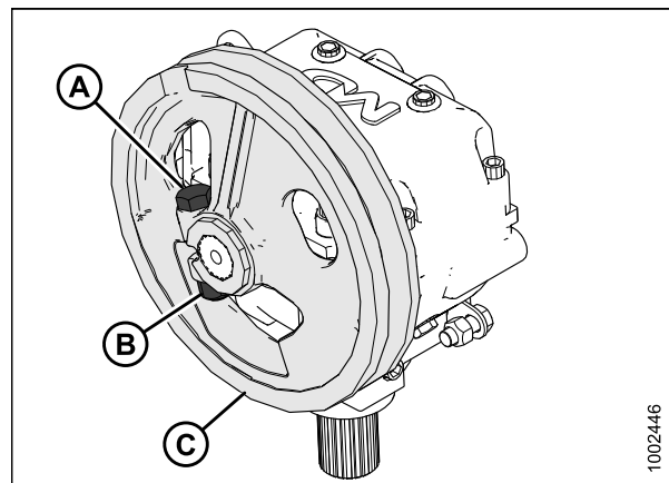
Рисунок 5.121: Редуктор привода ножа (МКШ) и шкив
