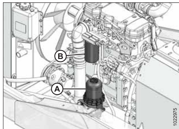
图 5.65: 燃油系统过滤器
