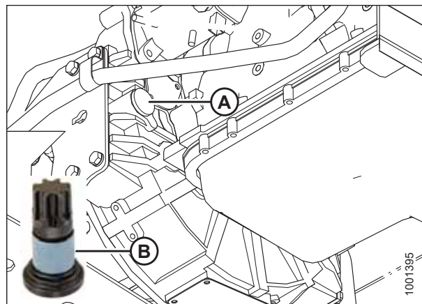
图 5.41: 用于盘动工具的检修孔位置
