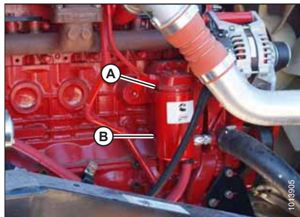
图 5.47: 发动机机油过滤器
