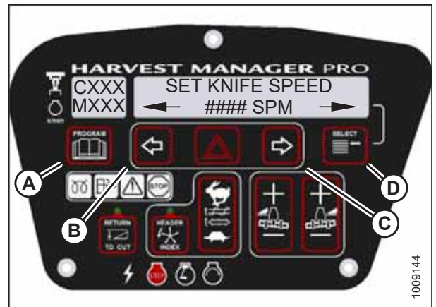
图 3.79: 割刀速度设置
