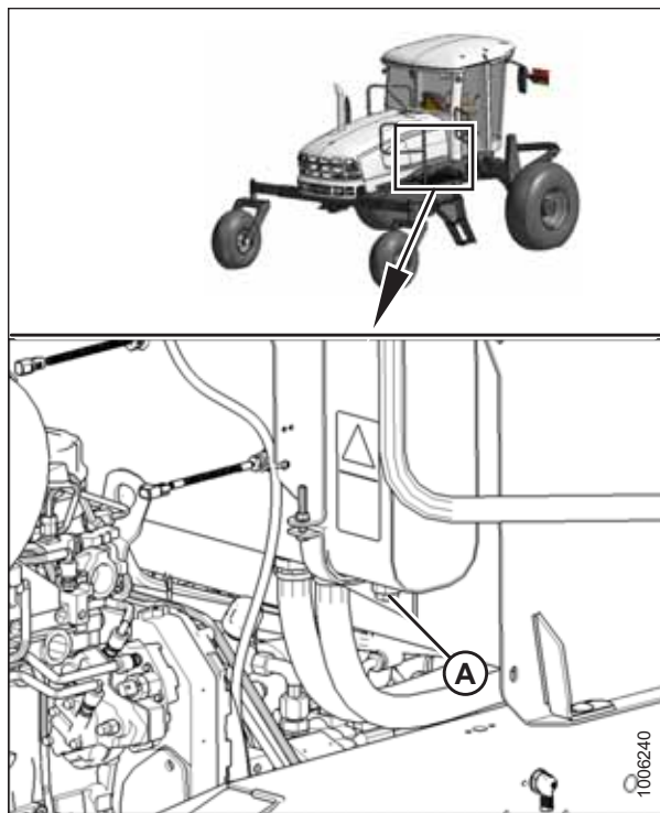
图 5.180: 液压油放油塞
