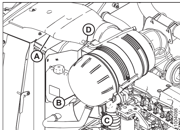
图 5.49: 发动机进气系统 (北美地区)
