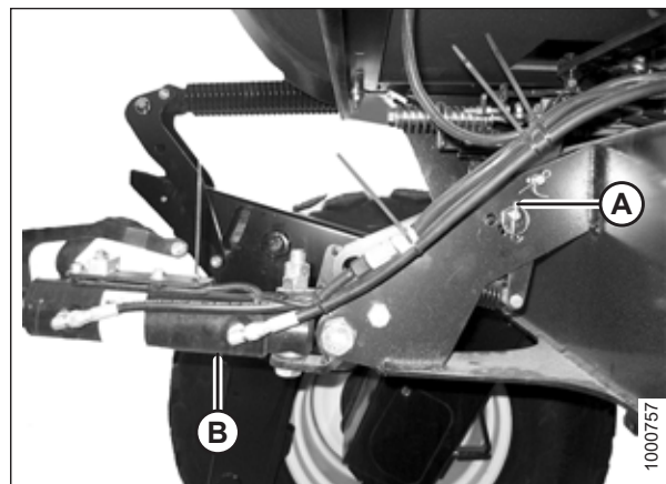
图 4.180: 不带自对准套件的液压中央升降
