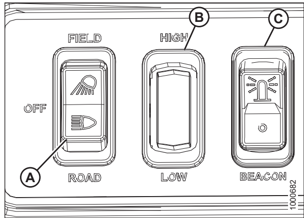
图 4.33: 灯开关
