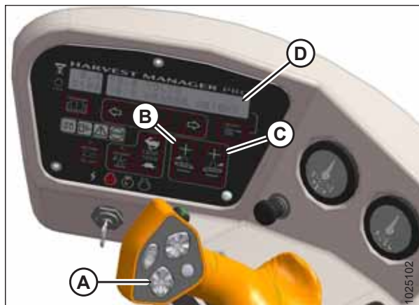
图 4.296: 操作员控制台
