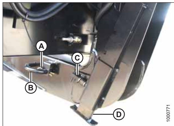
图 4.125: 割台支腿
