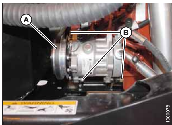
图 5.116: 空调压缩机
