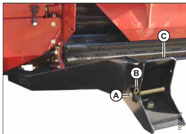
图 4.281: 割台连接座
