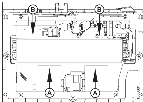
图 5.36: HVAC 系统
