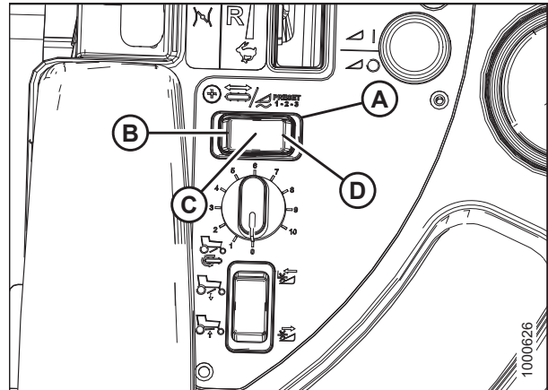
图 3.56: 割台开关
