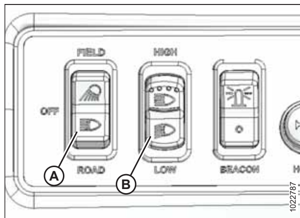
图 5.137: 道路灯开关 (俄罗斯除外)
