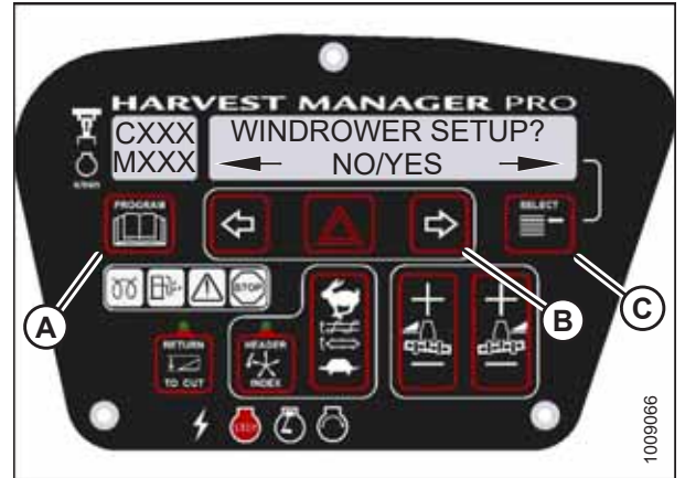
图 3.90: CDM 编程按钮
