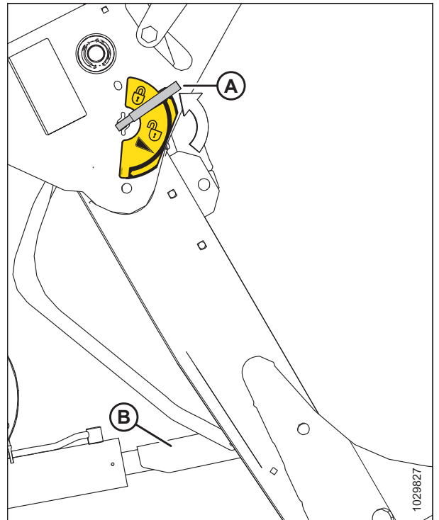
图 4.206: 安全撑杆
