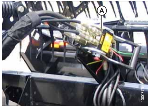
图 4.204: 拨禾轮液压系统
