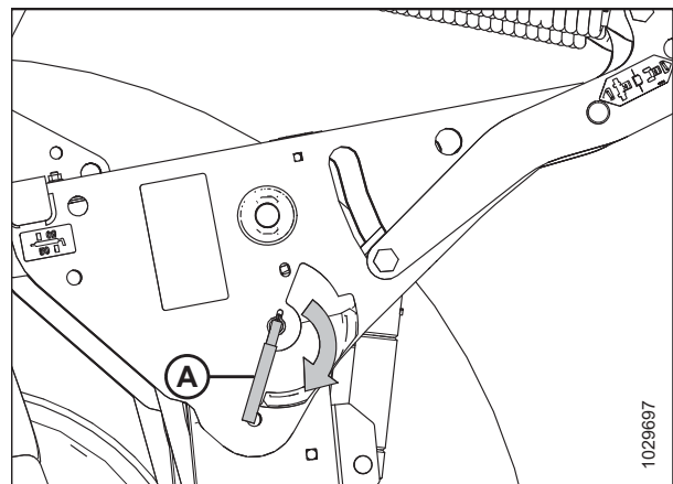
图 4.235: 安全撑杆控制杆
