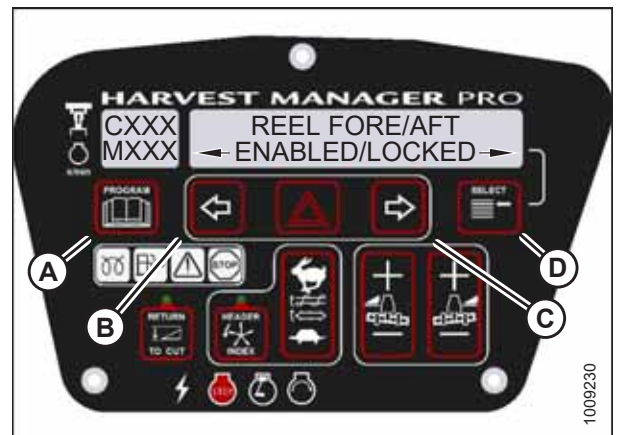
图 3.120: M155 拨禾轮前后移动控制装置锁定
