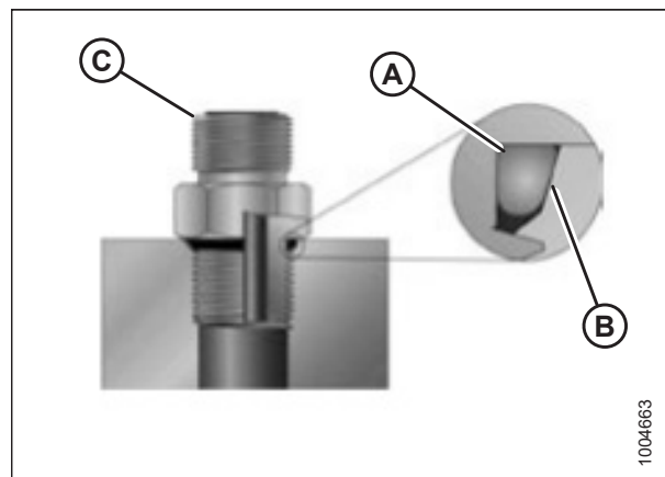
图 8.13: 液压接头
