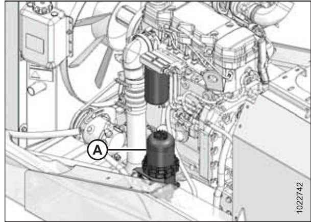
图 5.68: 初级燃油过滤器位置
