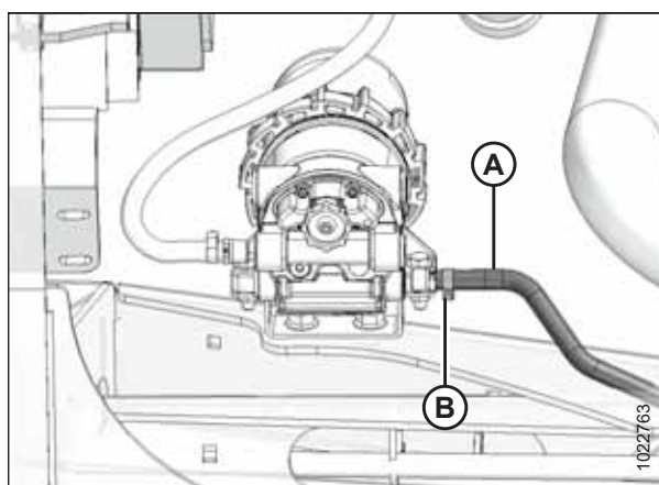
图 5.82: 燃油系统
