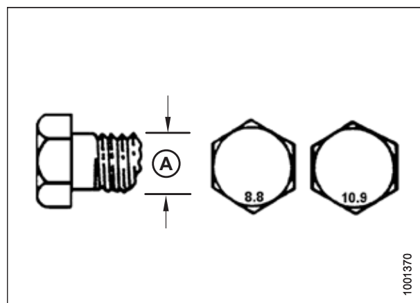
图 8.9: 螺栓等级
