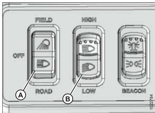
图 5.138: 道路灯开关 (仅限俄罗斯)
