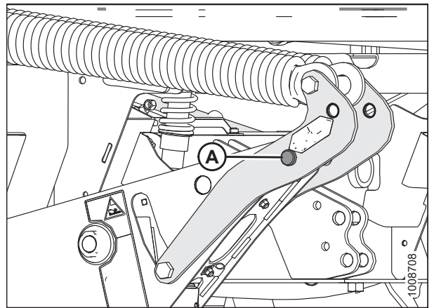
图 4.79: 浮动悬挂销 - 已接合
