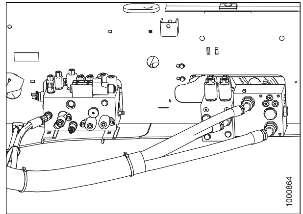
图 5.190: 液压阀组
