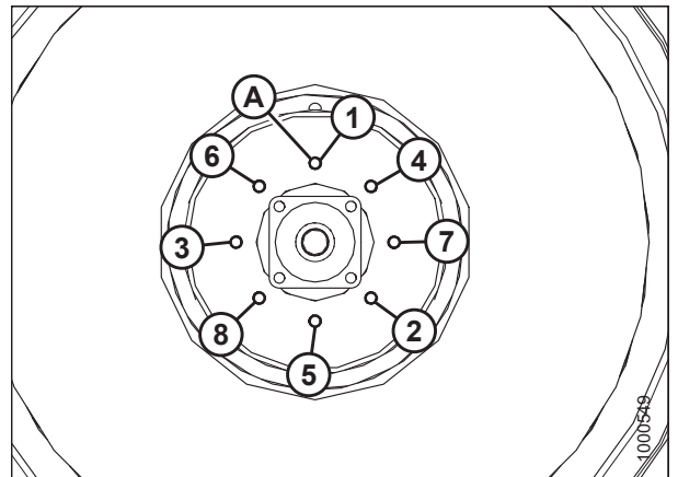
图 5.208: 叉式支撑从动轮螺母拧紧顺序
