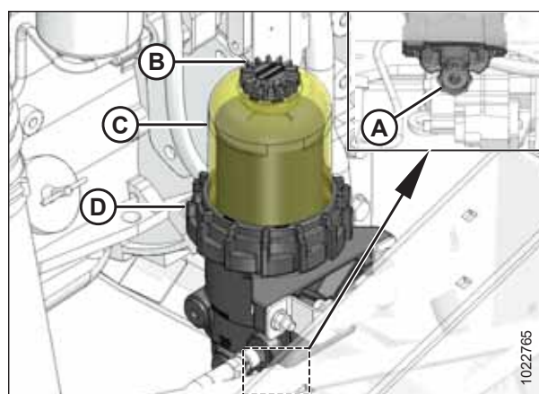
图 5.84: 初级燃油过滤器
