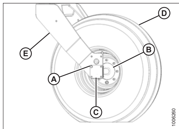
图 5.216: 叉式支撑从动轮
