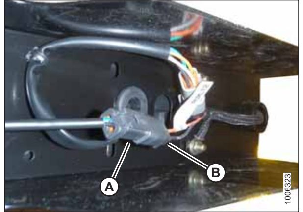
图 5.154: HID 辅助灯线束
