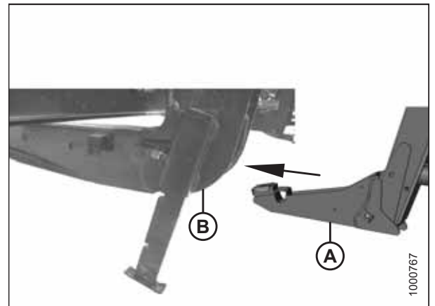
图 4.106: 割台支腿和连接座
