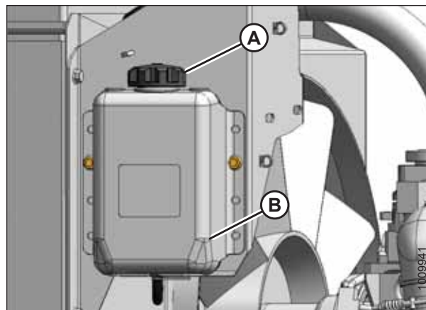
图 5.94: 冷却液回收箱
