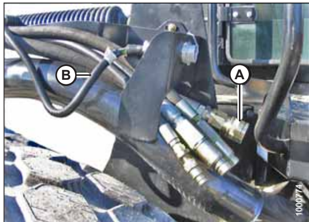
图 4.115: 割台驱动软管和线束
