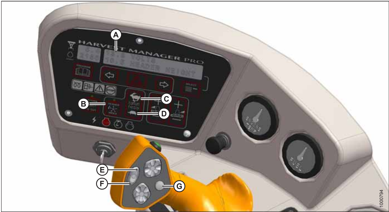
图 4.300: 操作员控制台
