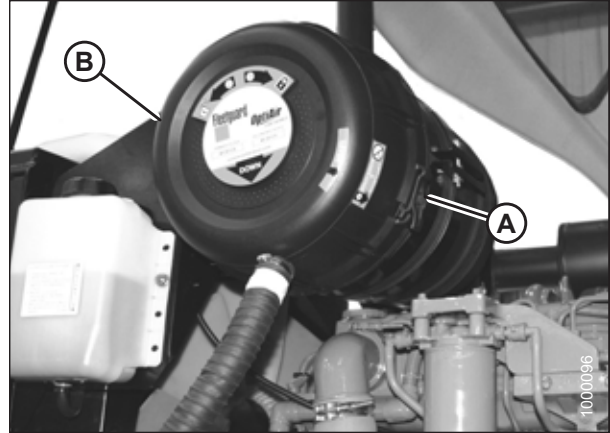
图 5.59: 发动机空气滤清器
