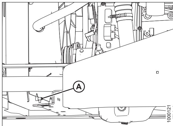
图 5.89: 散热器放水阀
