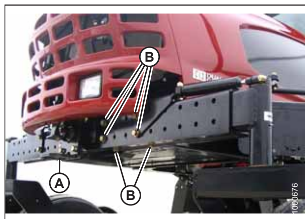
图 4.28: 从动轮伸长梁
