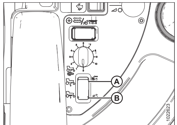
图 3.155: 放铺导板控制装置
