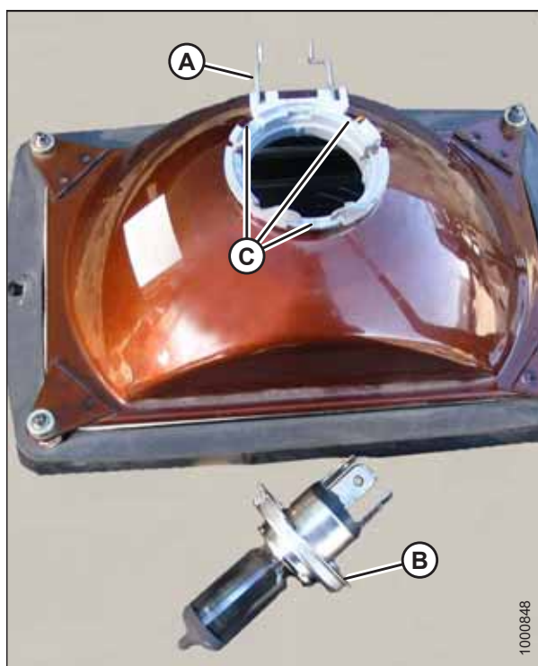
图 5.134: 前大灯组件
