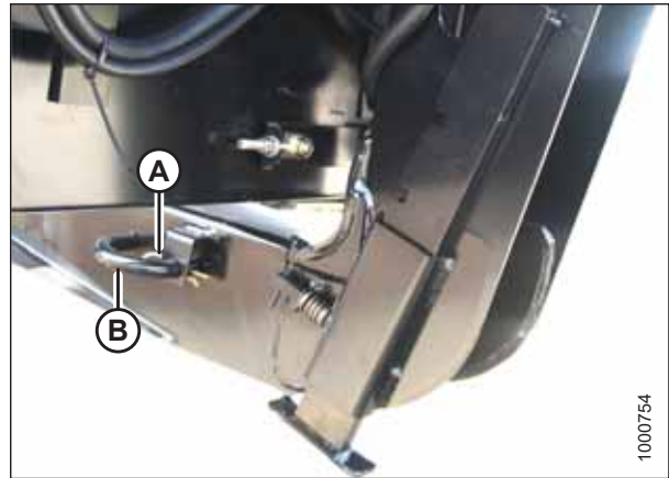
图 4.103: 割台支腿
