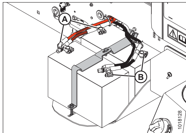
图 5.130: 蓄电池
