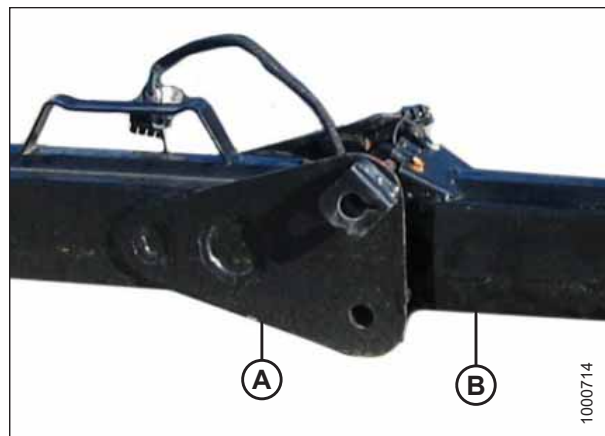
图 4.55: 运输钩
