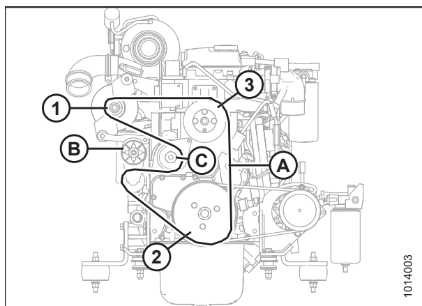
图 5.113: 发动机皮带
