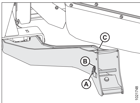
图 4.224: 割台支座
