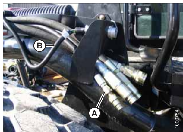
图 4.222: 割台驱动装置液压系统
