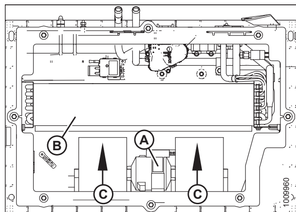
图 5.37: HVAC 系统
