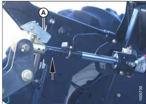
图 4.88: 中央升降
