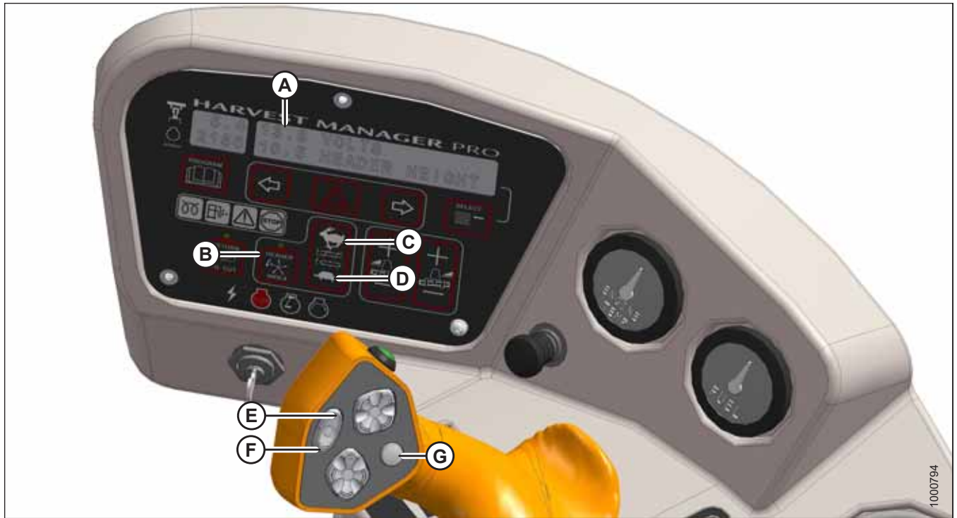
图 4.299: 操作员控制台
