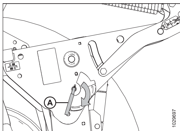
图 4.202: 安全撑杆控制杆
