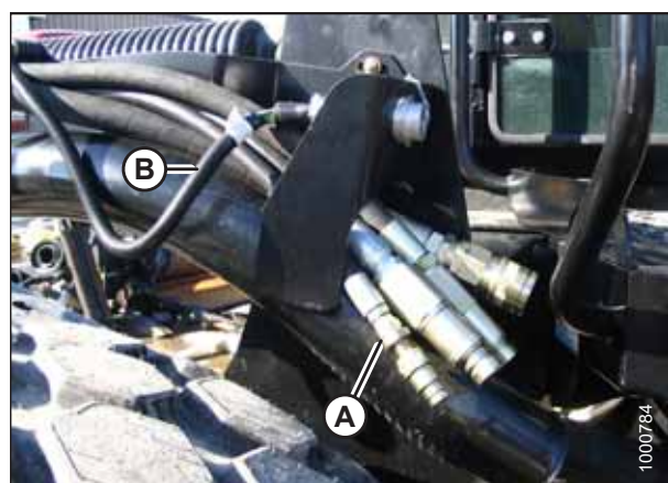
图 4.280: 割台驱动装置液压系统
