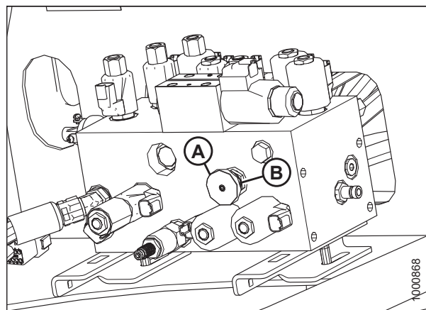
图 5.191: 多功能操纵阀箱
