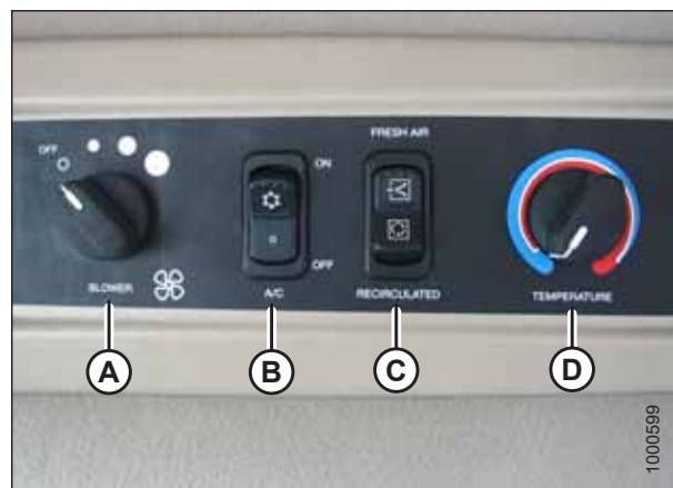
图 4.6: 温度控制装置
