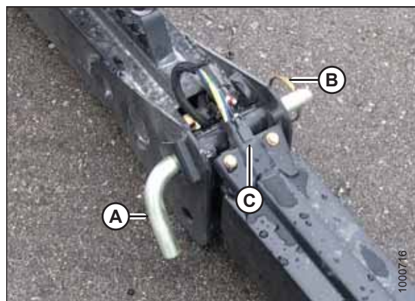
图 4.56: 运输钩
