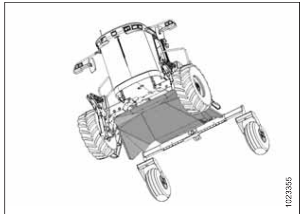
图 4.96: 放铺导板
