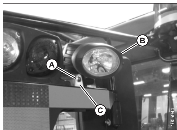
图 5.150: HID 辅助灯
