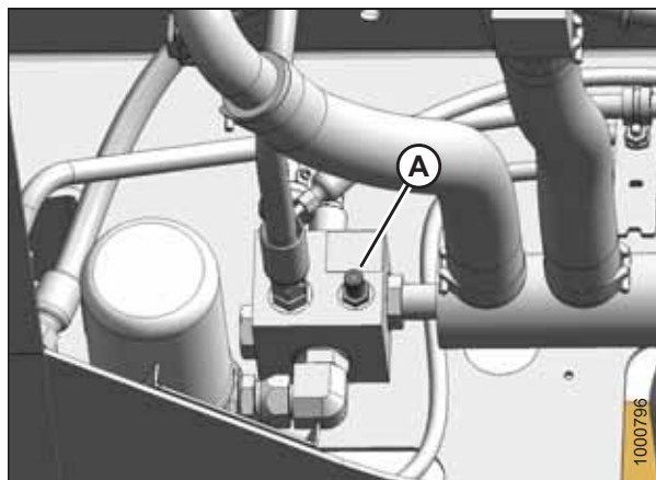
图 5.194: 充油泵测试口
