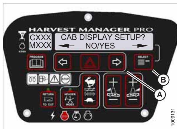
图 3.70: 驾驶室显示屏设置
