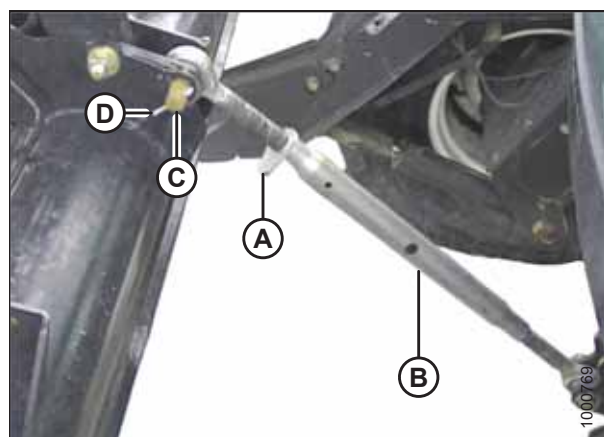
图 4.45: 机械升降
