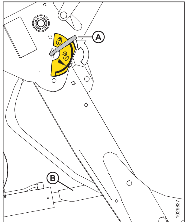
图 4.265: 安全撑杆
