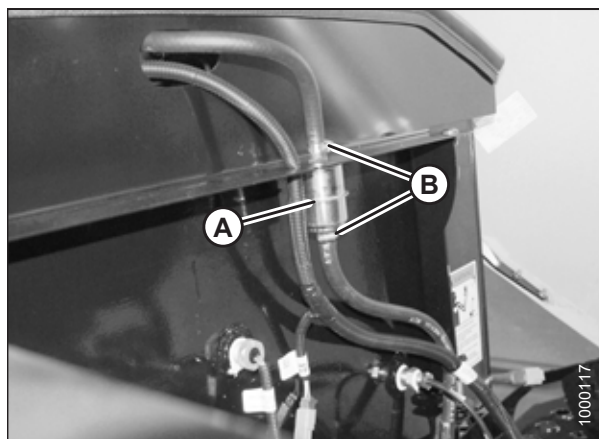
图 5.64: 油箱通气管
