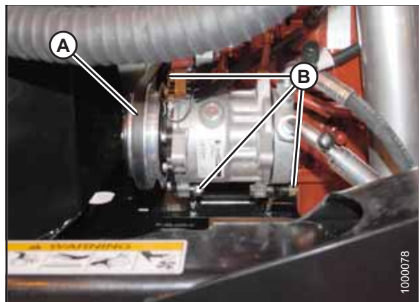
图 5.112: 空调压缩机
