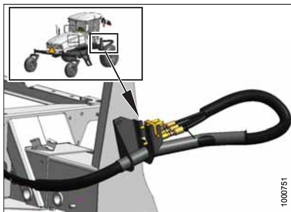
图 4.284: 带式输送割台拨禾轮液压系统
