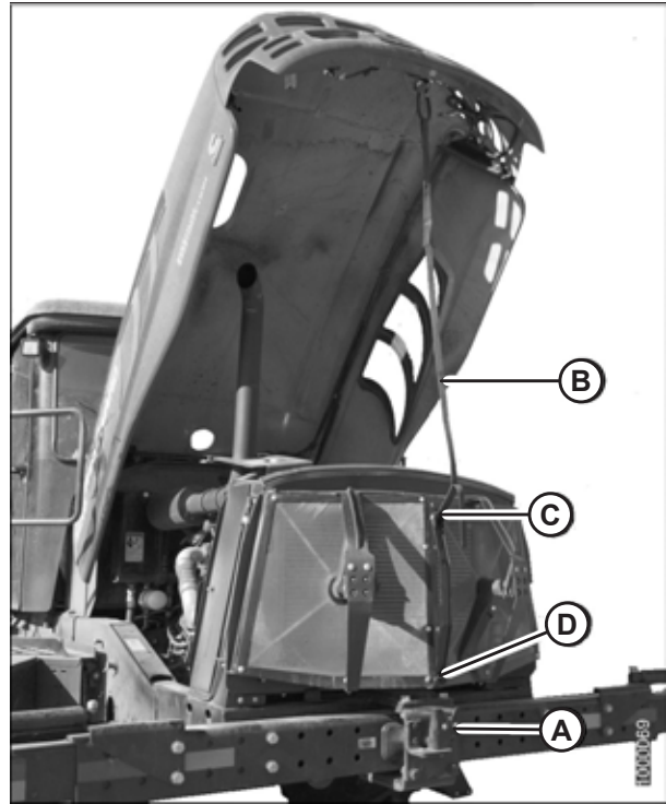
图 5.3: 机罩打开 (较高位置)
