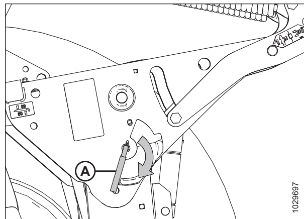
图 4.210: 安全撑杆
