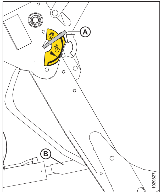
图 4.154: 安全撑杆
