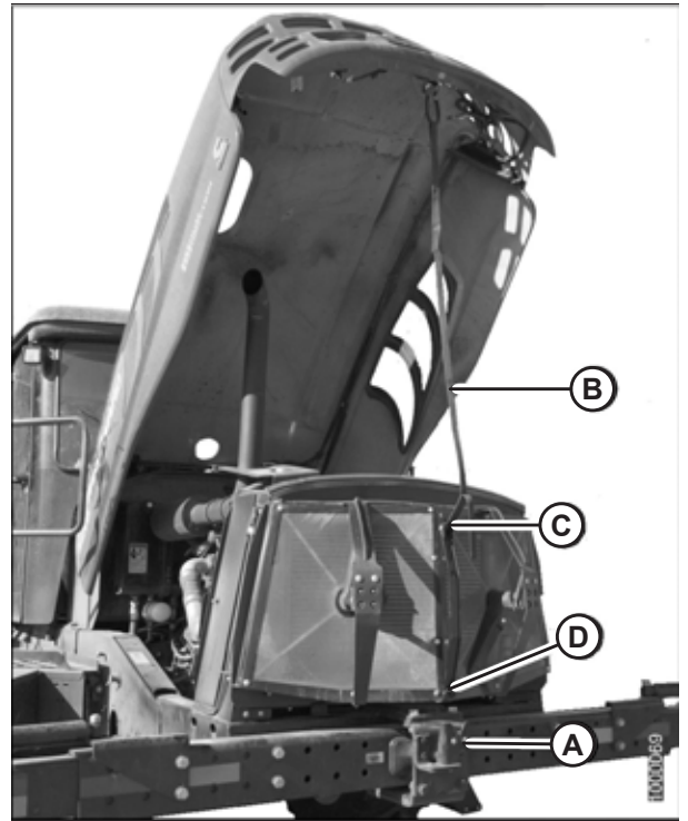
图 5.4: 机罩打开 ( 较高位置 )
