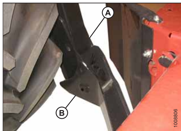
图 4.255: 割台支座
