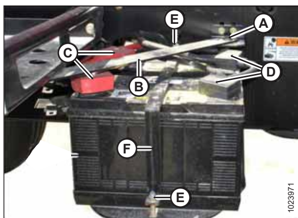
图 5.125: 蓄电池
