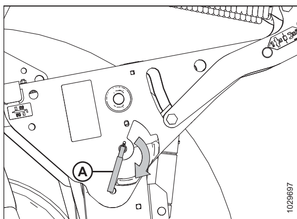
图 4.147: 安全撑杆
