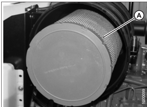
图 5.55: 发动机空气滤清器初级滤芯
