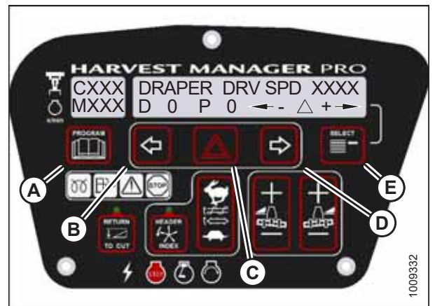
图 3.191: 输送带驱动装置
