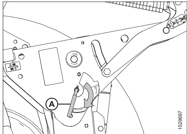
图 4.268: 安全撑杆
