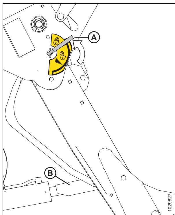
图 4.170: 安全撑杆
