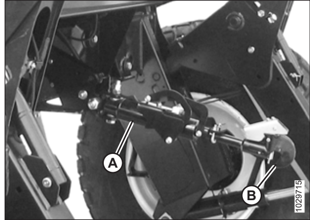
图 4.108: 液压中央升降
