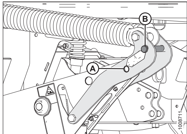
图 4.219: 割台浮动悬挂提升臂部件
