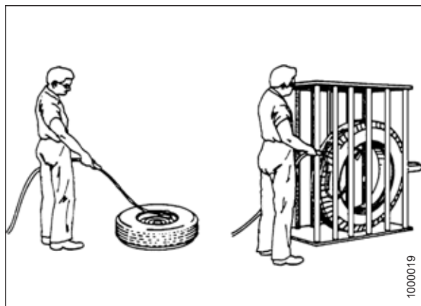
图 5.207: 安全地为轮胎充气
