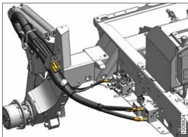
图 4.282: 带式输送割台液压系统
