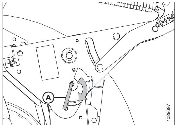
图 4.69: 安全撑杆
