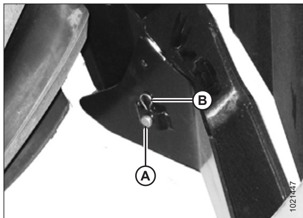
图 4.259: 割台支座
