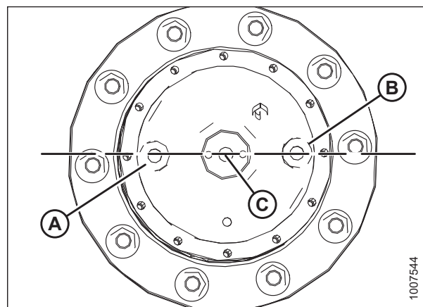
图 5.197: 驱动轮轮毂
