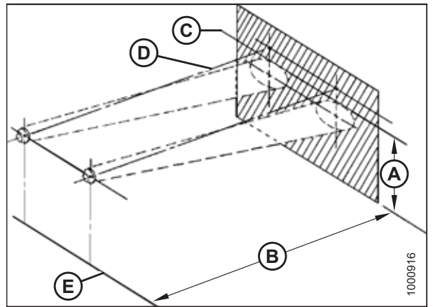
图 5.140: 前大灯光束定位
