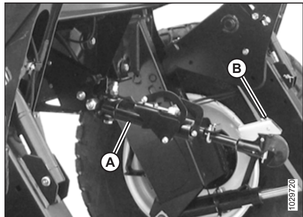
图 4.230: 液压中央升降
