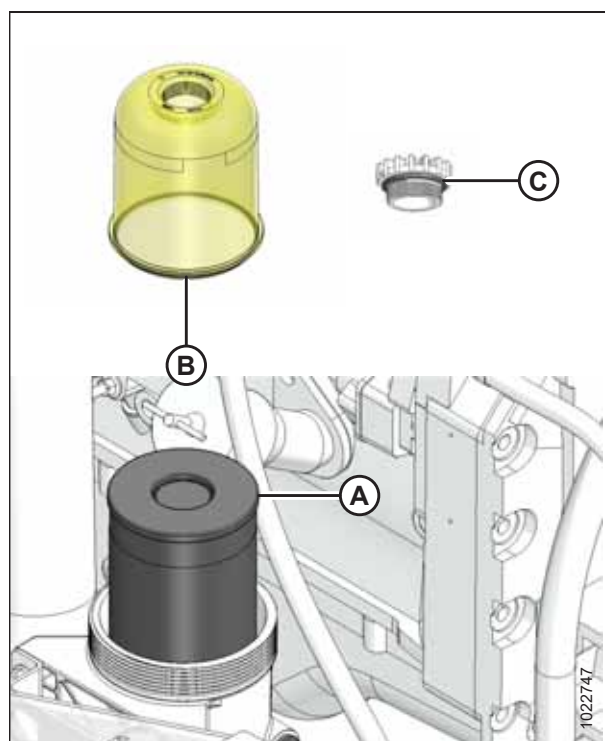
图 5.70: 初级燃油过滤器
