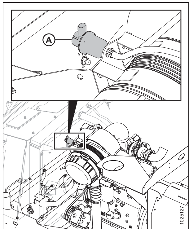
图 5.60: 发动机空气滤清器
