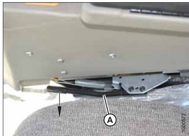
图 5.16: 座椅调整手柄
