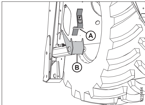
图 5.206: 驱动轮支腿支承点
