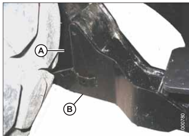
图 4.217: 割台连接座
