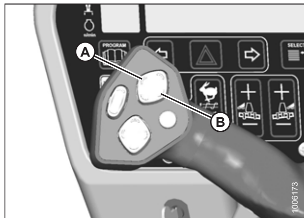
图 4.285: 地速控制杆
