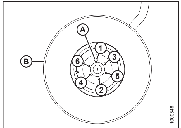
图 5.209: 成型臂支撑从动轮螺母拧紧顺序
