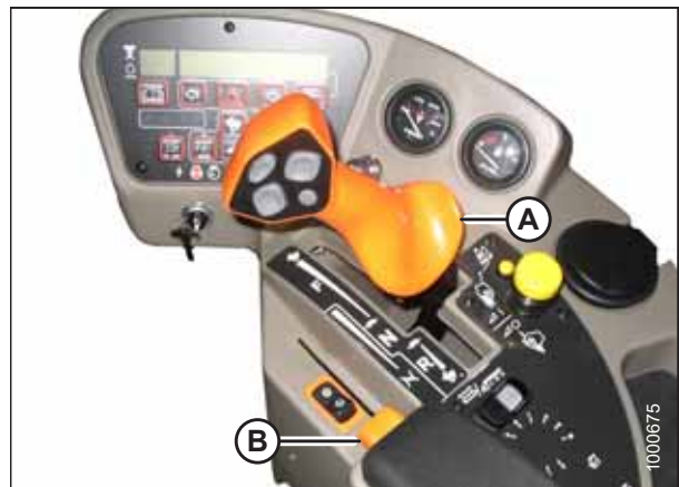
图 4.27: 操作员控制台
