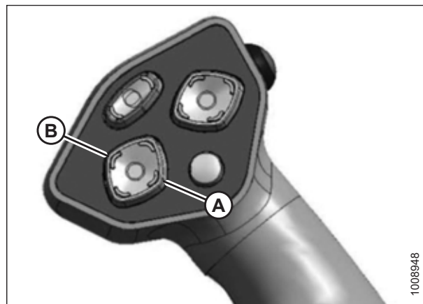
图 4.269: 地速控制杆
