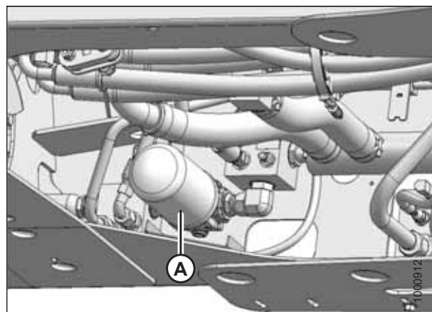
图 5.183: 充油过滤器
