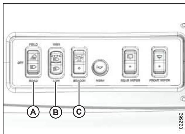
图 3.17: 顶篷控制台 ( 俄罗斯除外 )
