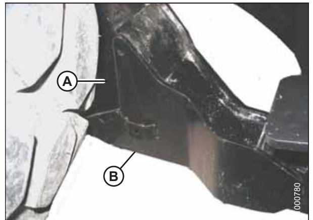
图 4.228: 割台支座
