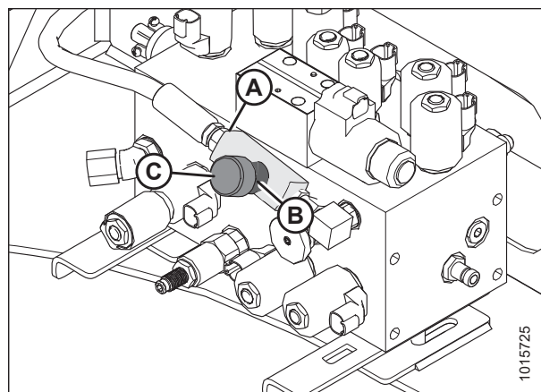
图 5.192: 多功能操纵阀箱
