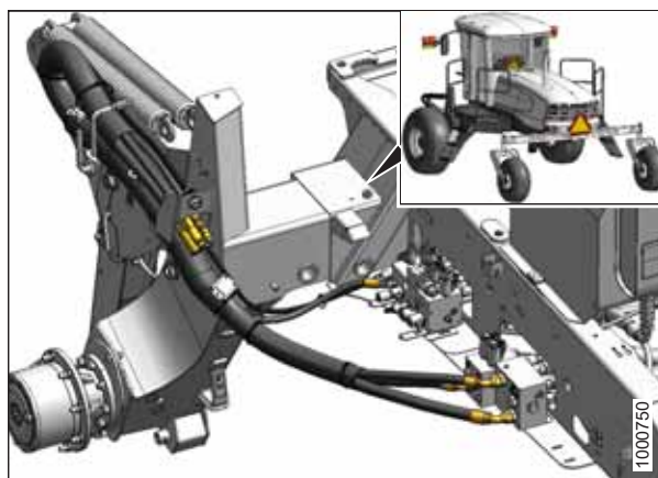
图 4.283: 带式输送割台驱动装置液压系统
