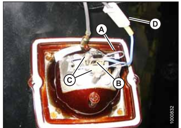
图 5.157: 后泛光灯组件
