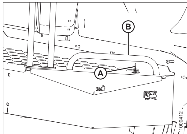
图 5.10: 平台闩锁
