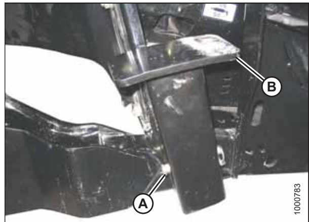
图 4.172: 割台支座
