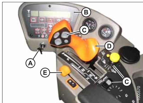
图 3.1: 操作员控制台
