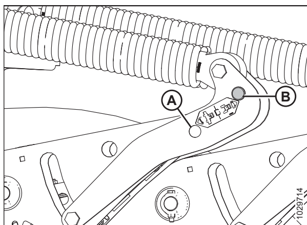
图 4.225: 浮动悬挂提升臂部件
