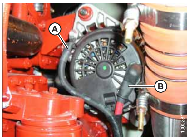
图 5.117: 交流发电机
