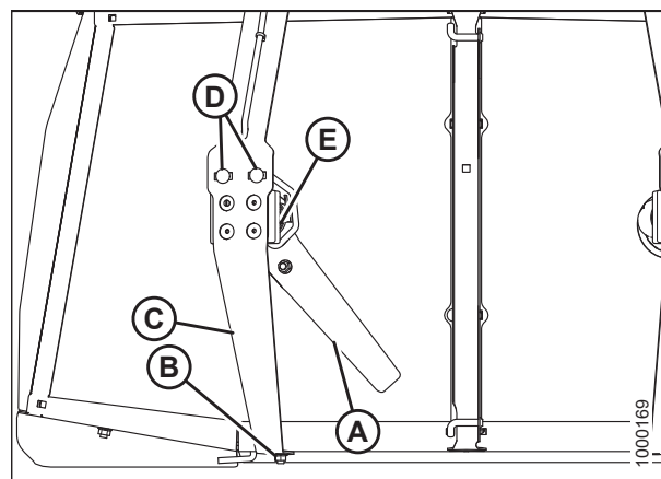
图 5.105: 驱尘器
