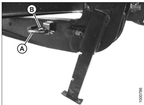
图 4.152: 割台支座
