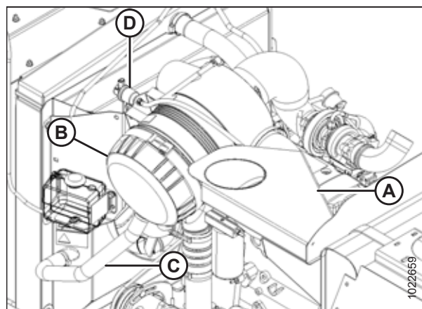
图 5.50: 发动机进气系统 (出口)
