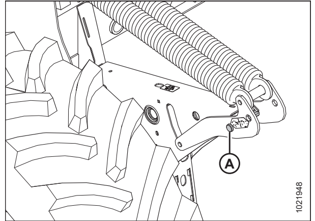
图 3.148: 浮动悬挂销 – 右侧
