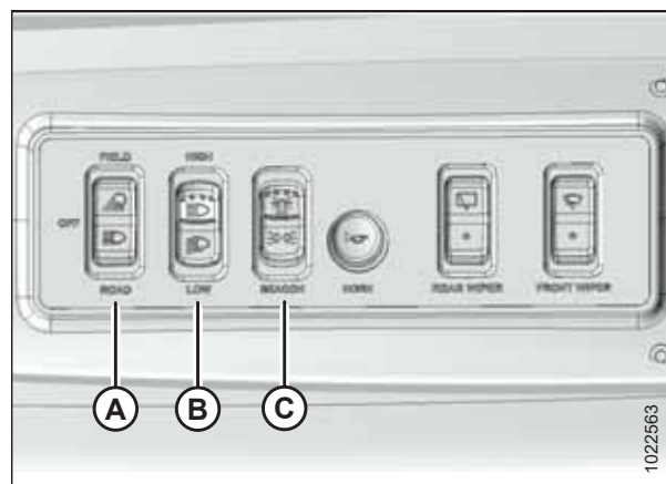
图 3.18: 顶篷控制台 ( 俄罗斯 )
