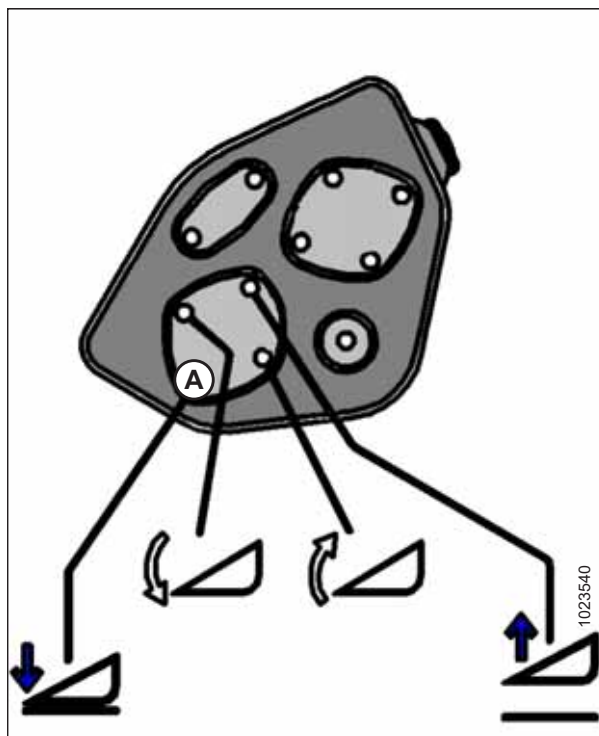
图 3.143: GSL 上的割台高度控制装置
