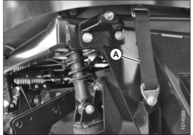
图 5.24: 驾驶室悬置系统
