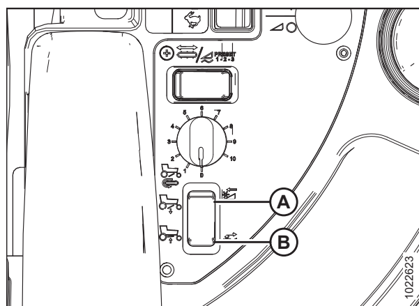
图 3.157: 放铺导板控制装置
