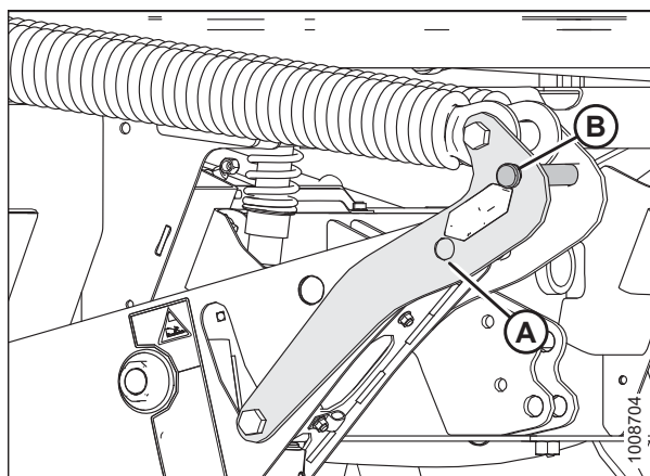
图 4.146: 割台浮动悬挂提升臂部件
