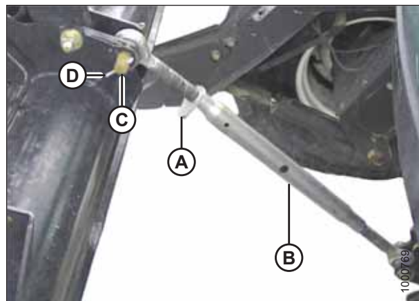
图 4.221: 机械中央升降
