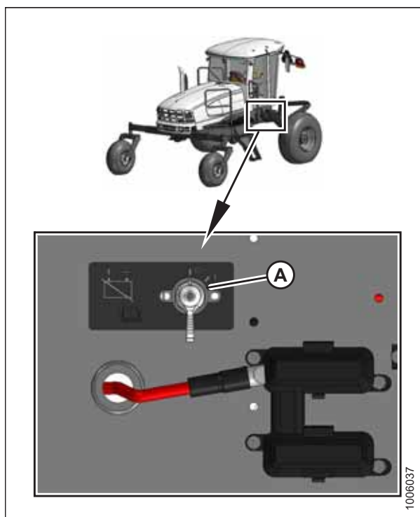
图 5.124: 蓄电池总断开开关
