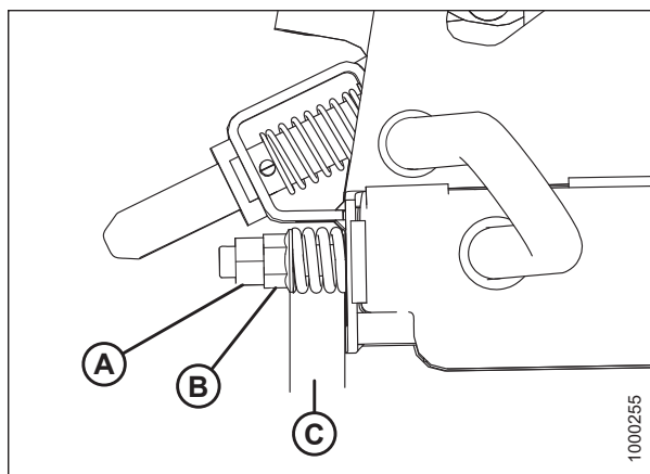
图 5.23: 转向张力调整装置
