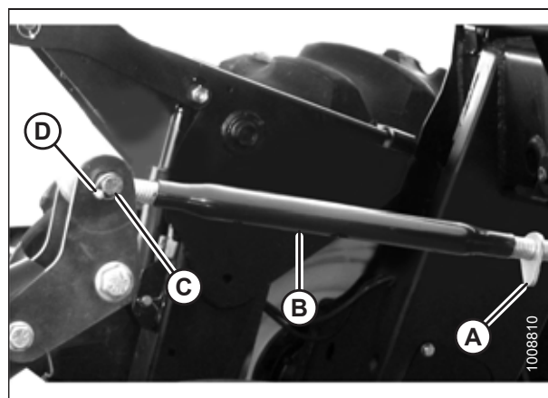
图 4.256: 机械中央升降
