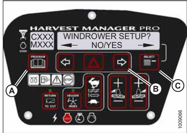
图 3.84: CDM 编程按钮
