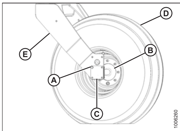
图 5.213: 叉式支撑从动轮
