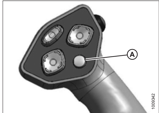
图 3.52: 地速控制杆
