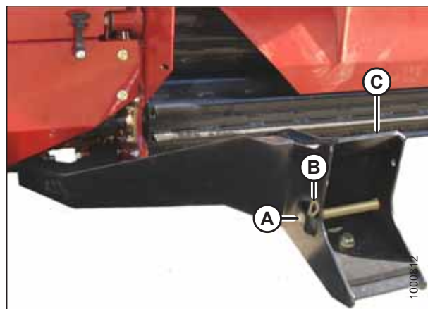
图 4.275: 割台连接座
