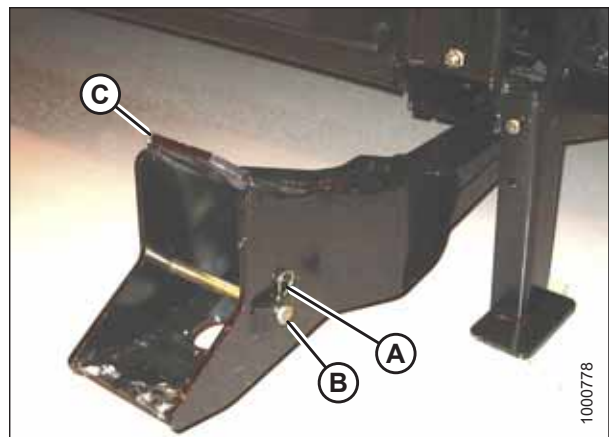
图 4.162: 割台连接座
