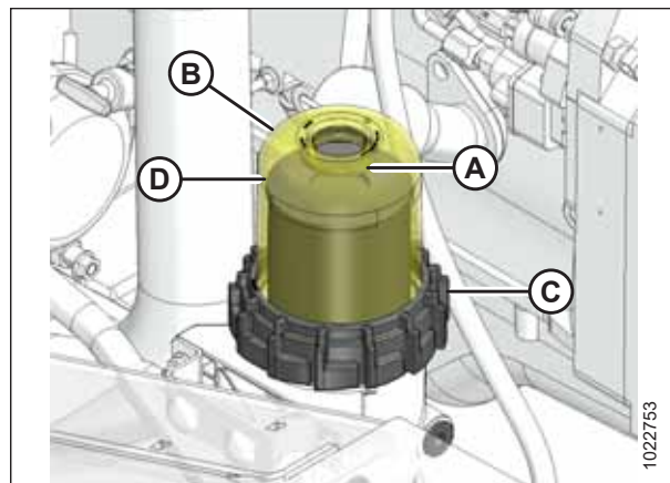
图 5.73: 初级燃油过滤器
