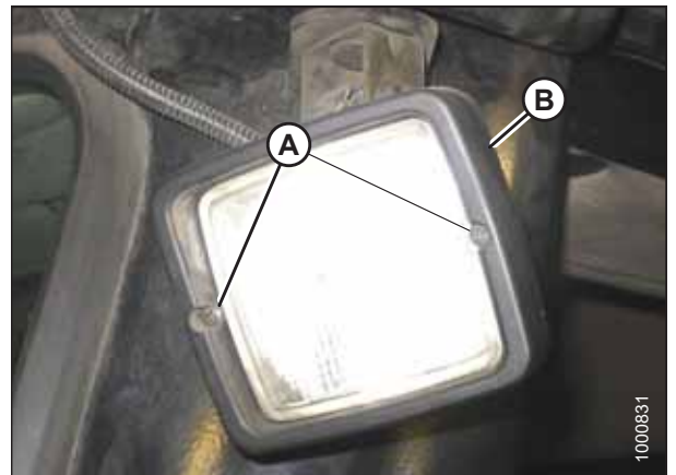
图 5.158: 后泛光灯
