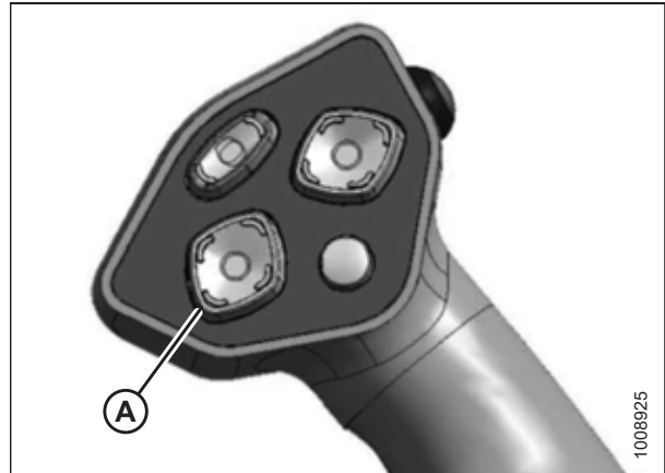
图 4.132: 地速控制杆
