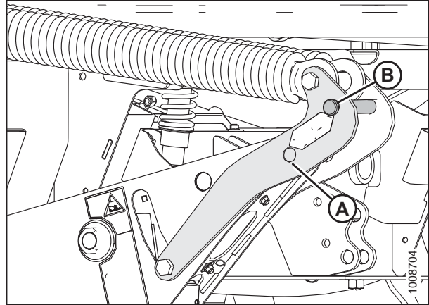
图 4.41: 提升臂
