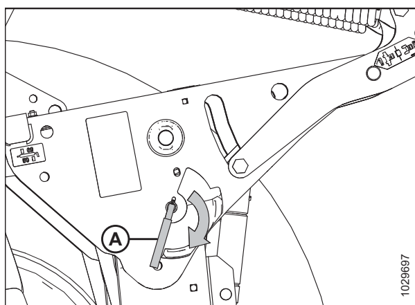
图 4.277: 安全撑杆
