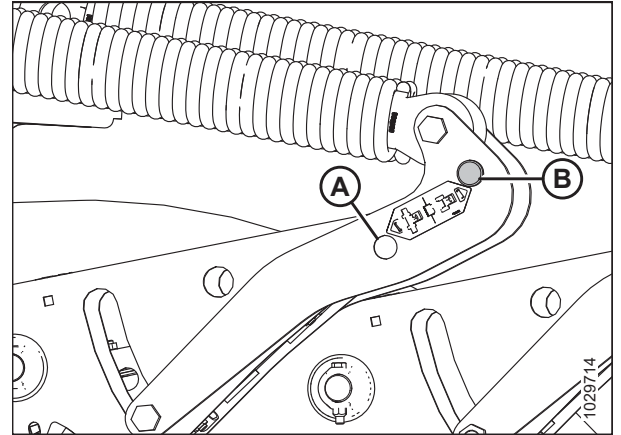
图 4.100: 割台浮动悬挂提升臂部件
