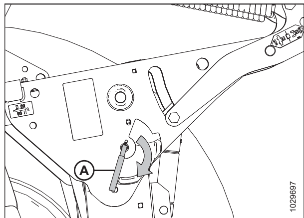
图 4.157: 安全撑杆
