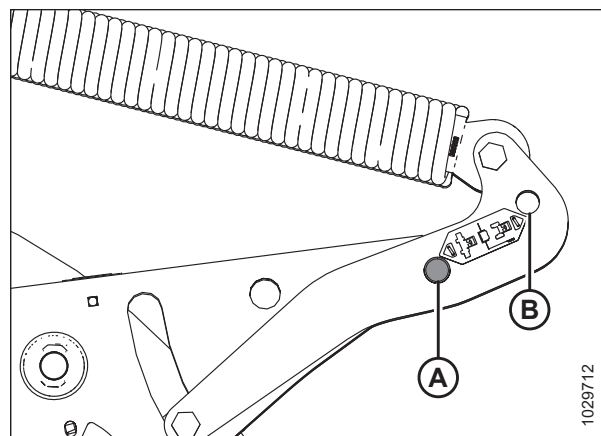
图 4.248: 割台浮动悬挂提升臂部件
