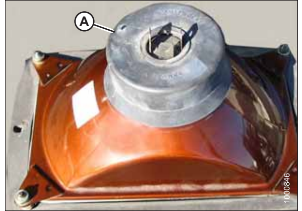
图 5.135: 前大灯组件
