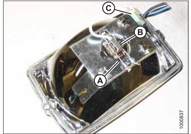
图 5.145: 泛光灯组件
