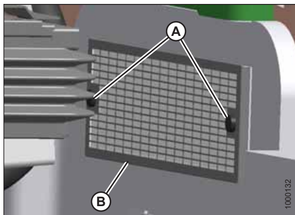
图 5.30: 回流空气过滤器
