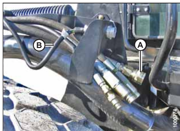
图 4.191: 割台驱动软管和线束
