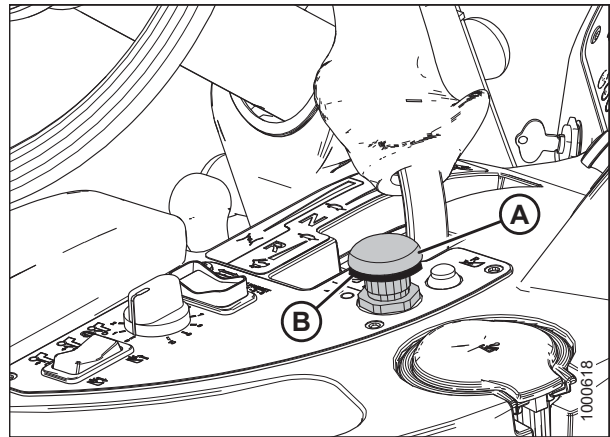
图 4.292: 割台驱动装置按钮
