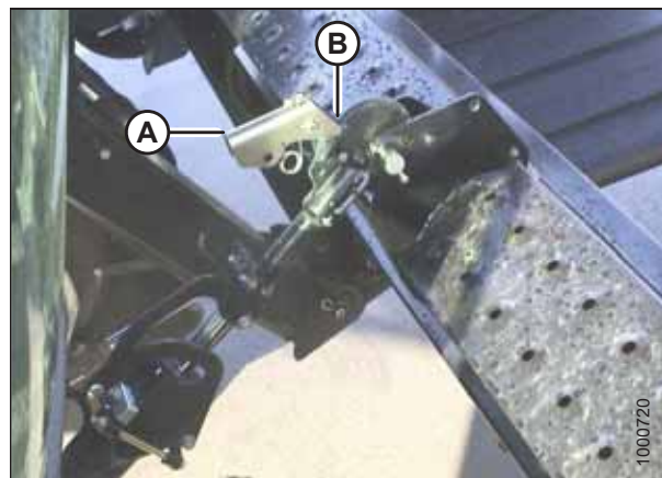
图 4.44: 液压升降
