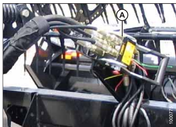
图 4.149: 拨禾轮液压系统
