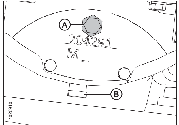
图 5.109: 齿轮箱润滑油放油塞
