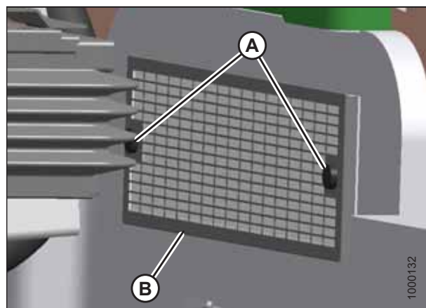
图 5.32: 回流空气过滤器
