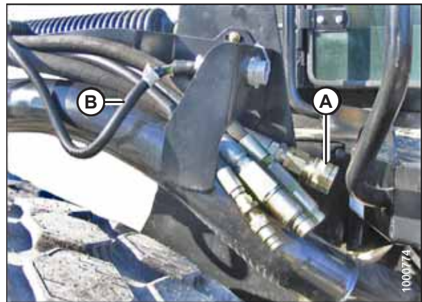
图 4.263: 割台驱动软管和线束
