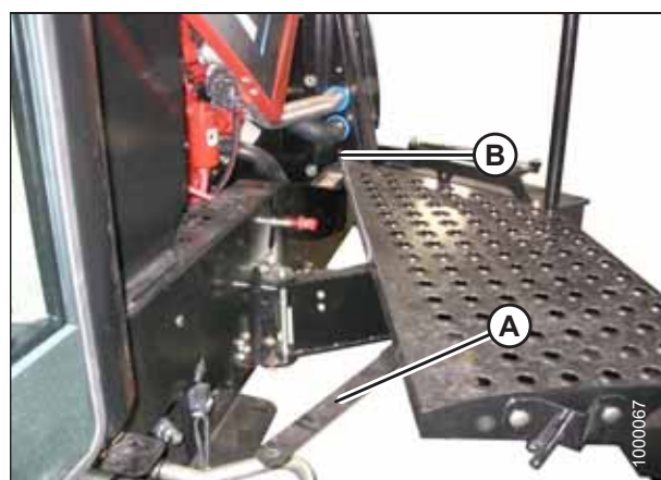
图 5.11: 平台
