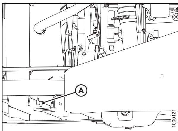
图 5.91: 散热器放水阀
