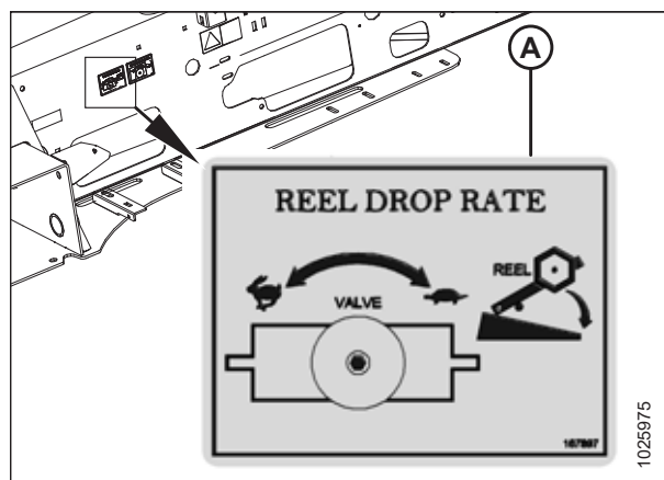
图 5.193: 贴标
