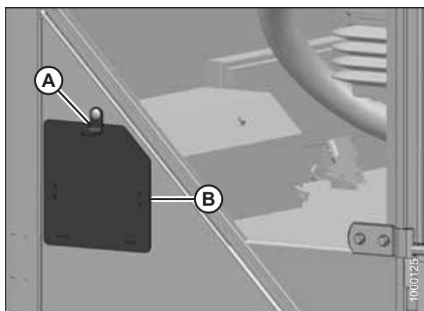
图 5.25: 过滤器托盘
