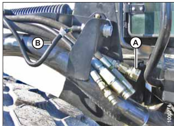
图 4.148: 割台驱动装置液压系统
