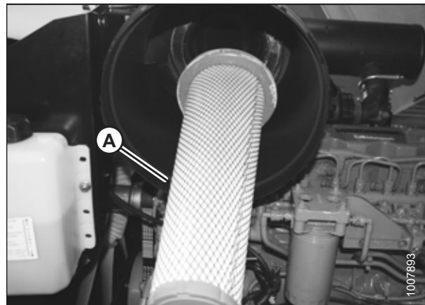
图 5.62: 次级滤芯
