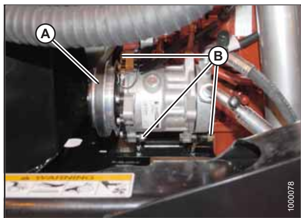
图 5.114: 空调压缩机
