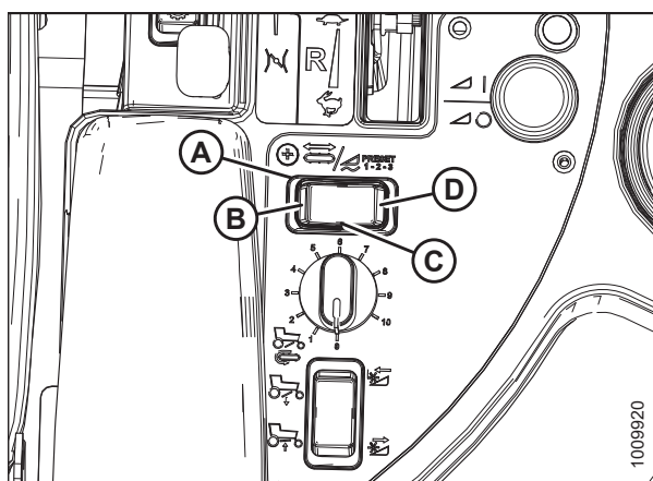
图 4.297: 输送带支承平移开关
