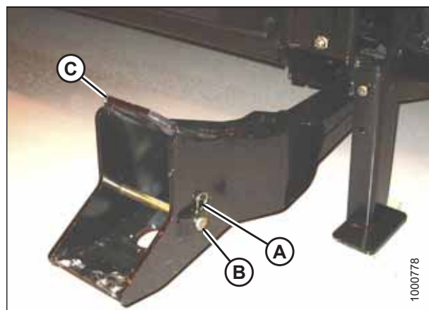
图 4.223: 割台连接座
