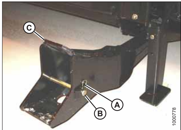
图 4.214: 割台连接座
