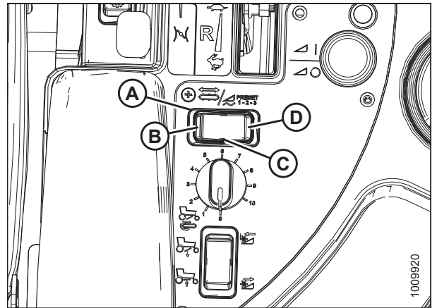
图 4.295: 输送带支承平移开关
