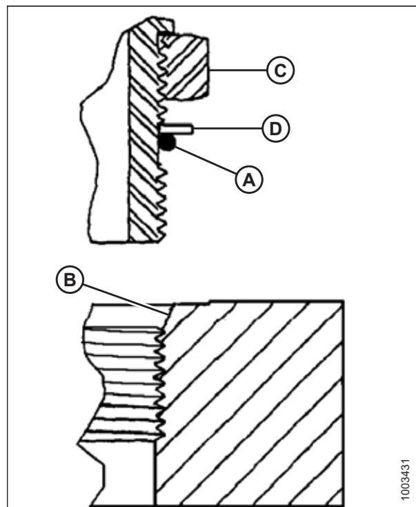
图 8.11: 液压接头
