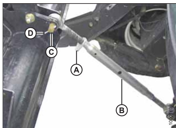
图 4.134: 机械中央升降
