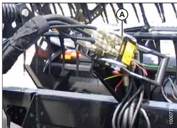
图 4.159: 拨禾轮液压系统
