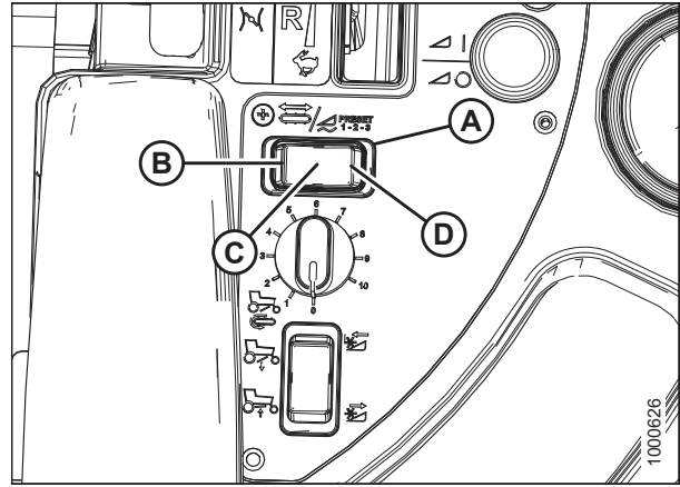
图 3.55: 割台开关
