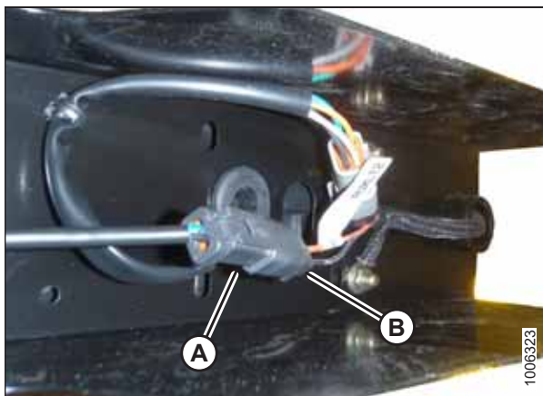
图 5.151: HID 辅助灯线束
