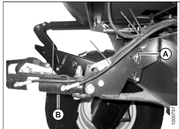
图 4.241: 不带自对准套件的液压中央升降
