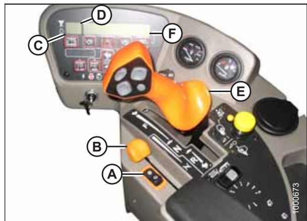
图 4.22: 操作员控制台
