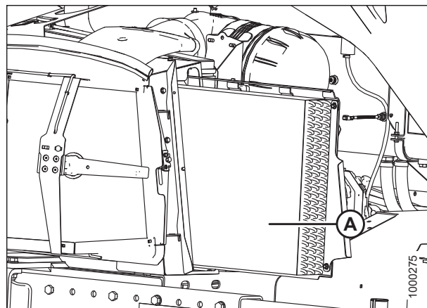
图 5.101: 空调冷凝器总成
