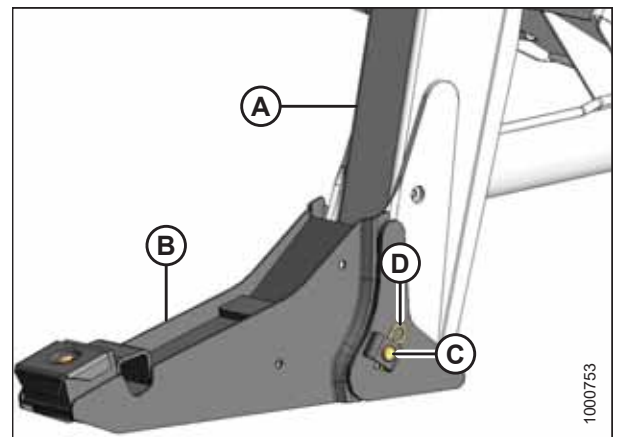
图 4.102: 割台连接座
