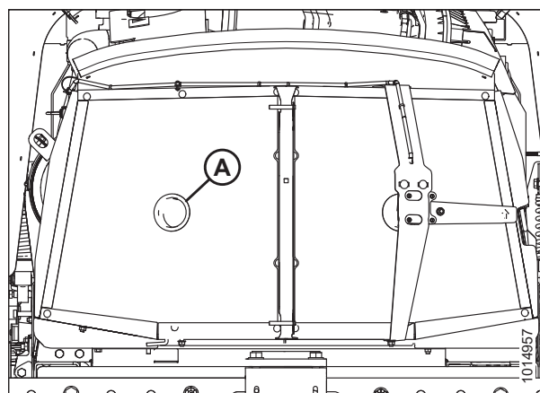
图 5.98: 冷却箱滤网
