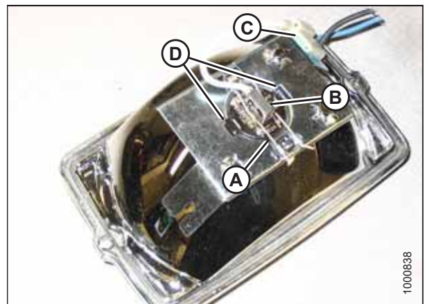
图 5.146: 泛光灯组件
