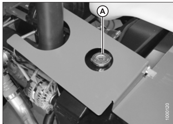
图 5.88: 散热器盖子
