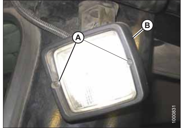
图 5.156: 后泛光灯
