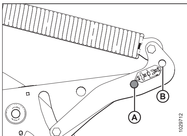
图 4.260: 割台浮动悬挂提升臂部件
