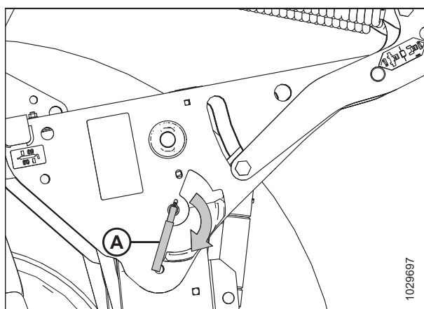
图 4.261: 安全撑杆控制杆
