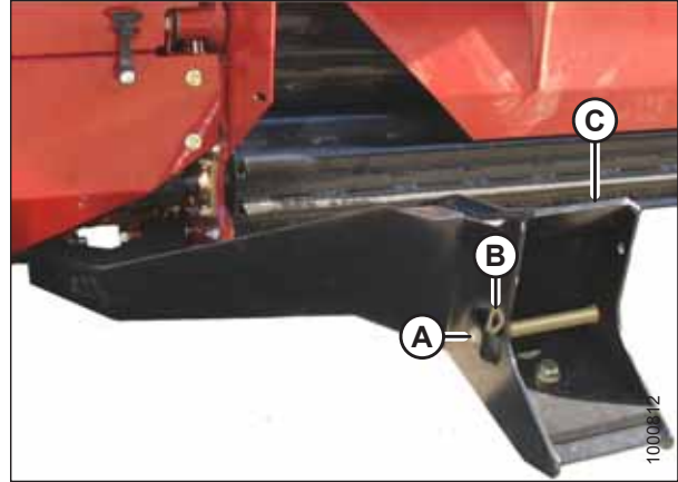
图 4.272: 割台连接座
