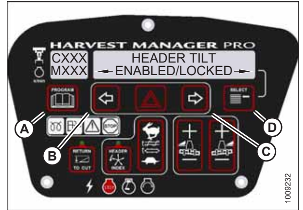
图 3.114: 割台倾斜控制装置锁定
