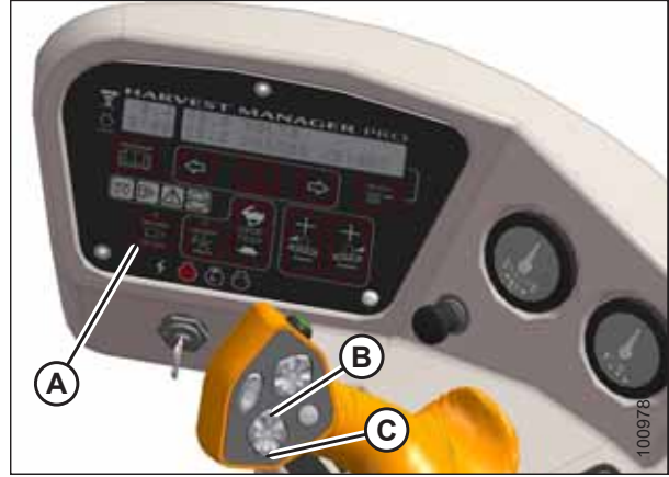
图 4.95: 操作员操作台
