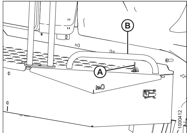
图 5.13: 平台闭锁
