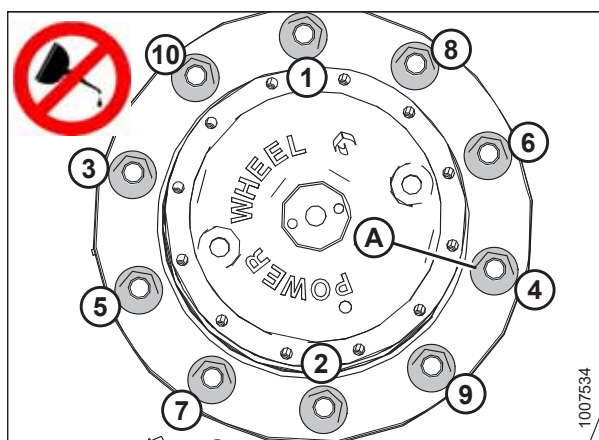
图 5.196: 车轮螺母拧紧顺序
