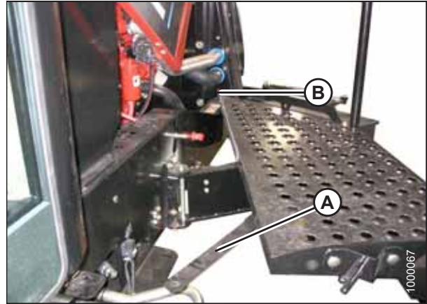
图 5.12: 平台
