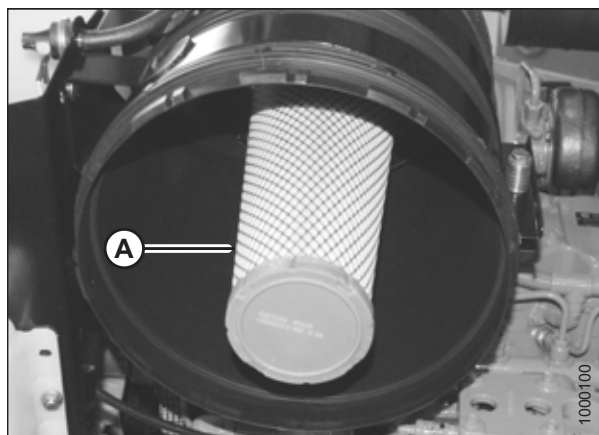
图 5.61: 次级滤芯
