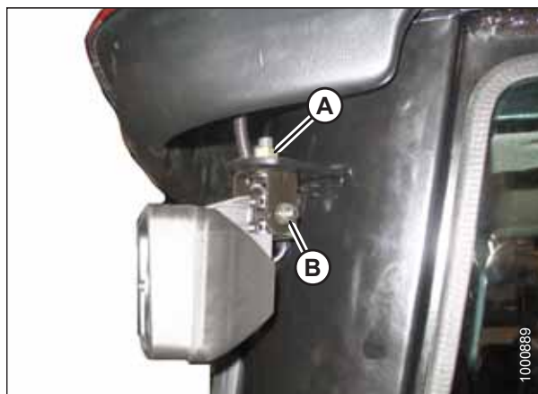
图 5.155: 后泛光灯
