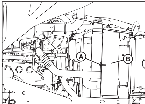
图 5.102: 左侧冷却器检修门
