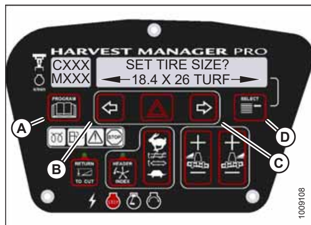
图 3.107: 轮胎尺寸
