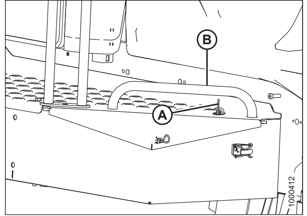
图 5.6: 平台门锁
