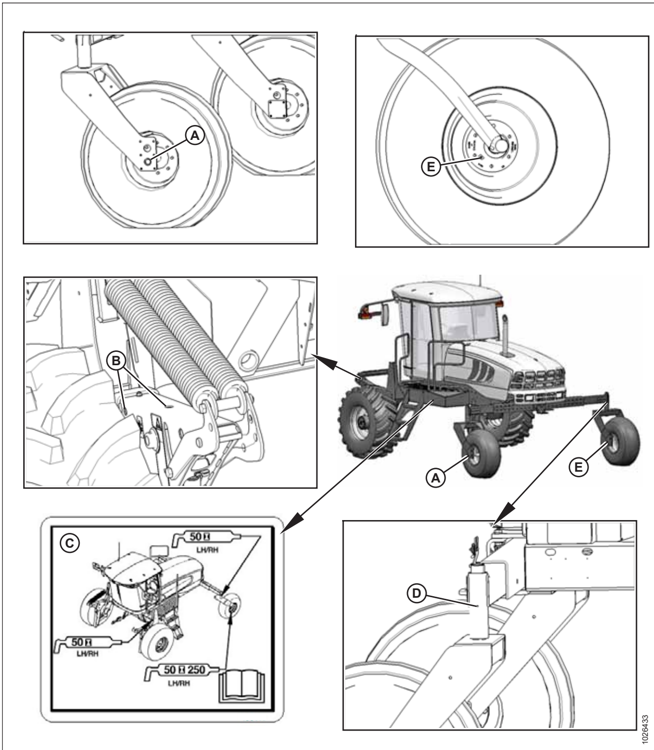
图 5.15: 润滑点
