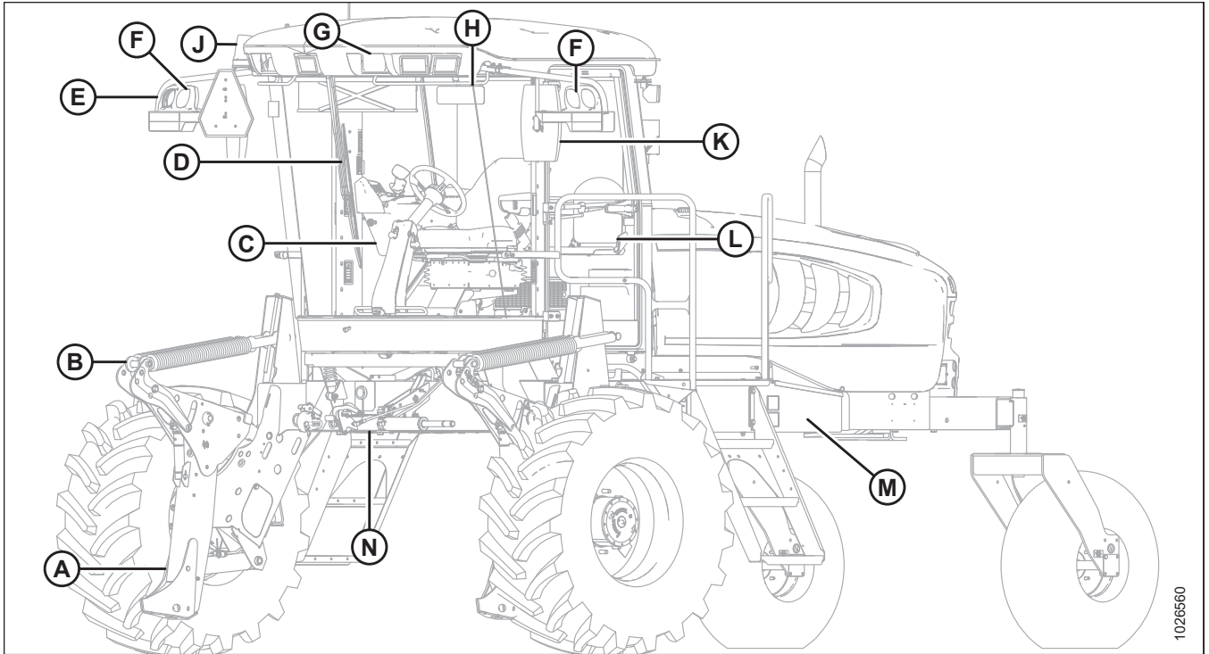
图 2.5: 驾驶室前置正视图
