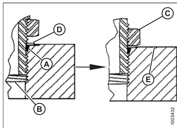
图 8.12: 液压接头
