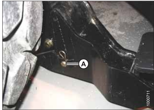
图 4.199: 割台支座
