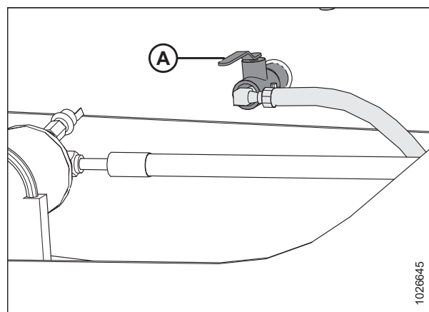
图 5.79: 燃油切断阀
