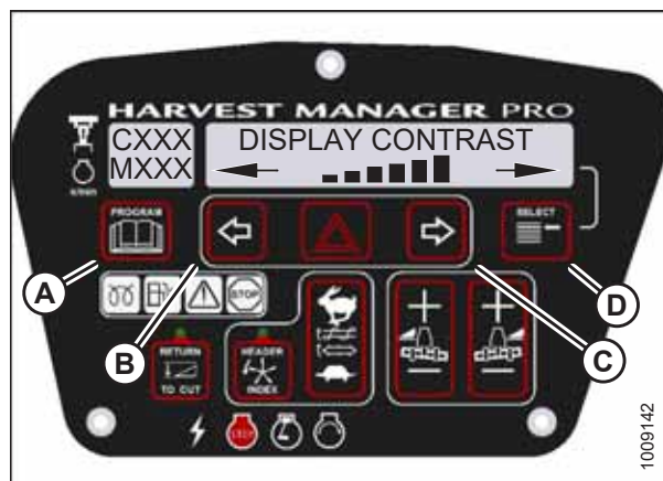
图 3.77: 显示屏对比度设置
