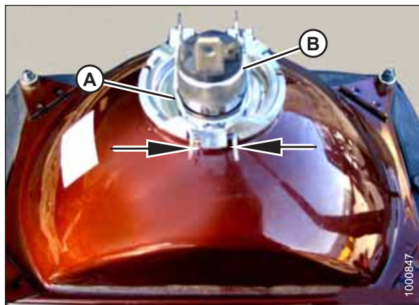
图 5.133: 前大灯组件
