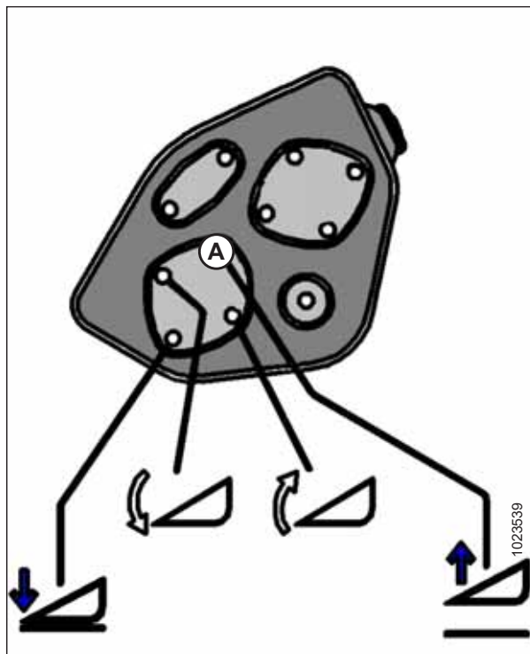
图 3.142: GSL 上的割台高度控制装置
