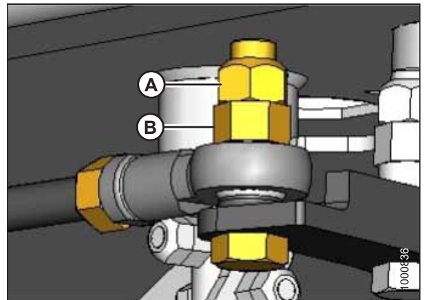
图 5.22: 转向连杆
