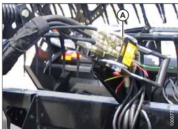
图 4.130: 拨禾轮液压系统
