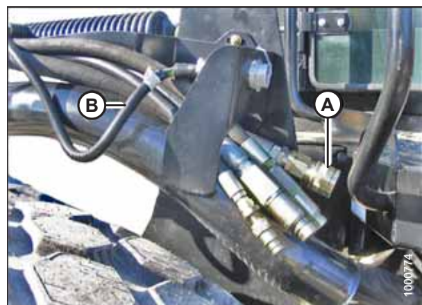
图 4.176: 割台驱动软管和线束
