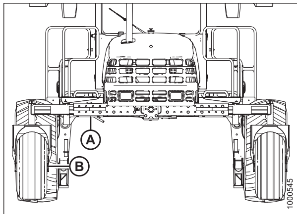
图 5.212: 从动轮和行走梁 - 发动机前置视图
