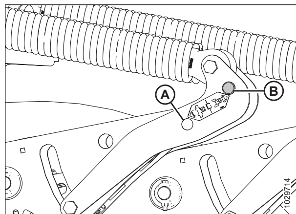
图 4.163: 割台浮动悬挂提升臂部件
