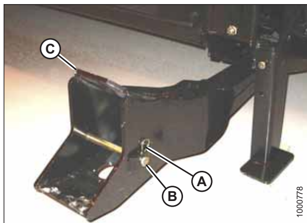
图 4.177: 割台连接座
