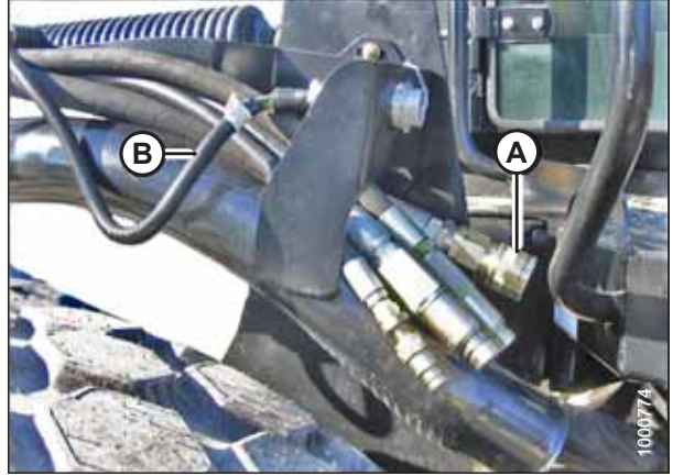
图 4.203: 割台驱动软管和线束
