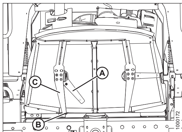
图 5.99: 驱尘器组件
