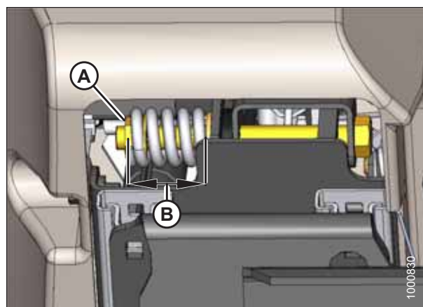
图 5.17: GSL 调整弹簧
