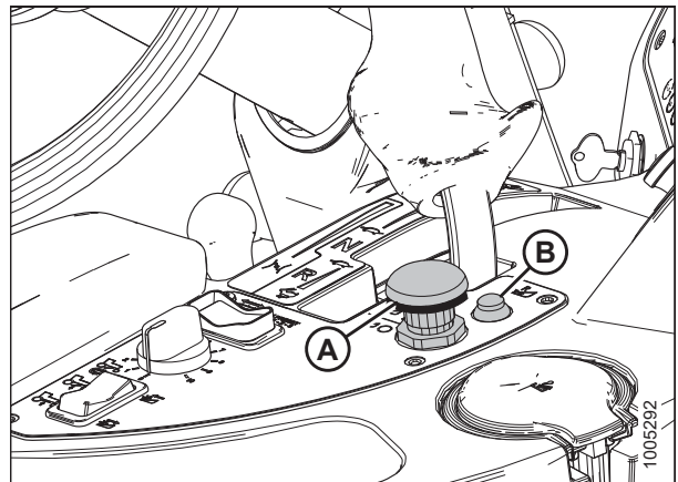
图 3.49: 割台驱动装置开关
