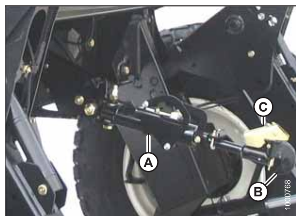
图 4.212: 液压中央升降
