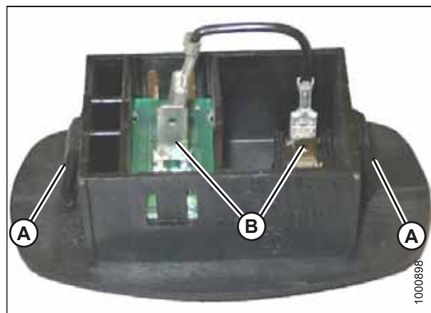
图 5.167: 环境照明灯组件
