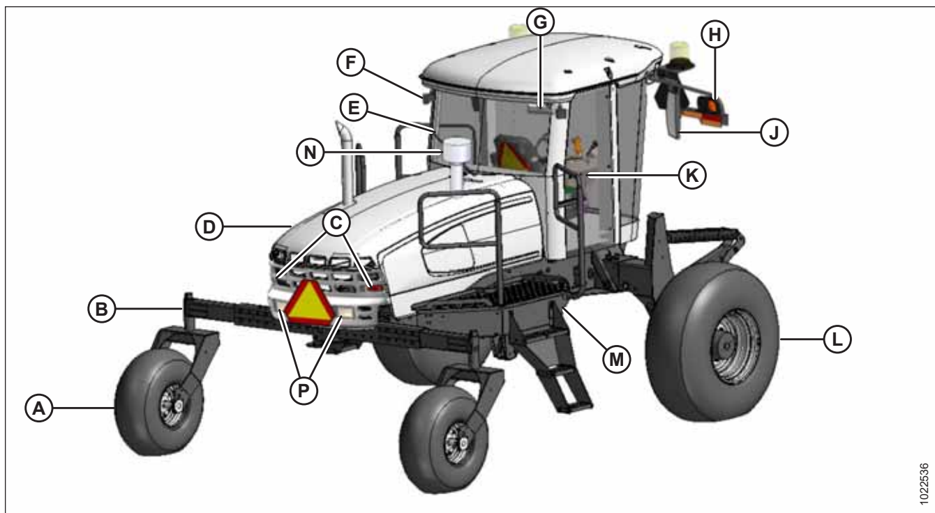
图 2.6: 驾驶室前置后视图
