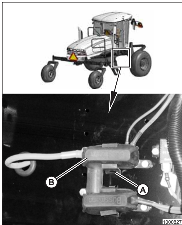
图 5.174: 125A 主保险丝
