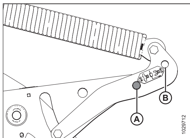
图 4.201: 割台浮动悬挂提升臂部件
