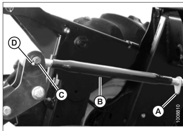
图 4.196: 机械中央升降
