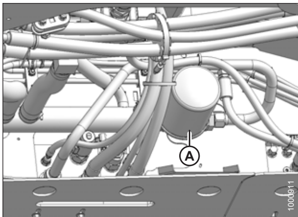
图 5.184: 回流滤油器
