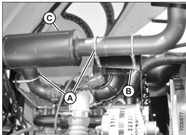
图 5.111: 排气系统
