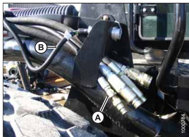
图 4.271: 割台驱动装置液压系统
