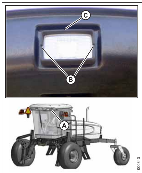
图 5.144: 前泛光灯
