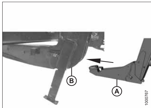
图 4.133: 割台支腿和连接座
