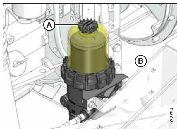
图 5.74: 初级燃油过滤器
