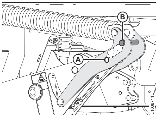
图 4.209: 割台浮动悬挂提升臂部件
