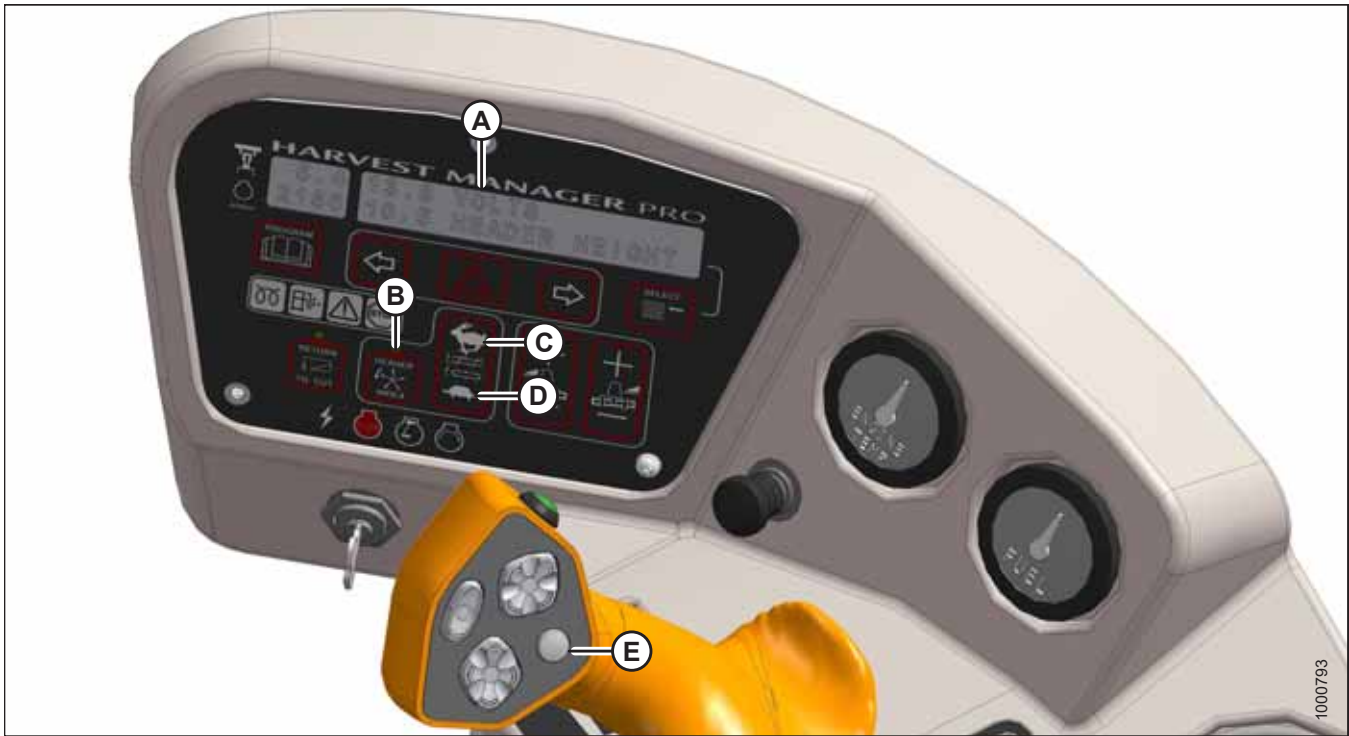
图 4.290: 操作员控制台
