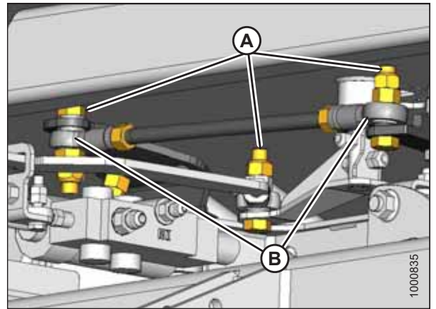
图 5.21: 转向连杆
