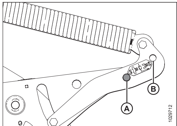
图 4.173: 割台浮动悬挂提升臂部件
