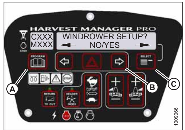
图 3.98: CDM 编程按钮
