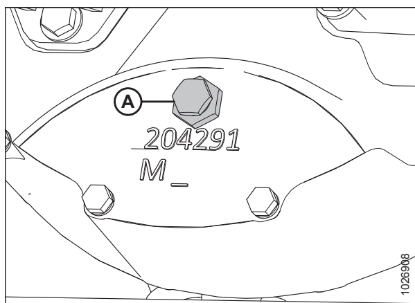
图 5.107: 齿轮箱润滑油检查塞
