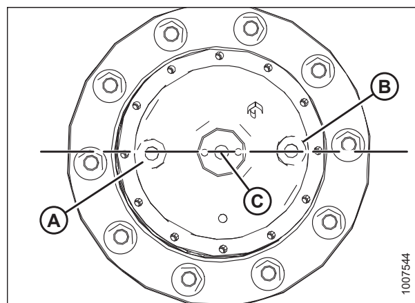
图 5.198: 驱动轮轮毂
