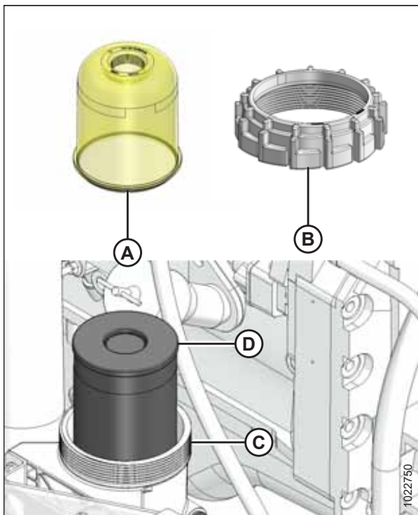
图 5.71: 初级燃油过滤器
