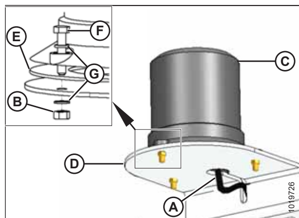
图 5.162: 更换信号灯
