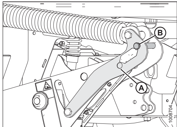
图 4.267: 割台浮动悬挂提升臂部件
