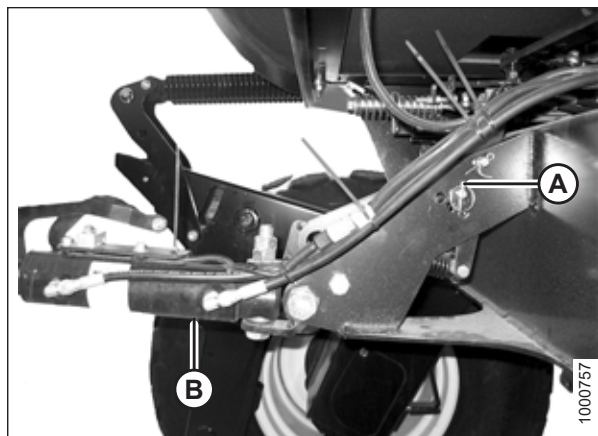
图 4.119: 不带自对准套件的液压中央升降
