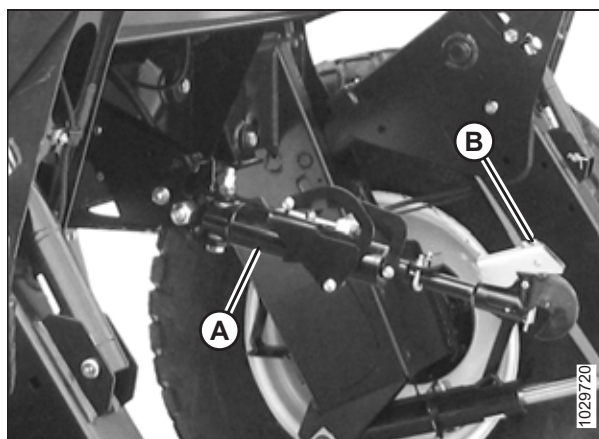
图 4.168: 液压中央升降
