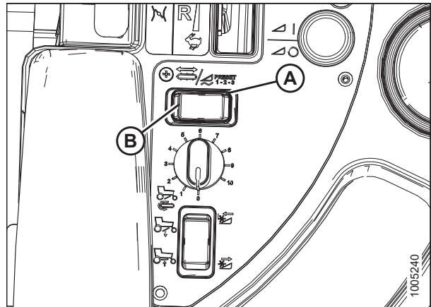
图 4.73: 浮动悬挂预设值开关
