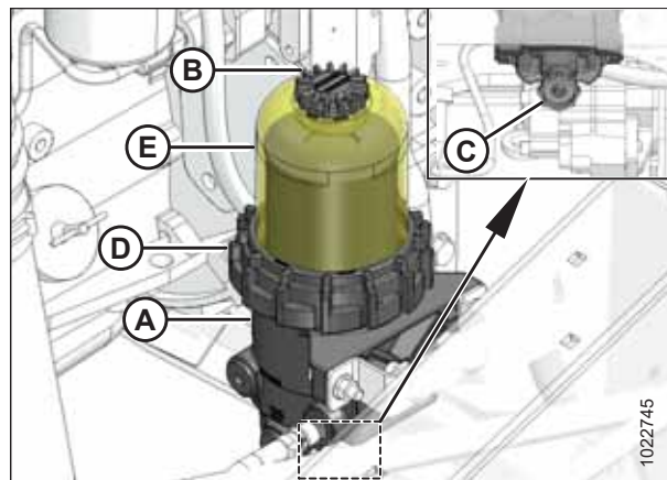
图 5.69: 初级燃油过滤器
