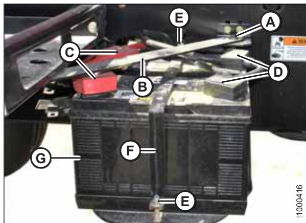
图 5.128: 蓄电池
