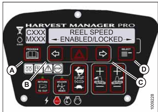
图 3.135: 拨禾轮速度控制装置锁定
