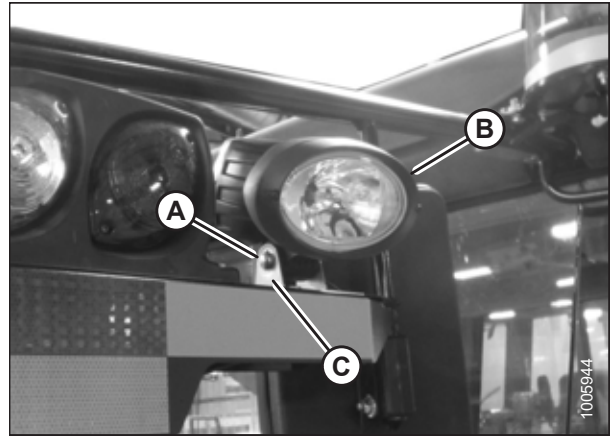
图 5.148: HID 辅助灯
