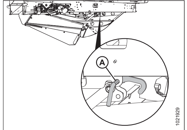
图 4.97: 放铺导板锁定装置
