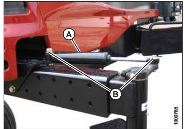
图 5.219: 缓冲器
