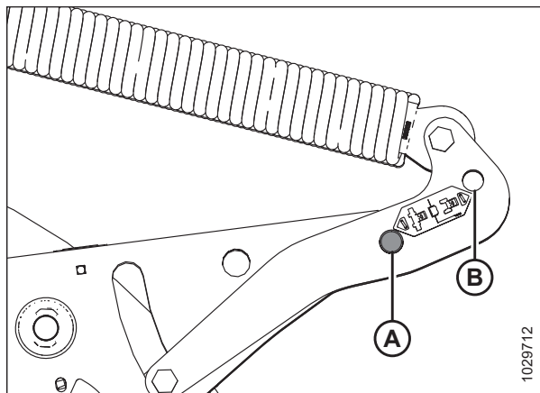
图 4.126: 割台浮动悬挂提升臂部件
