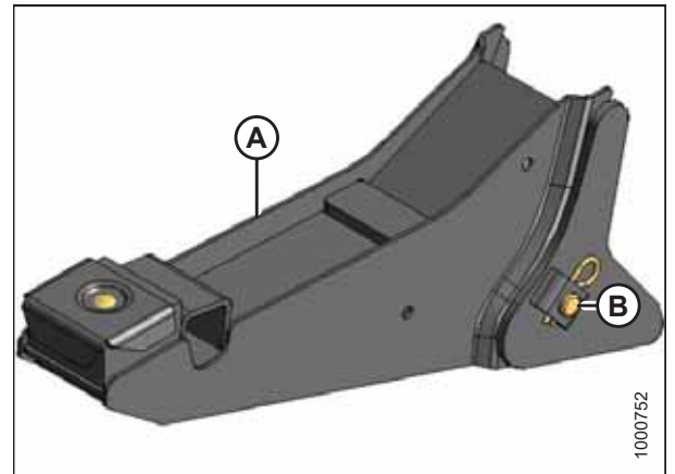
图 4.101: 割台连接座
