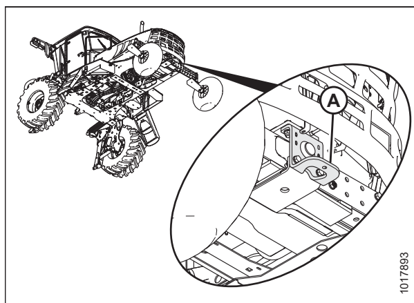
图 4.65: 紧急牵引
