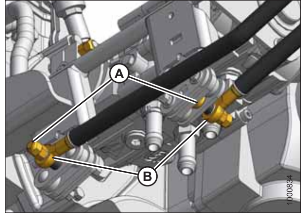
图 5.20: 转向拉杆 (泵末端)
