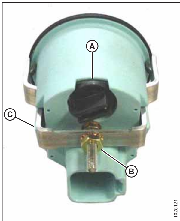
图 5.164: 控制台仪表的背面
