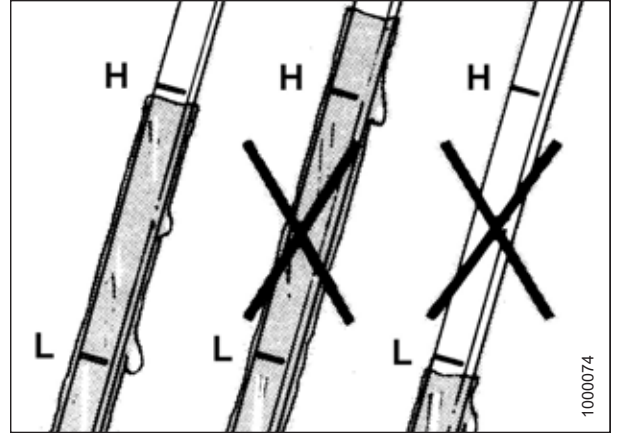
图 5.179: 液压油油位
