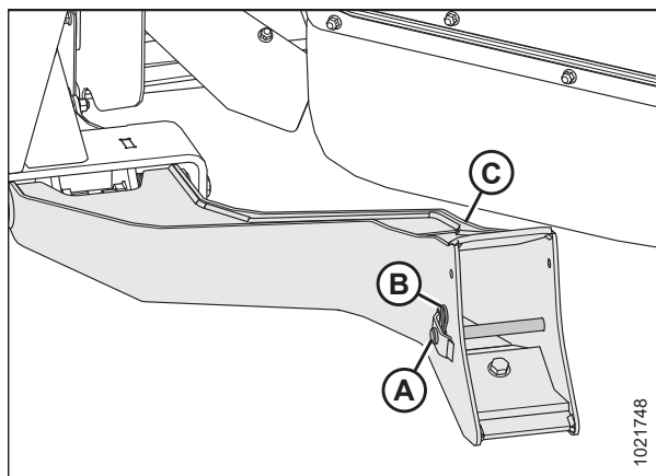
图 4.252: 割台支座
