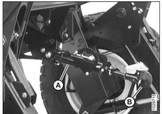
图 4.244: 液压中央升降
