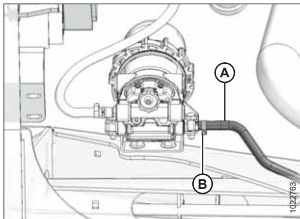
图 5.80: 燃油系统
