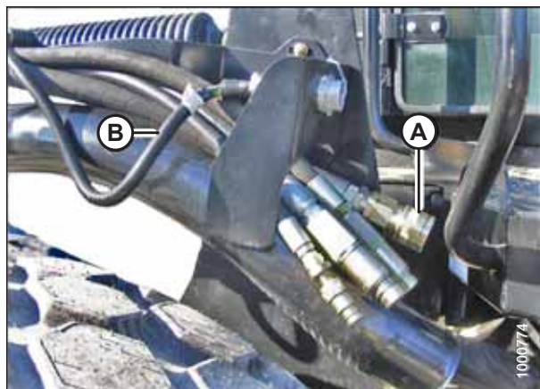
图 4.237: 割台驱动软管和线束
