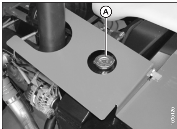
图 5.86: 发动机冷却系统
