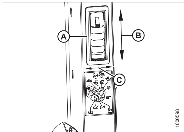
图 3.27: 可调百叶盒
