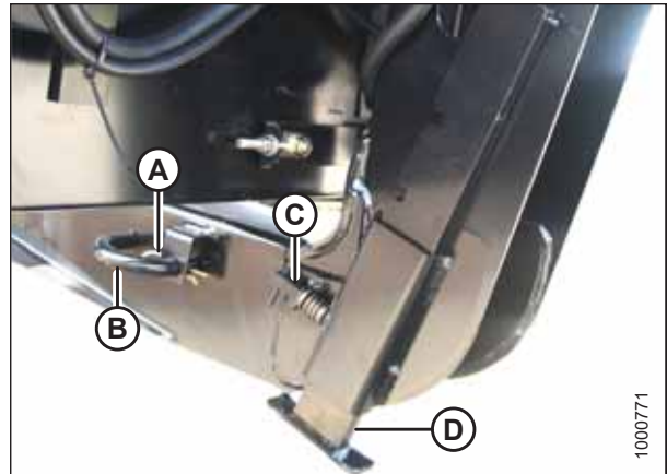
图 4.137: 割台支腿
