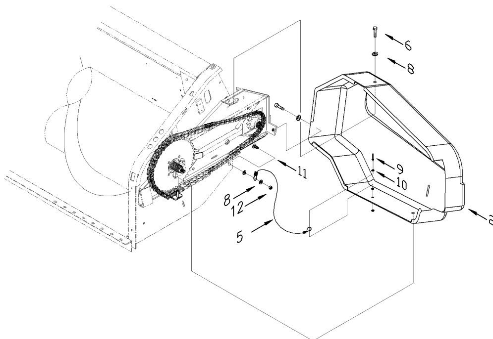
LEFT SIDE
