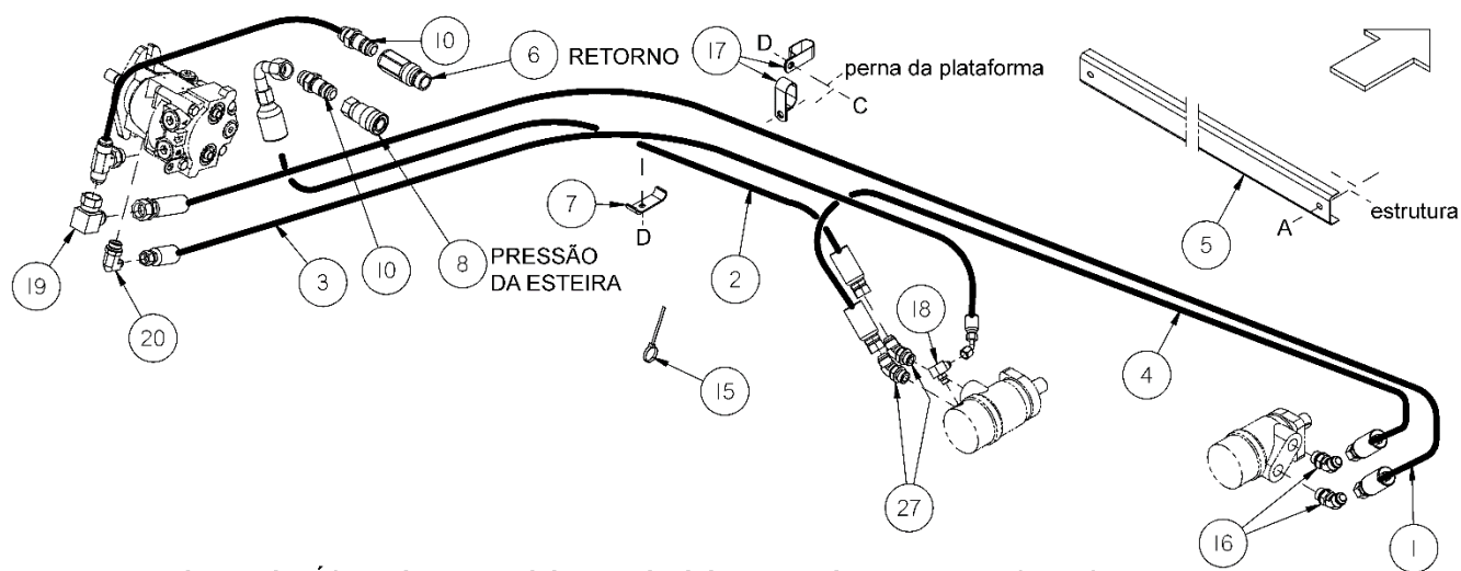
PLATAFORMAS RÍGIDAS DE 15' COM DESLOCAMENTO MANUAL DO DECK
