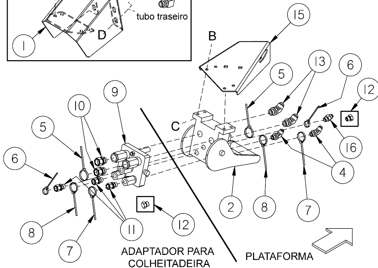
PLATAFORMA COLHEITADEIRA
