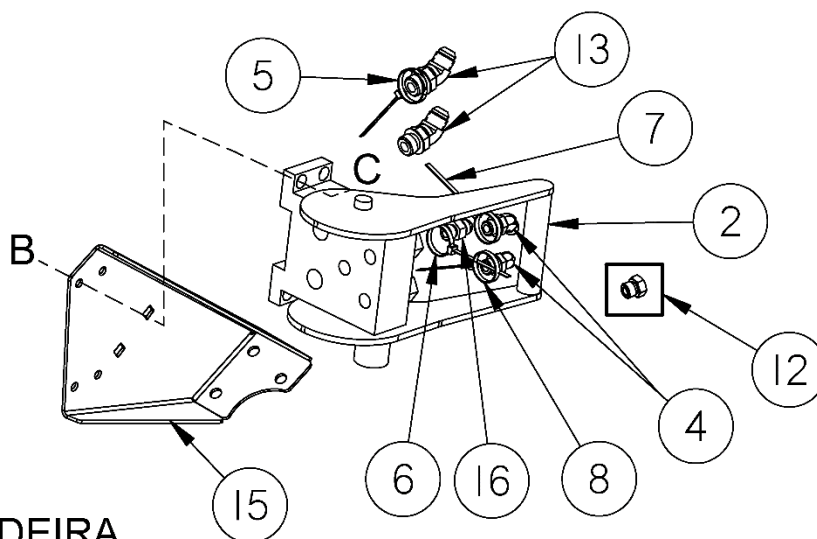
ADAPTADOR PARA COLHEITADEIRA
