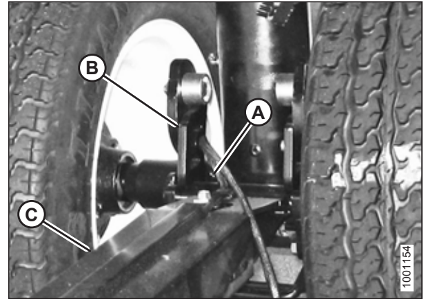
pav. 3.61: Standžiosios vilkties fiksatorius
