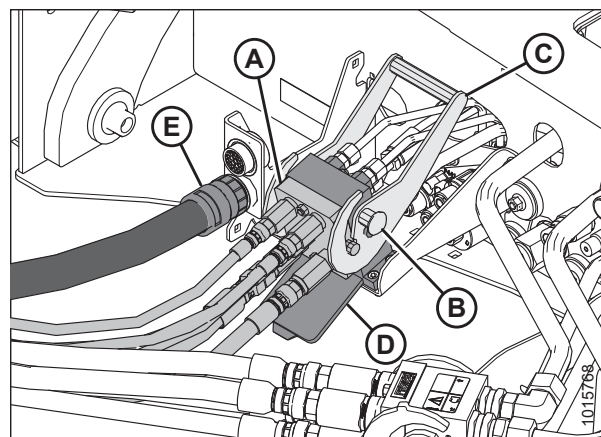
pav. 4.11: Transporterio / lenktuvų daugiaelementė jungtis
