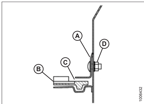
pav. 5.129: Užpakalinio skydo deflektorius
