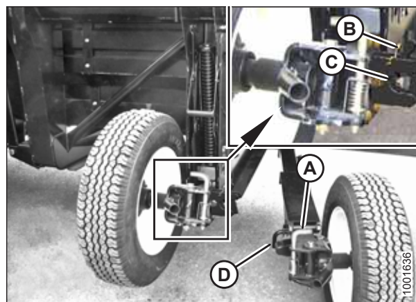
pav. 3.72: Galiniai ratai
