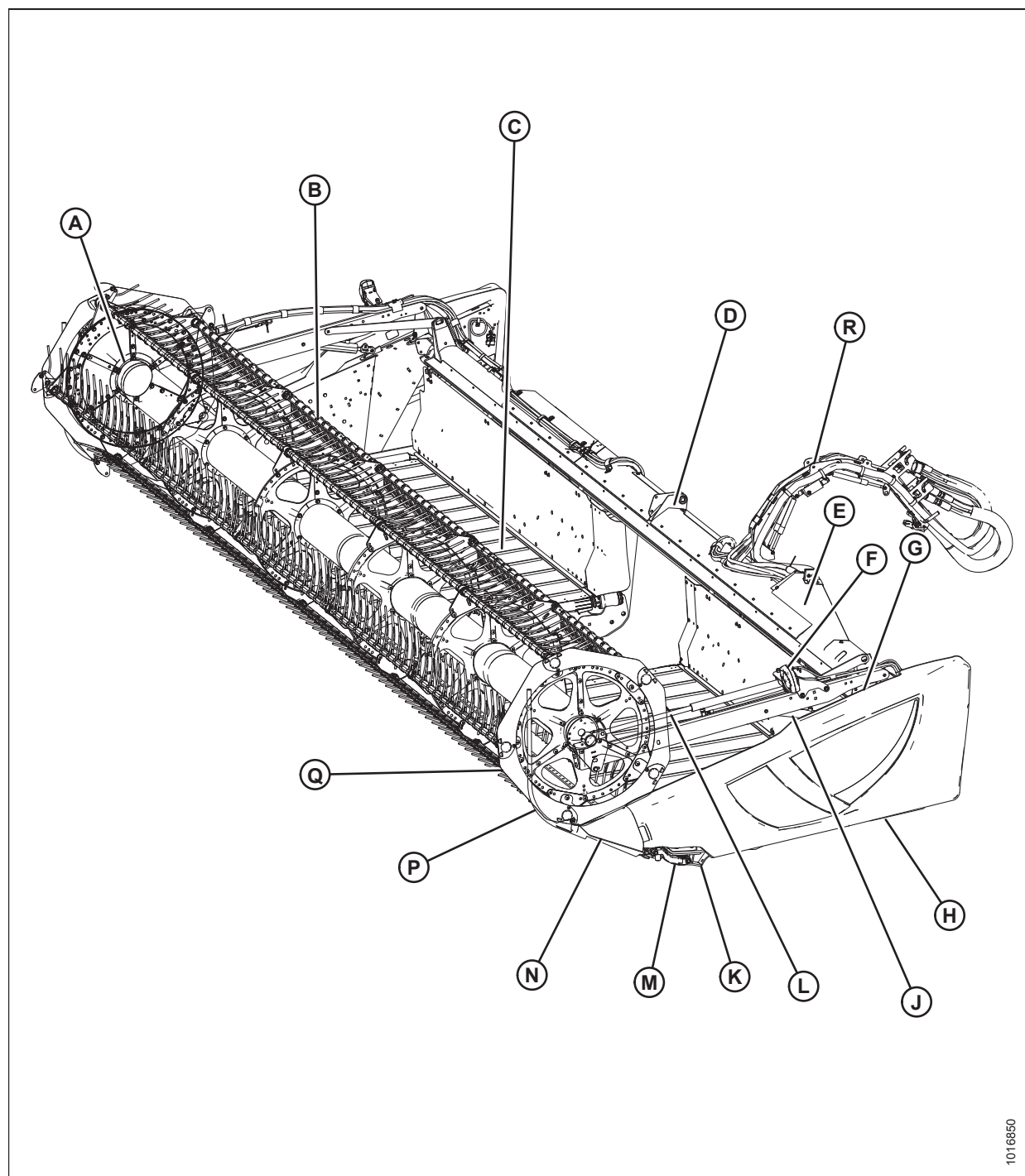
pav. 2.1: Pradalginės javapjovės pjaunamosios komponentai
