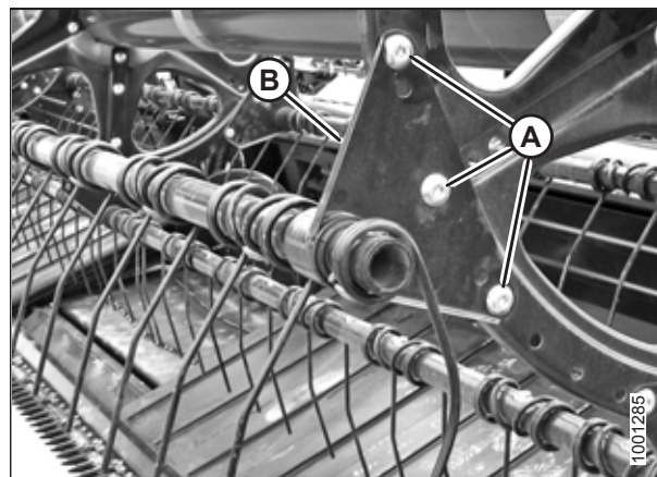
pav. 5.176: Virbo vamzdelio svirtas
