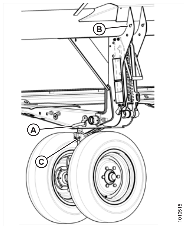
pav. 3.77: Kairieji priekiniai ratai
