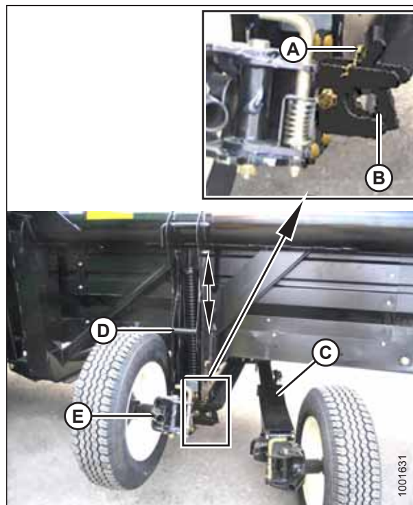
pav. 3.78: Ašių atskyrimas
