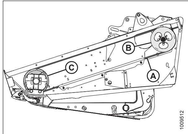
pav. 5.76: Dalgio pvara
