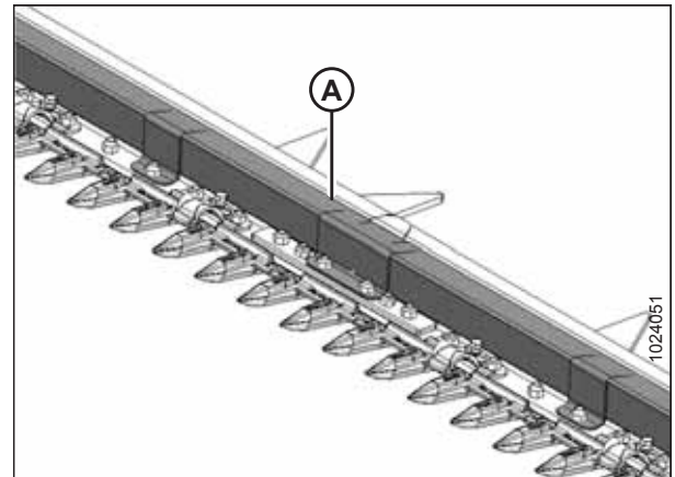
pav. 6.9: Akmenų blokavimo įtaisas
