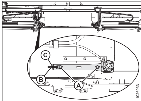
pav. 5.120: Kairysis platformos pavaros volelis – dešinioji pusė yra priešinga
