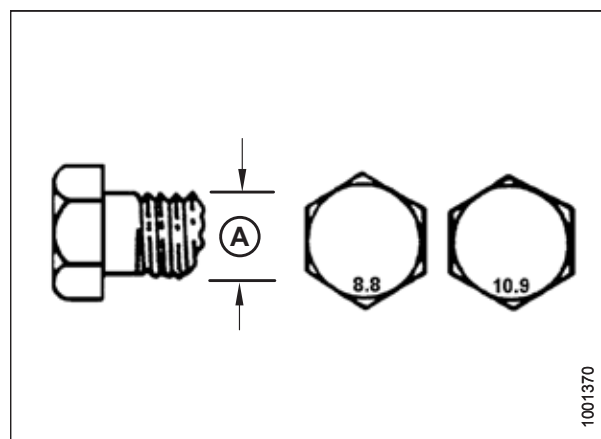
pav. 9.6: Varžtų klasės
