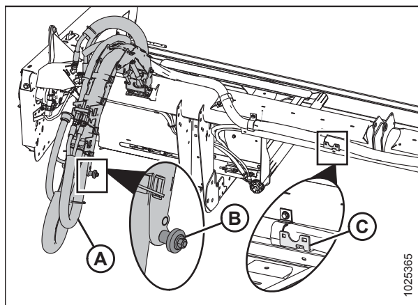
pav. 4.14: Hidraulinė žarnų valdymo sistema – taikoma D115X pjaunamosioms
