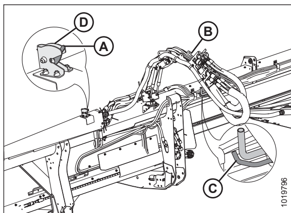
pav. 4.13: Hidraulinė žarnų valdymo sistema – taikoma visoms pjaunamosioms, išskyrus D115X
