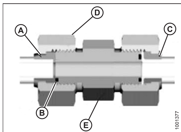
pav. 9.15: Hidraulinis tvirtinimo elementas
