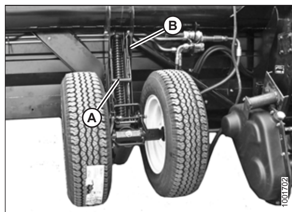
pav. 3.20: Kairieji ratai
