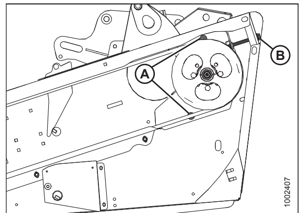
pav. 5.74: Dvigubų dalgį pavara be laiko nuostatos
