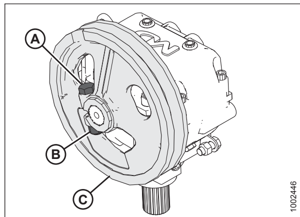
pav. 5.53: Dalgių pavarų dėžė ir skriemulys
