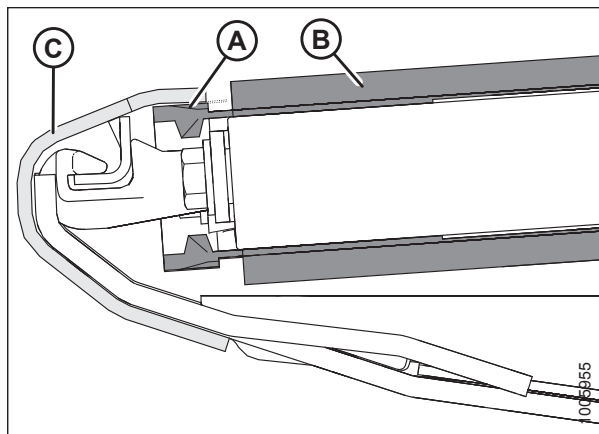
pav. 5.124: Transporterio sandariklis
