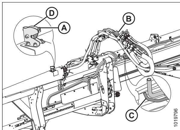
pav. 4.3: Hidraulinė žarnų valdymo sistema – taikoma visoms pjaunamosioms, išskyrus D115X
