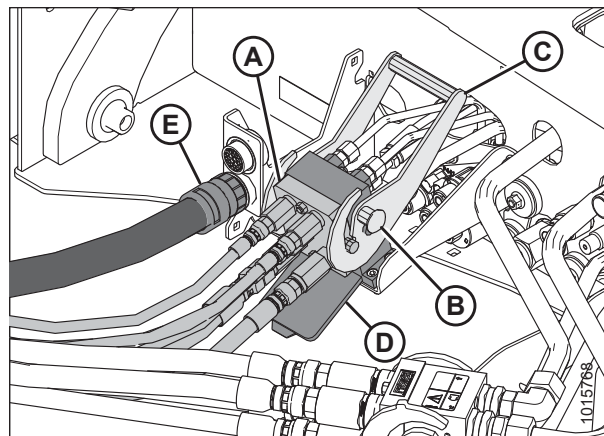
pav. 4.6: Transporterio / lenktuvų daugiaelementė jungtis
