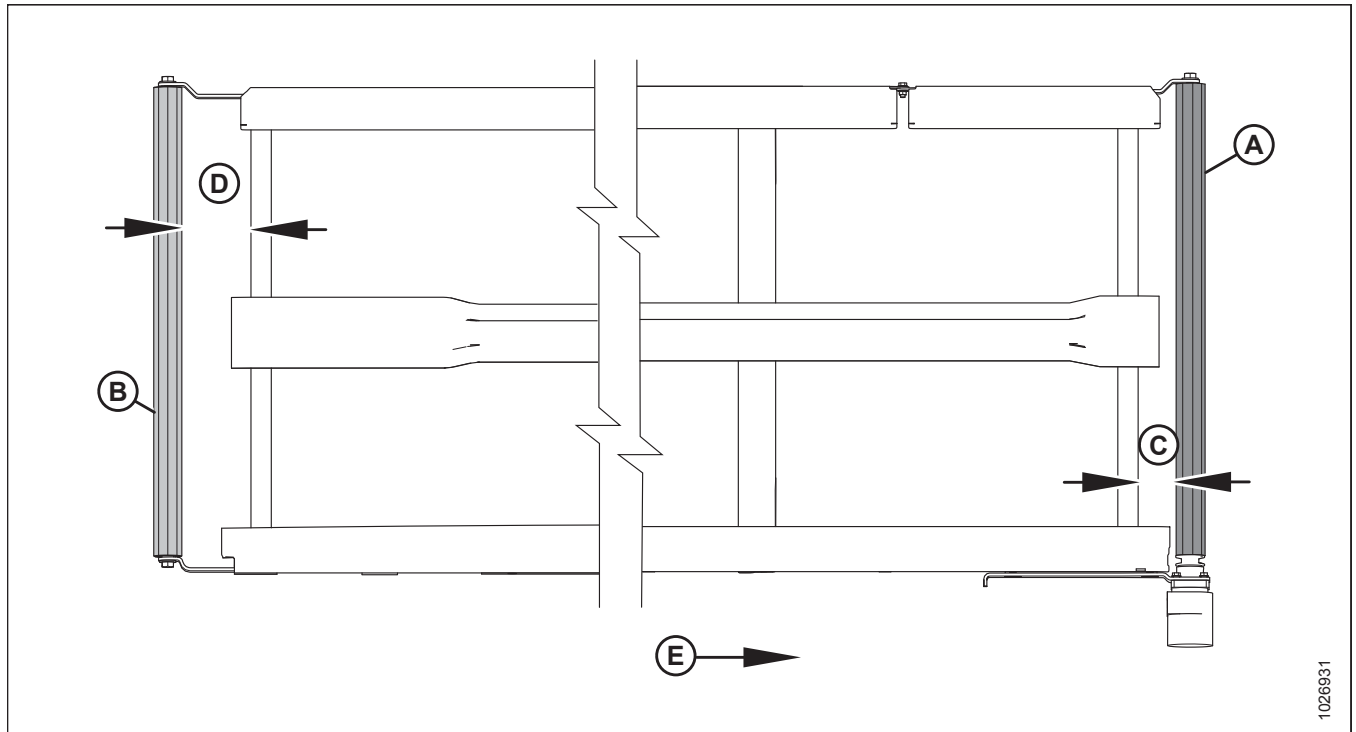
pav. 5.119: Transporterio vyniojimo apžvalga
