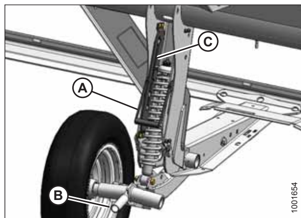
pav. 3.23: Stabilizavimo ratas
