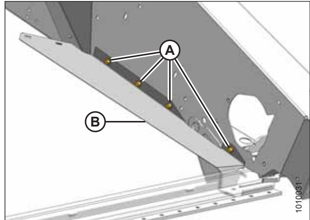
pav. 5.158: Priekinis deflektorius
