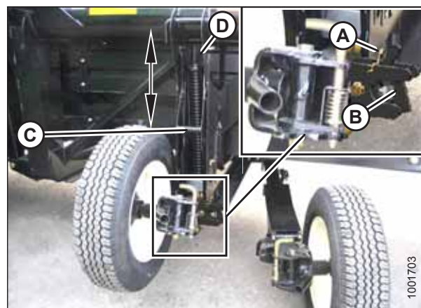
pav. 3.19: Dešinieji ratai
