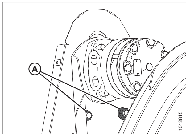
pav. 5.233: Viengubų lenktuvų pavara – dvigubų lenktuvų pavara yra panaši
