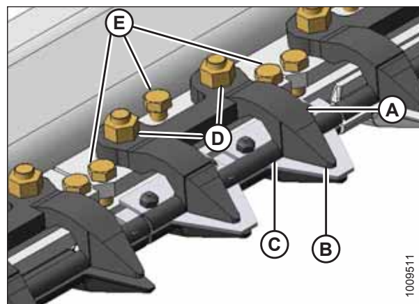
pav. 5.42: Raženos apsaugos
