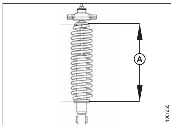
pav. 3.25: Spyruoklės suspaudimas
