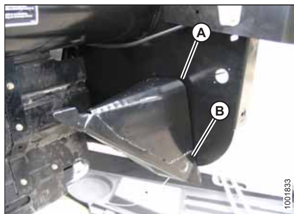
pav. 3.41: Saugomas pasėlių skirtuvas
