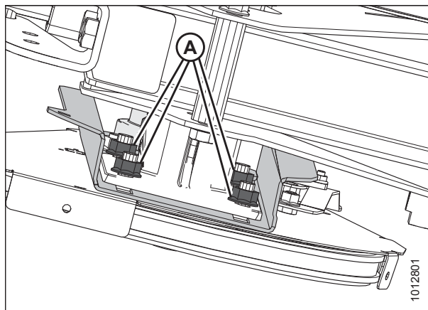
pav. 5.234: Viengubų lenktuvų pavara – vaizdas iš lenktuvų apatinės pusės
