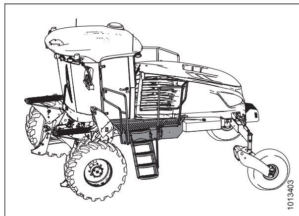
pav. 4.8: Kairioji pradalginės javapjovės platforma
