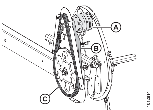
pav. 5.232: Viengubų lenktuvų pavara – dvigubų lenktuvų pavara yra panaši
