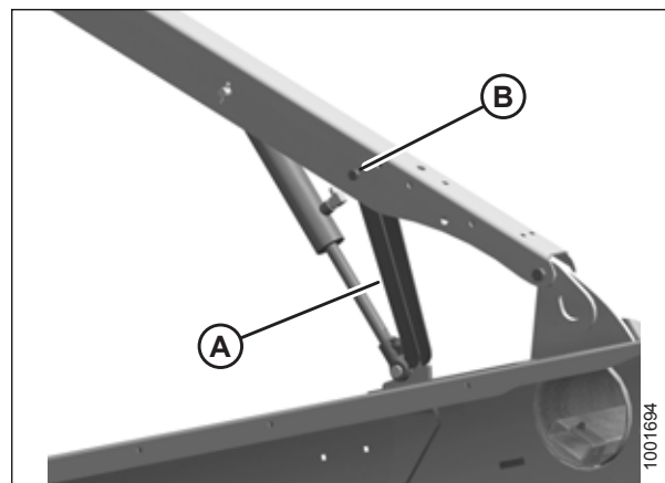
pav. 3.3: Užfiksuota lenktuvų saugos atrama – pavaizduota kairioji pusė
