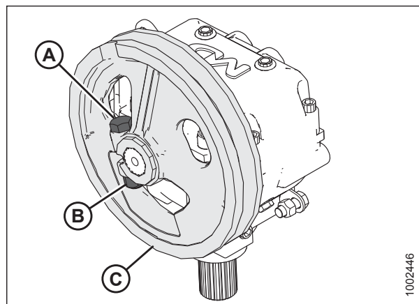
pav. 5.55: Dalgių pavarų dėžė ir skriemulys
