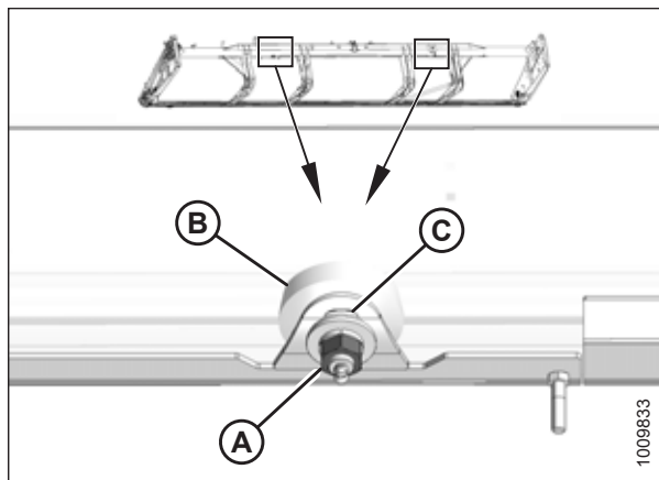
pav. 5.105: Kryžminio veleno atrama
