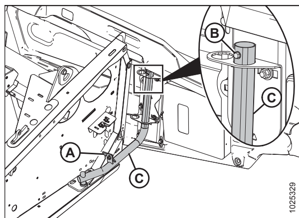
pav. 3.12: Kairės pusės galinis gaubtas ant D1X serijos juostinės pjaunamosios
