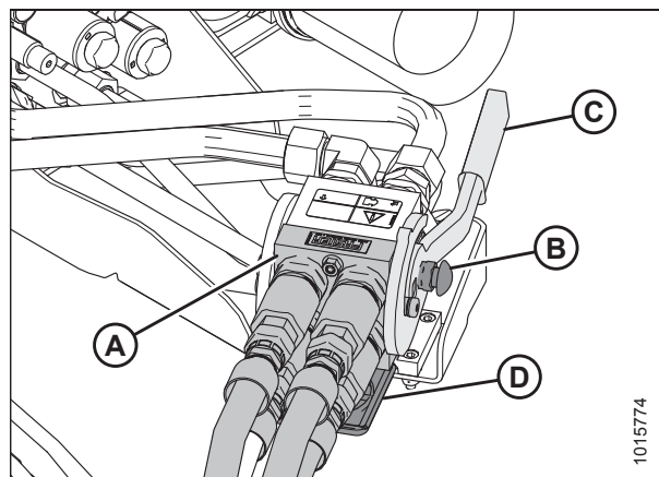
pav. 4.7: Dalgio / lenktuvų pavaros daugiaelementė jungtis
