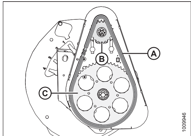
pav. 5.256: Lenktuvų pvara
