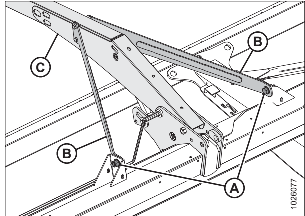
pav. 5.173: Lenktuvų vidurinisys atraminis svartas
