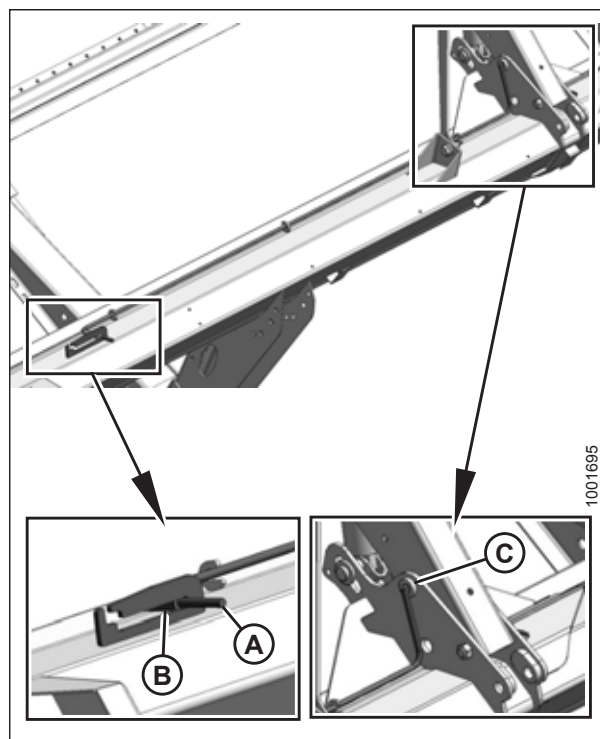
pav. 5.123: Lenktuvų saugos atrama – centrinis svirtas
