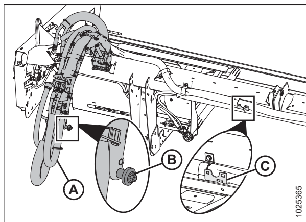
pav. 4.4: Hidraulinė žarnų valdymo sistema – taikoma D115X pjaunamosioms
