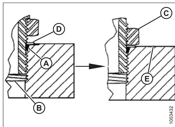
pav. 9.12: Hidraulinis tvirtinimo elementas
