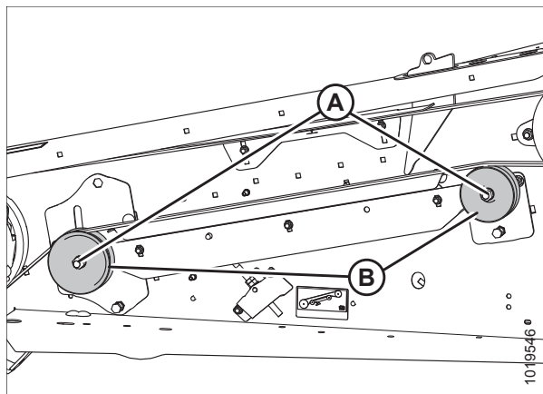
pav. 5.92: Kairiojo dalgio pavara
