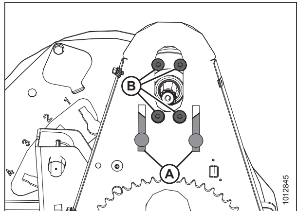
pav. 5.246: Lenktuvų pavaros variklio tvirtinimo angos
