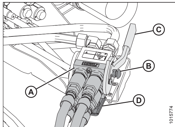
pav. 4.10: Dalgio / lenktuvų pavaros daugiaelementė jungtis
