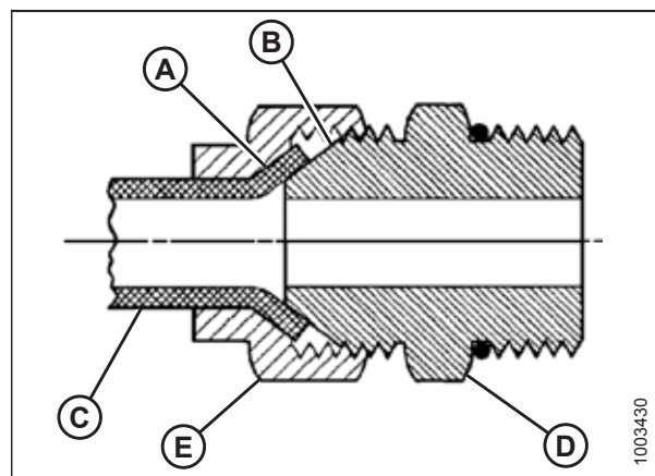
pav. 9.10: Hidraulinis tvirtinimo elementas
