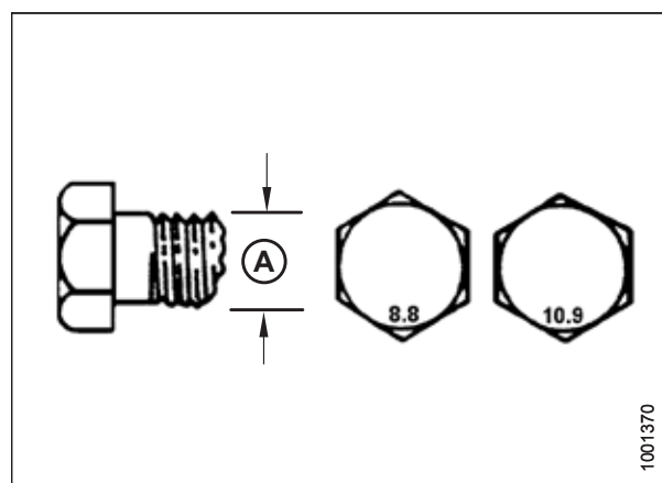
pav. 9.5: Varžtų klasės
