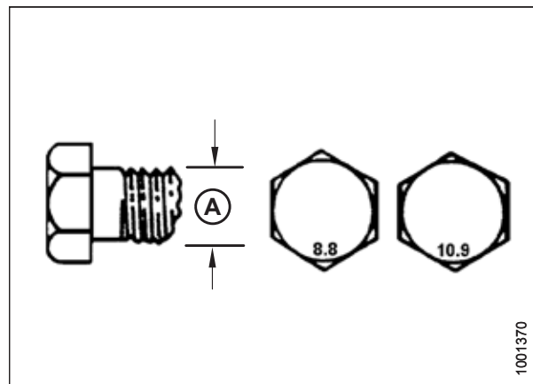
pav. 9.9: Varžtų klasės
