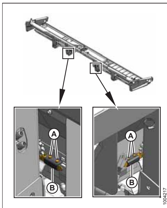
pav. 3.54: Vidiniai hidraulinio platformos poslinkio stabdikliai
