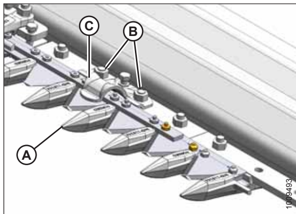
pav. 5.32: Smailios apsaugos
